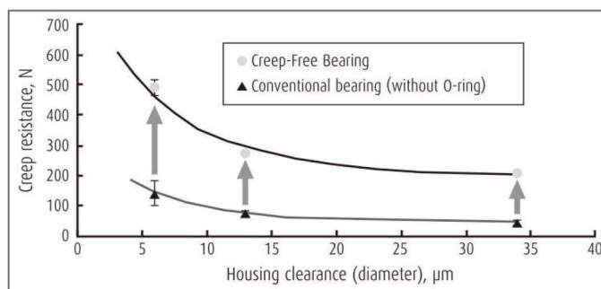
Fig. 2 Creep limit load test (example: 6204)
