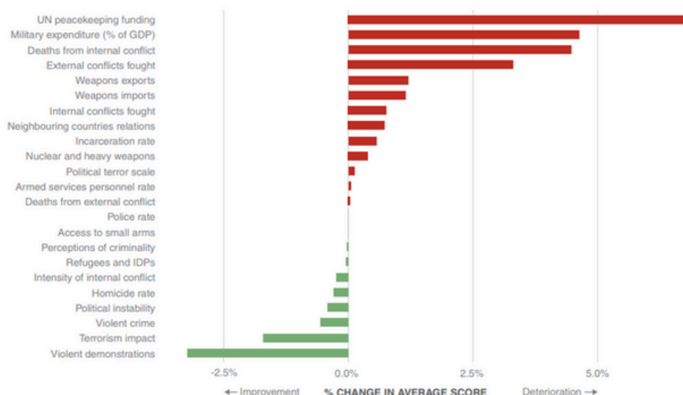
Figura 1 – Alteração percentual na pontuação do indicador de paz global, 2023-2024
