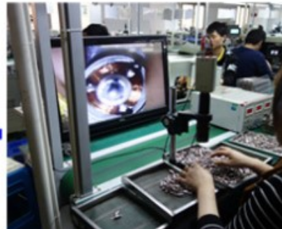
转子检测器
