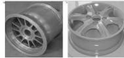
Şekil 15. AZ80 magnezyum tekerlek (A) Magnezyum alaşımlı dövme (Nguyen, 2017), (B) Ekstrüde edilmiş Mg alaşımlı tekerlekler (14×6) J (Liu, 2023)
