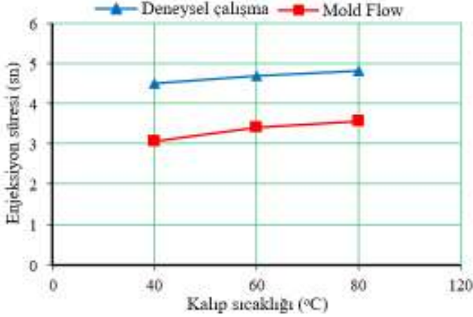
Şekil 13. 200 °C ergimiş plastik sıcaklığı için hoparlör, lamba ve ikaz düğme yuvası elemanında kalıp sıcaklığına bağlı olarak enjeksiyon sürelerinin değişimi
