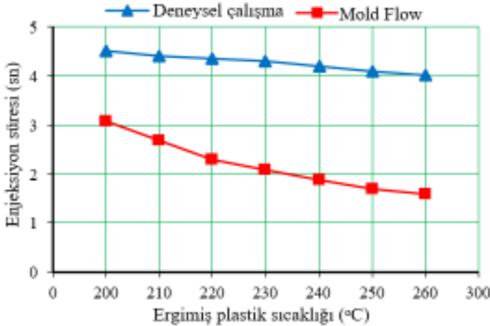
Şekil 10. 40 °C kalıp sıcaklığı için hoparlör, lamba ve ikaz düğme yuvası elemanında ergimiş plastik sıcaklığına bağlı olarak enjeksiyon sürelerinin değişimi
