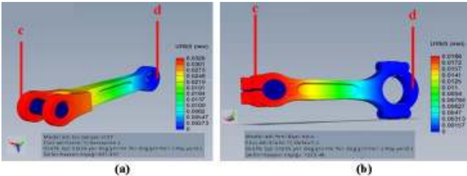
Şekil 12. Commer TS3 dizel motorunda kullanılan ve DIN St37-2 çeliğinden imal edilmesi düşünülen (a) orijinal ve (b) tasarlanan biyel kollarının Y-şekilli ayak kısmındaki iki yuva deliğine pim geçirilerek orta kısmından statik yük uygulanarak gerçekleştirilen sanal çekme deneyi sonucunda oluşan şekil değiştirme değerleri
