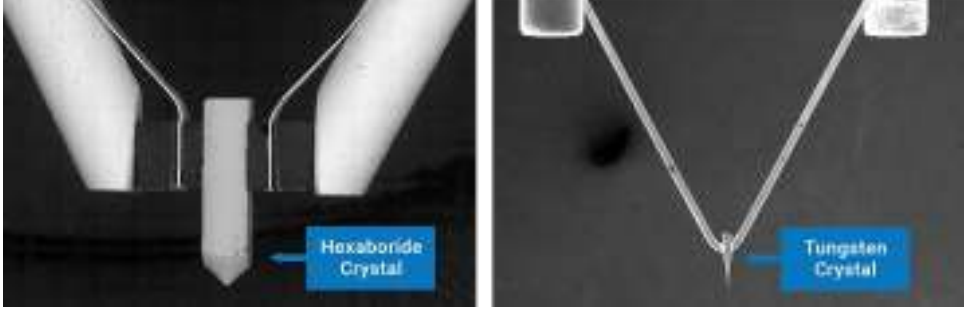
Şekil 1.2 Termiyonik elektron kaynağının (sol) ve Phenom Pharos'un alan emisyon tabancasının (sağ) SEM görüntüleri, elektronların yayıldığı uç malzemesini göstermektedir.
