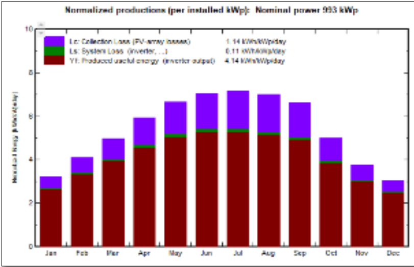
Şekil 9. Normalize edilmiş üretim ve sistem kayıp değeriğerlerinin aylara göre değışimi
