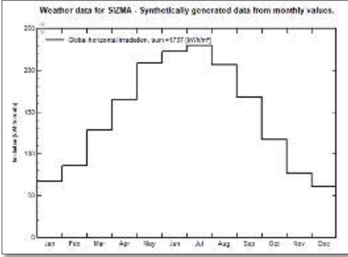
Şekil 6. Seçilen lokasyon için aylara göre ışınlm şiddetinin değışimi
