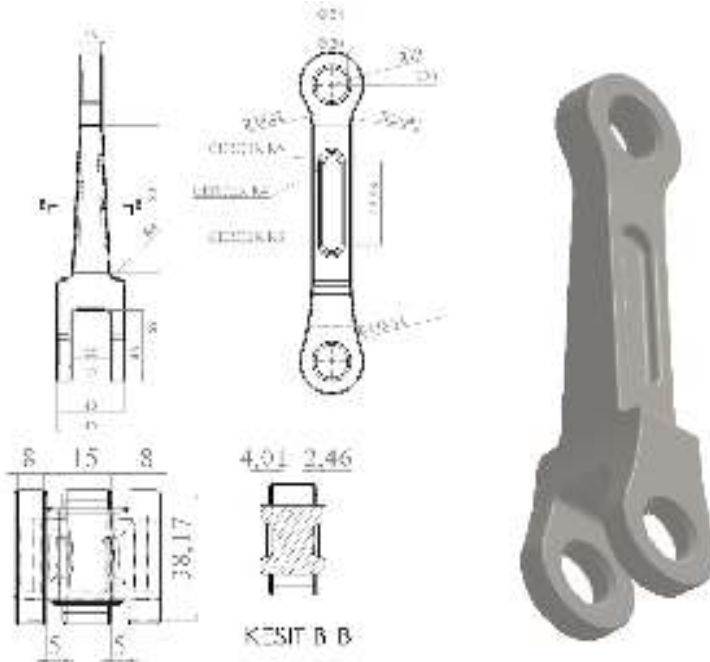
Şekil 5. “Commer TS3” motorunda kullanılan orijinal Y-şekilli biyel kolunun teknik resim çizimi ve üç boyutlu görüntüsü.
