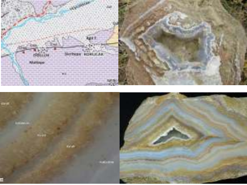
Şekil 6. Tokat İli Döller ve Gümenek Bölgelerindeki Kalsedon Oluşumları (Arık ve Ruşen, 2022).
