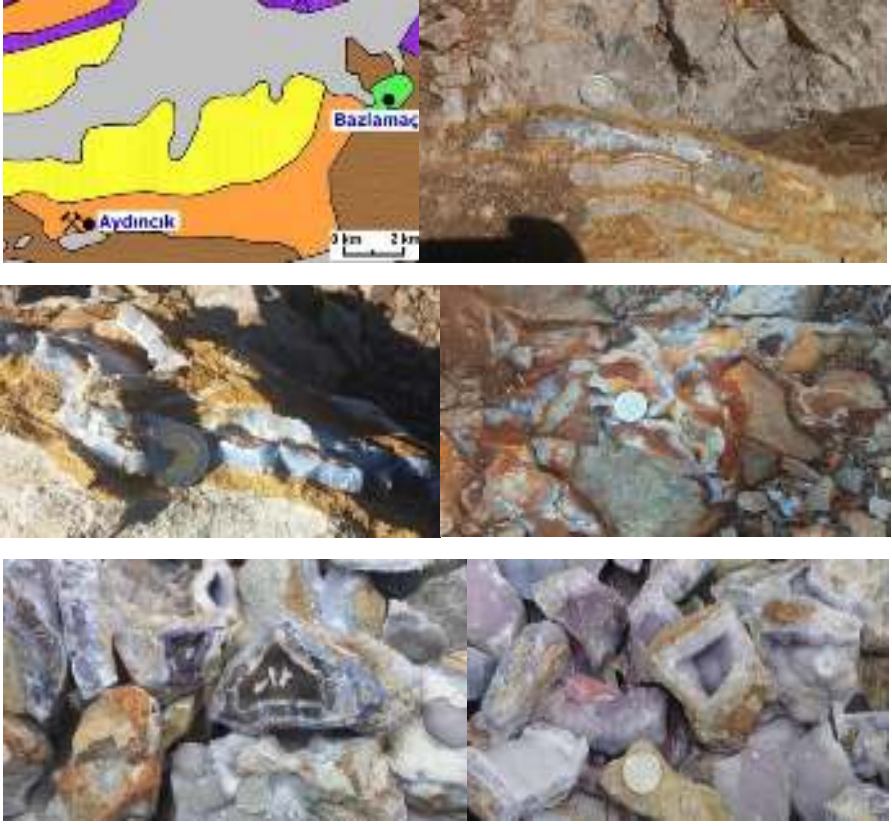
Şekil 10. Yozgat Aydıncık Bölgesindeki Kalsedon Oluşumları (Kaydu Akbudak vd., 2018).
