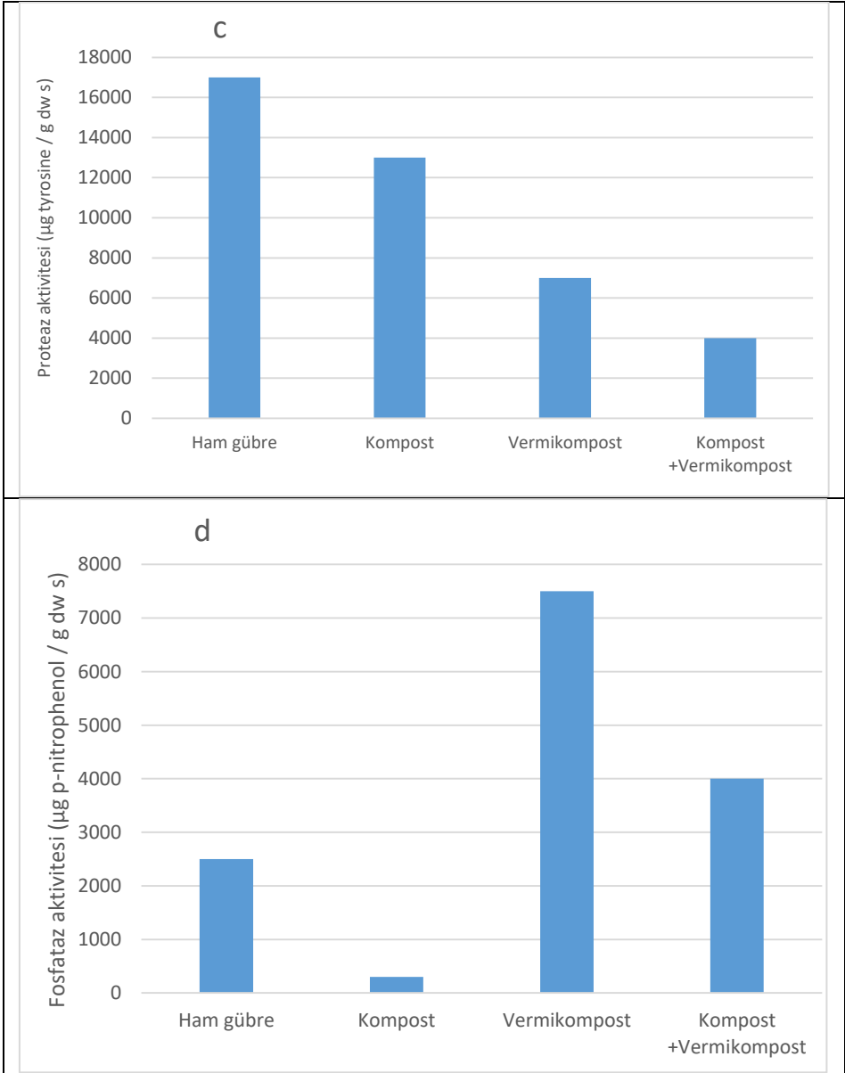
Şekil 5. (a) Dehidrogenaz aktivitesi, (b) \beta glukozidaz aktivitesi, (c) Proteaz aktivitesi, (d) Ham sığır gübresindeki fosfataz aktivitesi, kompostlamanın aktif fazı, Solucan gübresi ve aktif fazın sonuna kadar kompostlama artı solucan gübresi (Kompostlama + Solucan gübresi)
