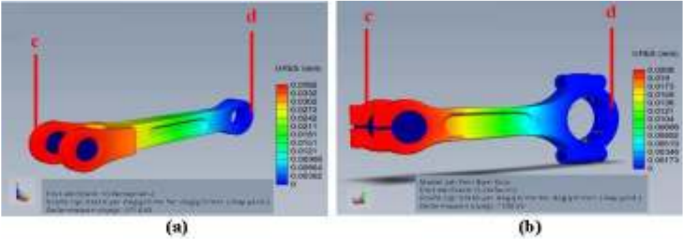
Şekil 14. Commer TS3 dizel motorunda kullanılan ve AISI 304 östenitik paslanmaz çelikten imal edilmesi düşünülen (a) orijinal ve (b) tasarlanan biyel kollarının Y-şekilli ayak kısmındaki iki yuva deliğine pim geçirilerek orta kısmından statik yük uygulanarak gerçekleştirilen sanal çekme deneyi sonucunda oluşan şekil değiştirme değerleri
