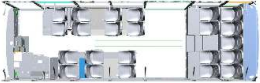
Şekil 3.1. M2 Kategorisinde bulunan Atak Class II aracının koltuk lay-outu
