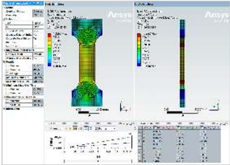
Şekil 32. 20 Aspect ratio numune için eşdeğer gerilme (Von Mises) dağılımı sonucu.
