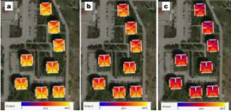
Şekil 7: Sonbahar mevsiminde çatı üstü güneş fotovoltaik potansiyelinin mekânsal dağılımı (a) Eylül; b) Ekim c) Kasım)
