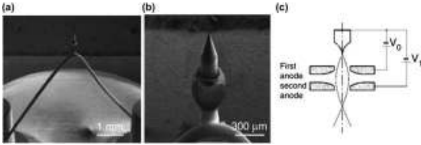
Şekil 1.4 FESEM genel şeması (üstte) (a) Sivri uçlu FEG, (b) ucun yüksek büyütmeli görüntüsü ve (c) FEG çalışma prensipleri (Zhou et al. 2007).
