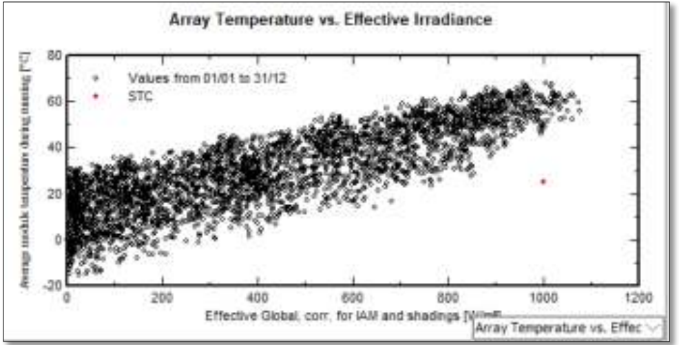
Şekil 8. Dizi sıcaklığı ile ışınlm şiddeti değışiminin değışimi
