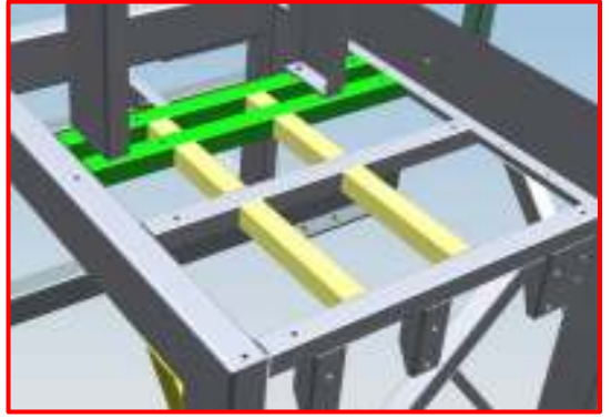
Şekil 3.29. 2.Mock-Up Koltuk Bağlantısı
