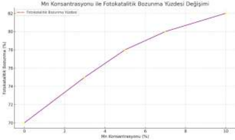
Şekil 3. ZnO-TiO 2 çekirdek-kabuk nanokompozitlerin farklı Mn konsantrasyonlarının (%0, %3, %5, %7, %10) fotokatalitik aktivite üzerindeki etkisi
