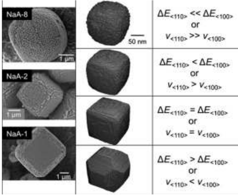
Şekil 1.11 NaA-1, -2 ve -8'in HRSEM görüntüleri ve \langle 100 \rangle ve \langle 110 \rangle boyunca bağıl hız artışı ile kaba taneli simülasyon yoluyla morfolojik tanımlama.(Cho et al. 2011)
