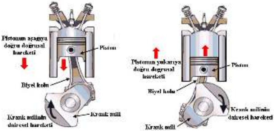
Şekil 2. Geleneksel biyel kolunun çalışma prensibi.
