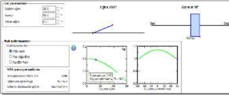
Şekil 5. Azimut açısı değeri 90° (üretim senaryosu-2)
