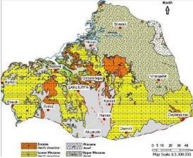
Şekil 2. Şanlıurfa jeoloji haritası (Akbaş vd. 2002)
