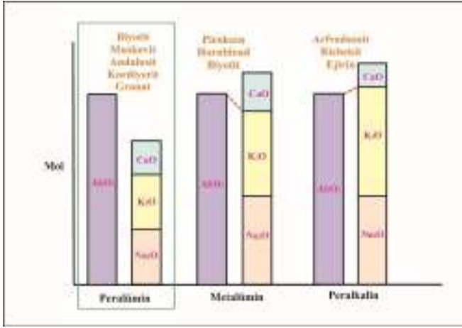
Şekil 2.3. S tipi granitoidlerin kimyasal sınıflaması (Shand, 1927; Clarke, 1992)
