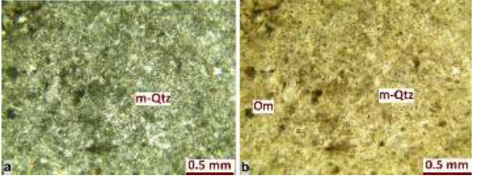
Şekil 7. İnceleme sahasındaki çörtlere ince kesit görüntüleri, m-Qtz: Mikrokristalin kuvars, Om: Opak mineral (a: Çift Nikol ; b: Tek Nikol).
