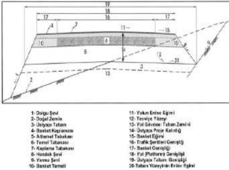
Şekil 1. Yol Üstyapısı Tip Enkesiti (KGM, 2008)
