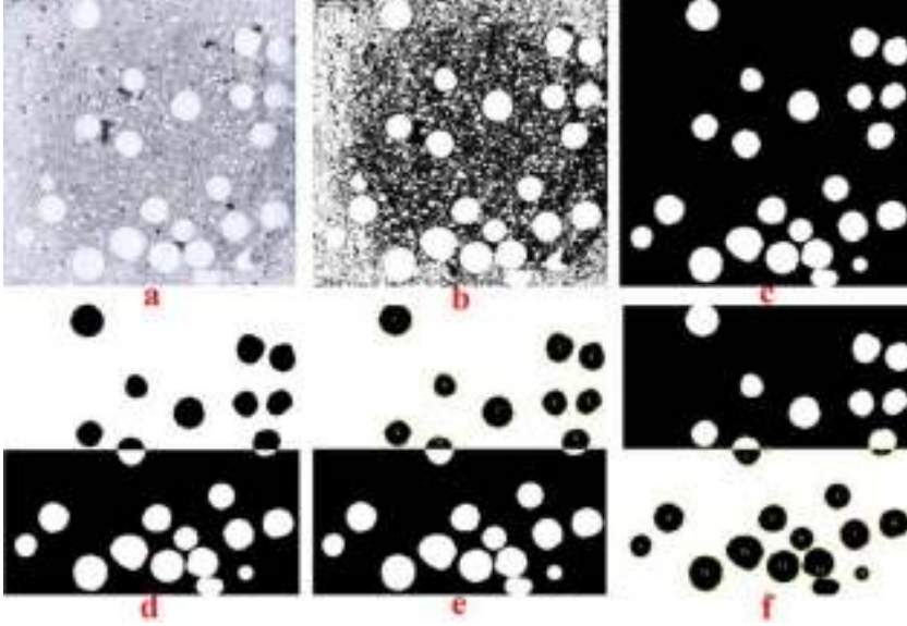
Şekil 7. Görüntü işleme aşamaları, a) Piksellerin gerçek ölçeğe dönüştürülmesi, b) Threshold uygulaması, c) Morfolojik filtre uygulaması, d) Siyah-Beyaz görüntünün tersine çevrilmesi, e) Üst bölüm analiz işlemi, f) alt bölüm analiz işlemi.
