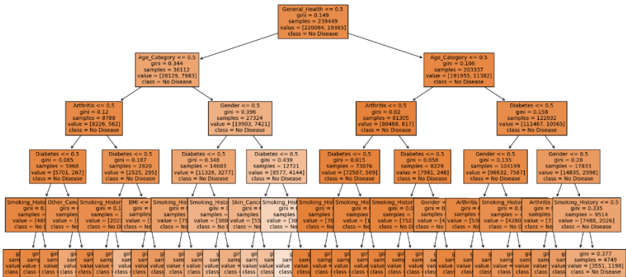
Şekil 1. Karar Ağacı
