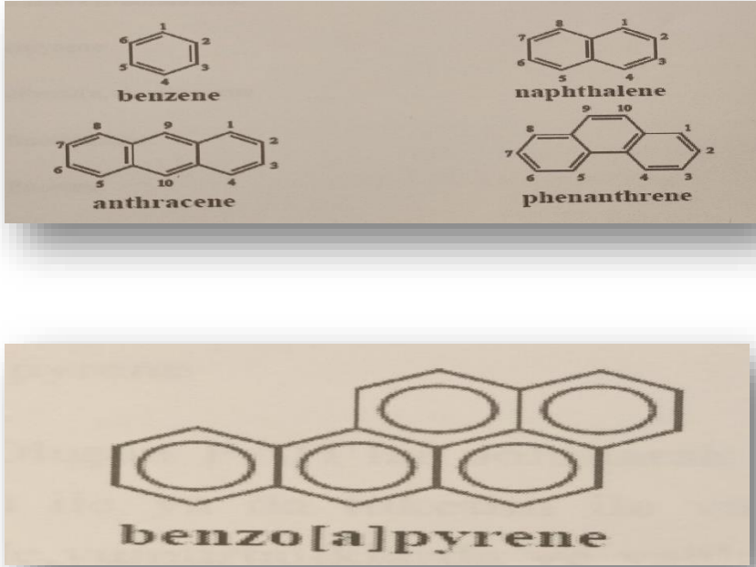
Şekil 2. Benzen formundaki karbon ve hidrojen içerikli çok halkalı bileşik
