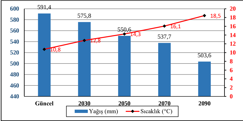
Şekil 2. Türkiye’de Yıllık Ortalama Sıcaklık (°C) ve Yıllık Toplam Yağış Değerlerinin (mm) Zamansal Değişimi (Günümüz-2100)
