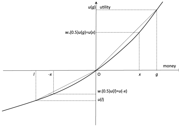
Şekil 1. Beklenti Teorisi
