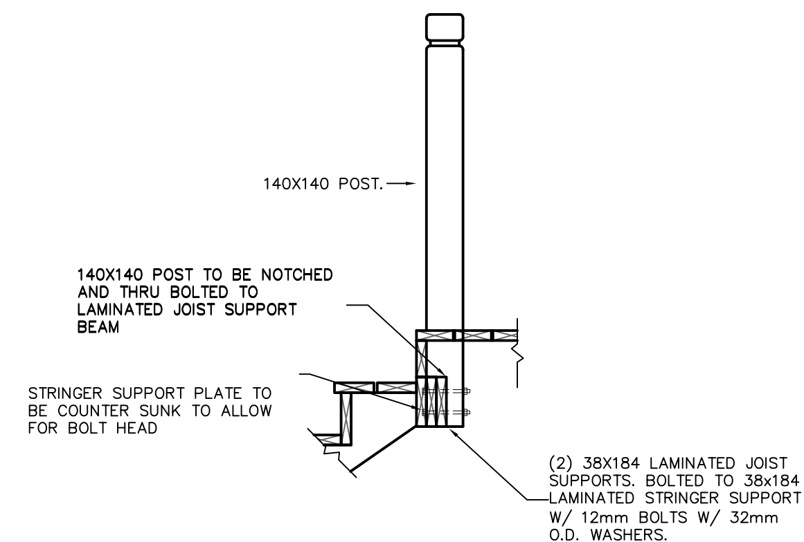
6 DETAIL 'B' SCALE: NTS
