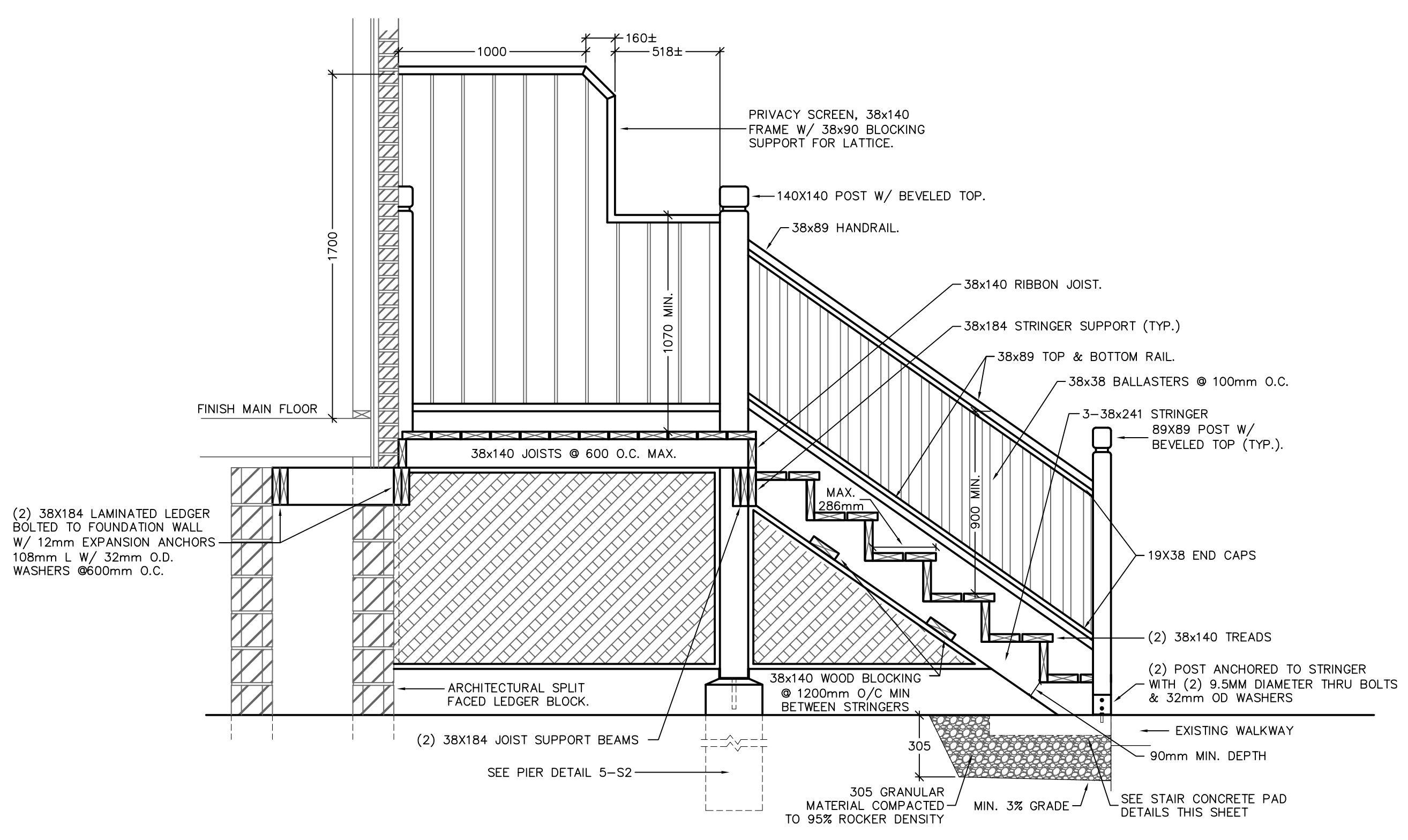
3 SECTION - SCALE: 1:20
