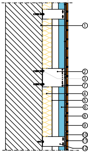
DÜŞEY KESİT
