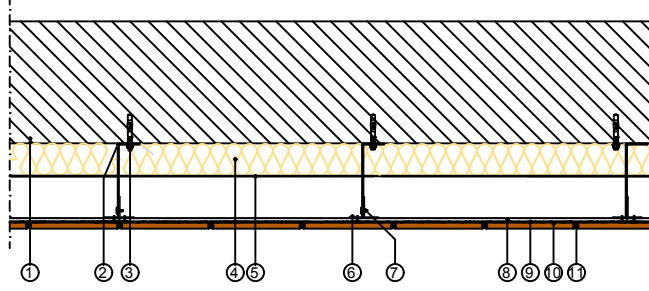
YATAY KESİT
