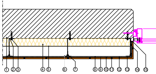
PENCERE KENARI PLAN DETAYI
