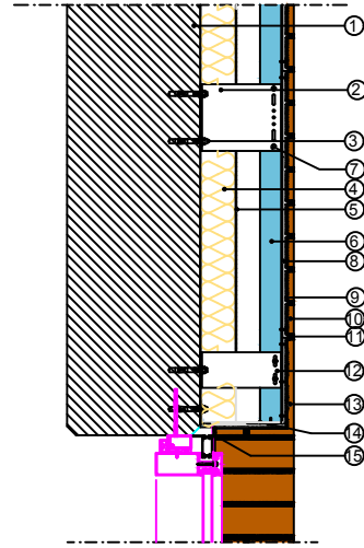
PENCERE ÜST BİTİM DETAYI
