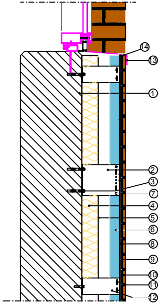
PENCERE ALT BİTİM DETAYI
