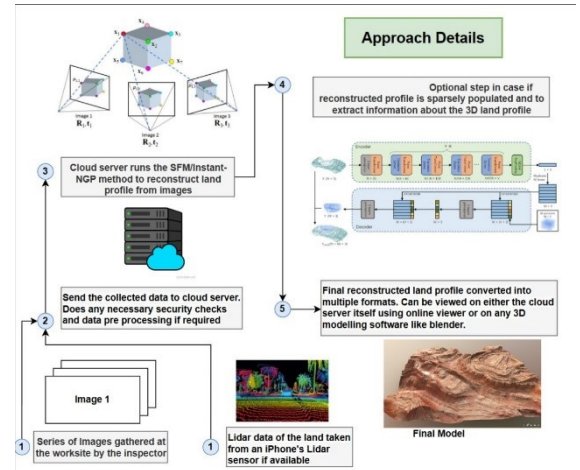
Fig. 1. SFM.
