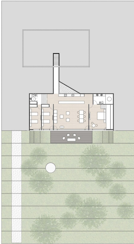
PLANTA CASA
