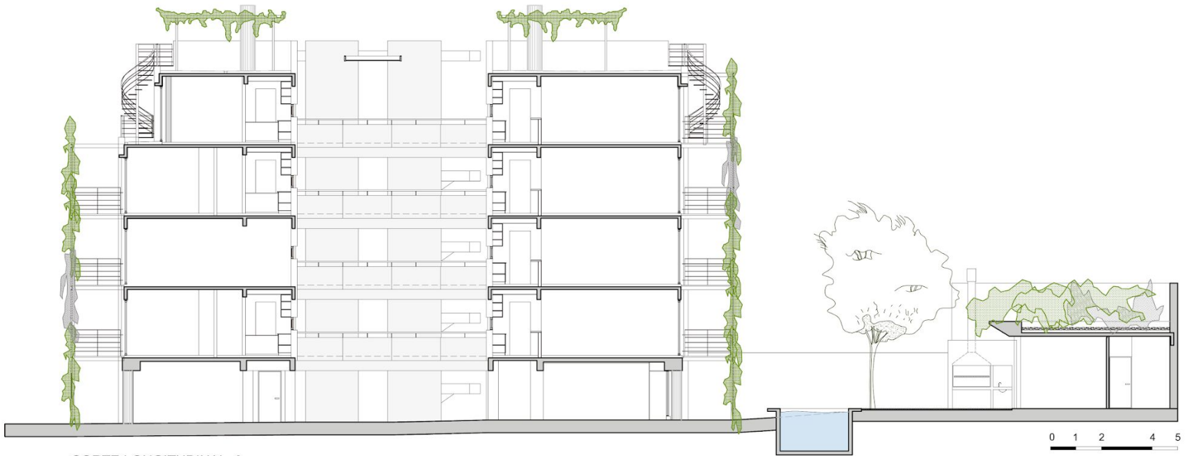
CORTE LONGITUDINAL A
