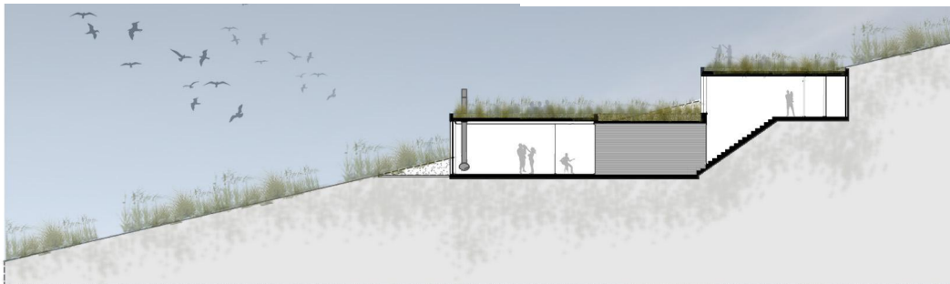
CORTE LONGITUDINAL
