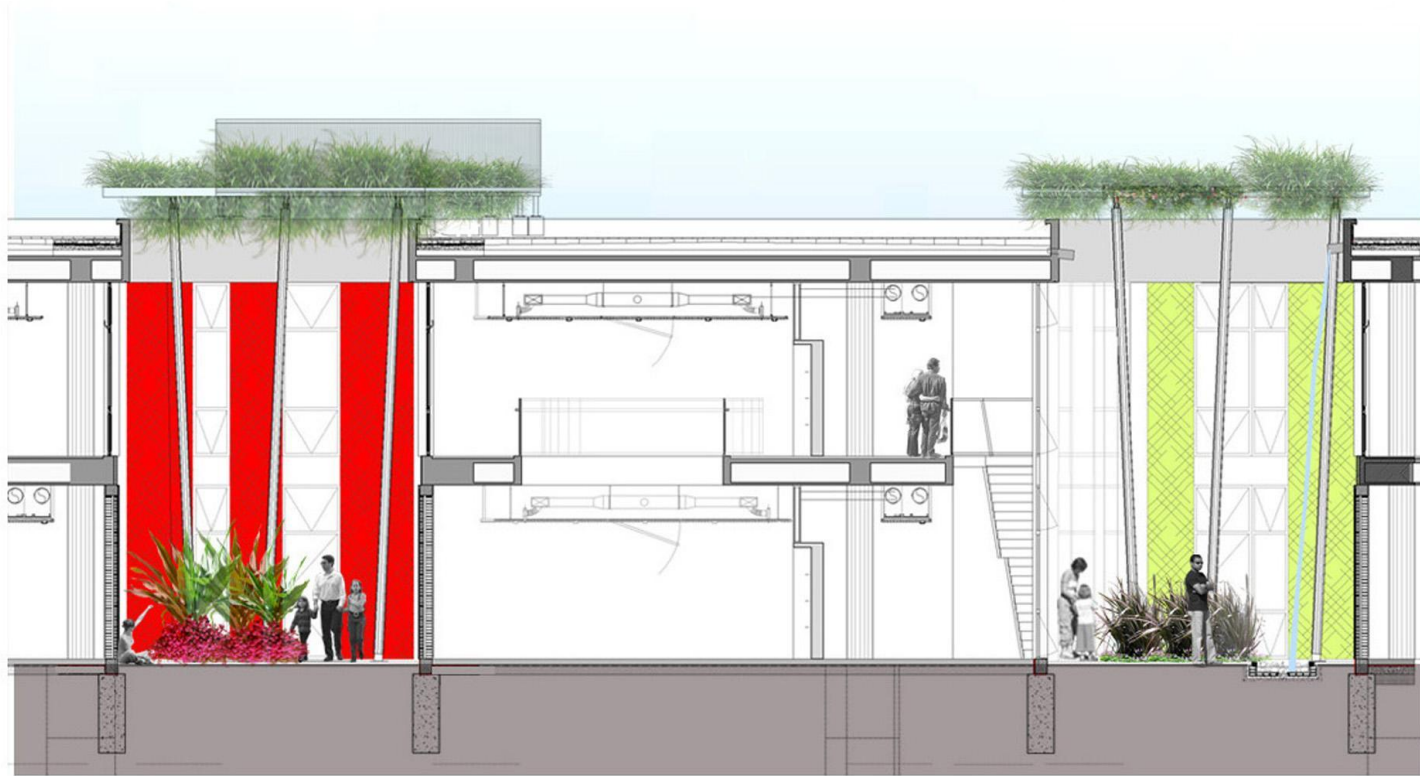
CORTE POR PATIOS
