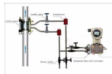
Orifice Flow Meter
