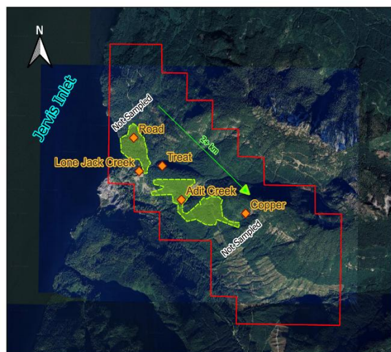
Jervis Property (Au-Ag-Cu-Zn)
