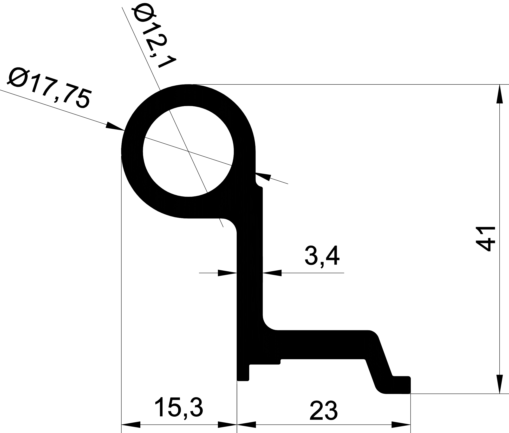
1463 0,819 Kg/m
