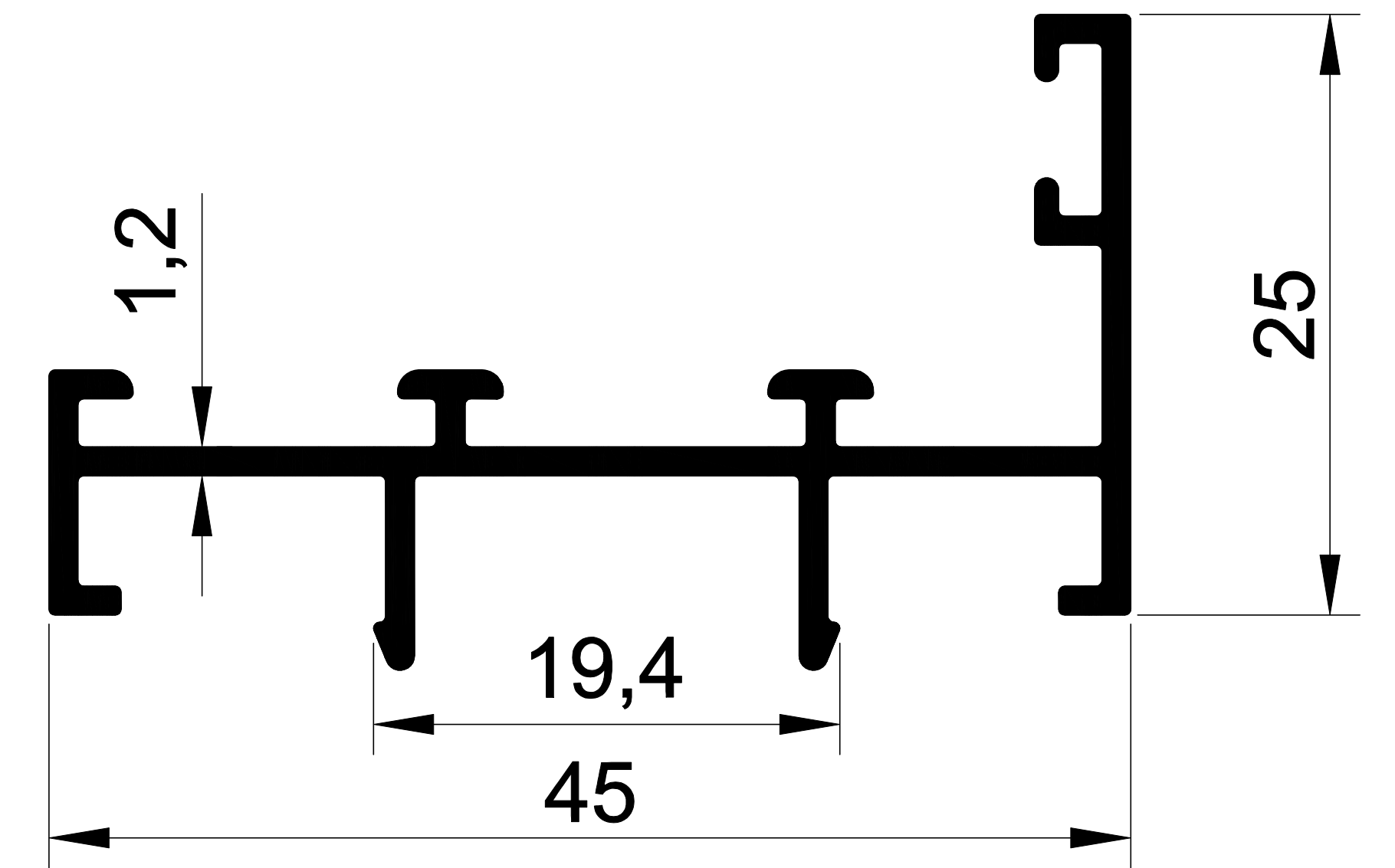
1378 0,392 Kg/m. 100'LÜK TUBA ADAPTÖR
