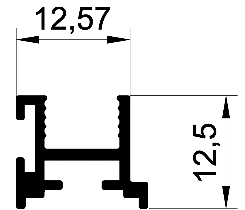
1169 0,152 Kg/m. SÜRME ÜST KANAT
