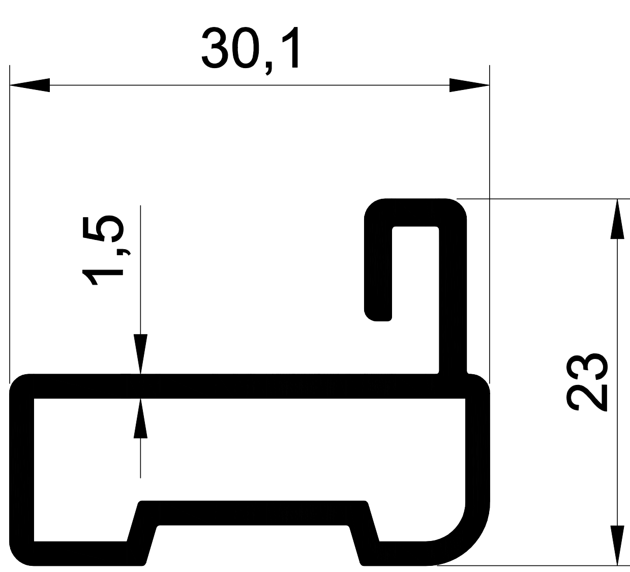
1210 0,422 Kg/m.
