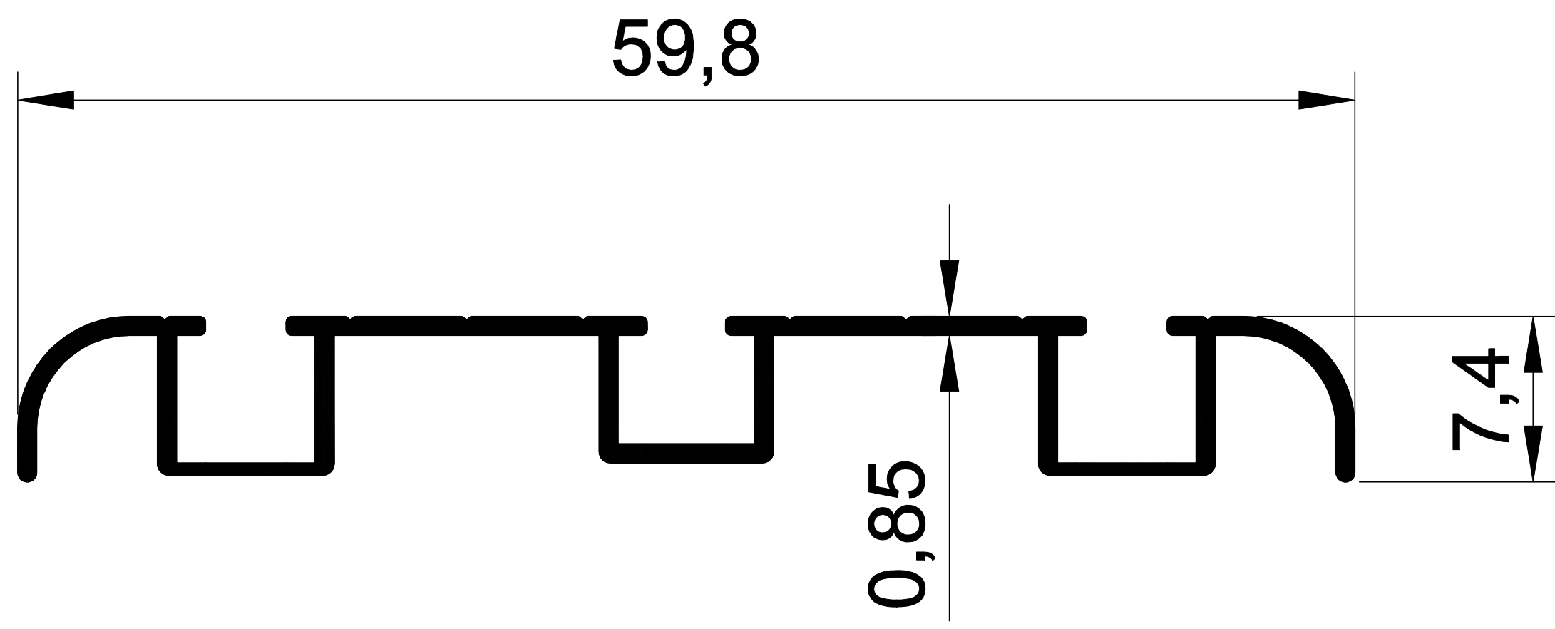
1311 0,249 Kg/m. 3'LÜ SÜRME EŞİKSİZ RAY
