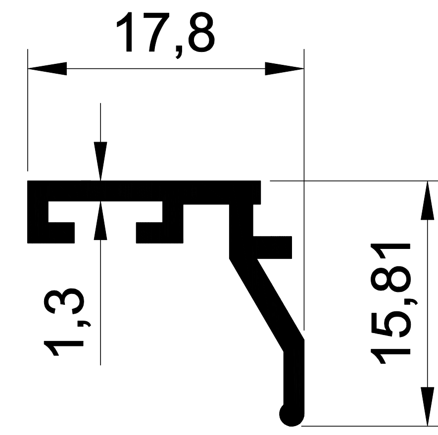
1192 0,154 Kg/m ISI CAM ÇİTASI
