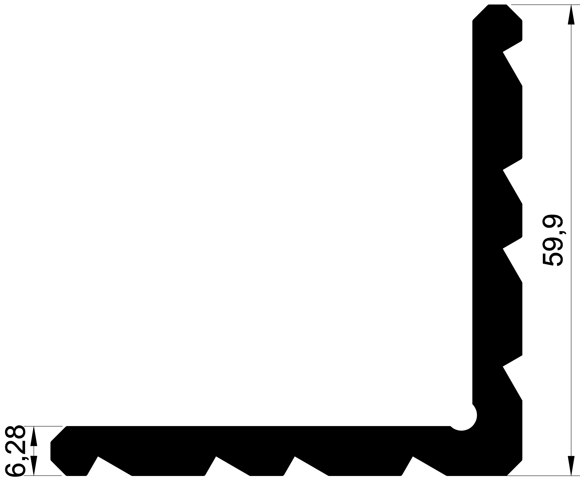
1401 1,748 Kg/m. 6 MM CEPHE KÖŞE
