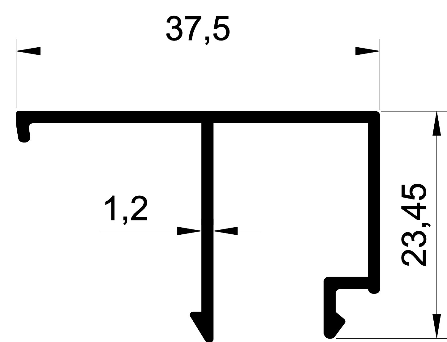
1203 0,298 Kg/m. SİSTEM TEK CAM ÇİTASI
