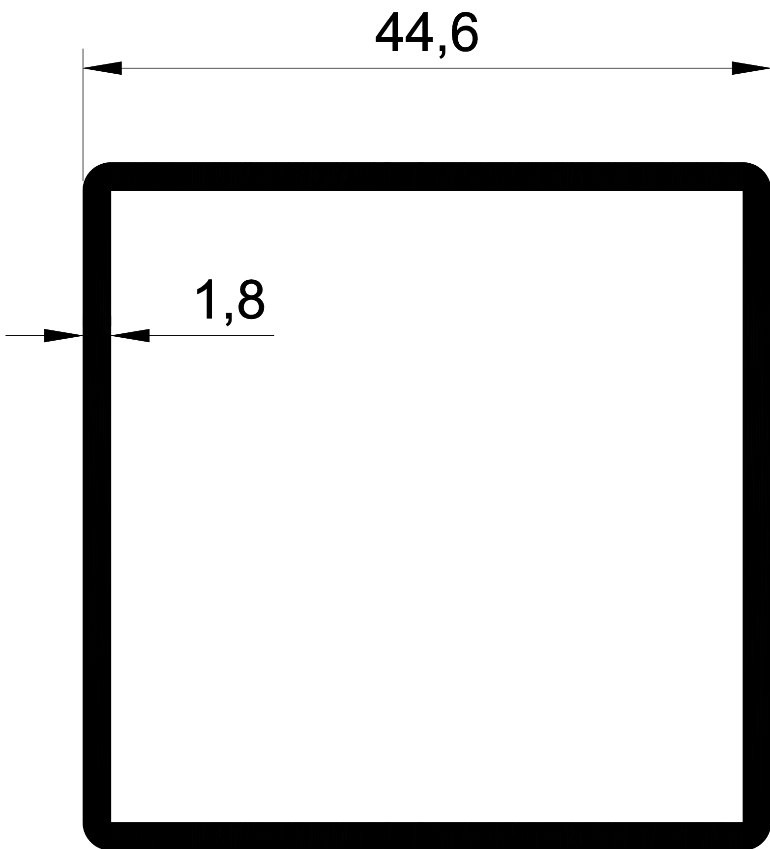
1049-C 0,828 Kg/m
