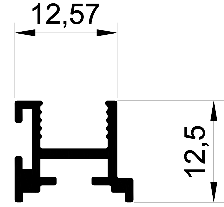
1169 0,152 Kg/m. SÜRME ÜST KANAT
