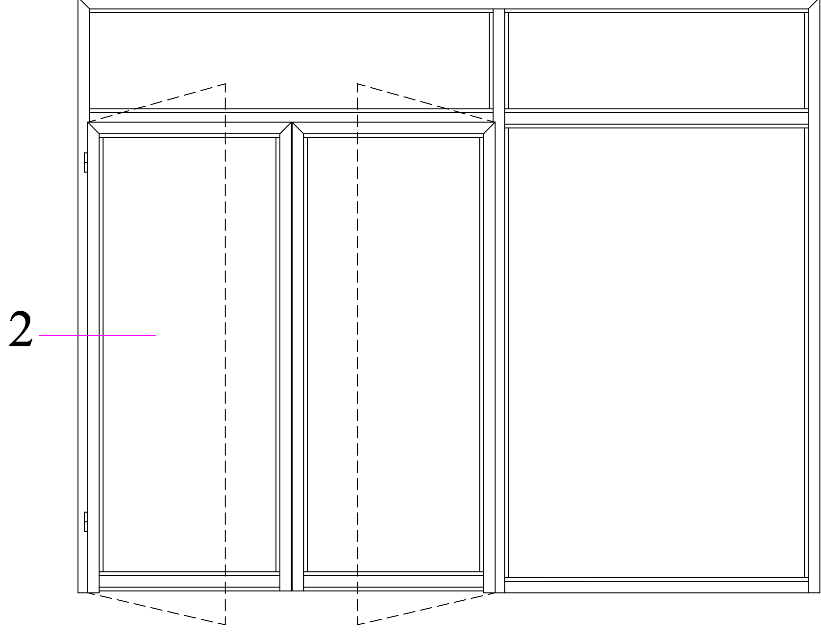
İÇE AÇILIR ÇİFT KAPI DETAYI
