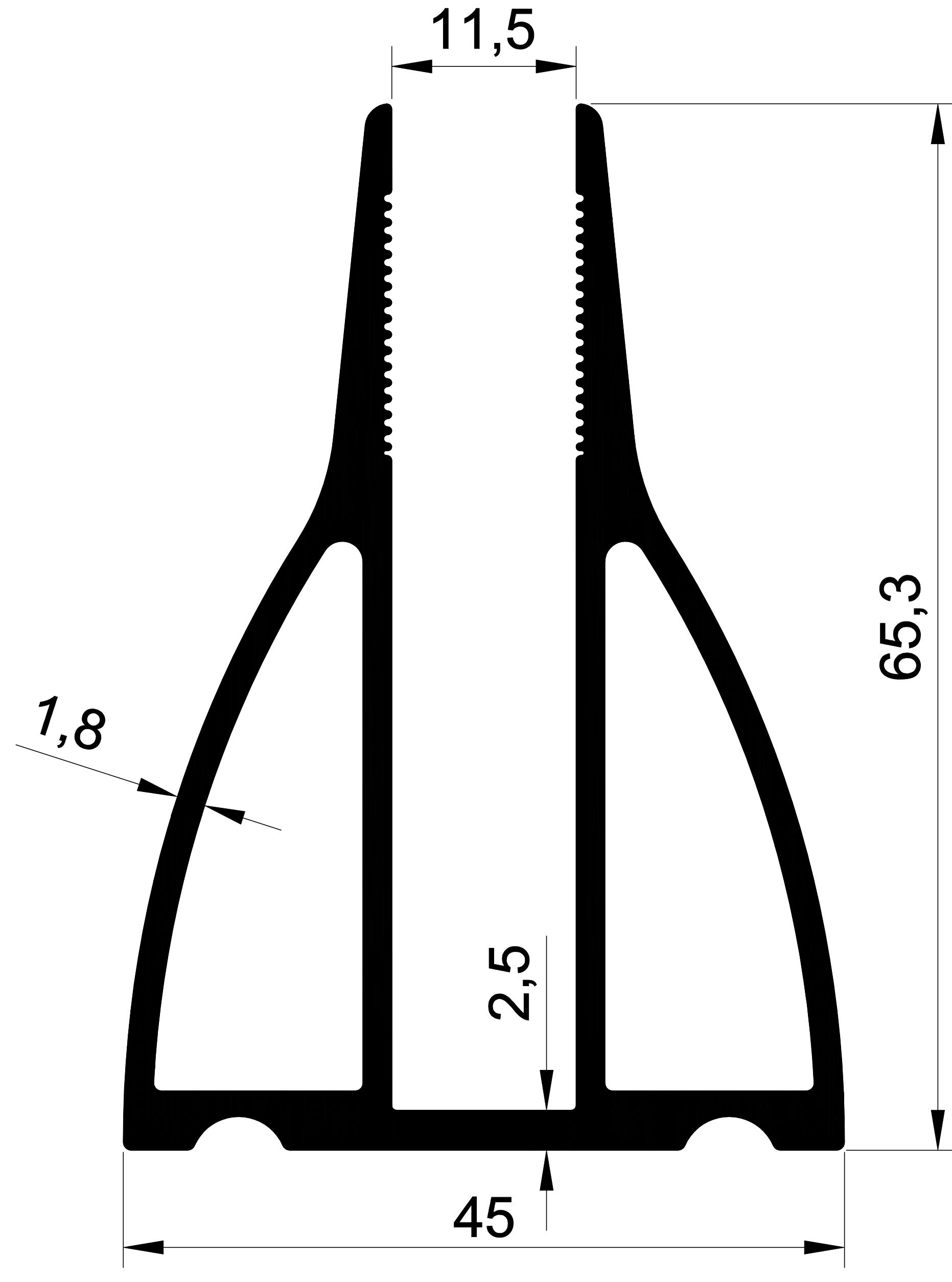
1428 1,482 Kg/m. 65 MM CAMLI KÜPEŞTE ALT BAZA ÇİFT TARAFLI
