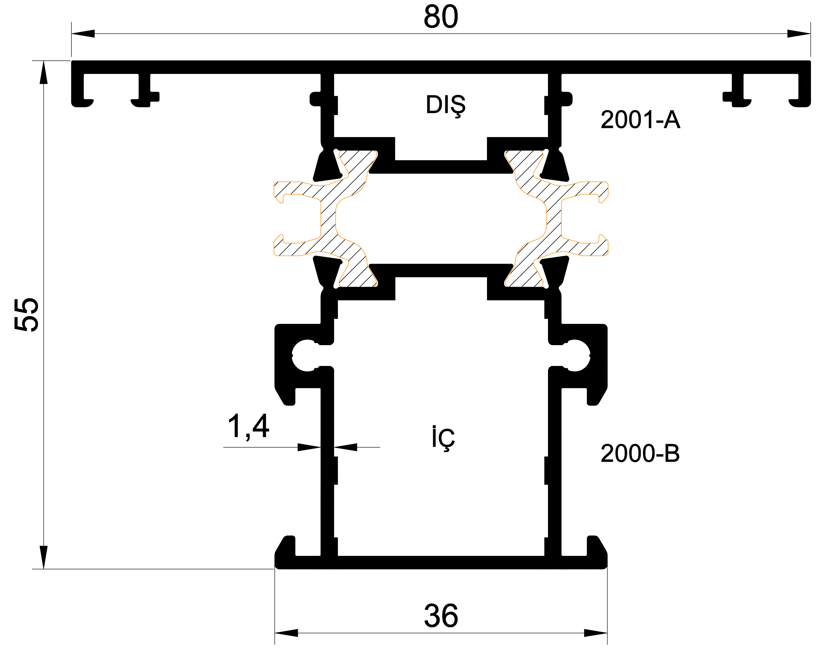
-55- 2001 1,283 Kg/m SİSTEM 55 ISI YALITIM ORTA
