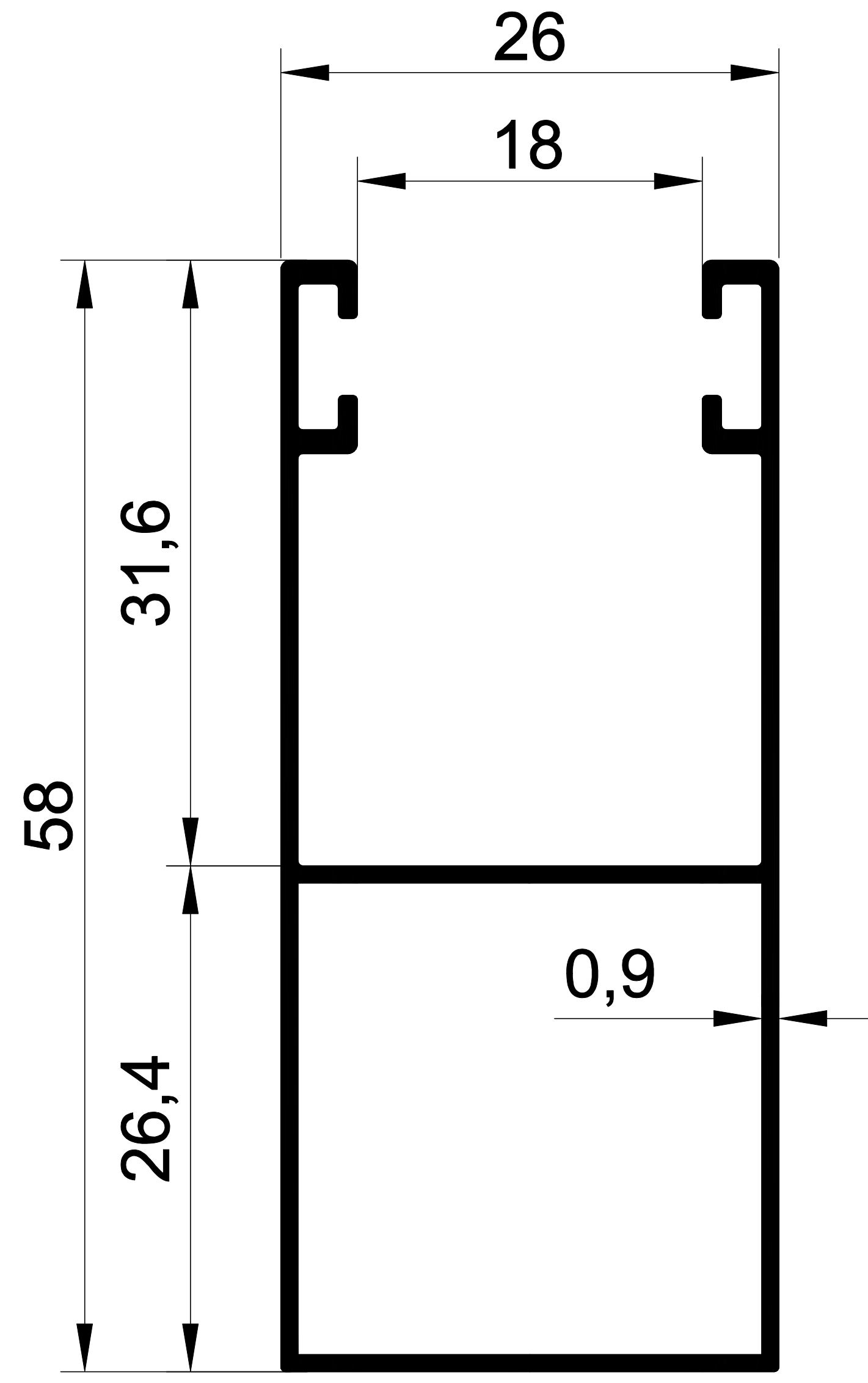
1340 0,461 Kg/m. 58'LİK DİKME
