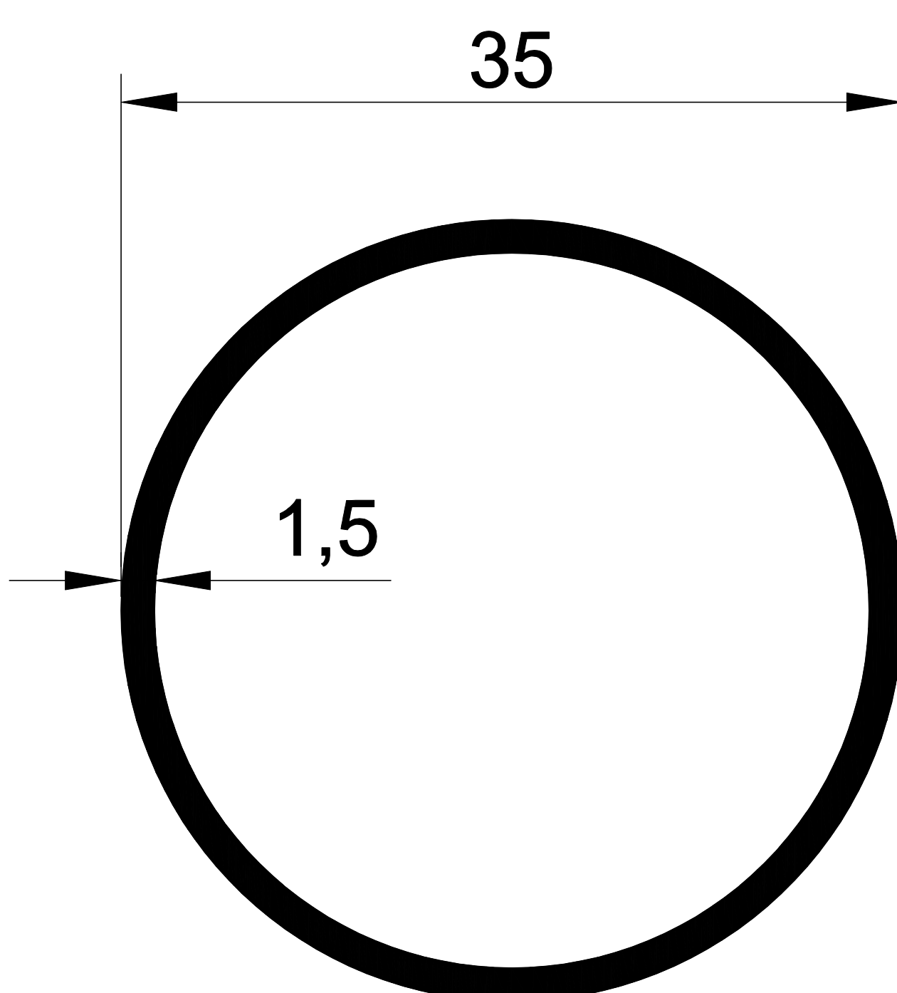
1070-C 0,420 Kg/m.
