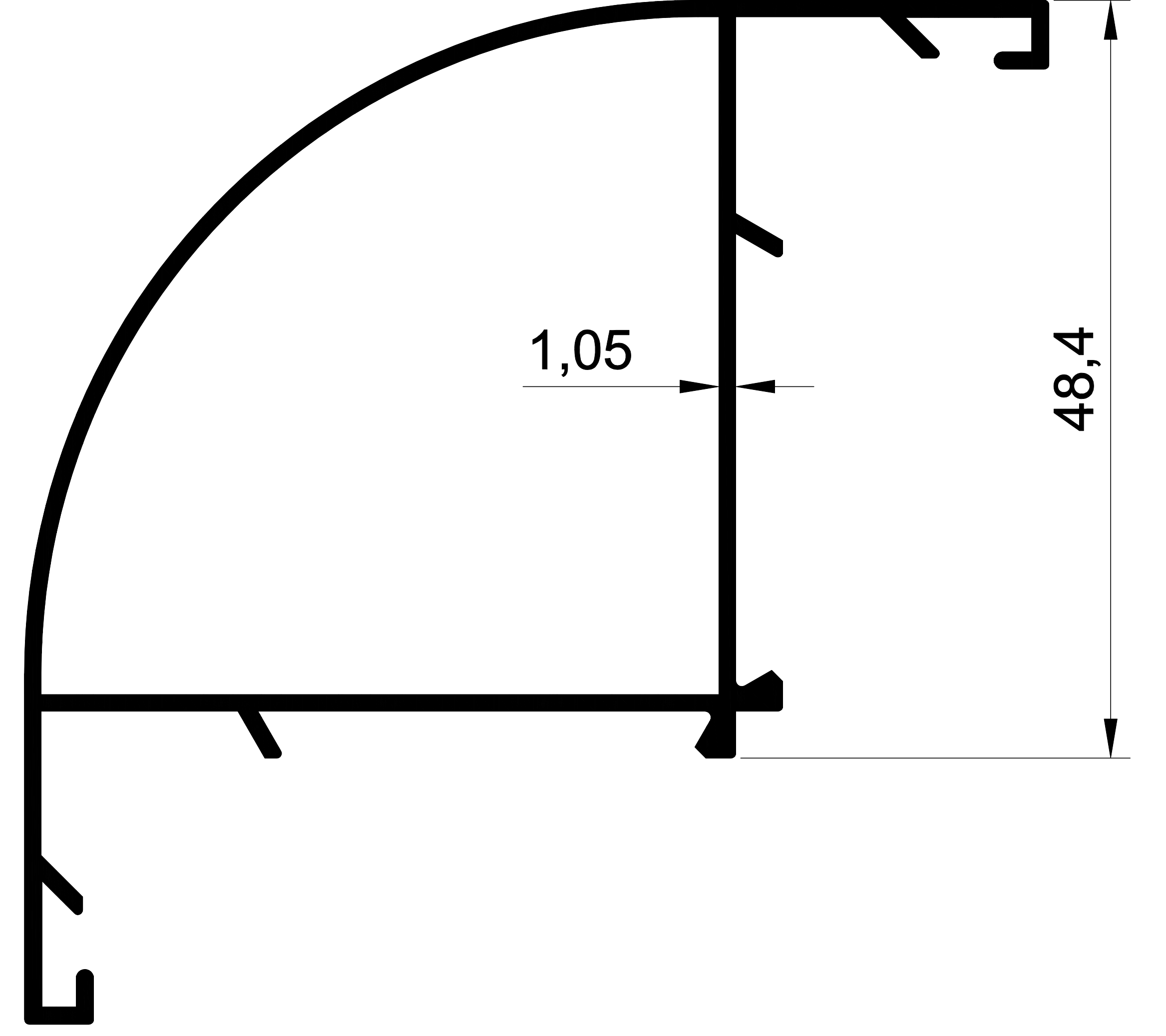
1100 0,677 Kg/m. ALDOKS OVAL KÖŞE DÖNÜŞ
