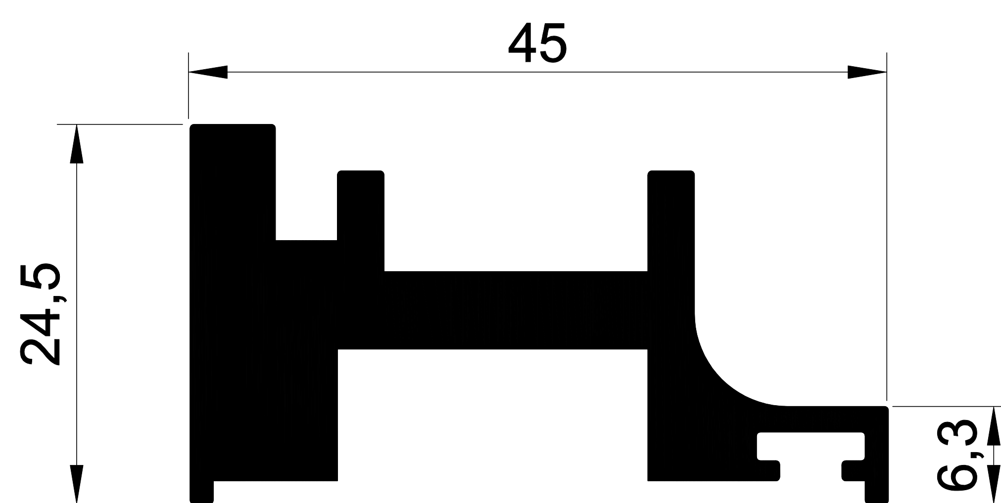
1223 1,140 Kg/m.
