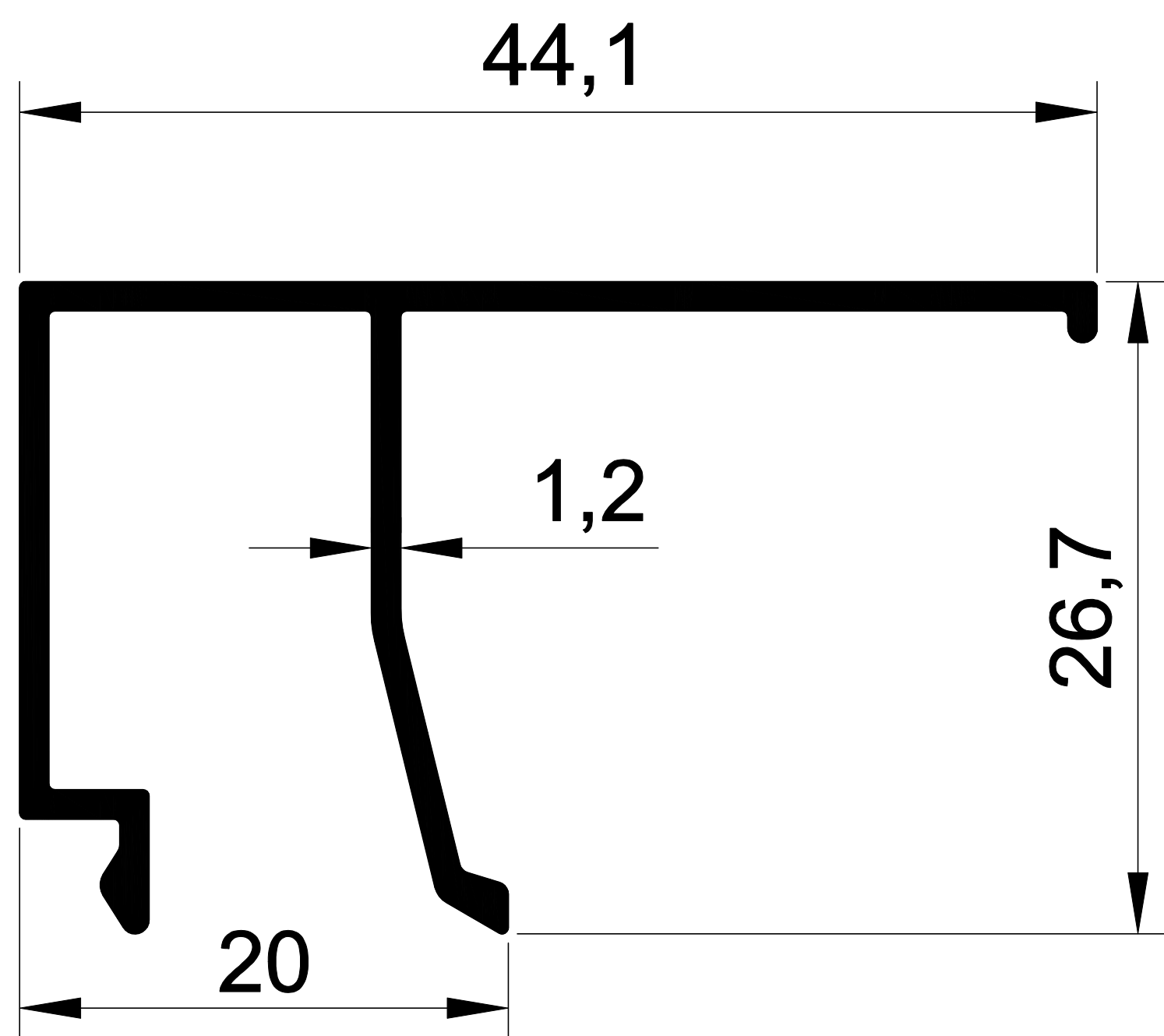
1405 0,336 Kg/m. BİM TEK CAM ÇİTASI
