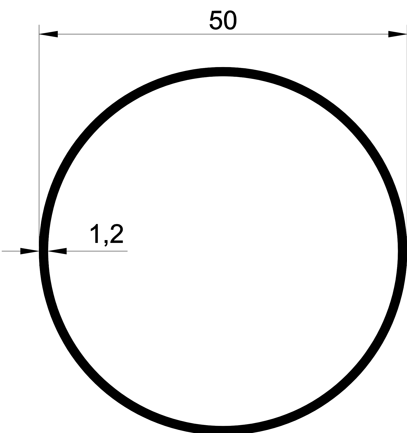
1344 0,493 Kg/m.
