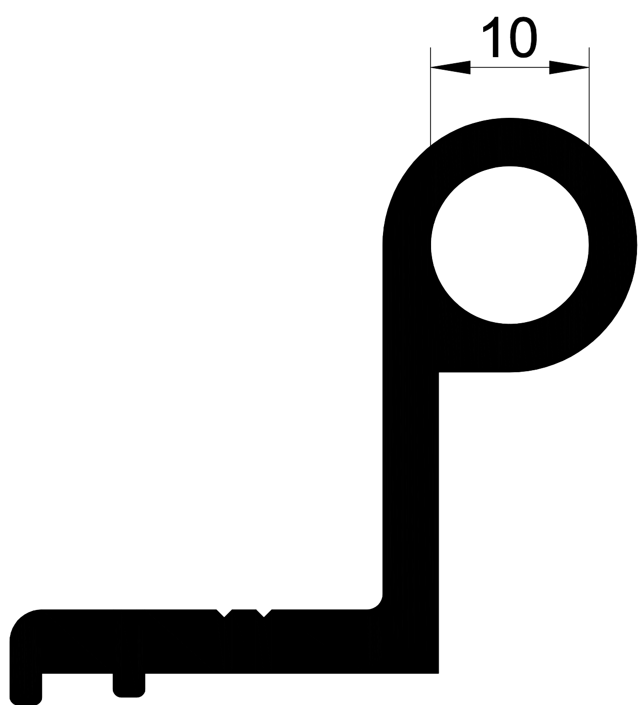
1230 0,818 Kg/m.
