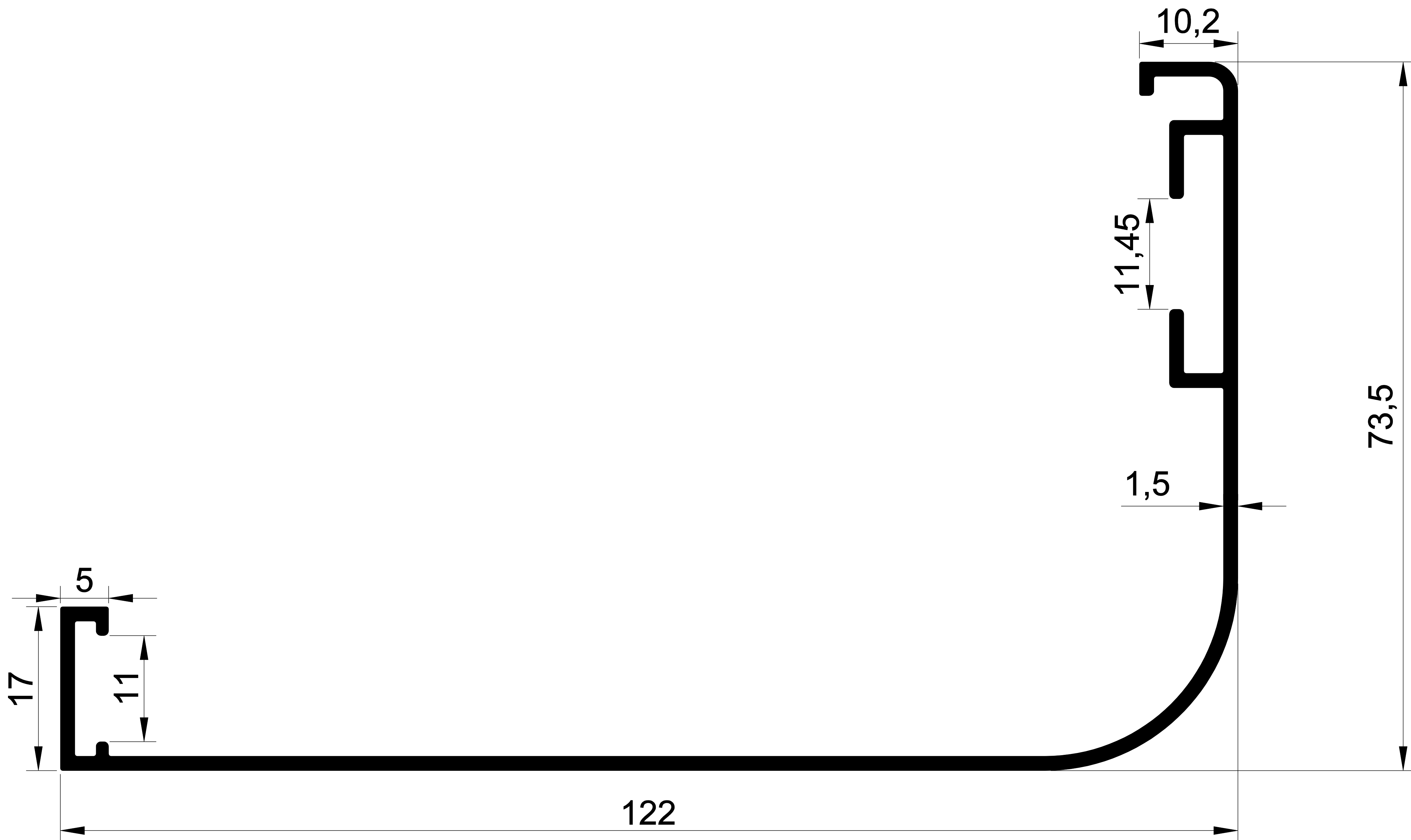
1424 0,980 Kg/m. MS-122'LİK PEERVAZ
