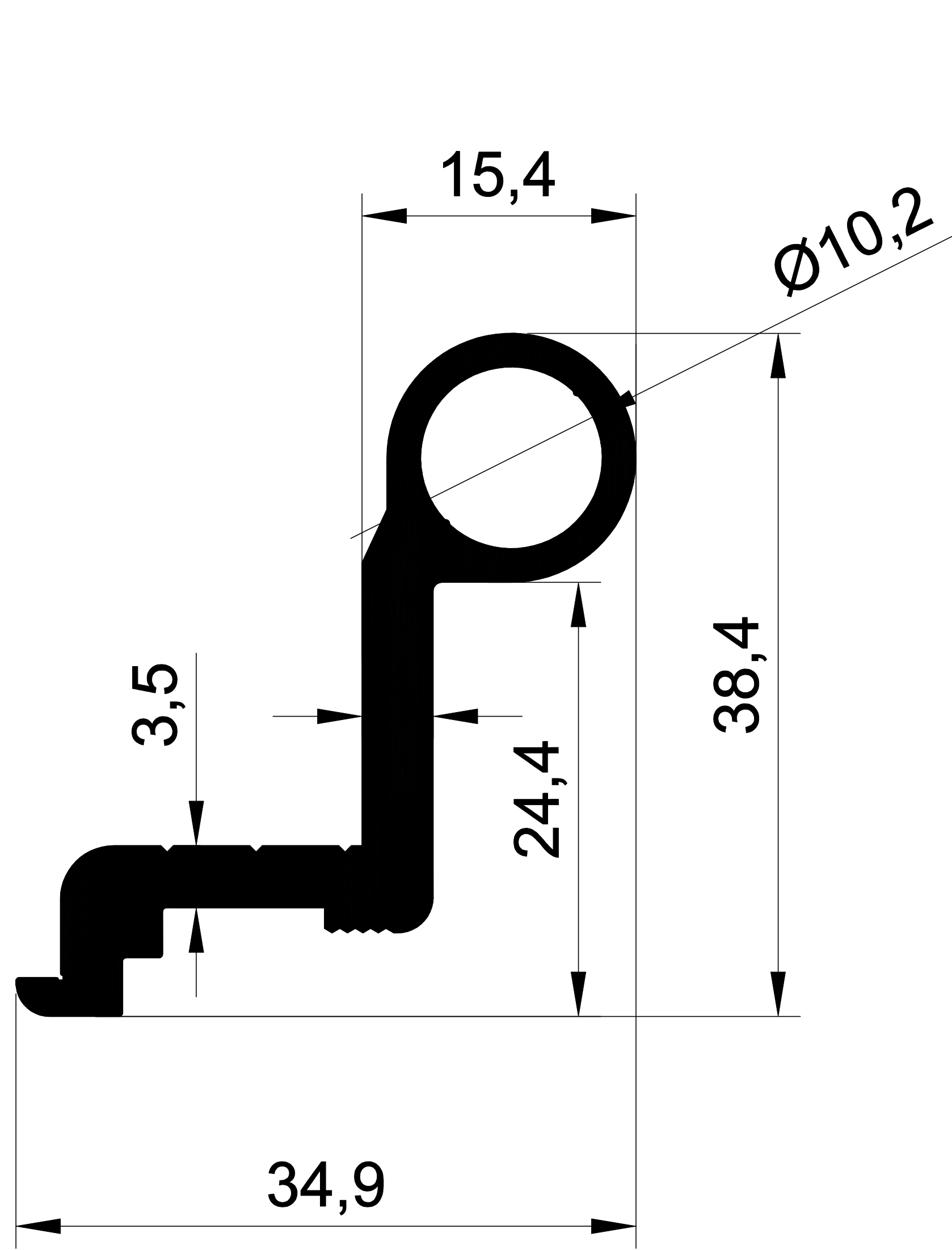
1006 0,694 Kg/m.
