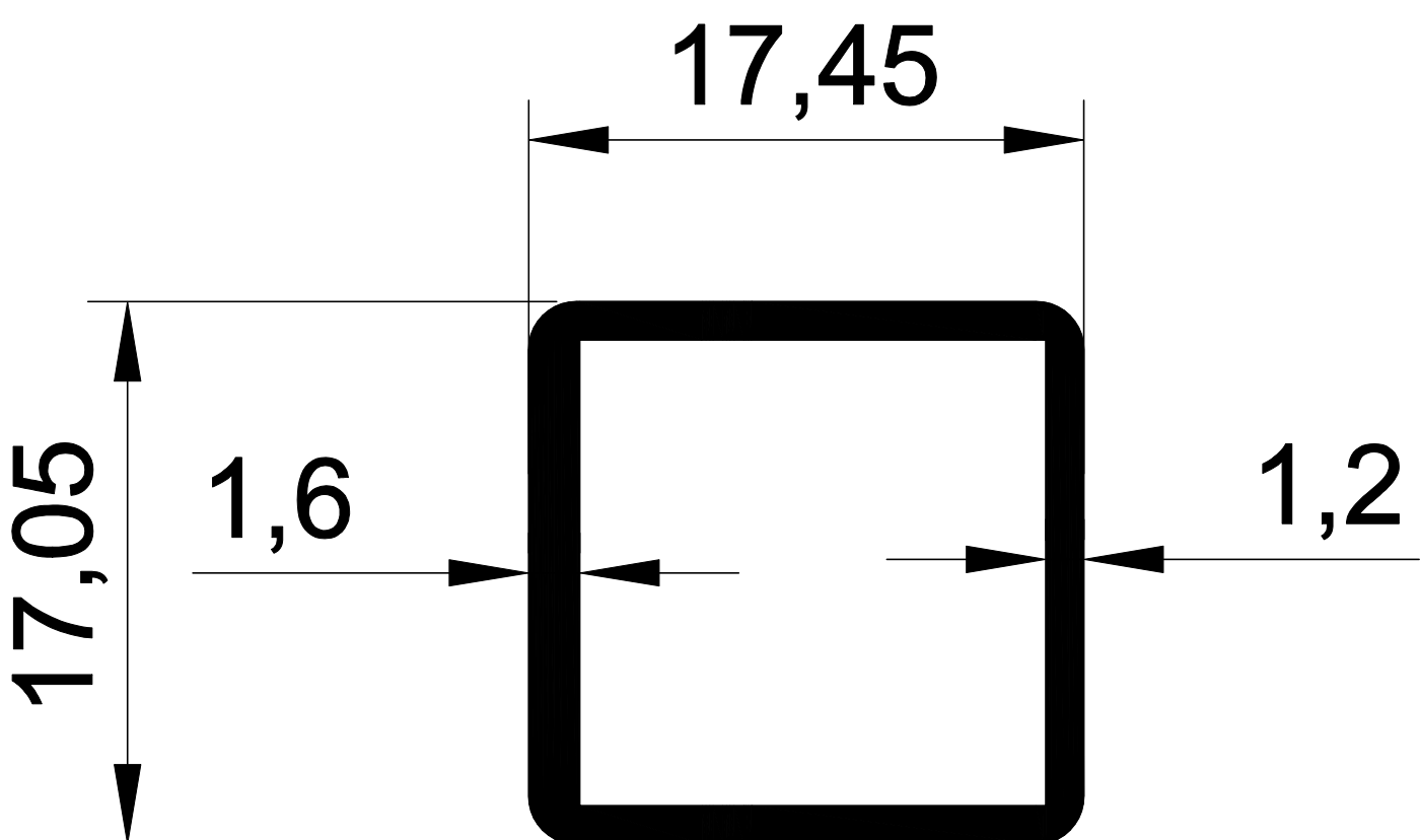
1324 0,220 Kg/m.
