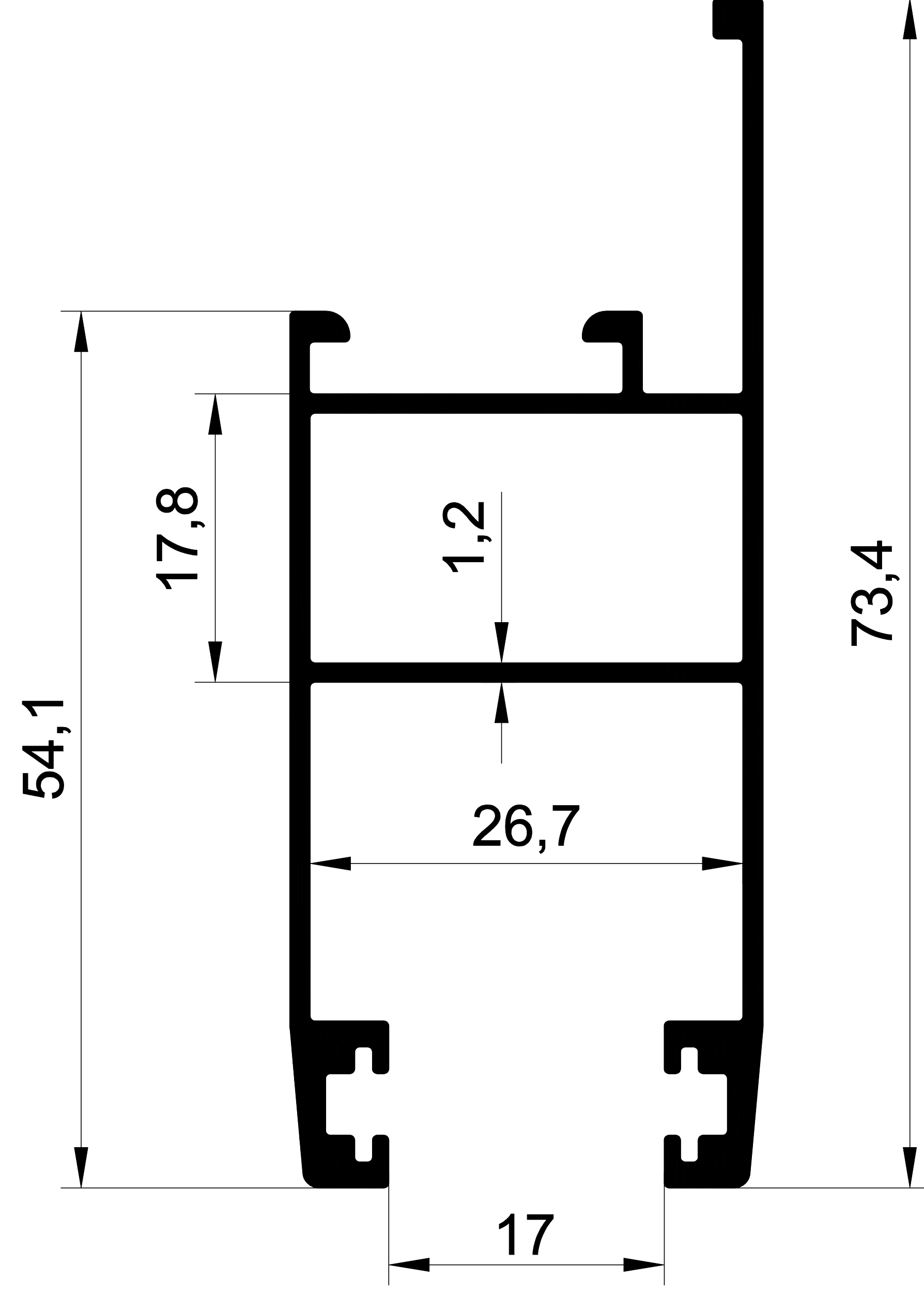
1382 0,803 Kg/m. 2000 SERİ SÜRME KANAT
