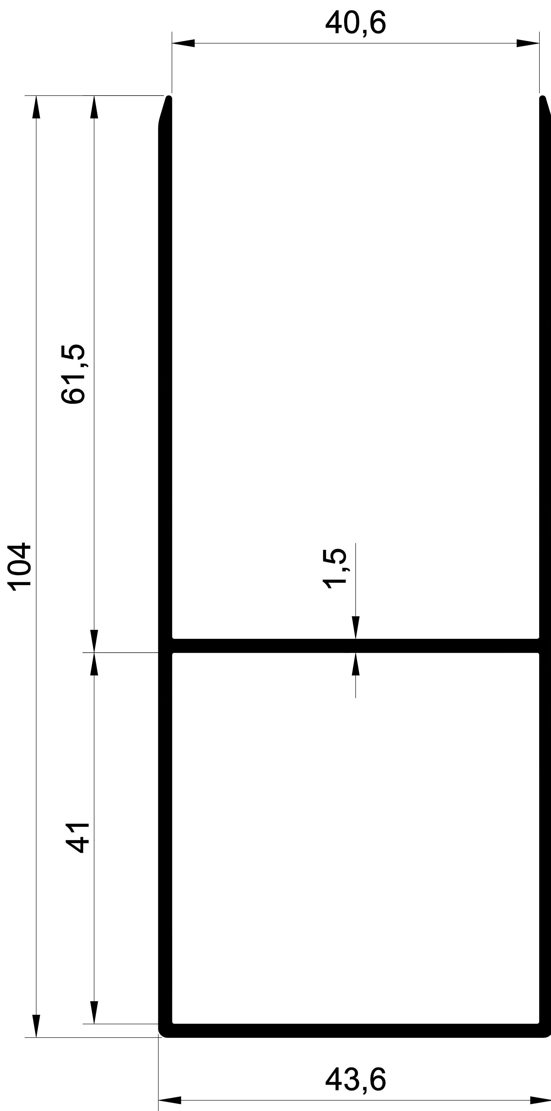
1252 1,168 Kg/m. CAM BALKON ETEK
