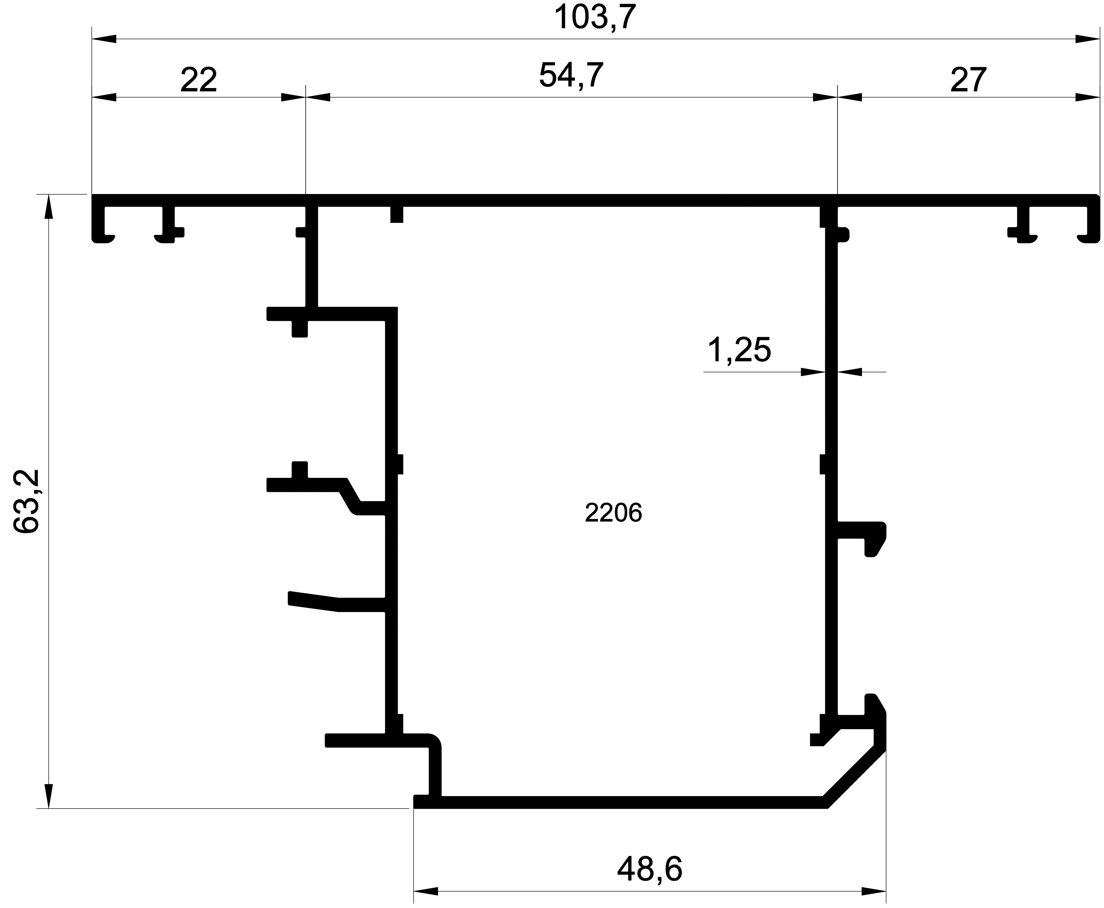
EK-55- 2206 1,267 Kg/m SİSTEM 55 DIŞA AÇILIR KAPI
