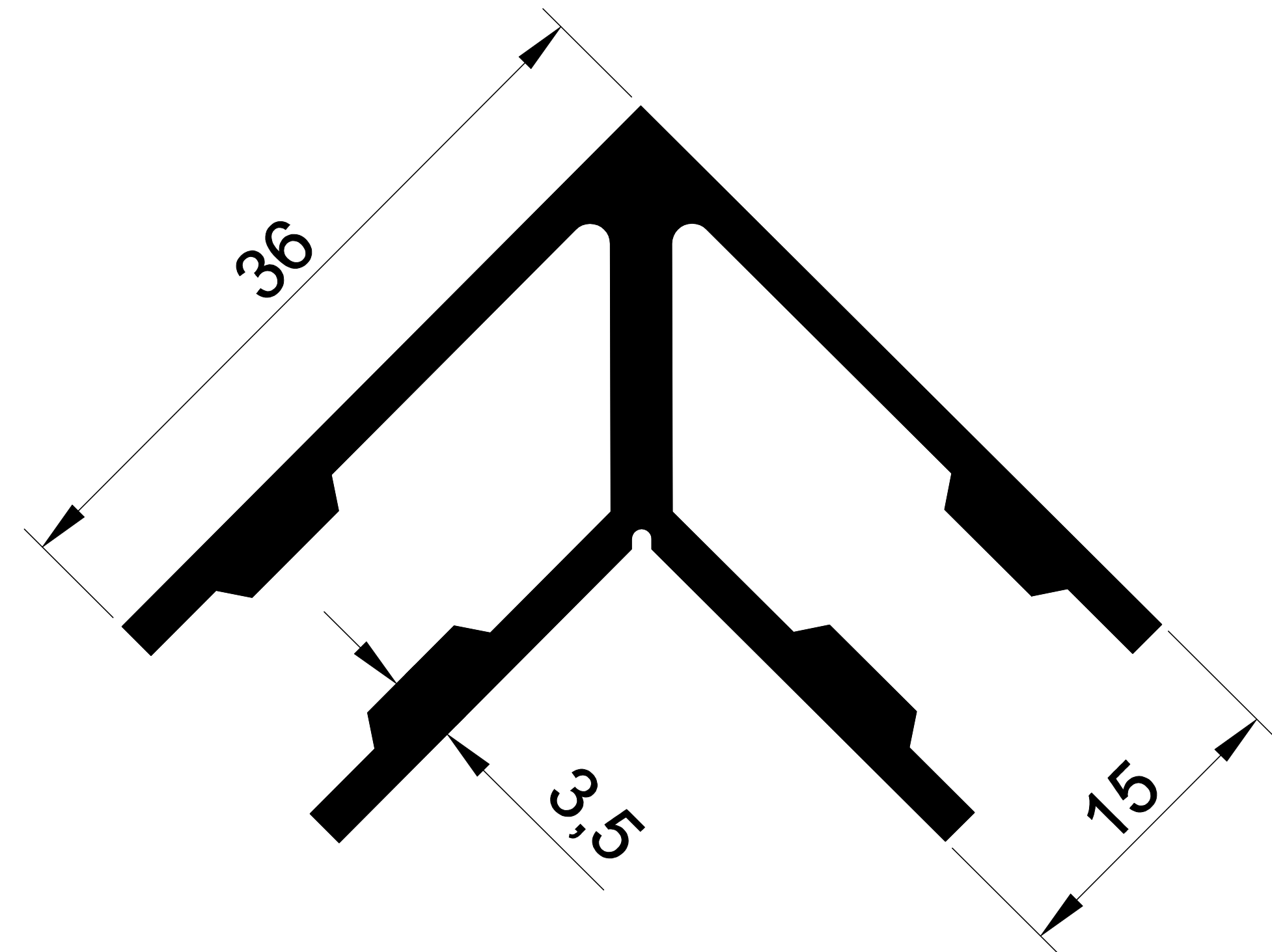
1096 0,863 Kg/m. DAR ÇAVUŞ (KÖŞE BAĞLANTI)
