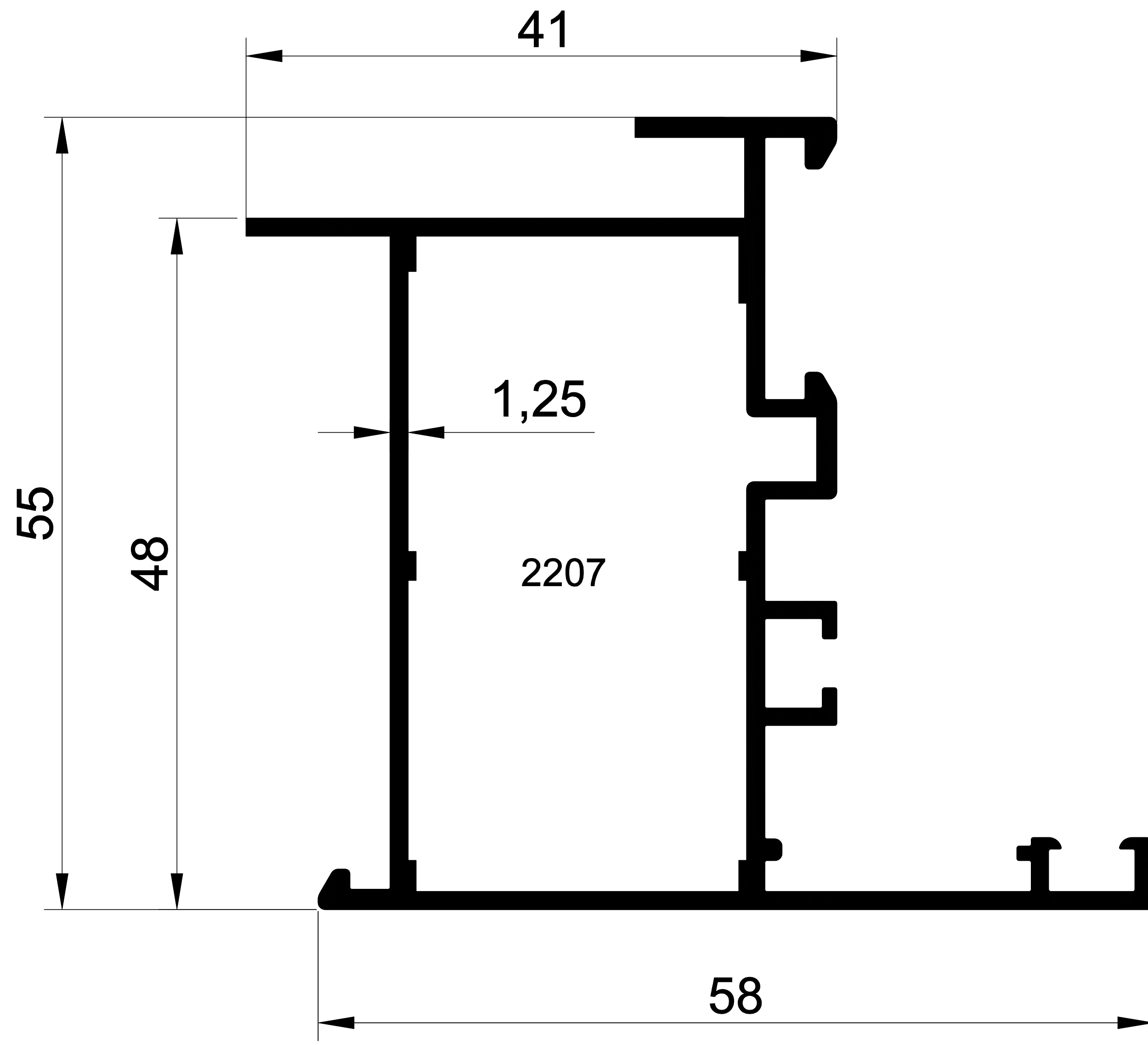
EK-55- 2207 0,860 Kg/m SİSTEM 55 TERS KAPI ADAPTÖRÜ
