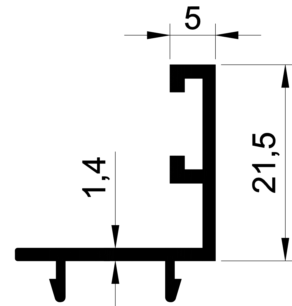
1352 0,231 Kg/m. C-60 TIRNAK
