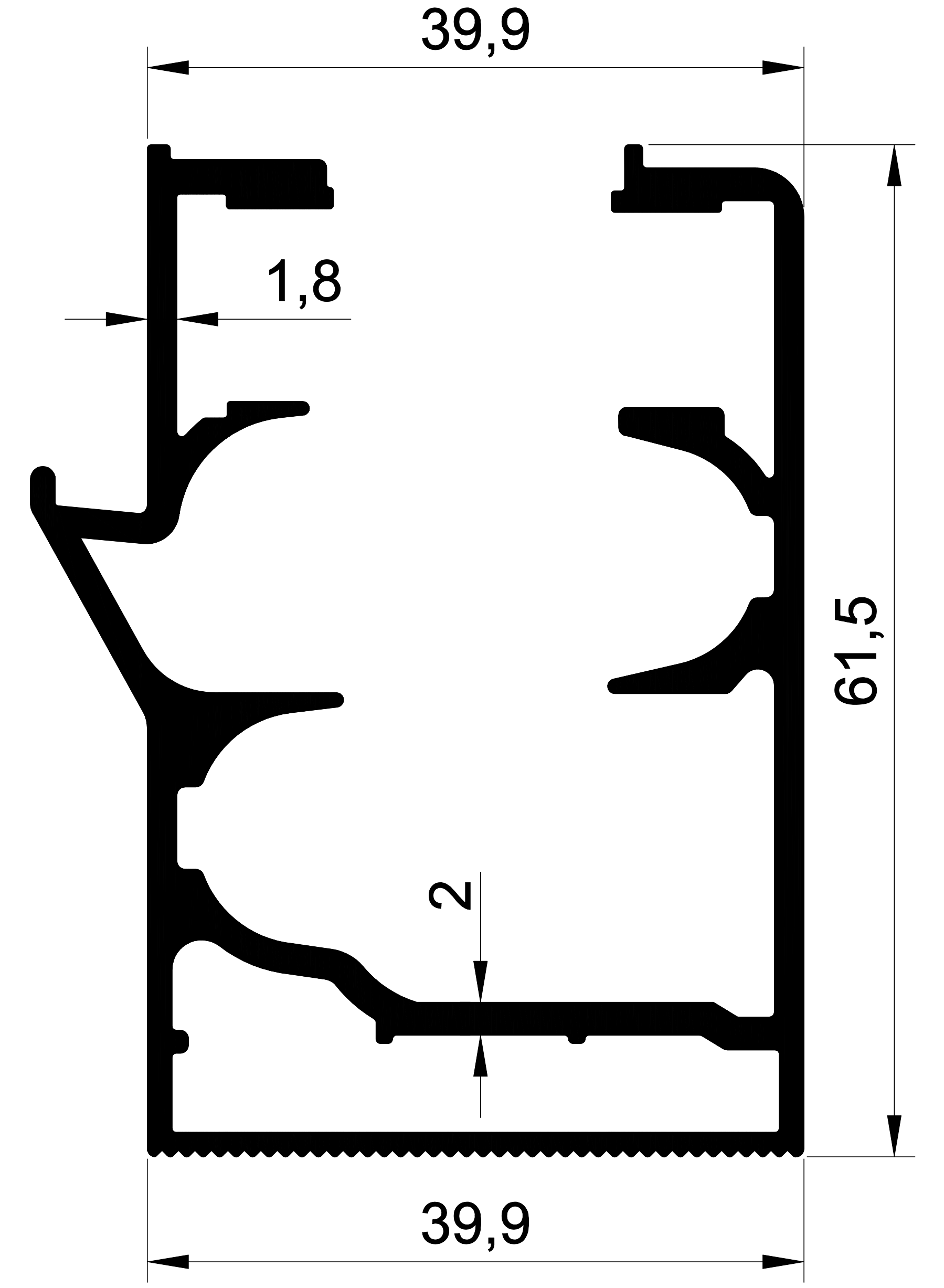
1315 1,361 Kg/m. ISI YALITIM ORTADAN DAMLALIKLI KASA
