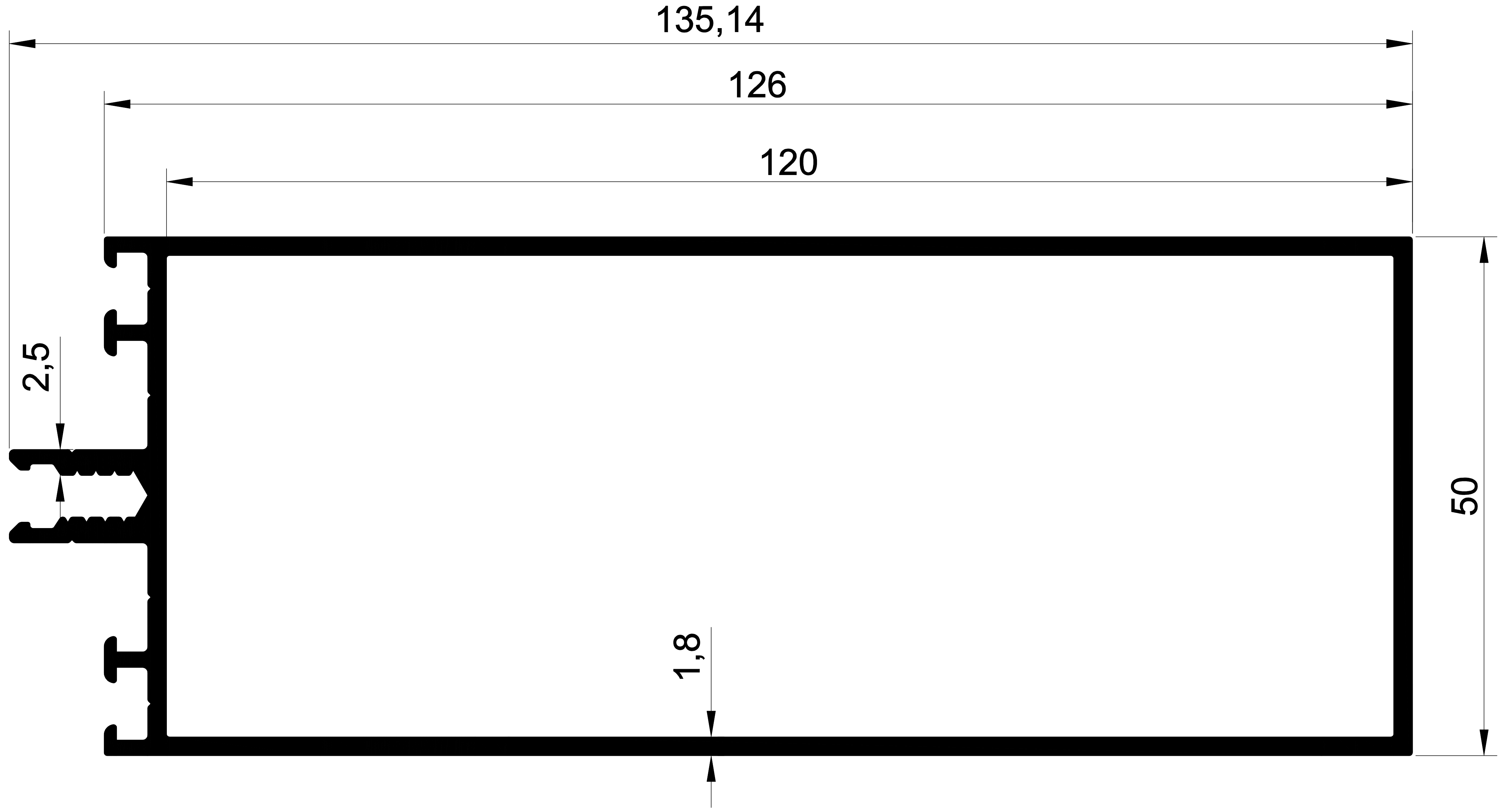
126'LIK CEPHE PROFİLİ
