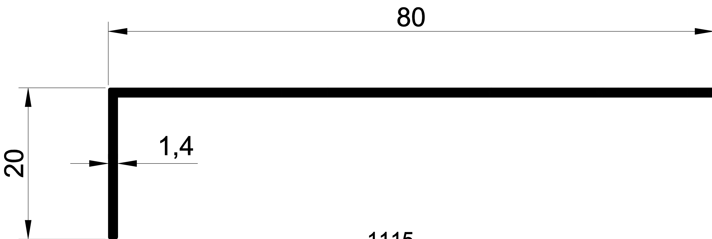
1115 0,335 Kg/m.
