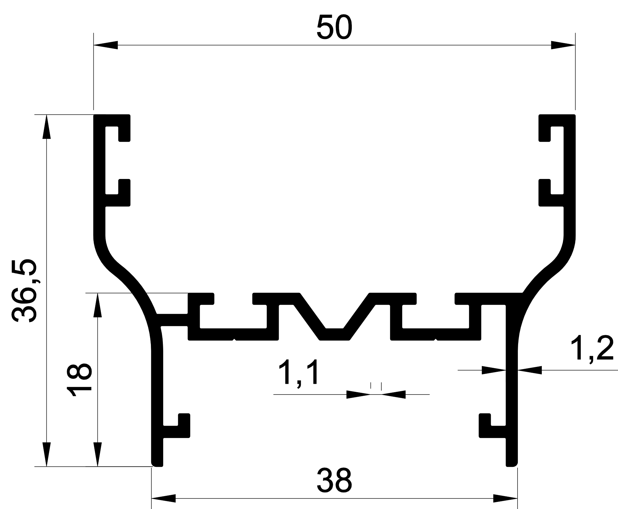
2301 0,537 gr/m ISICAMLI CAM BALKON PROFİLLERİ
