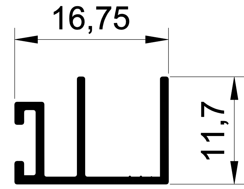
1171 0,122 Kg/m. SÜRME YAN ÇITA
