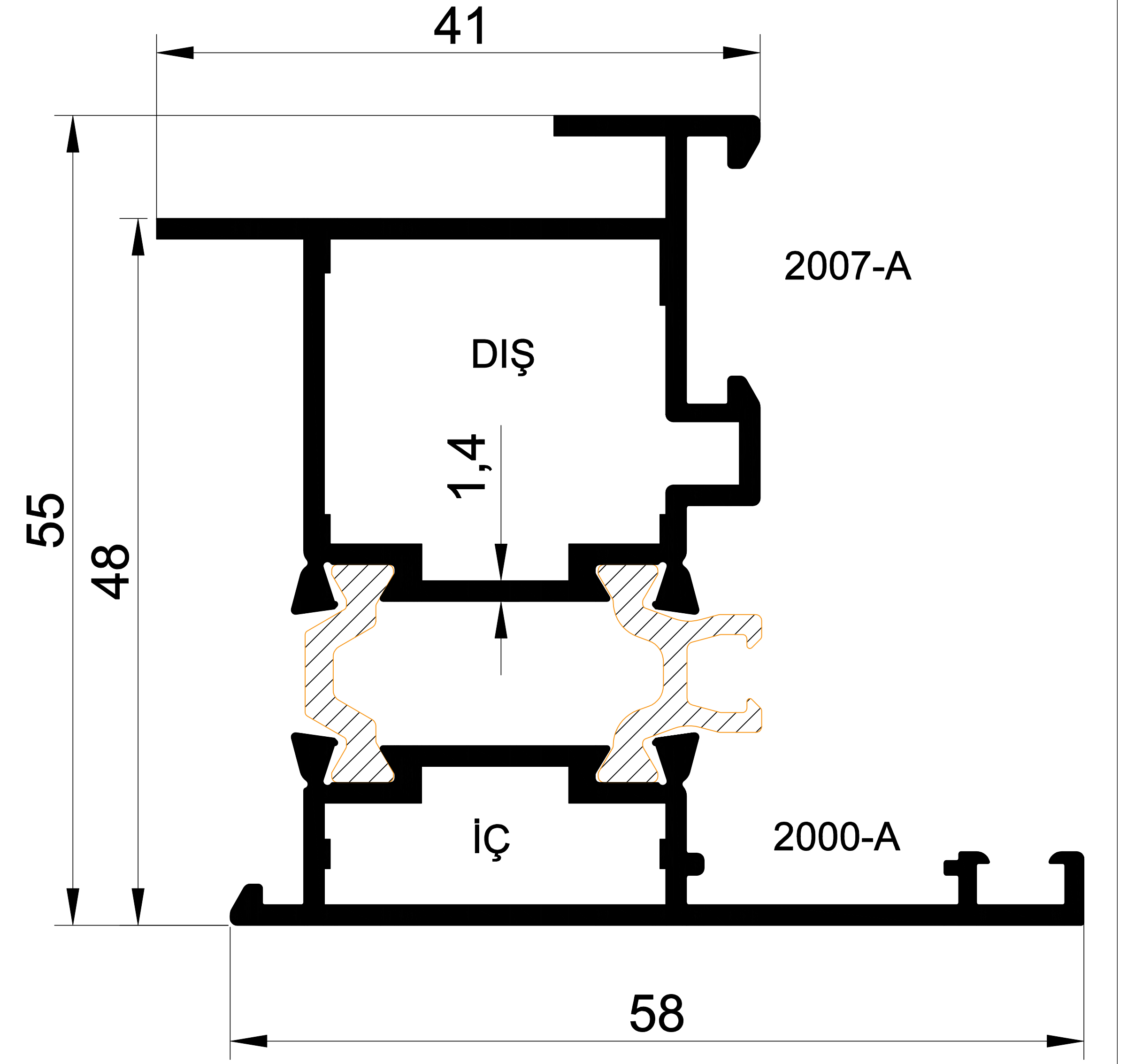
-55- 2007 1,084 Kg/m SİSTEM 55 ISI YALITIM TERS KAPI ADAPTÖRÜ
