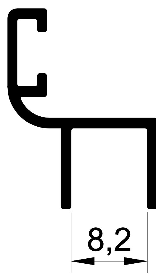
1252 1,168 Kg/m. CAM BALKON ETEK
