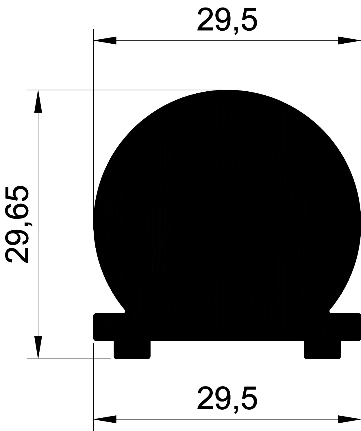
1298 1,938 Kg/m.
