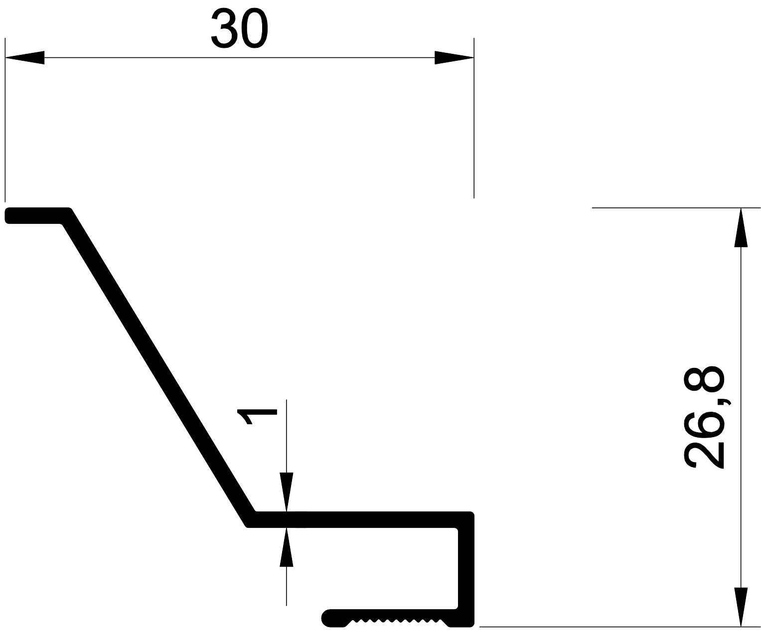
1174 0,146 Kg/m. DAMLALKI PROF.
