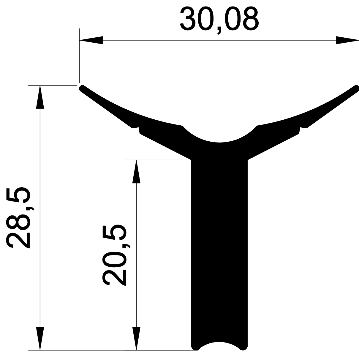
1339 0,478 Kg/m.
