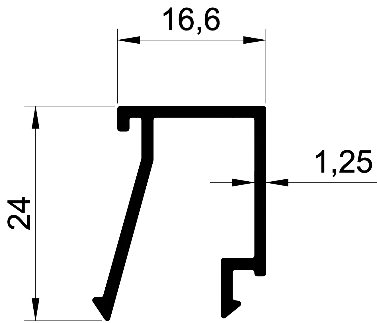
1383 0,241 Kg/m. 2000 SERİ SÜRME ÇITA
