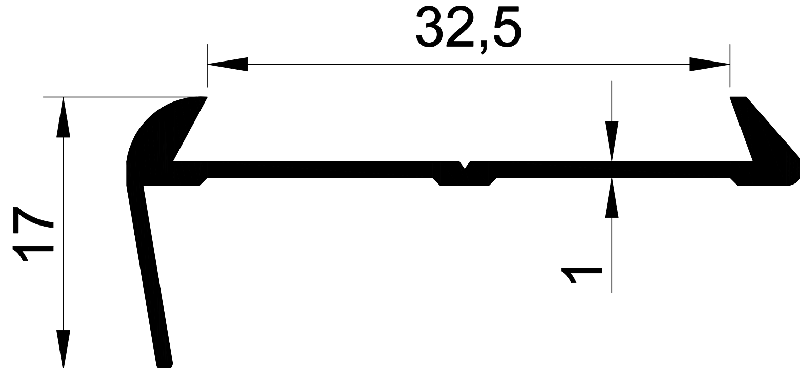
1366 0,213 Kg/m. MERDİVEN PROFİLİ
