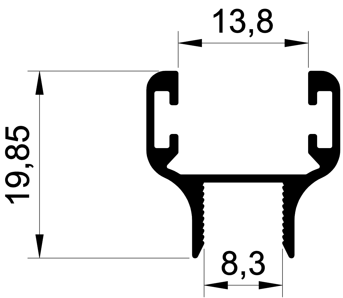
1150 1,008 Kg/m. CAM BALKON ETEK
