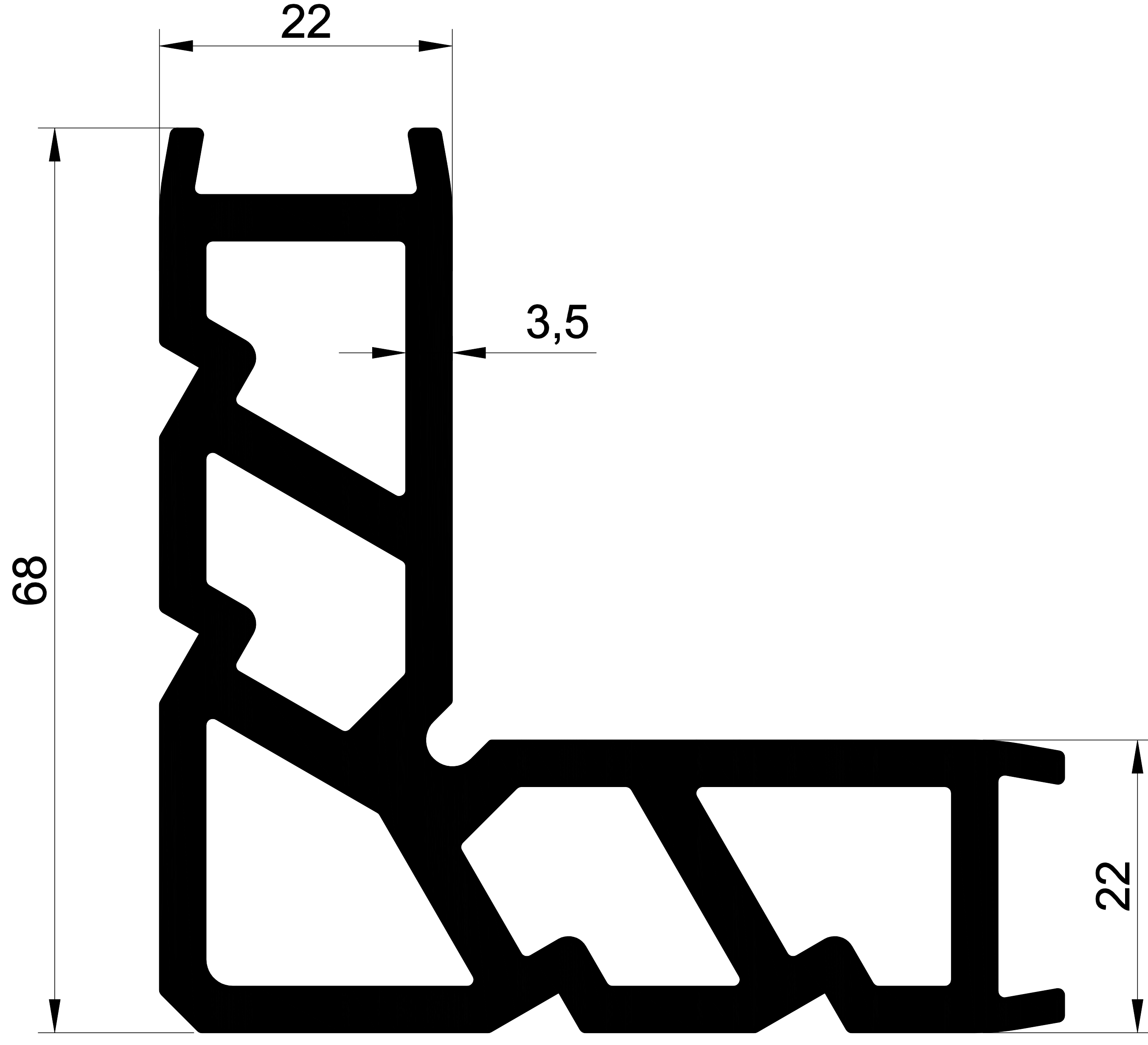
-55- 2012 3,238 Kg/m SİSTEM 55 KÖŞE TAKOZU
