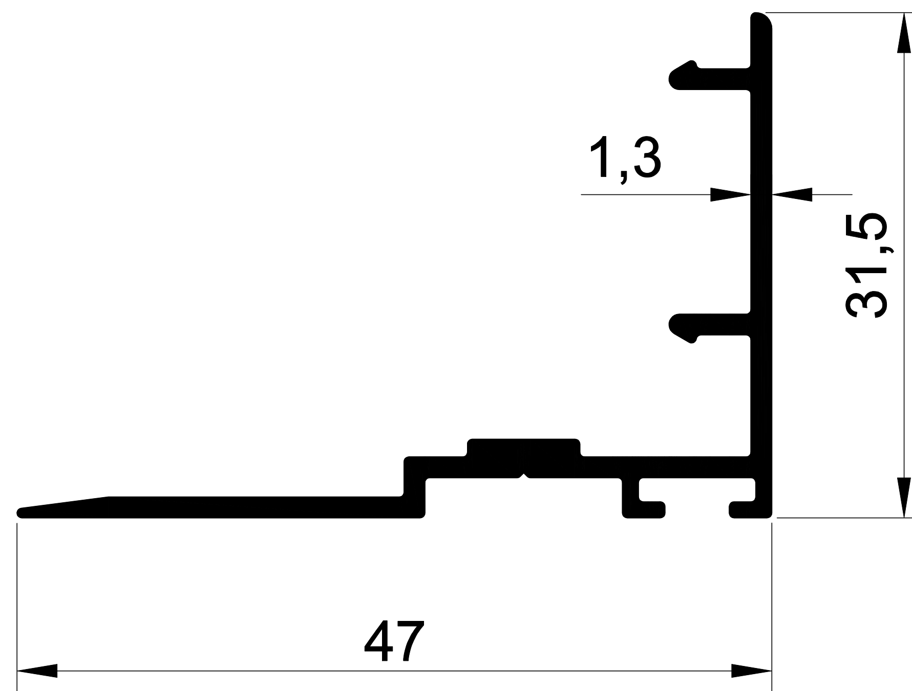
1384 0,346 Kg/m. 2000 SERİ SÜRME KENET
