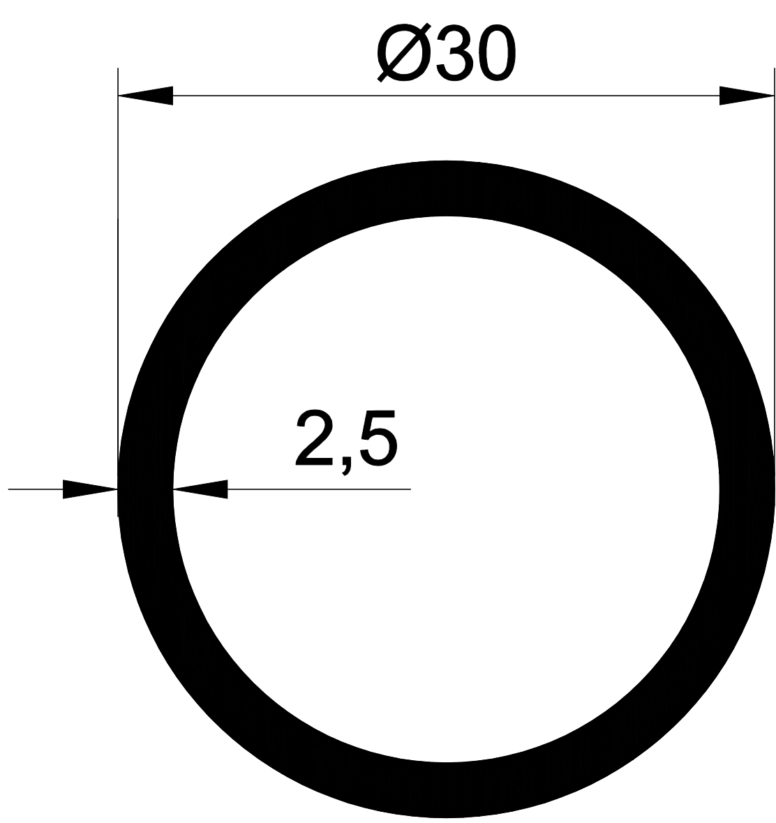
1275 0,585 Kg/m.
