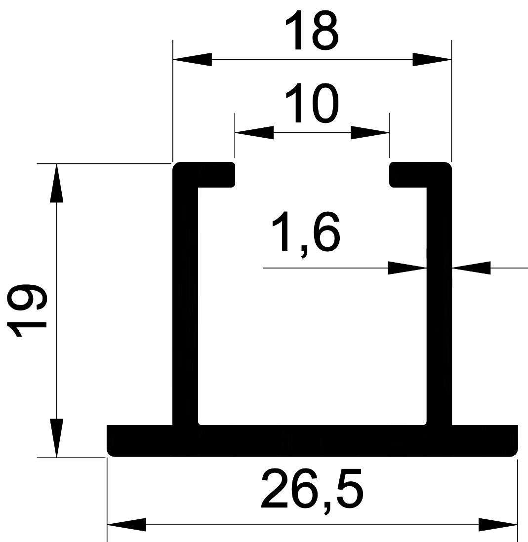
1245 0,312 Kg/m.
