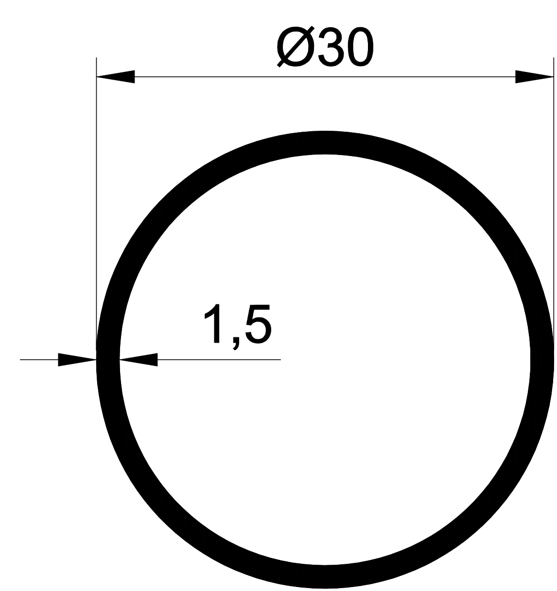
1004 0,363 Kg/m.
