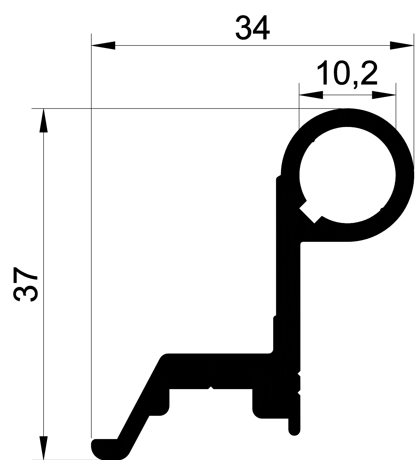
1137 0,574 Kg/m.
