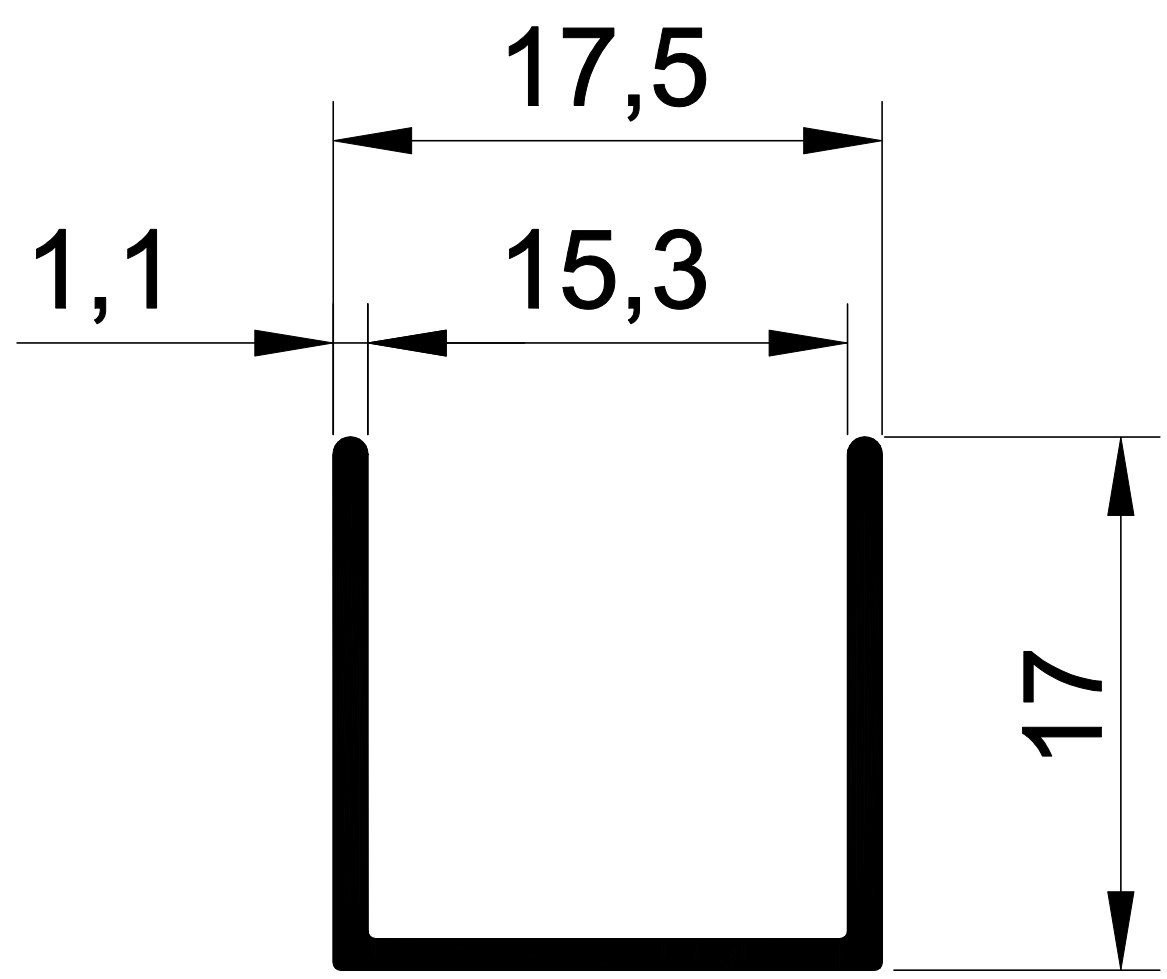
1179 0,141 Kg/m. PANJUR DAR U
