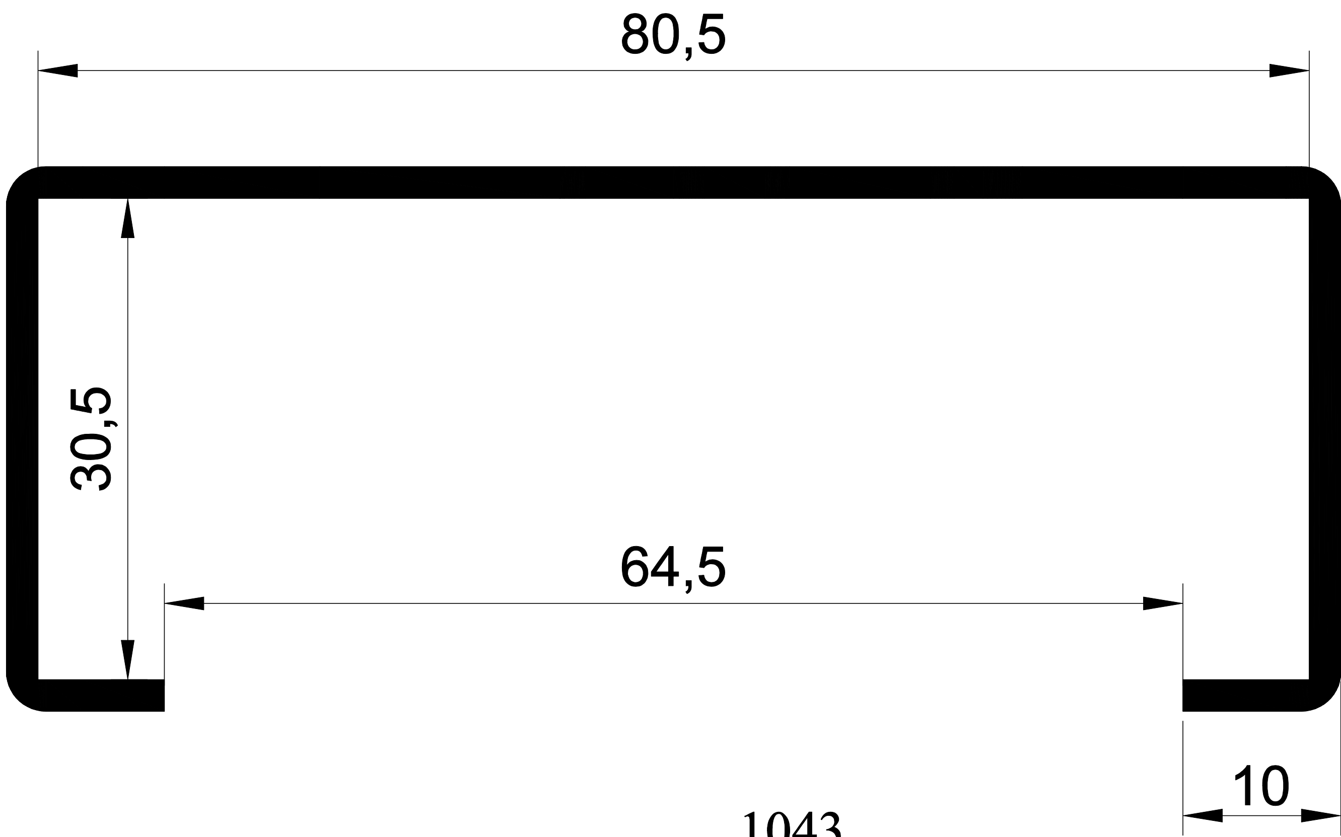
1043 0,882 Kg/m.
