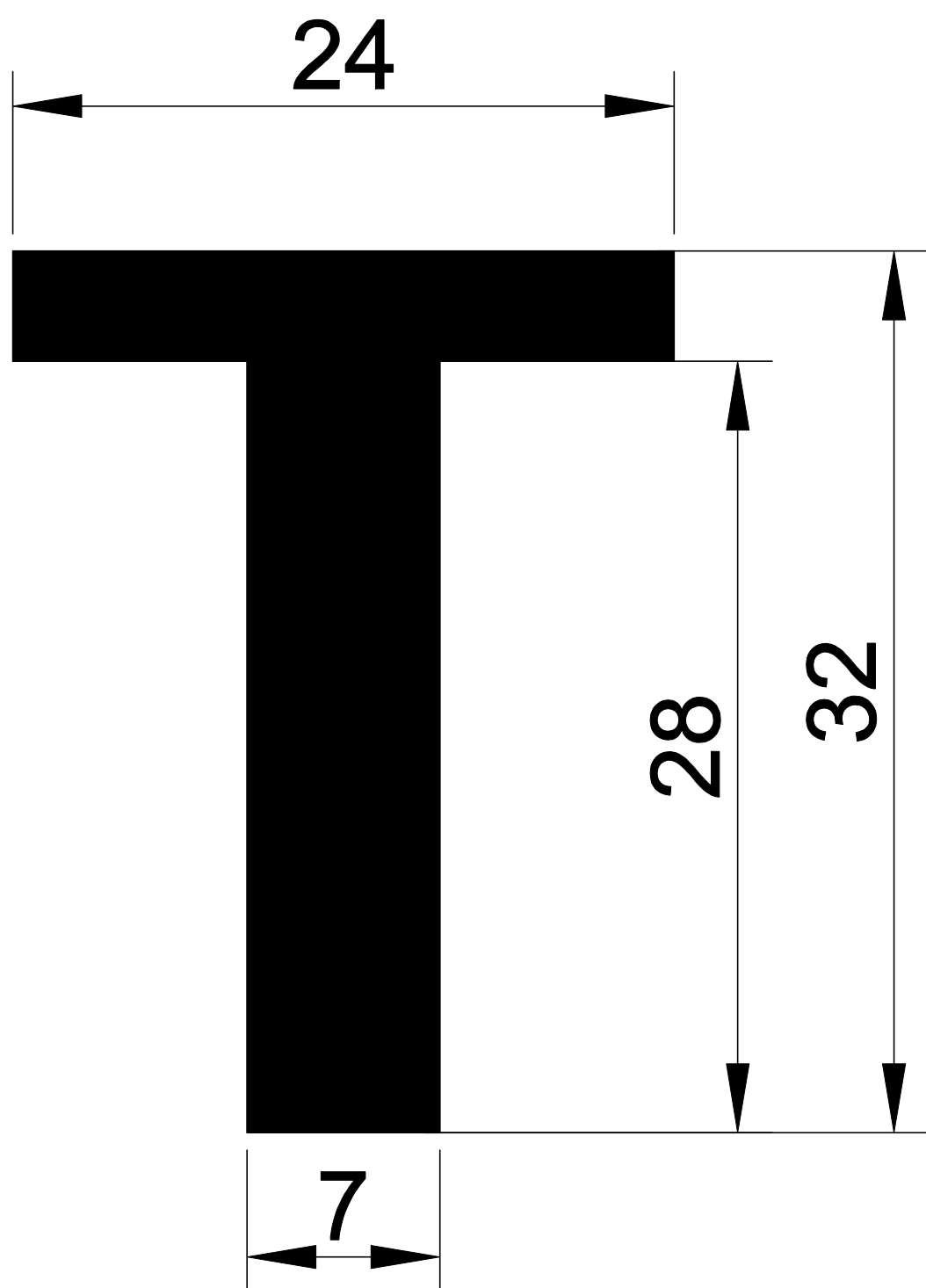
1073 0,792 Kg/m.
