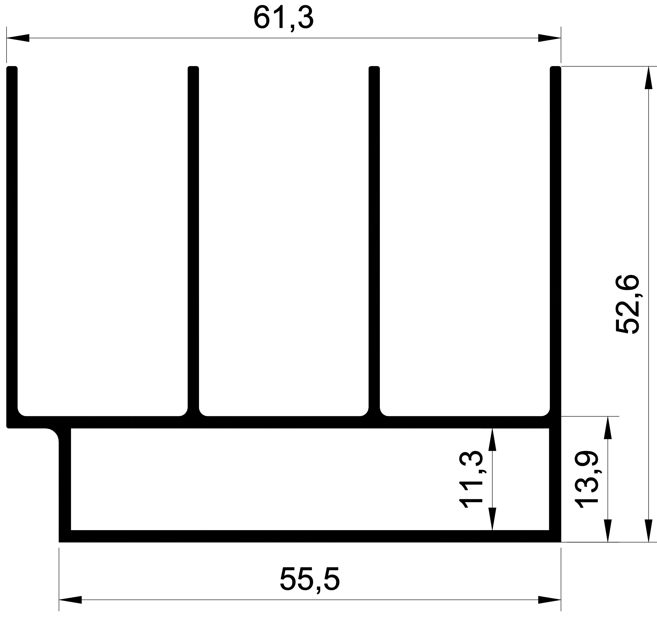
1313 1,000 Kg/m. 3'LÜ SÜRME KASA
