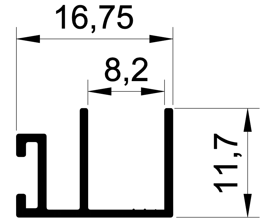
1171 0,122 Kg/m. SÜRME YAN ÇITA
