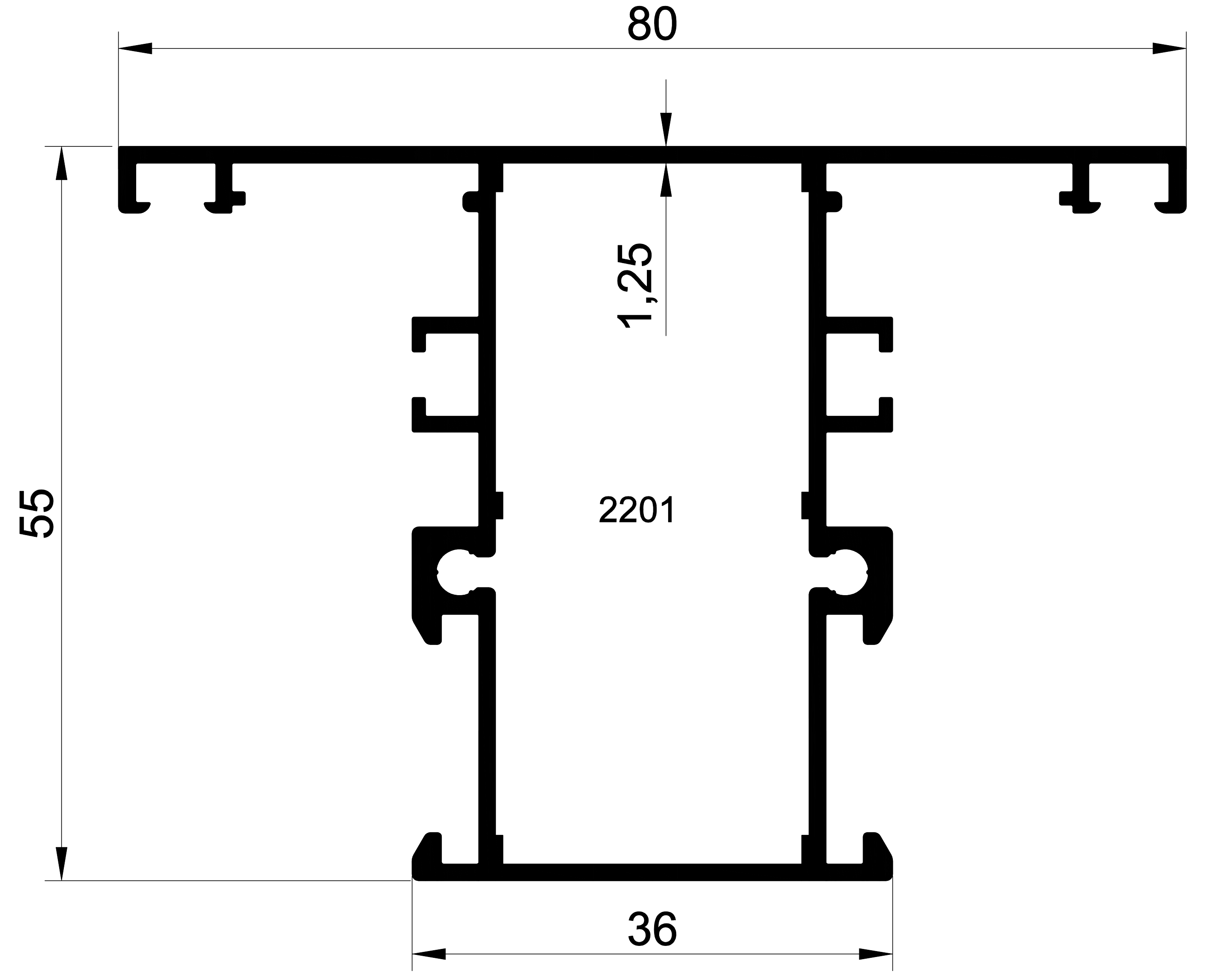
EK-55- 2201 1,073 Kg/m SİSTEM 55 YALITIMSIZ ORTA
