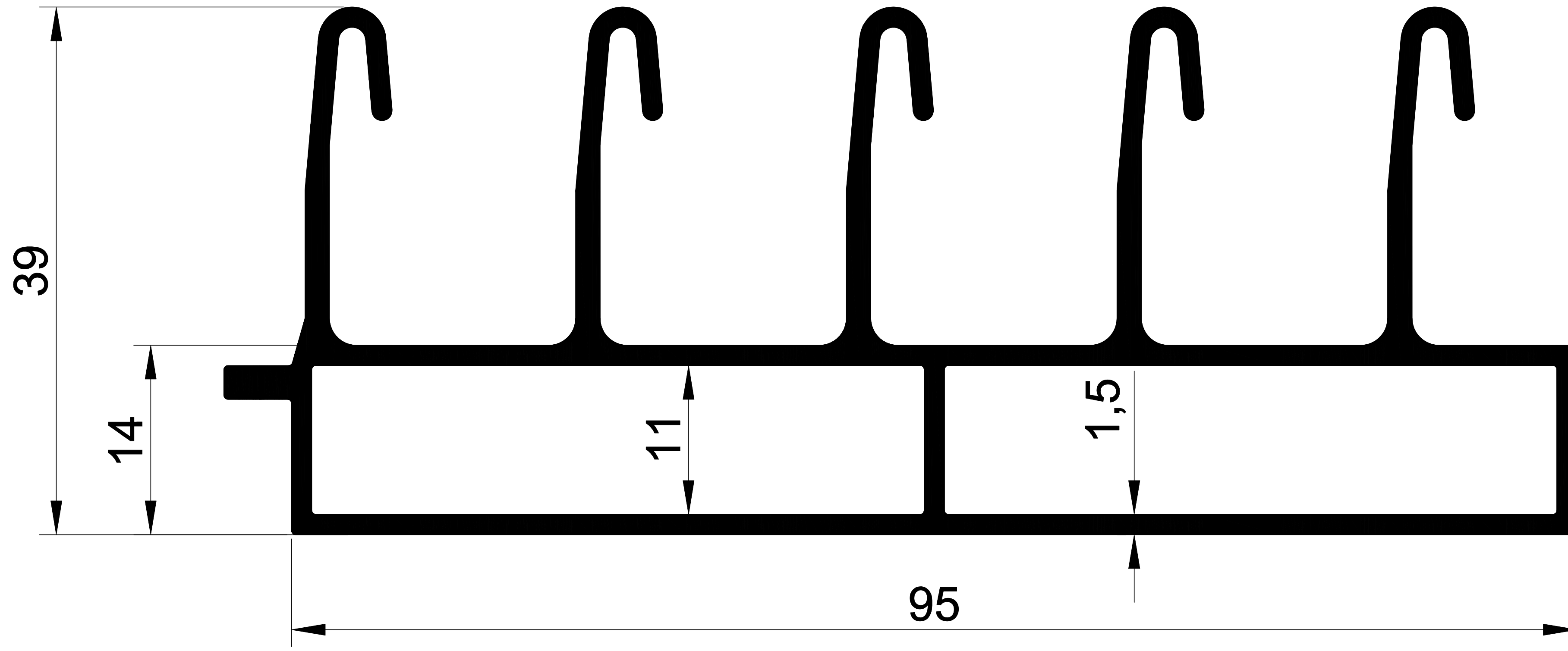
1165 1,410 Kg/m. SÜRME KASA
