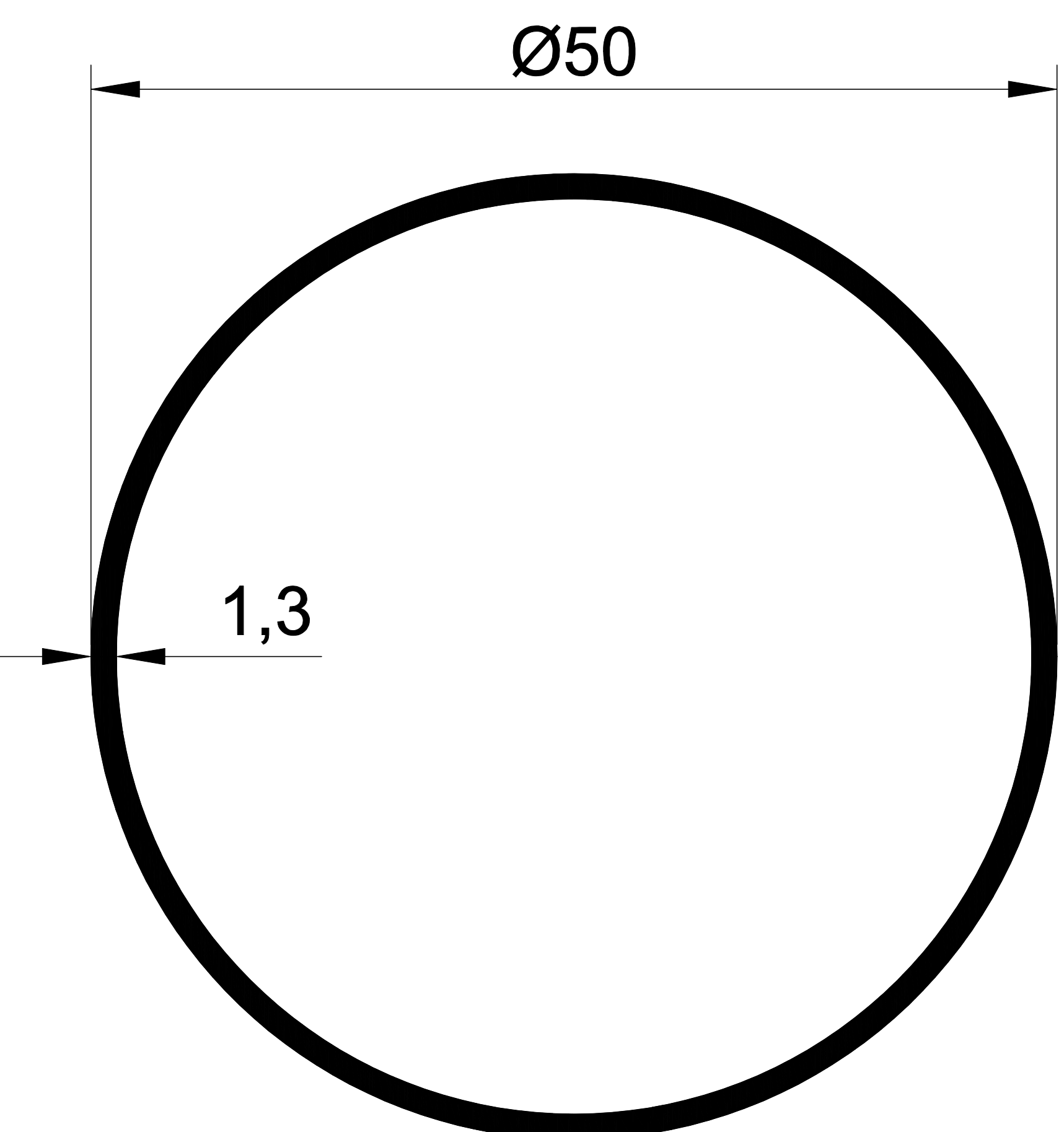
1066 0,539 Kg/m.
