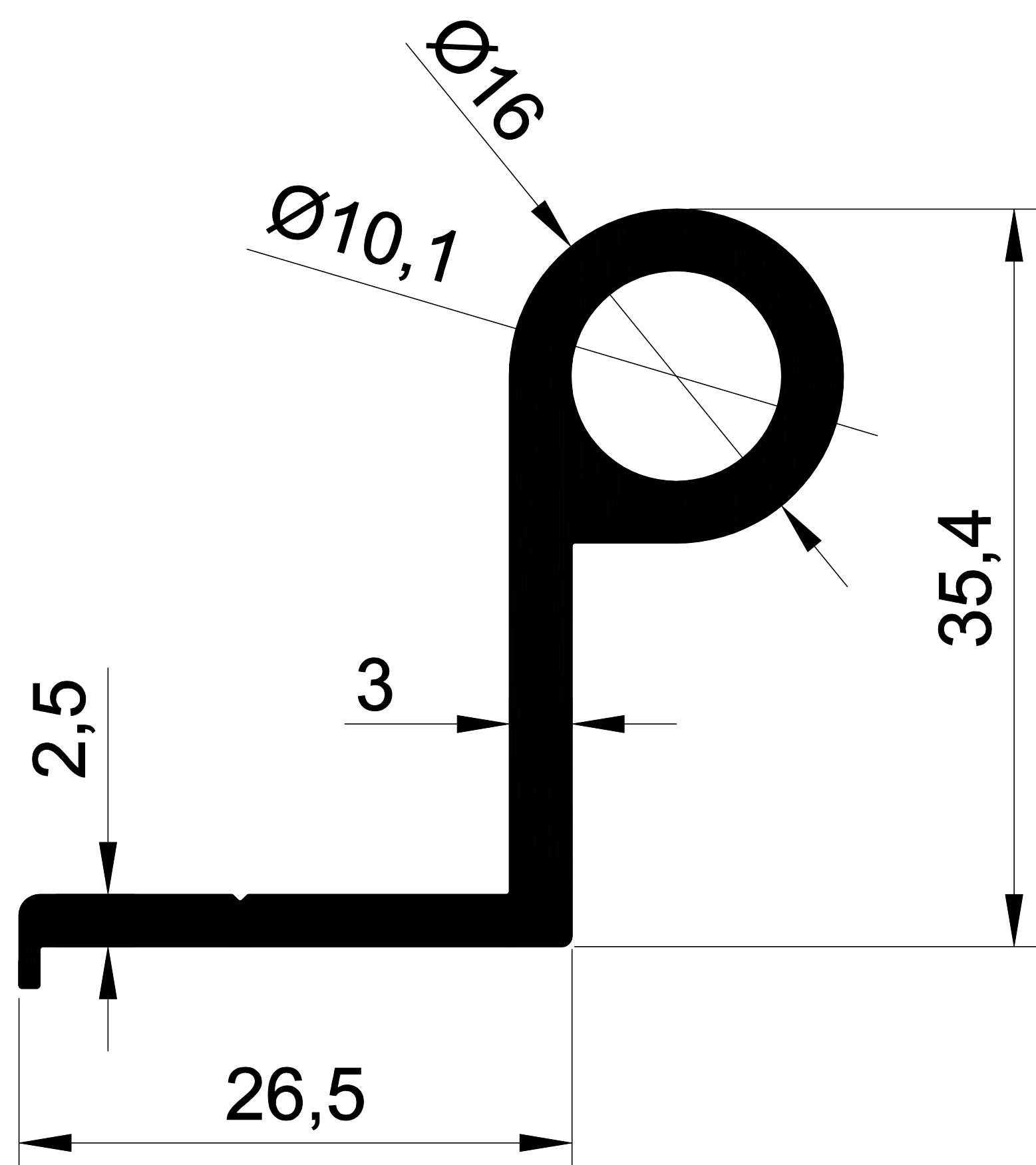
55- 2011 0,686 Kg/m SİSTEM 55 KANAT MENTEŞE
