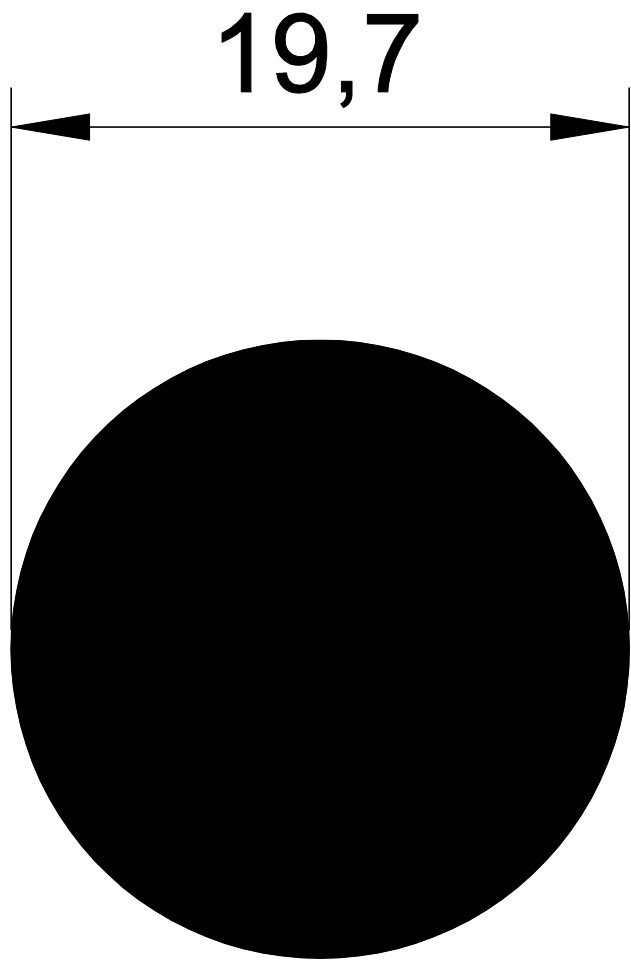
1060 0,826 Kg/m.
