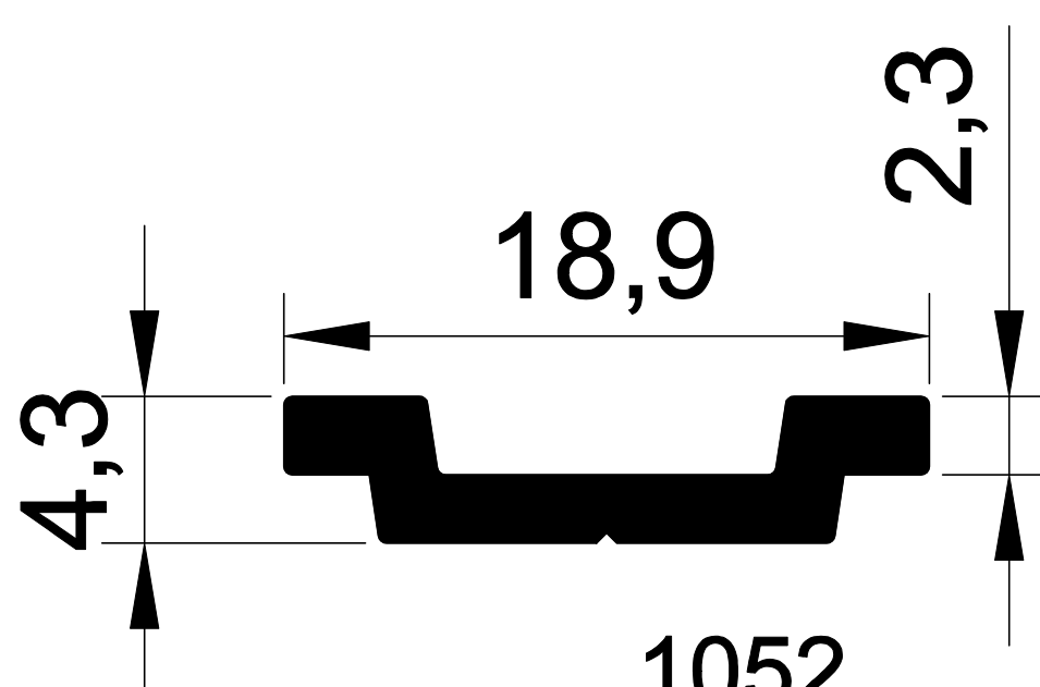
1052 0,127 Kg/m. TİJ ÇUBUĞU
