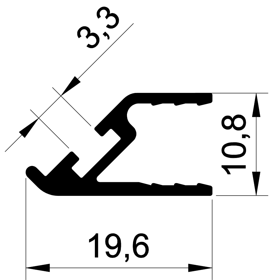
1249 0,152 Kg/m. CAM H
