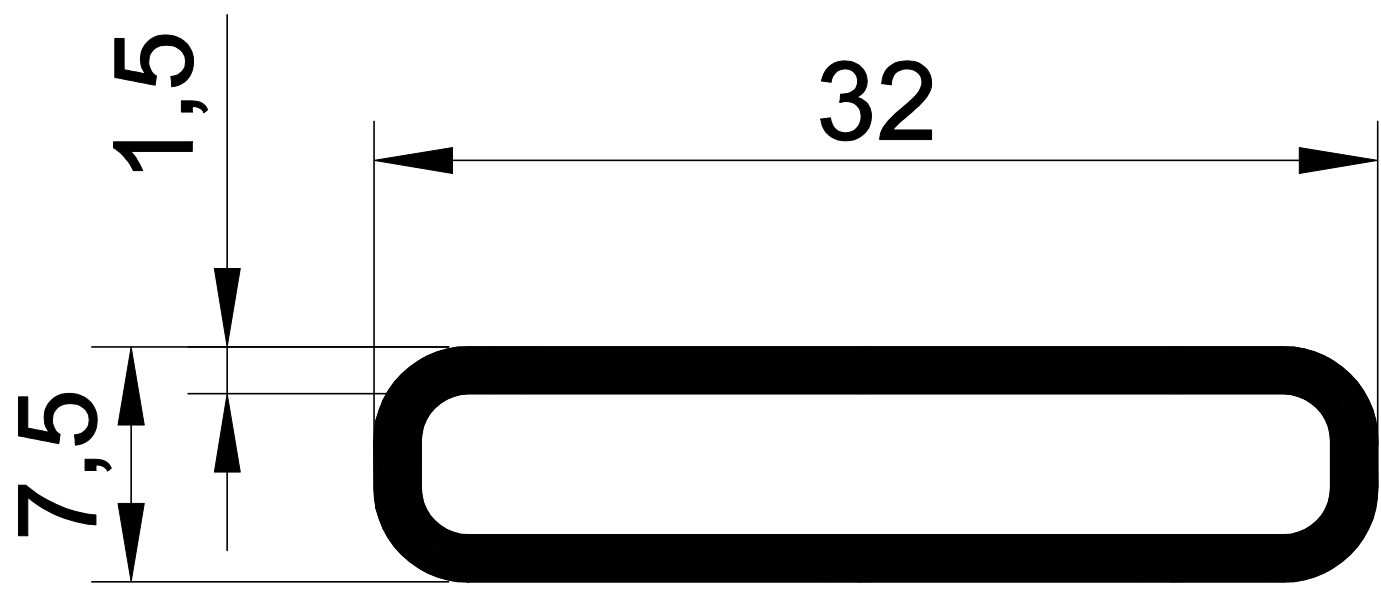
1124 0,282 Kg/m.
