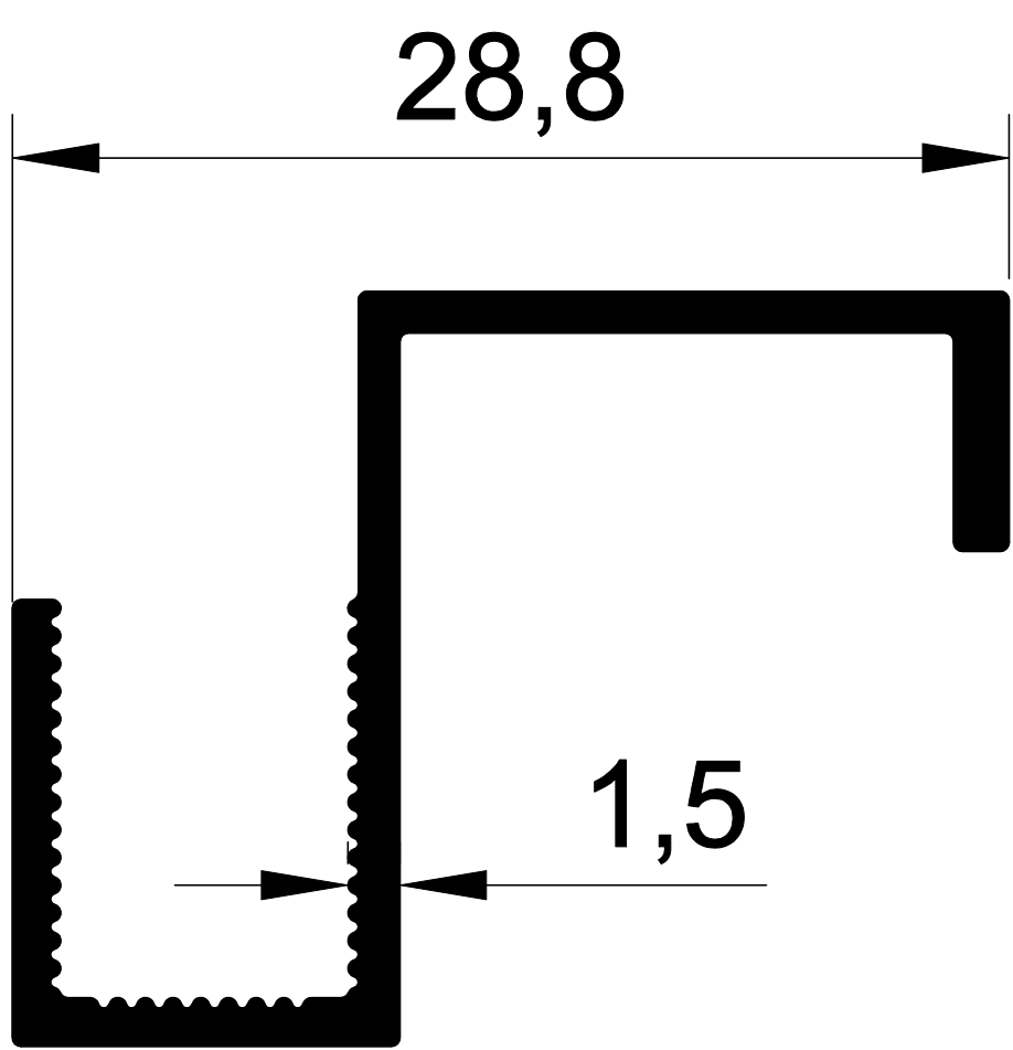
1448 0.236 Kg/m. C.B KOL PROFİLİ-1
