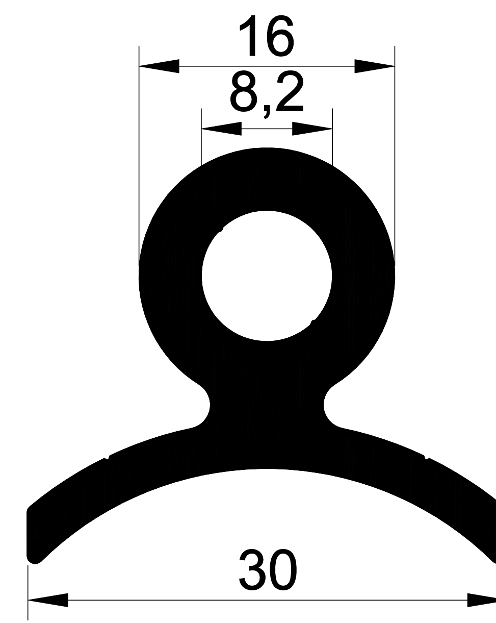
1177 0,699 Kg/m.
