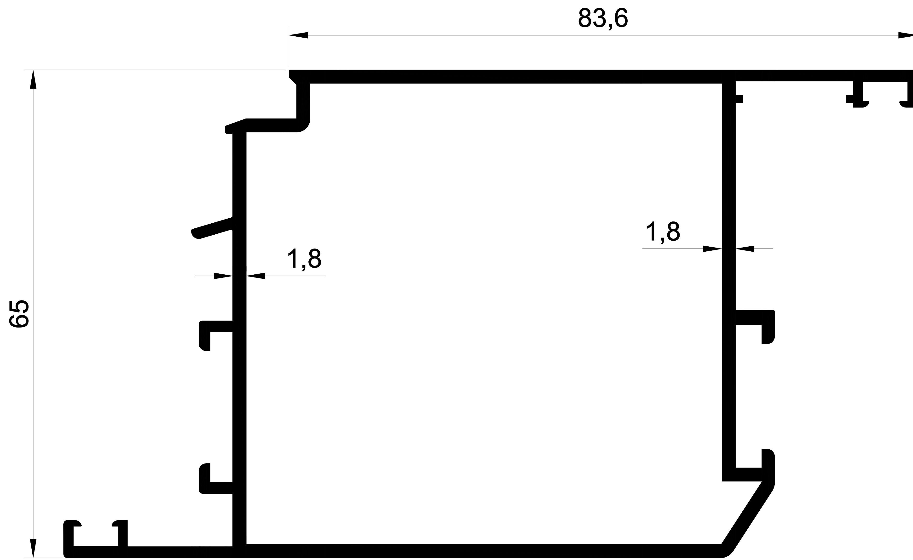
1202 1,667 Kg/m. SİSTEM BAZA KAPI
