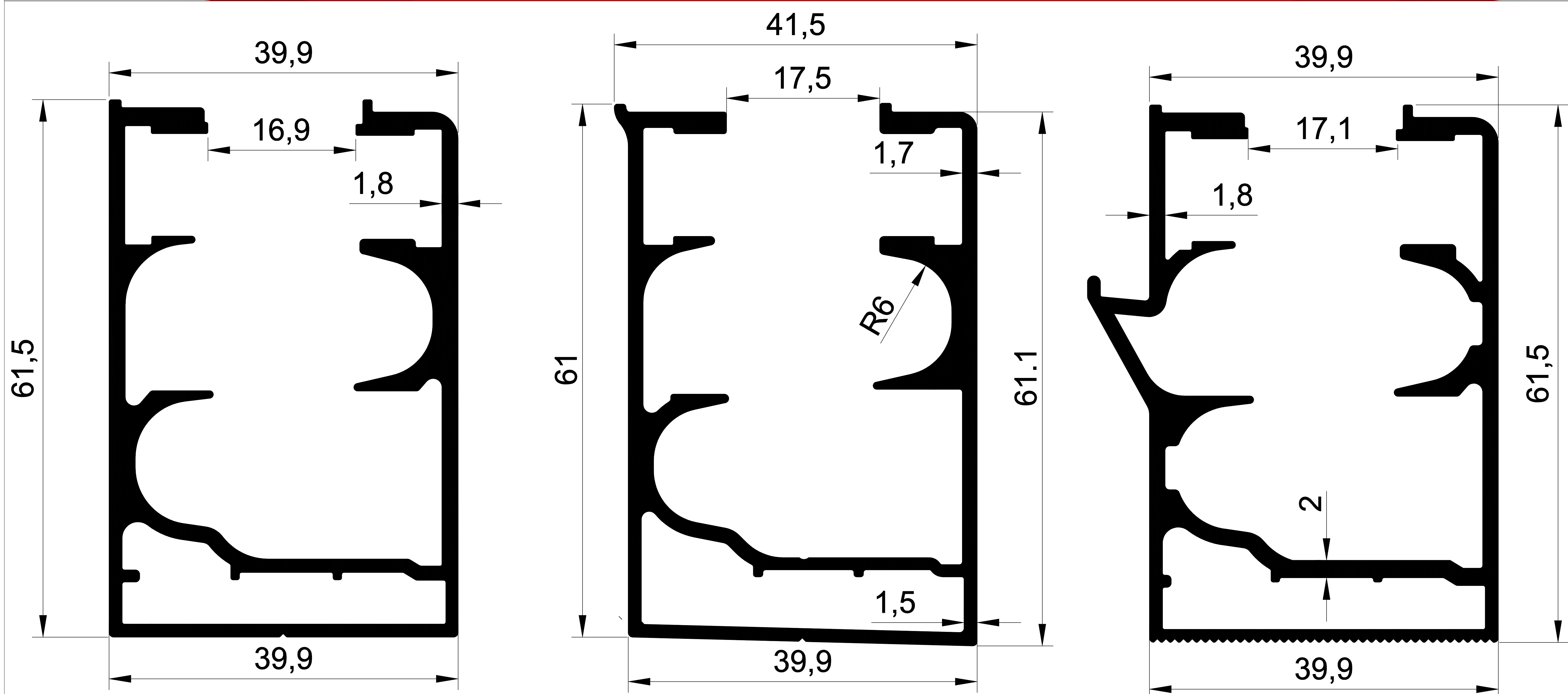
1187 1,350 Kg/m. BKS KASA
