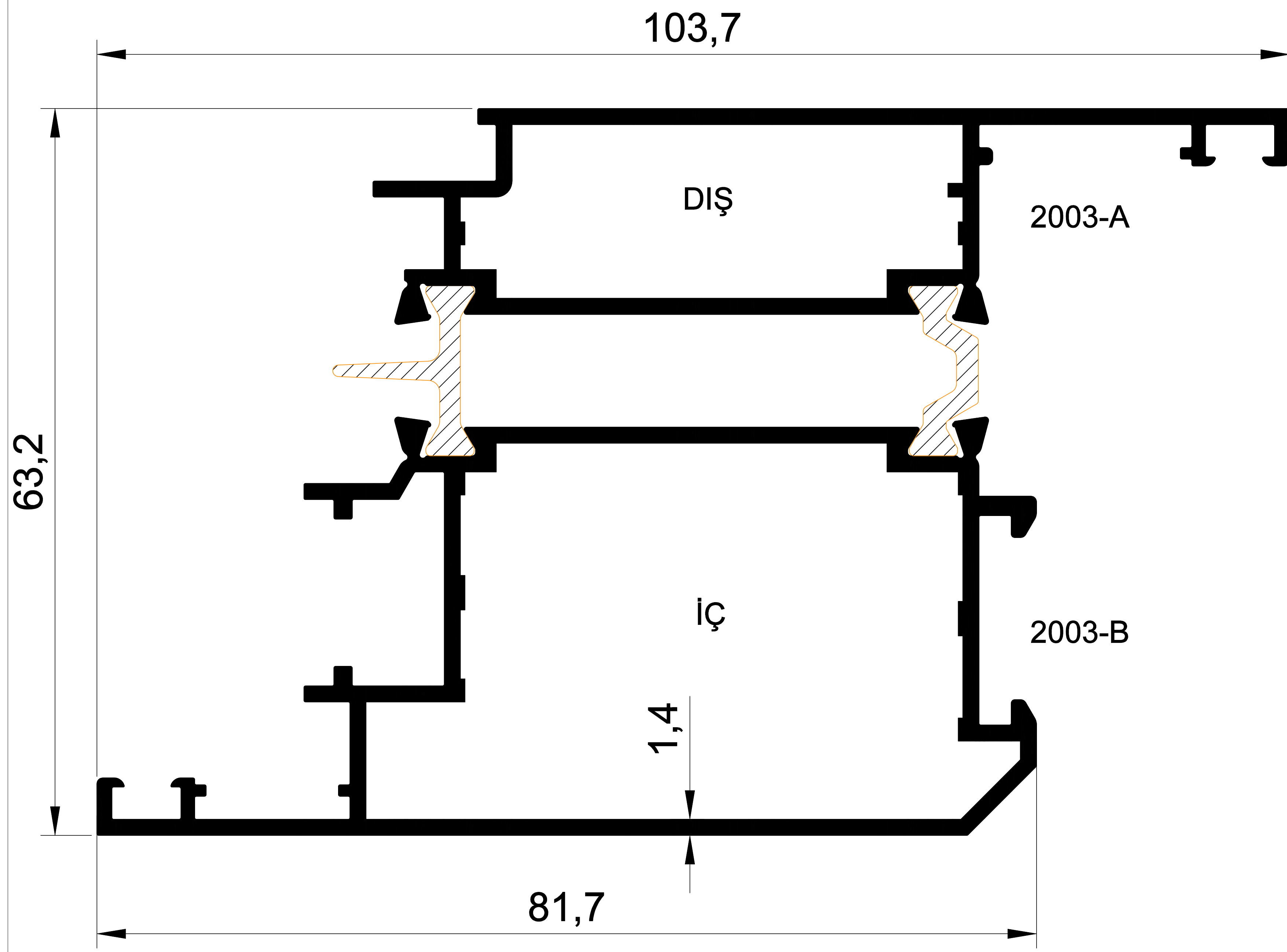
-55- 2003 1,697 Kg/m SİSTEM 55 ISI YALITIM IÇE AÇILIR KAPI
