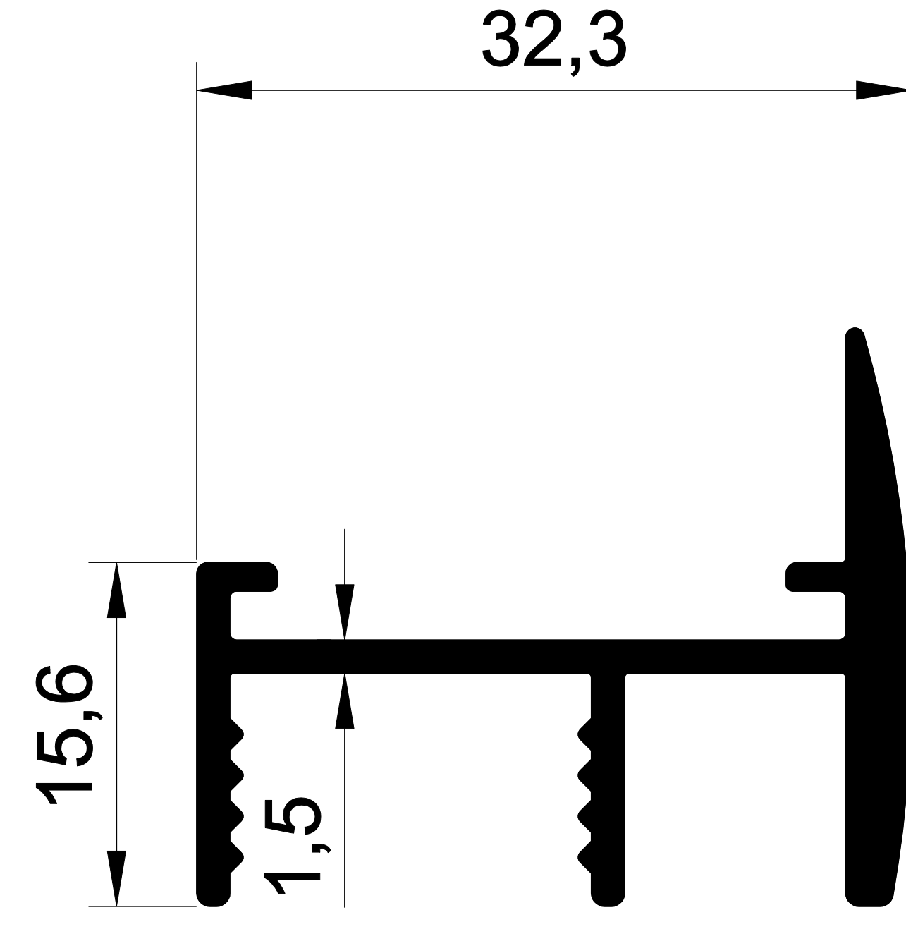
1157 0,457 Kg/m. MEBO KASA
