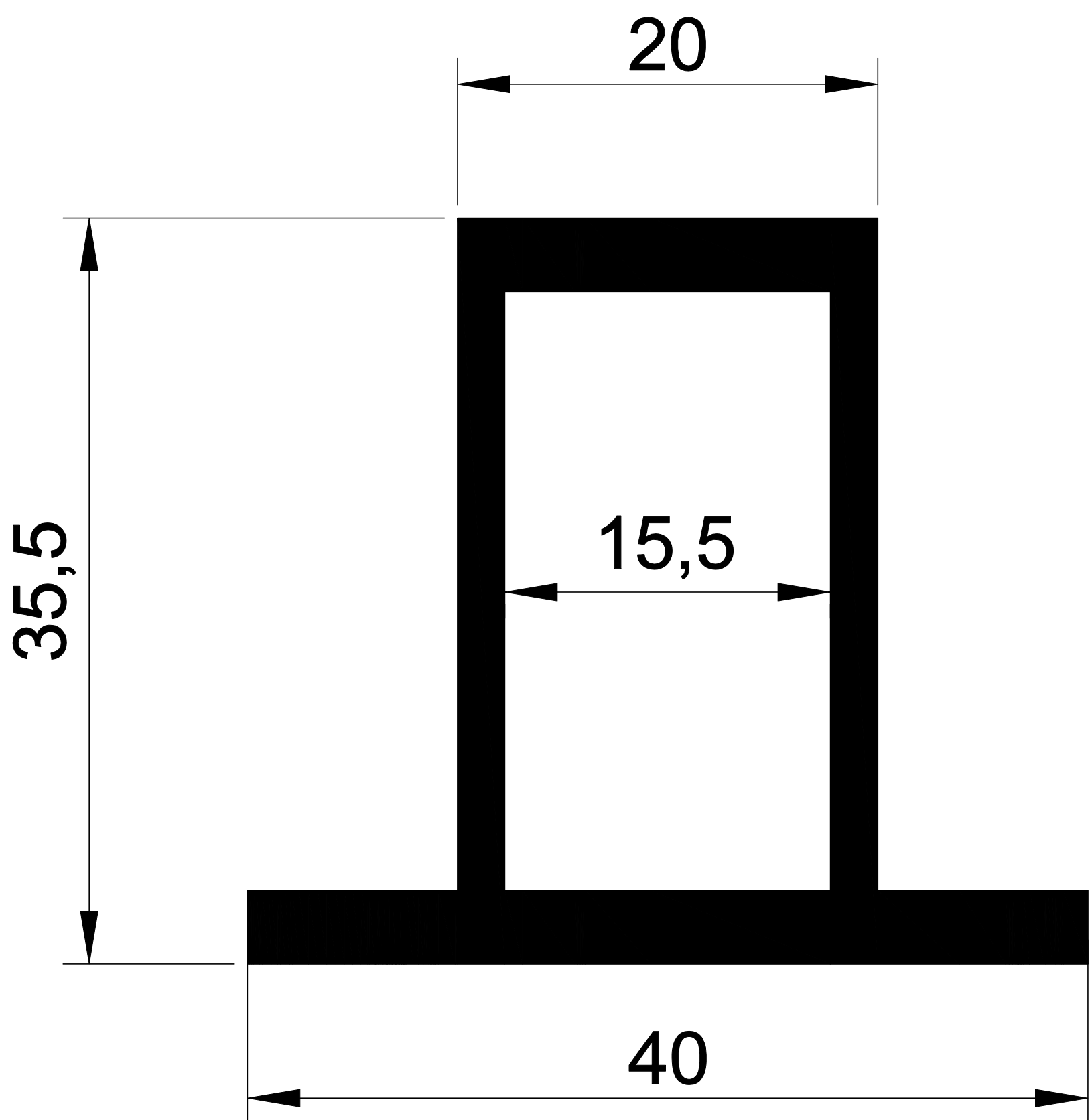
1242 0,916 Kg/m.
