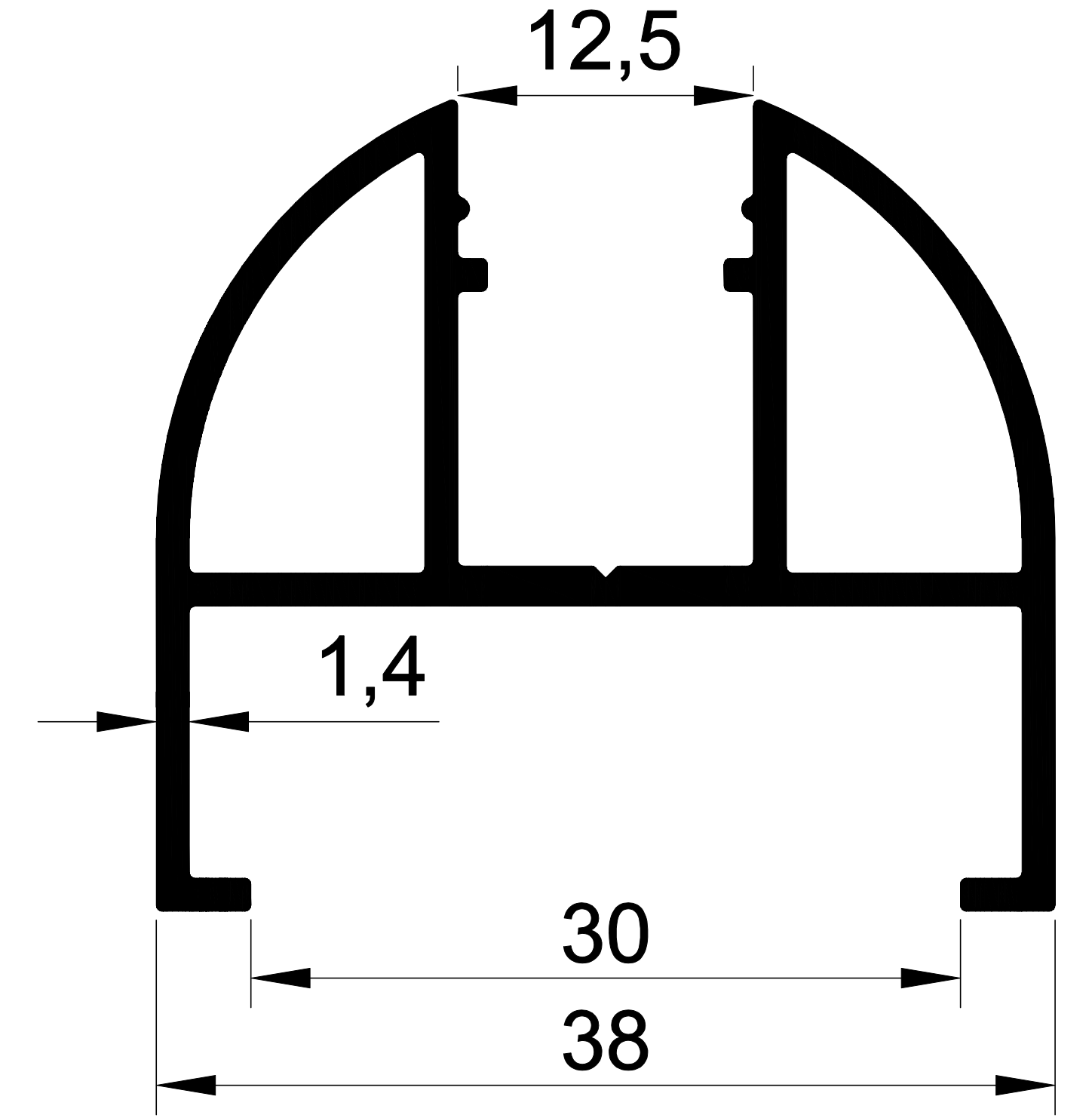
1365 0,607 Kg/m. ISI YALITIM KÖŞE DÖNÜŞ
