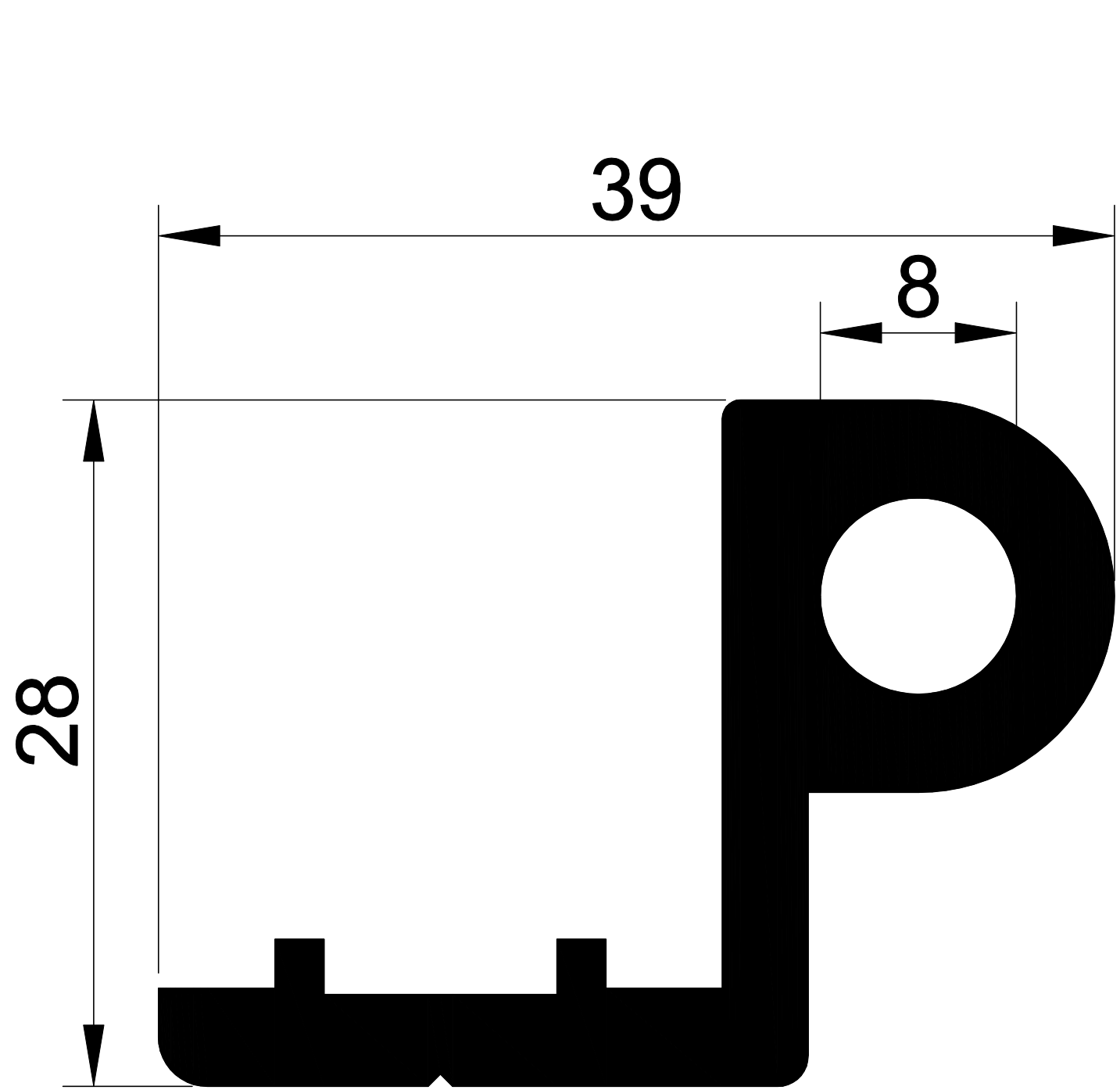
1228 0,856 Kg/m.
