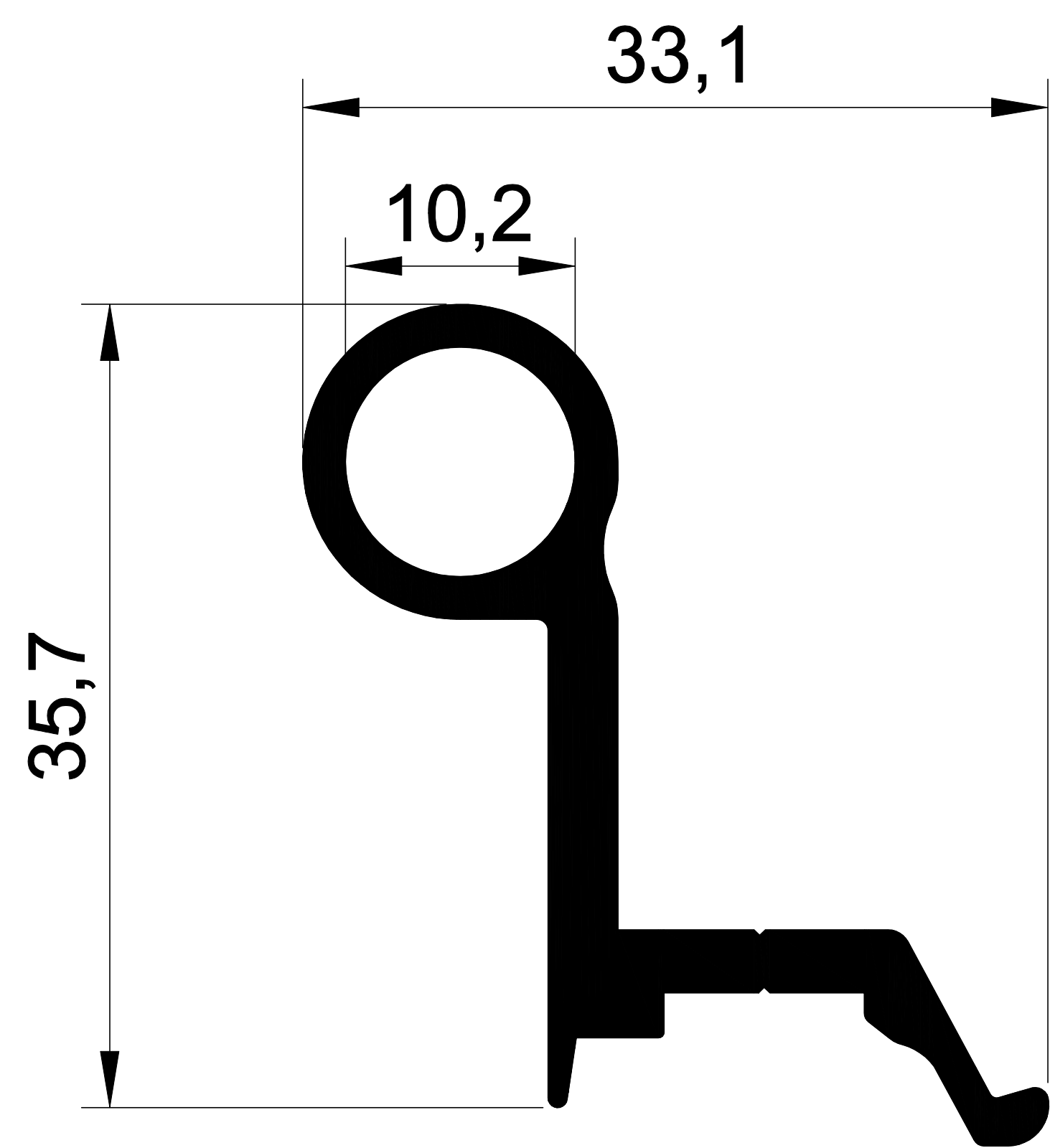
1254 0,550 Kg/m.
