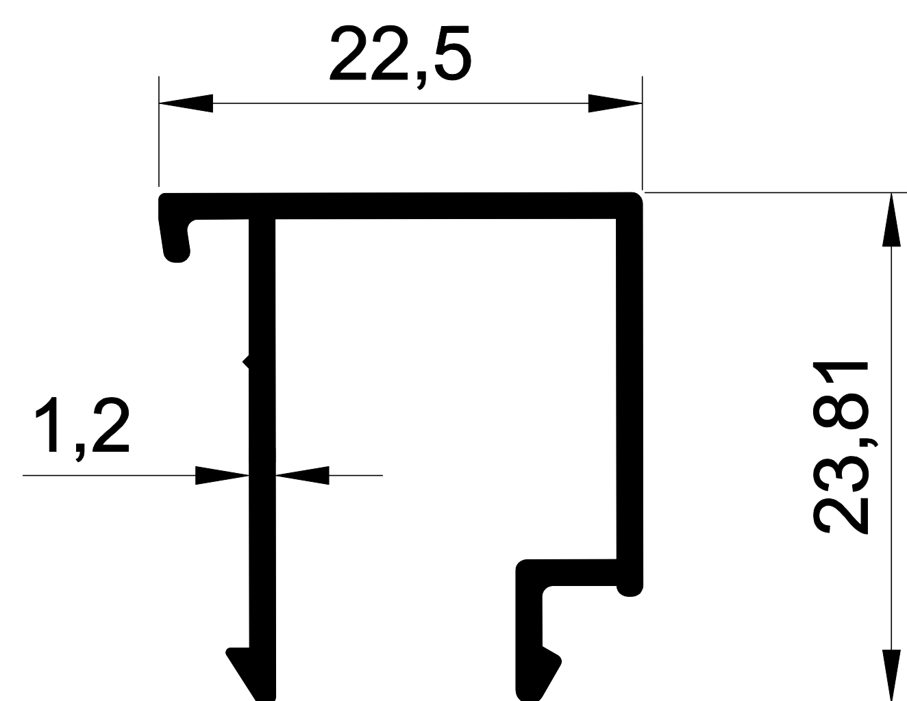
1204 0,249 Kg/m. SİSTEM ISI CAM ÇİTASI
