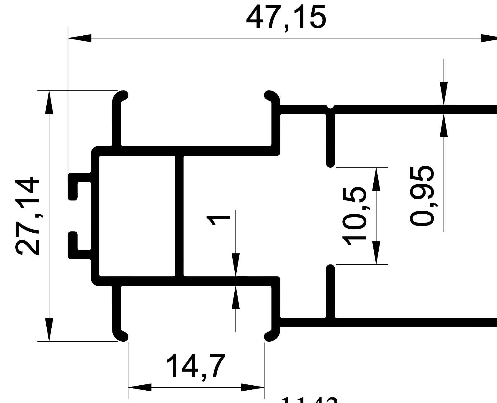
1143 0,409 Kg/m. PİLELİ SİNEKLİK KANAT
