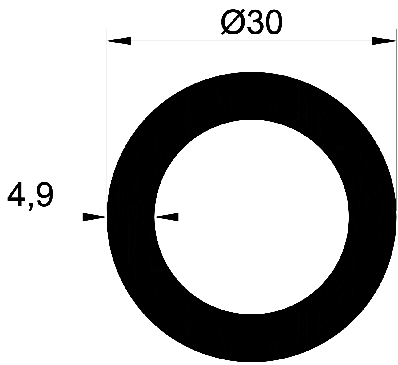
1002 0,393 Kg/m.
