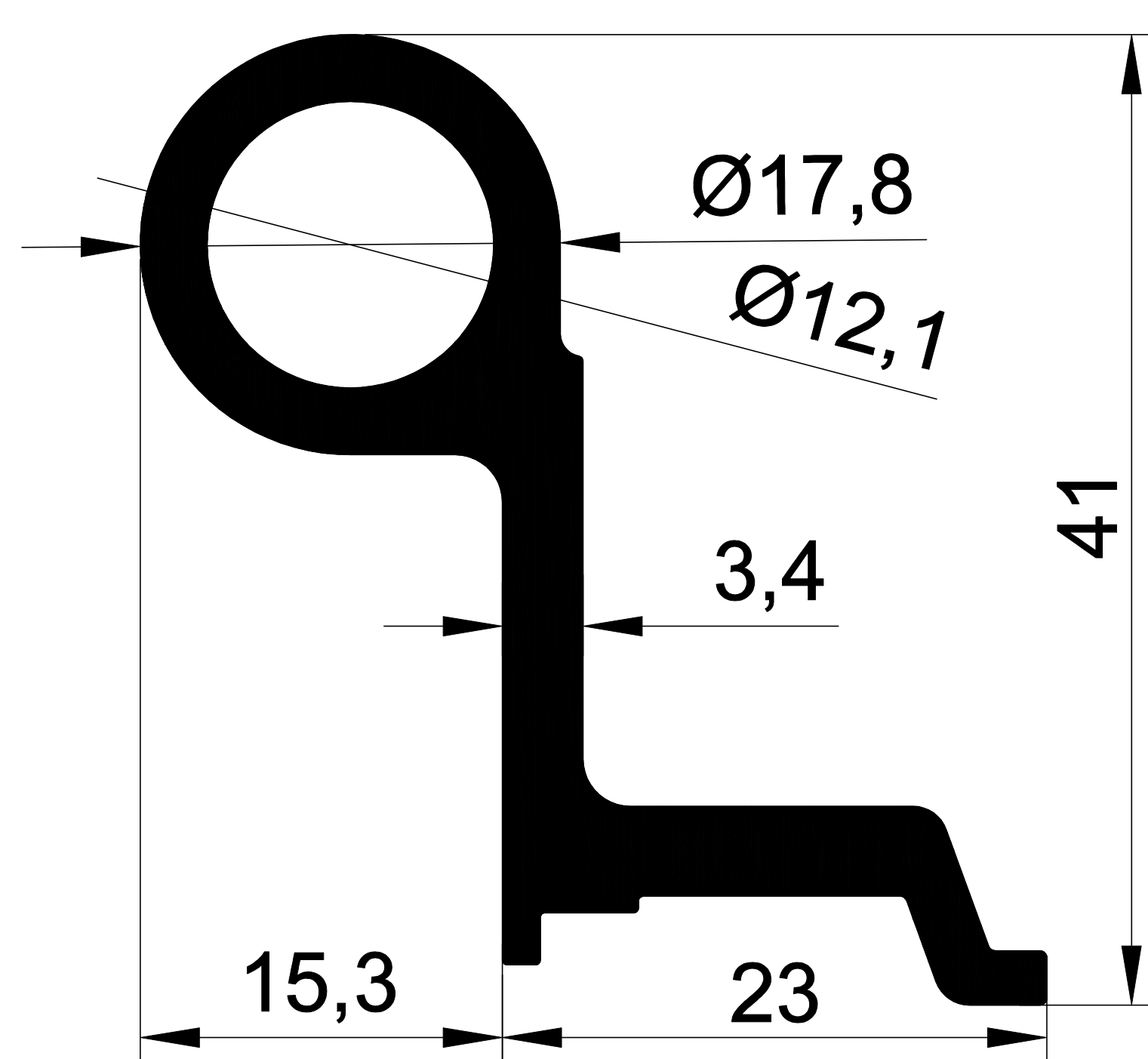
1463 0,819 Kg/m
