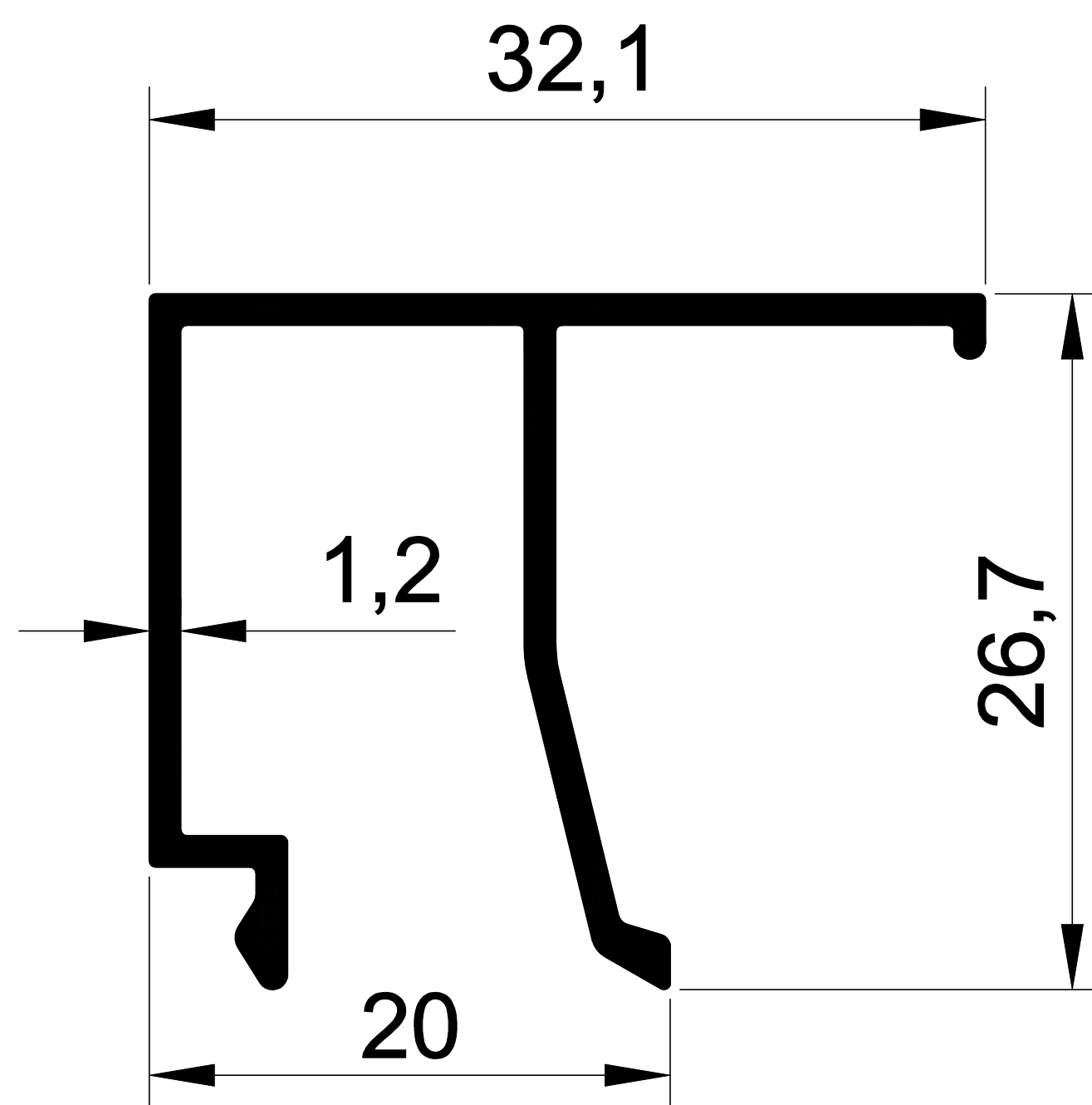
1404 0,297 Kg/m. BİM ISI CAM ÇİTASI
