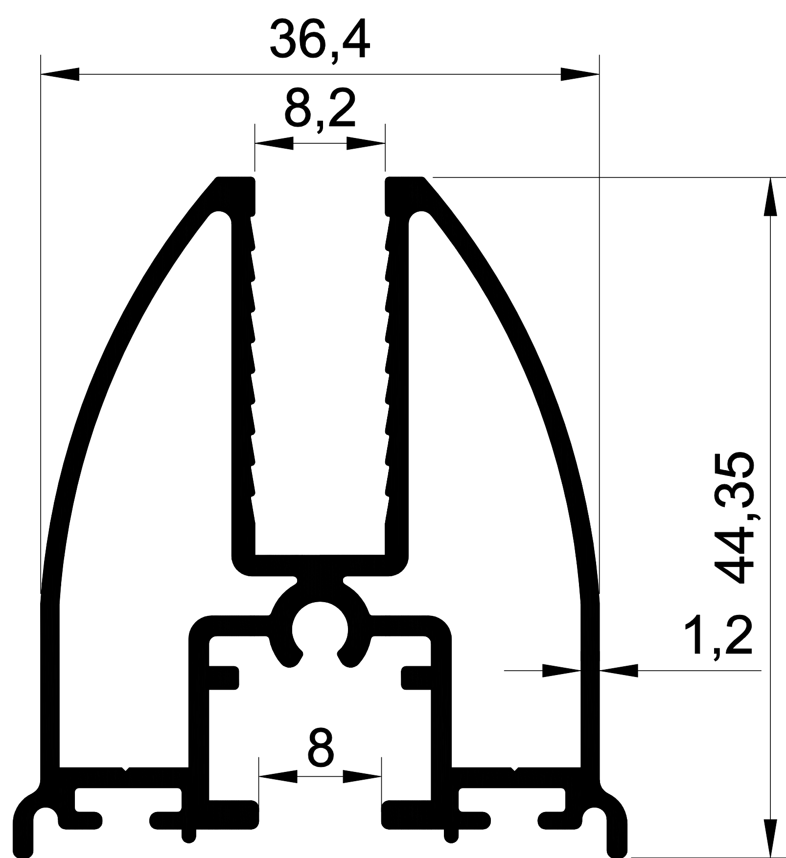
1191 0,881 Kg/m. FIRTINA KANAT
