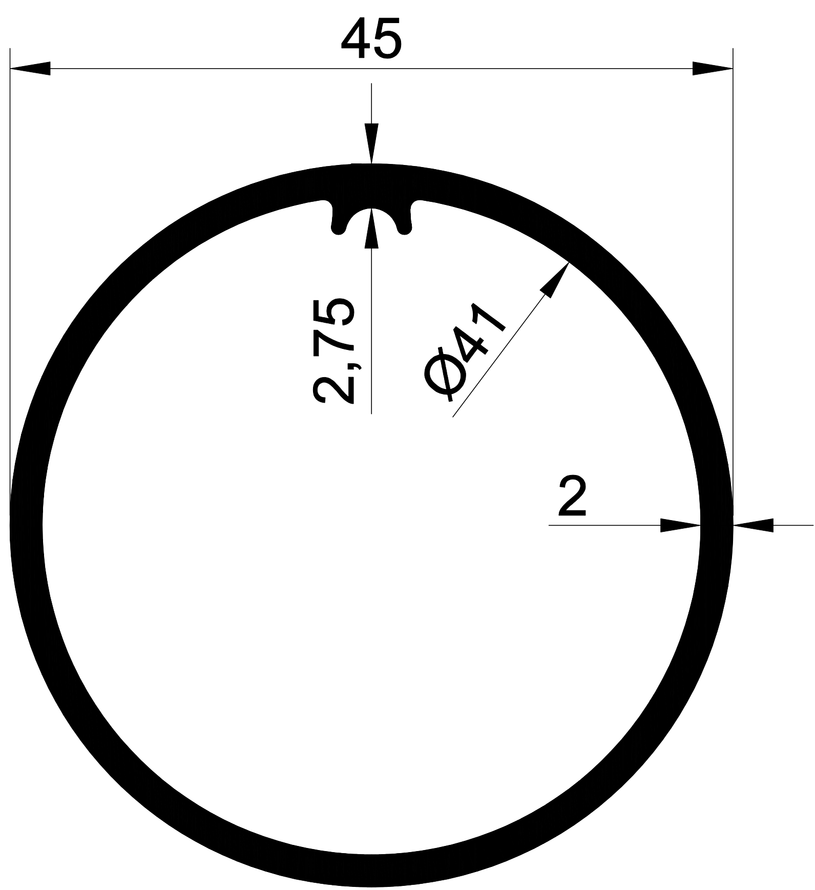
1018-C 0,752 Kg/m.
