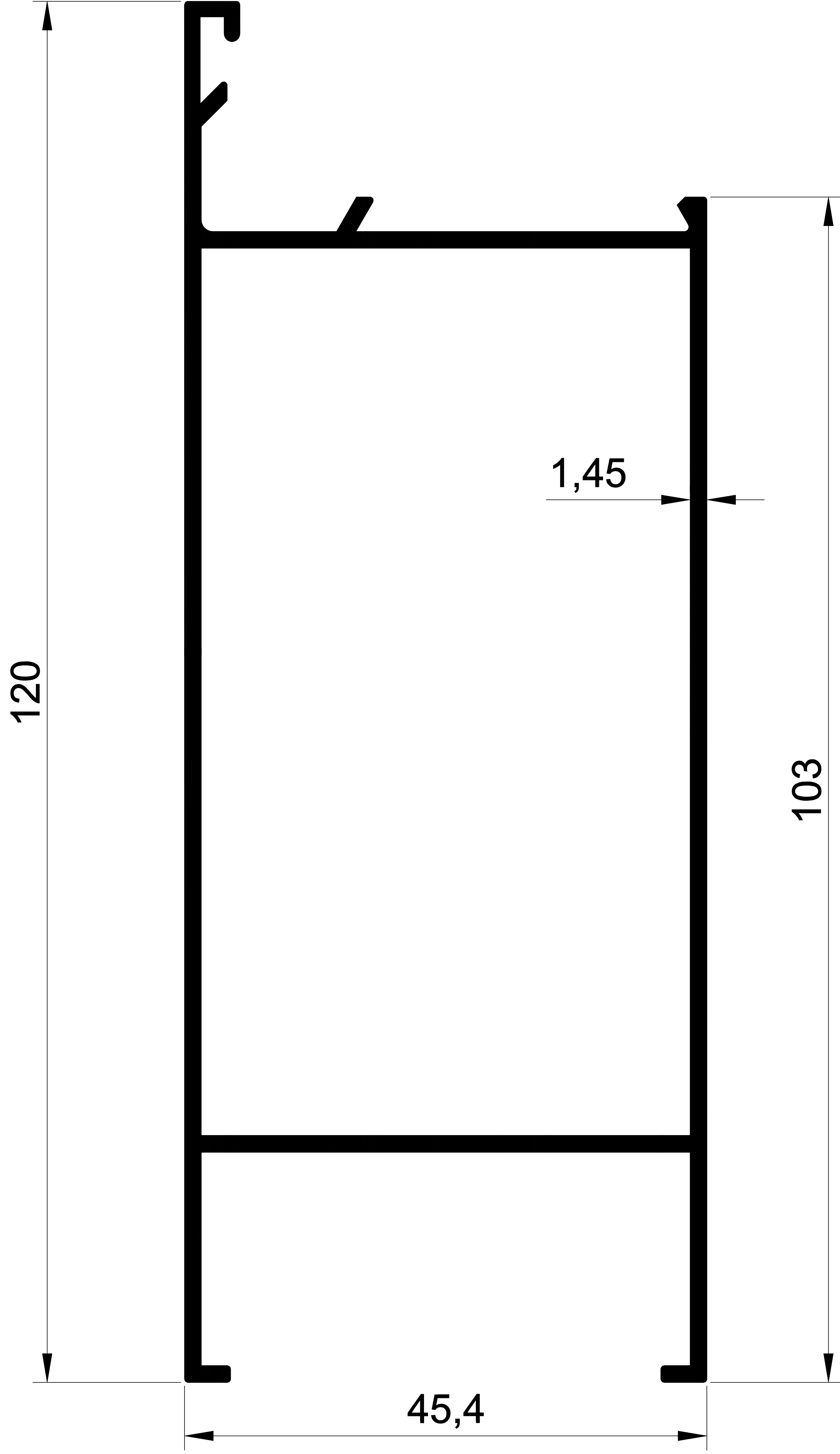
1107 1,279 Kg/m. ALDOKS ETEK
