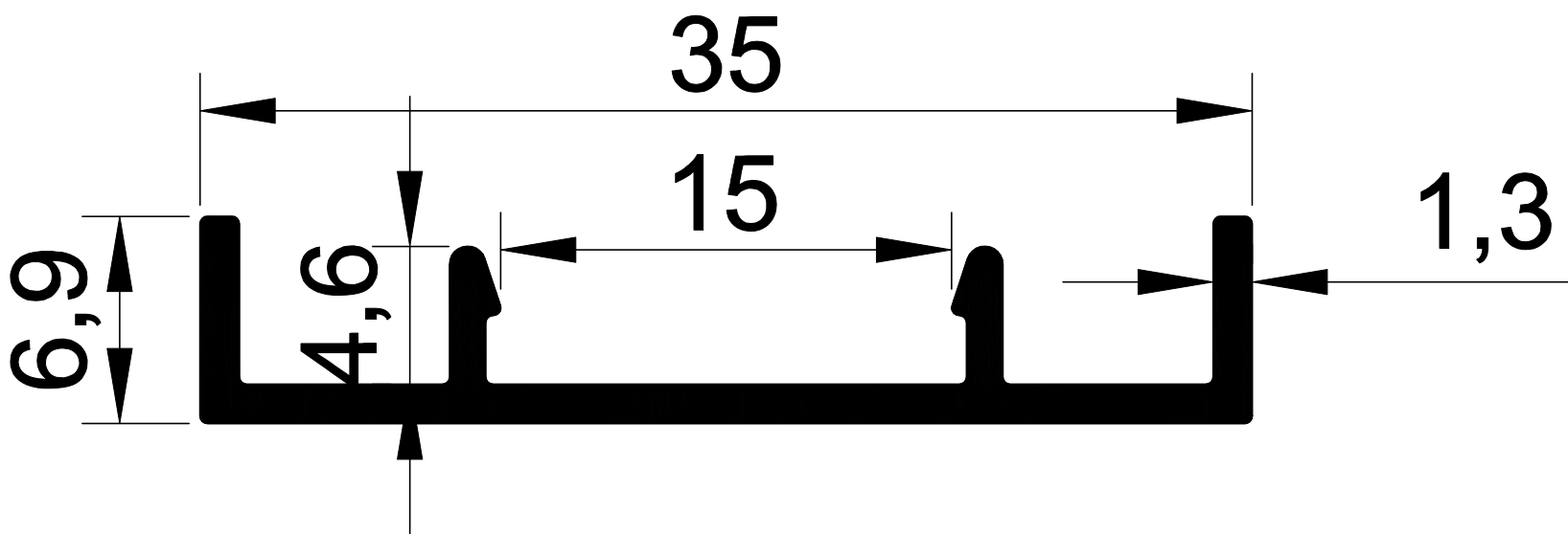
1416 0,195 Kg/m. JALUZİ OFİS BÖLME KAPAK
