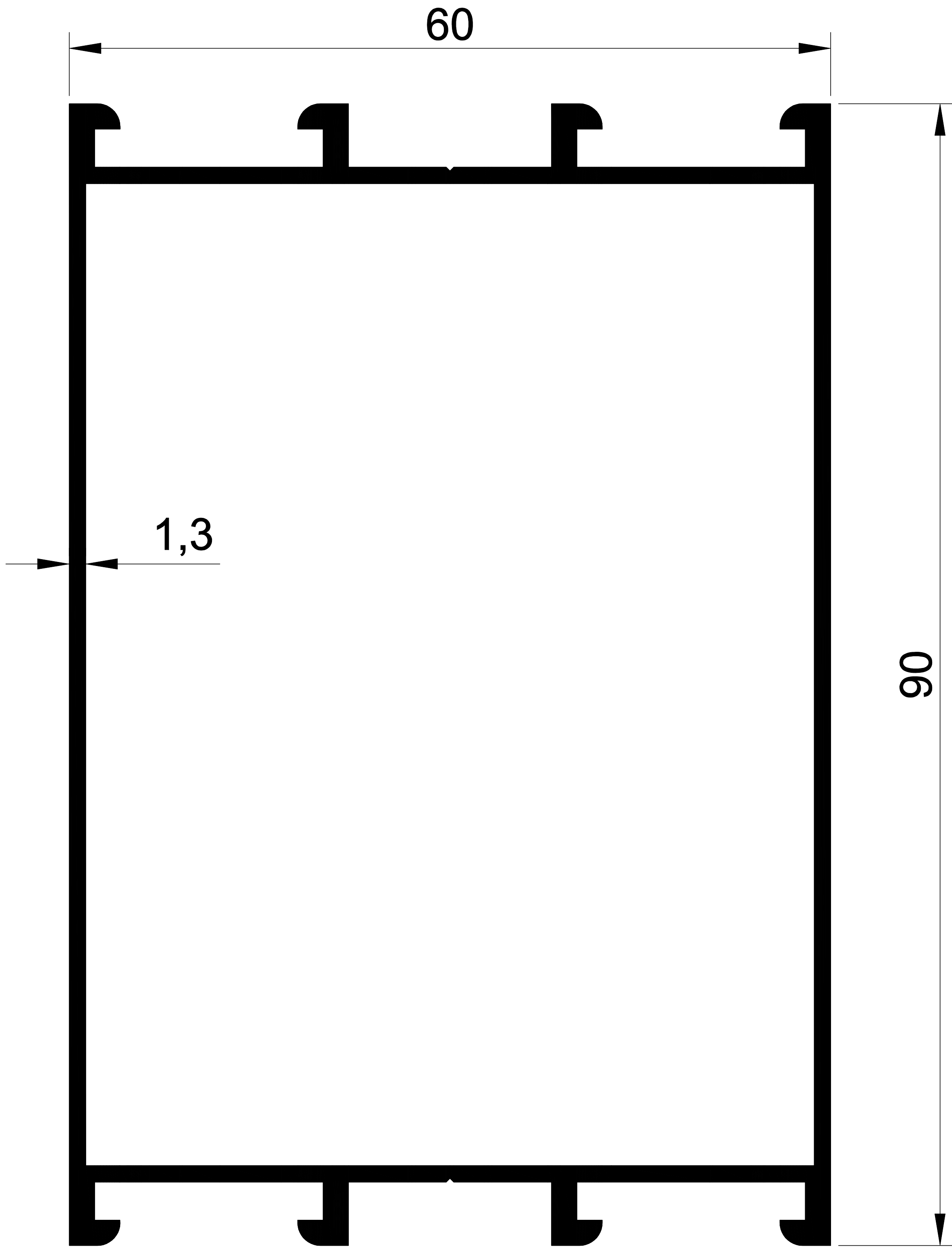
1084 1,255 Kg/m. C-90 KASA
