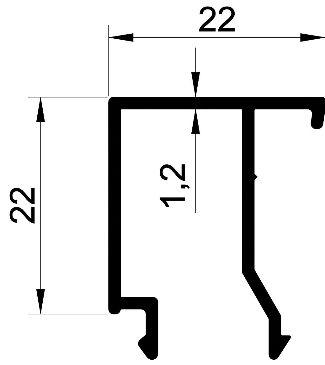
-55- 2008 0,264 Kg/m SİSTEM 55 ÇİFT CAM ÇITASİ
