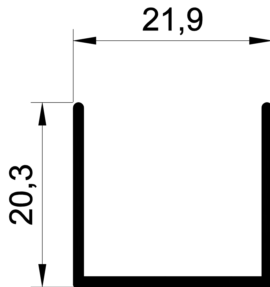
1158 0,187 Kg/m. 20 mm U PROFİL (KOMBİ U'SU)
