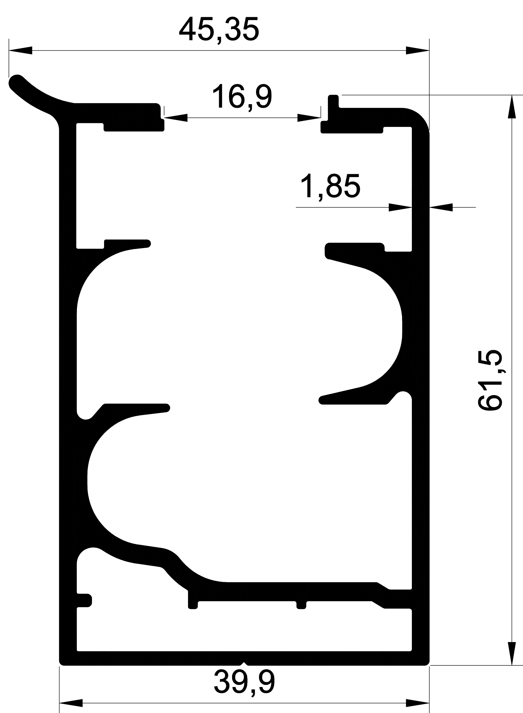
1290 1,428 Kg/m. BKS ÜSTTEN DAMLALIKLI KASA
