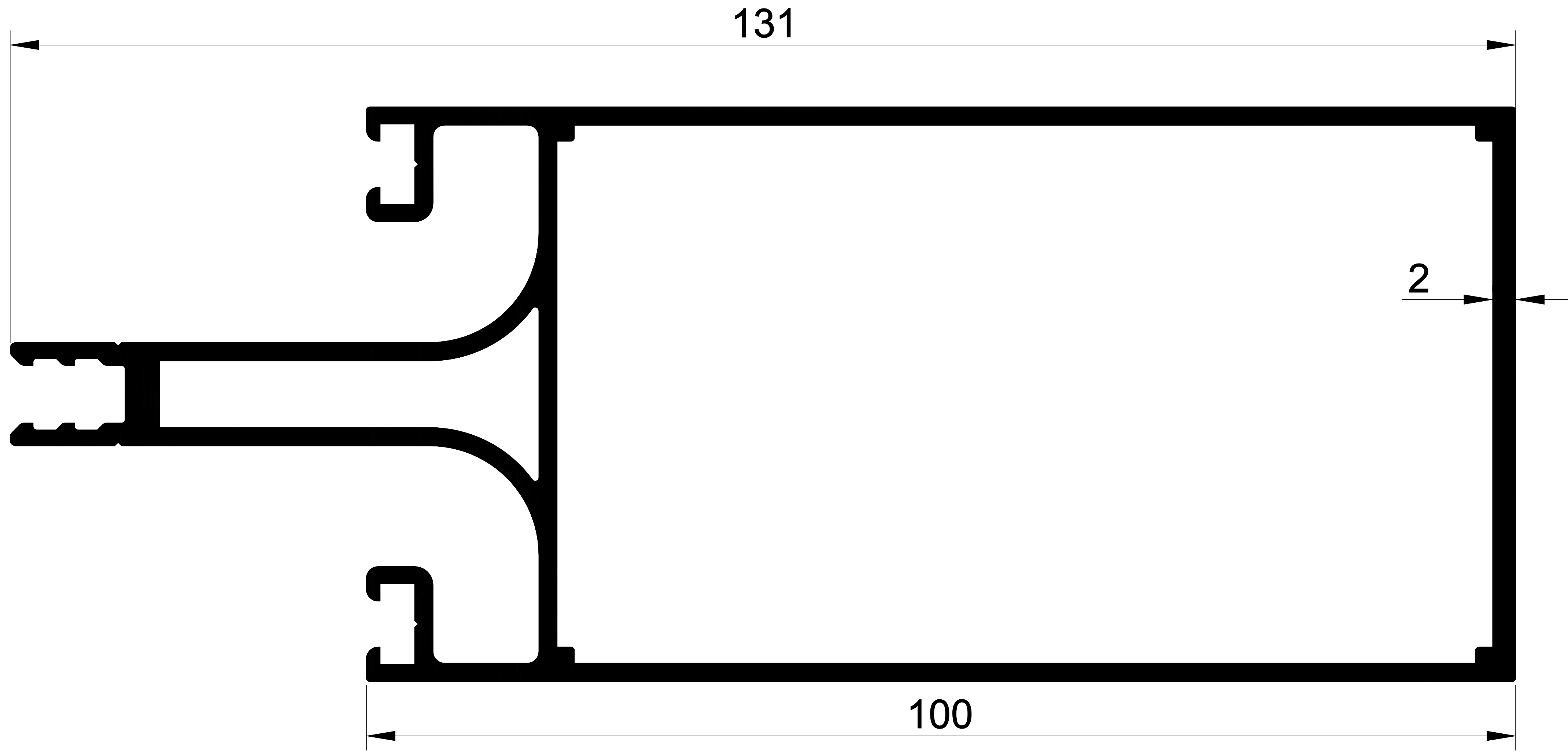
100'LÜK CEPHE PROFİLİ UZUN GAGA
