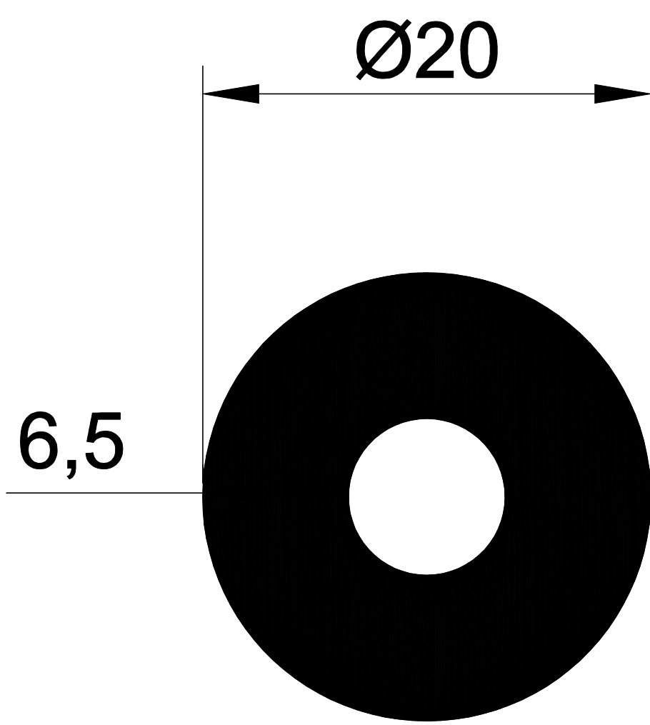
1030 0,748 Kg/m.
