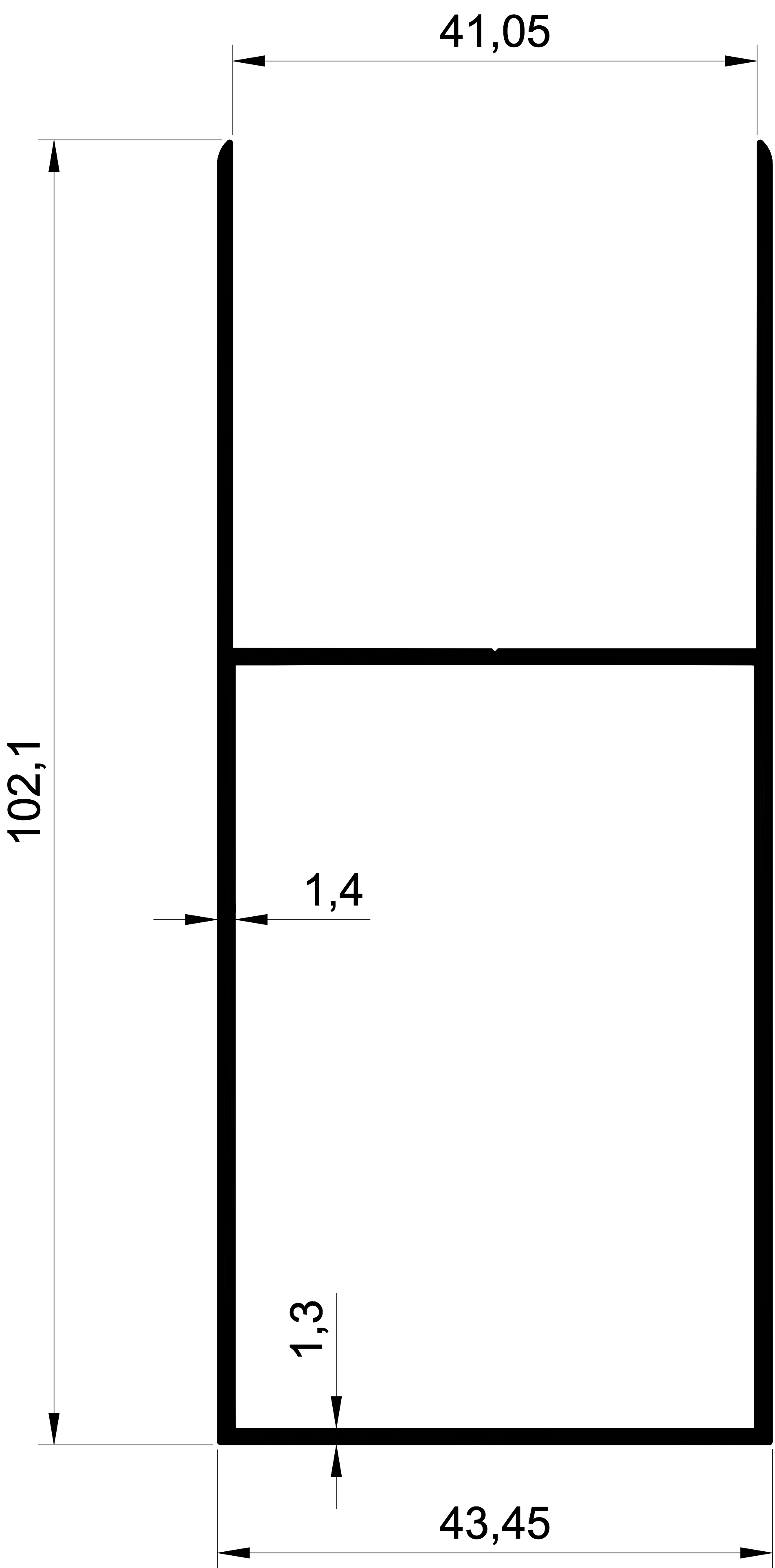
1150 1,008 Kg/m. CAM BALKON ETEK
