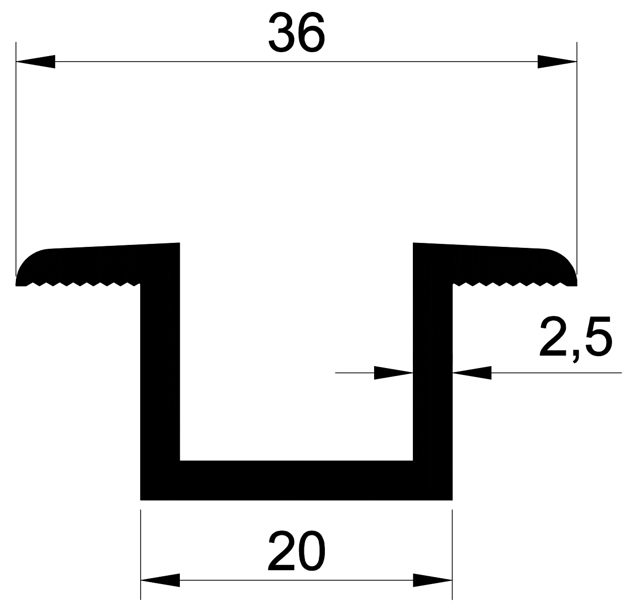
1430 0,420 Kg/m GES PANEL TUTUCU APARATI ORTA
