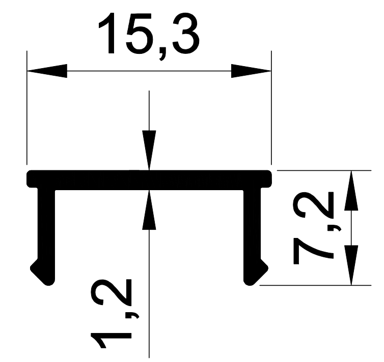
1268 0,084 Kg/m GEMİCİ KAPAĞI
