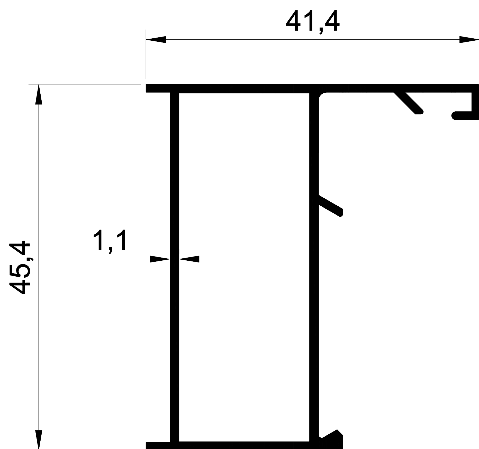
1103 0,458 Kg/m. ALDOKS DAR KASA
