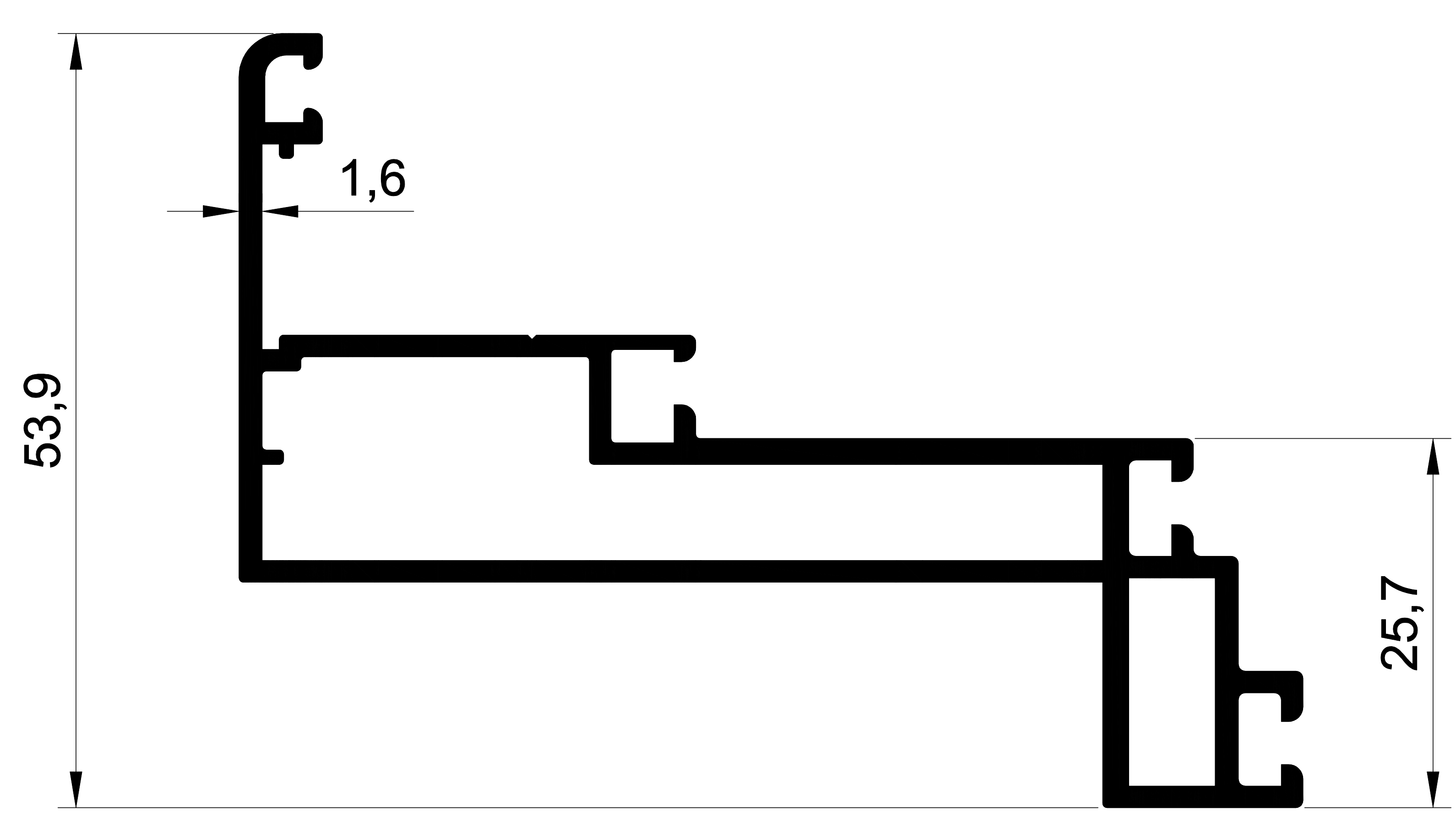
1392 1,343 Kg/m. CEPHE KANAT KASASI
