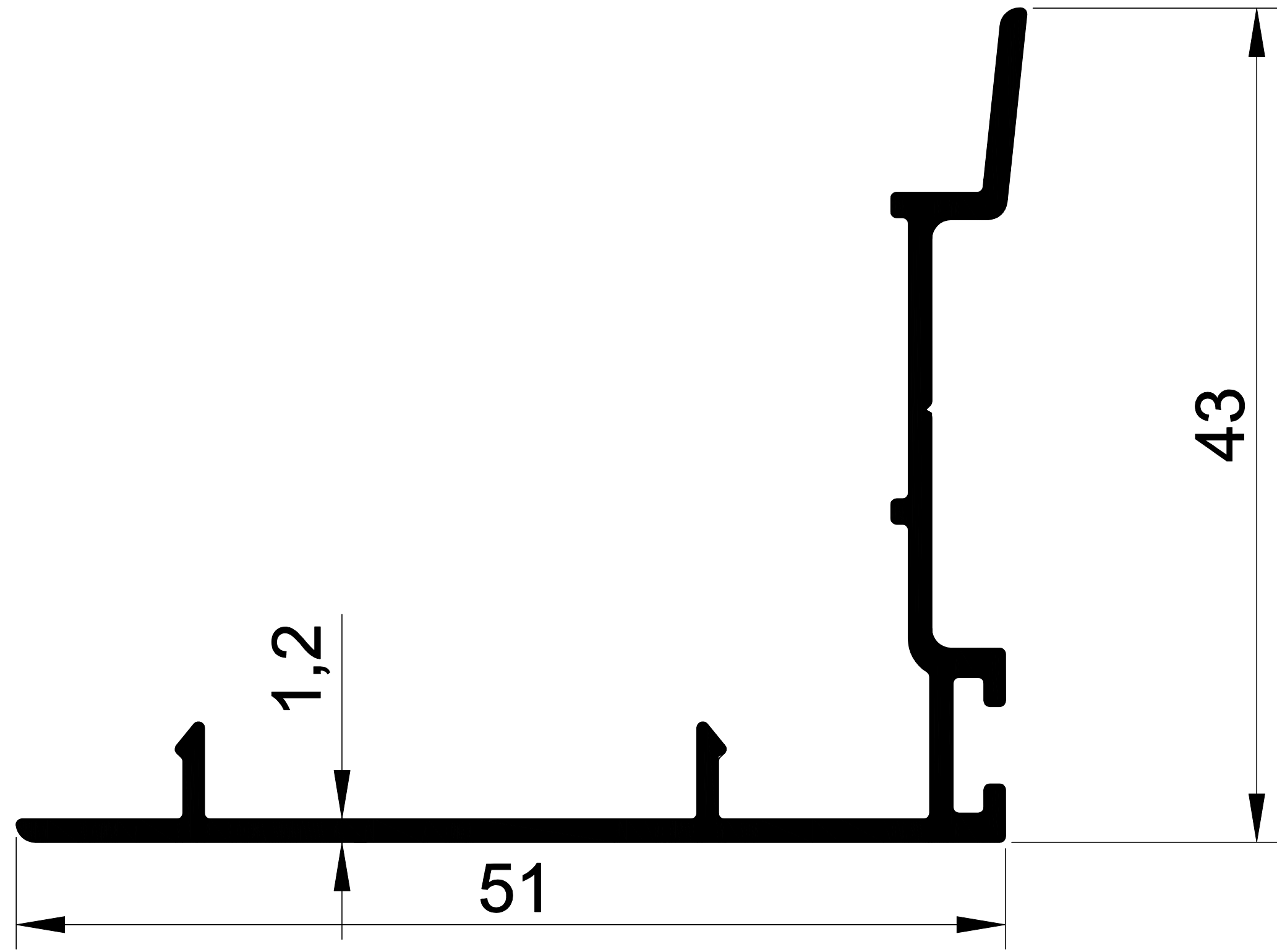
1387 0,379 Kg/m. 100'LÜK TUBA KENET
