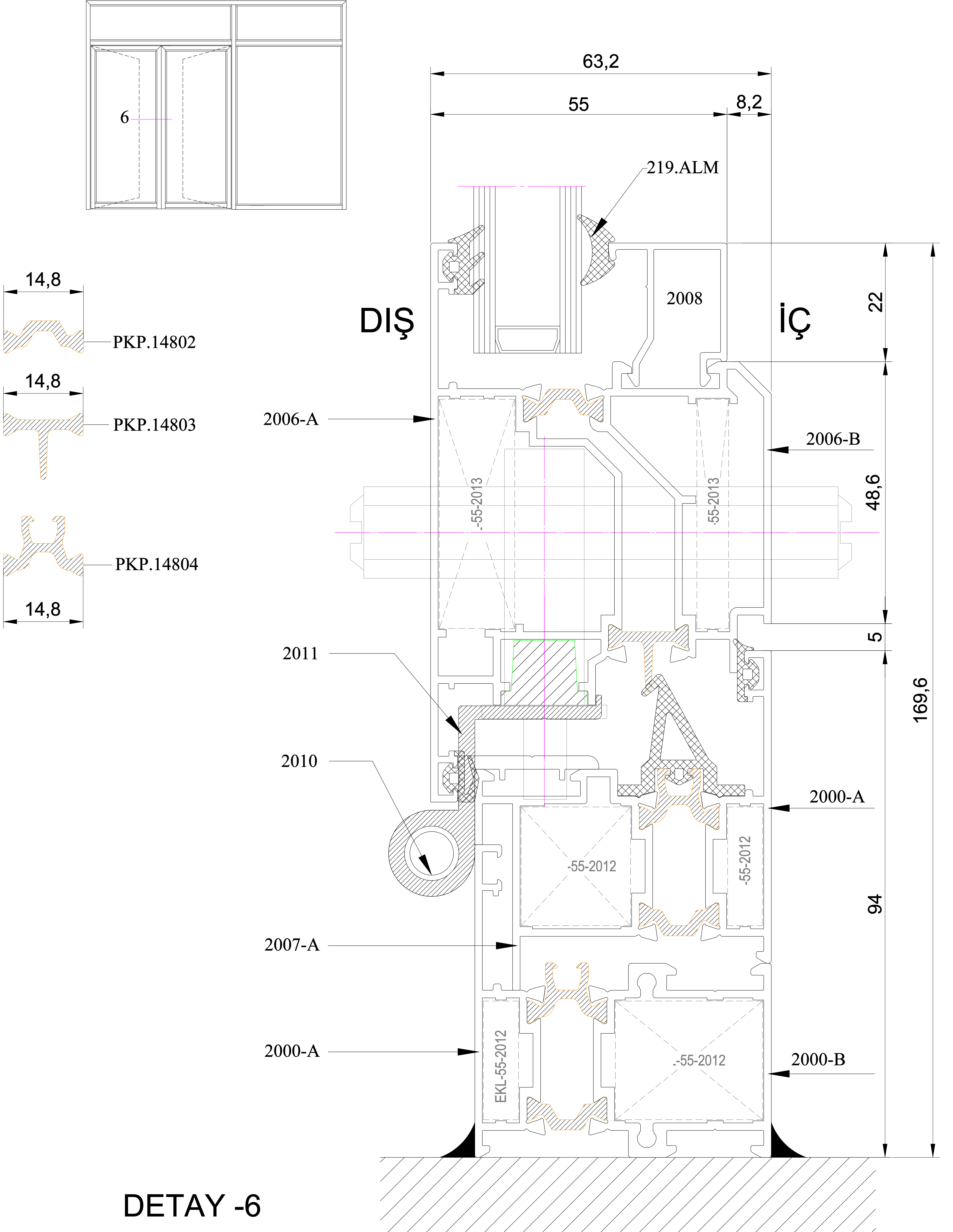
DIŞA AÇILIR ÇİFT KAPI DETAYI
