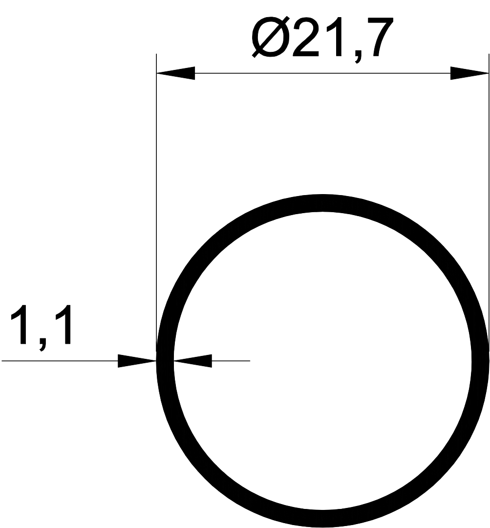
1056 0,192 Kg/m.
