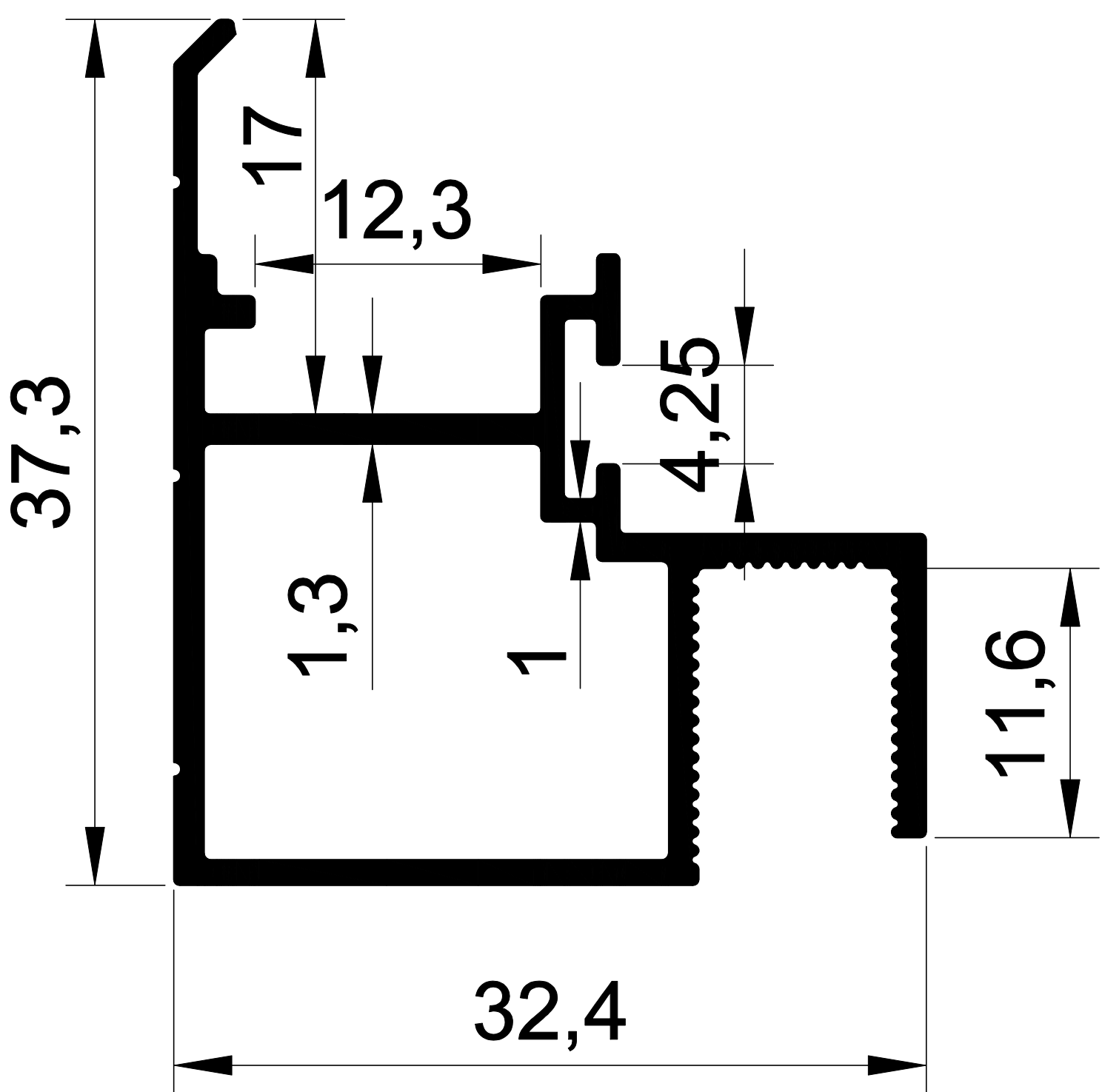
1449 0.440 Kg/m. C.B KOL PROFİLİ-2
