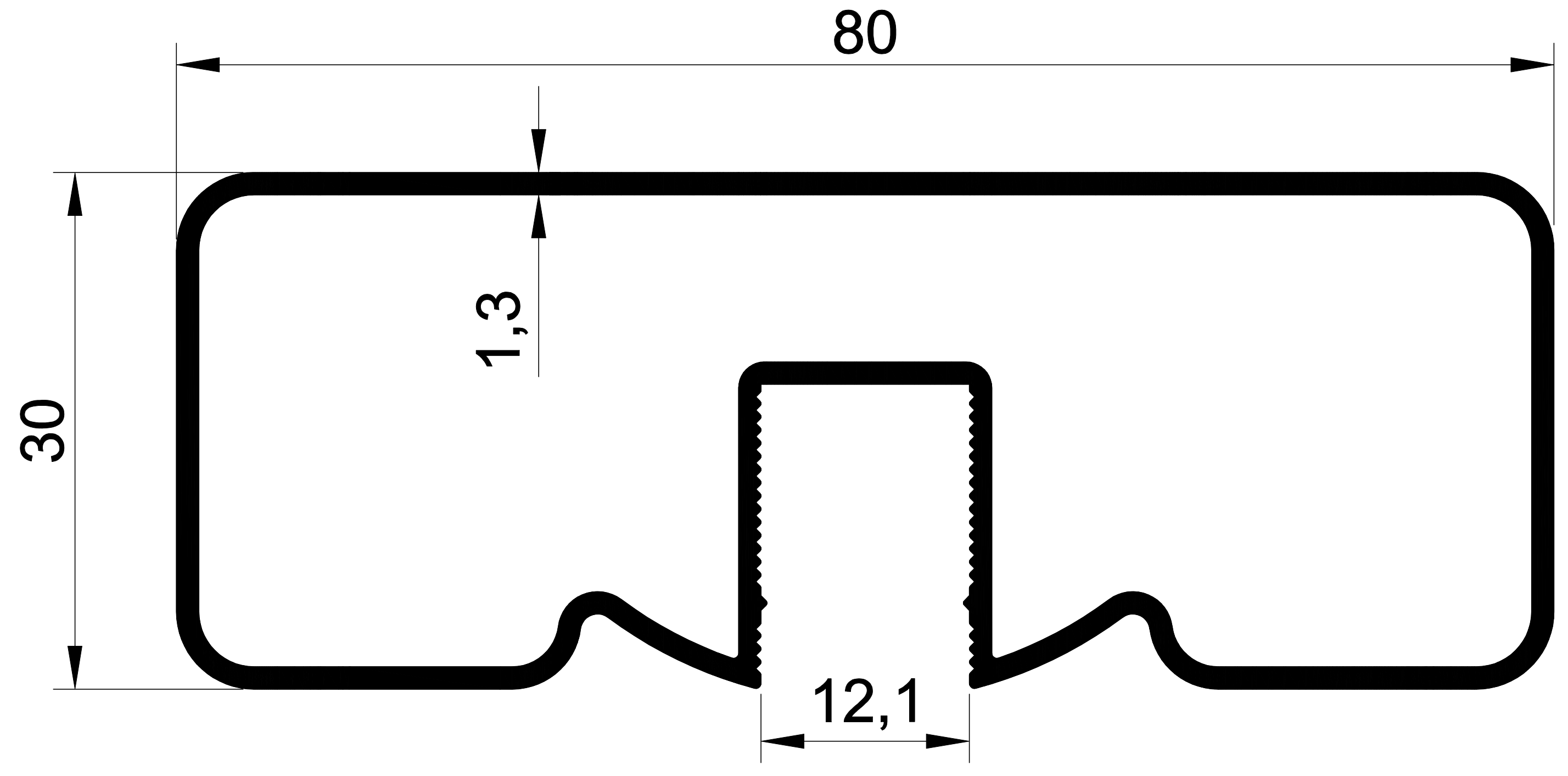
1130 0,870 Kg/m. 30X80 ORTADAN CAMLI
