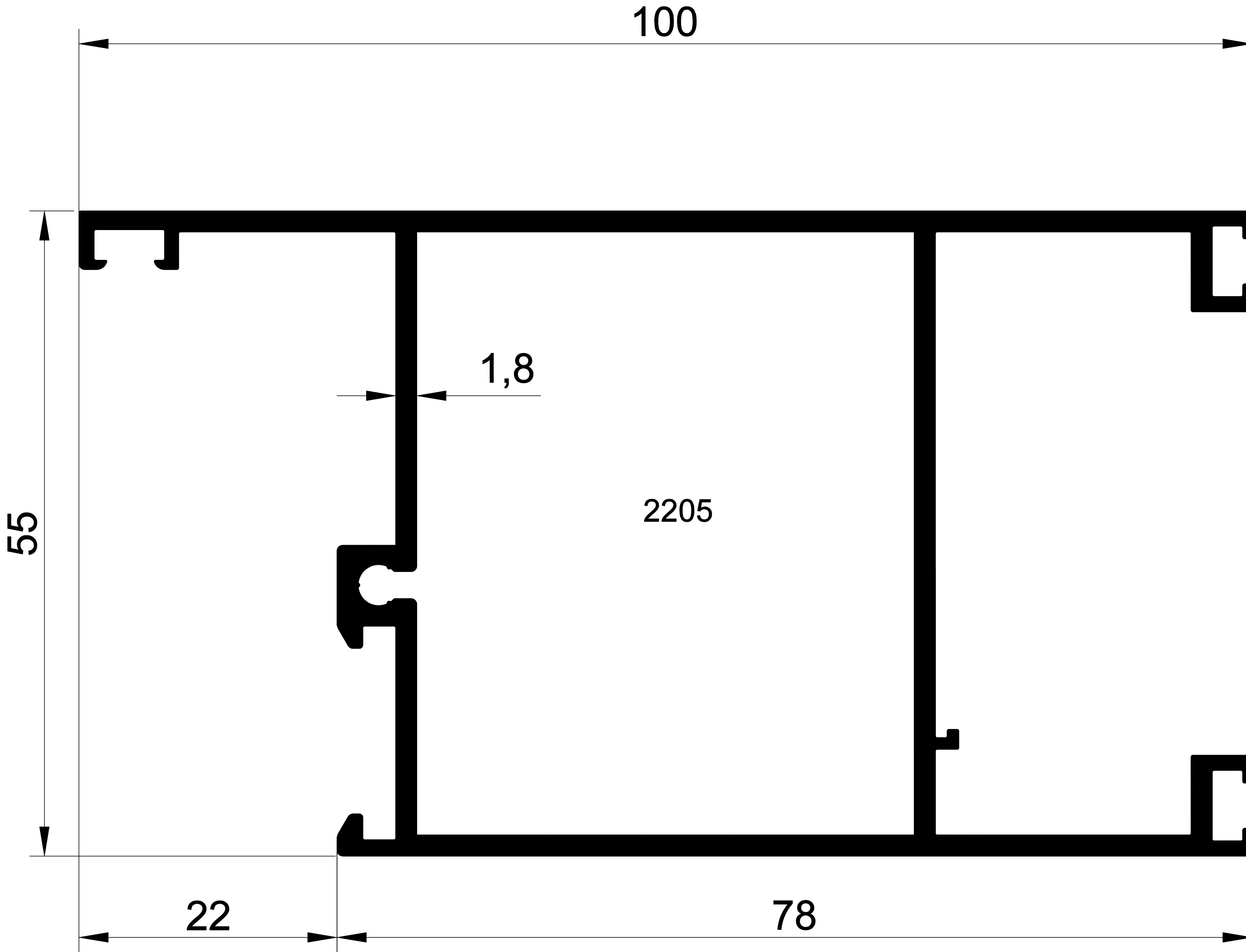
EK-55- 2205 1,561 Kg/m SİSTEM 55 YALITIMSIZ ETEK
