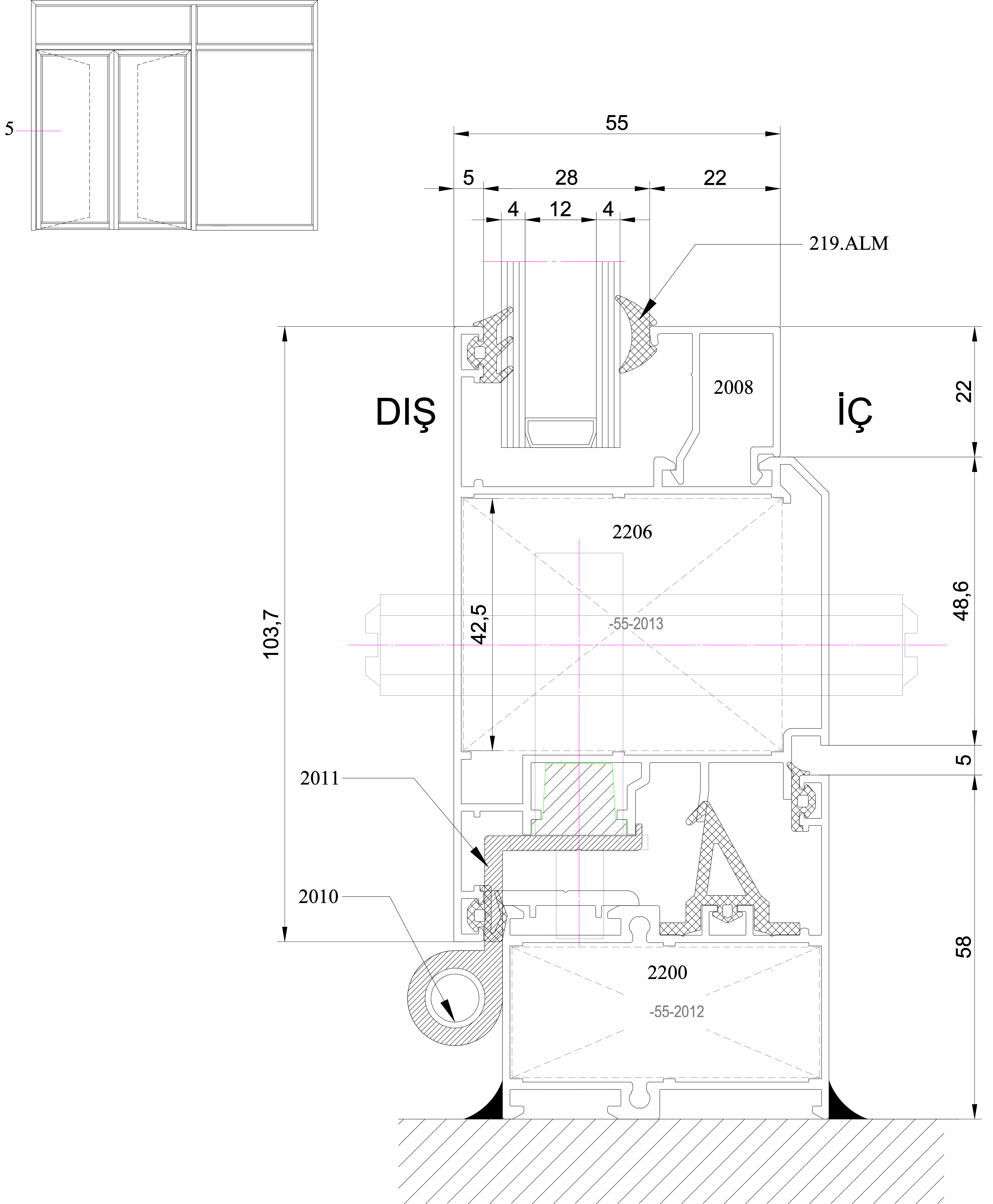
DIŞA AÇILIR ÇİFT KAPI DETAYI
