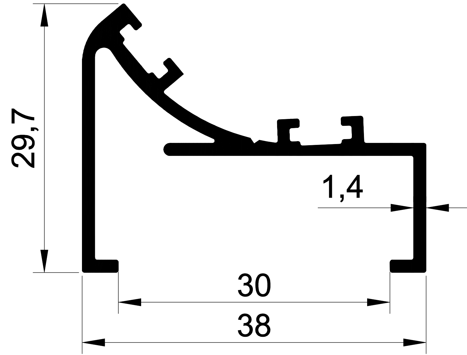
1364 0,430 Kg/m. ISI YALITIM EKSENAL KÖŞE DÖNÜŞ
