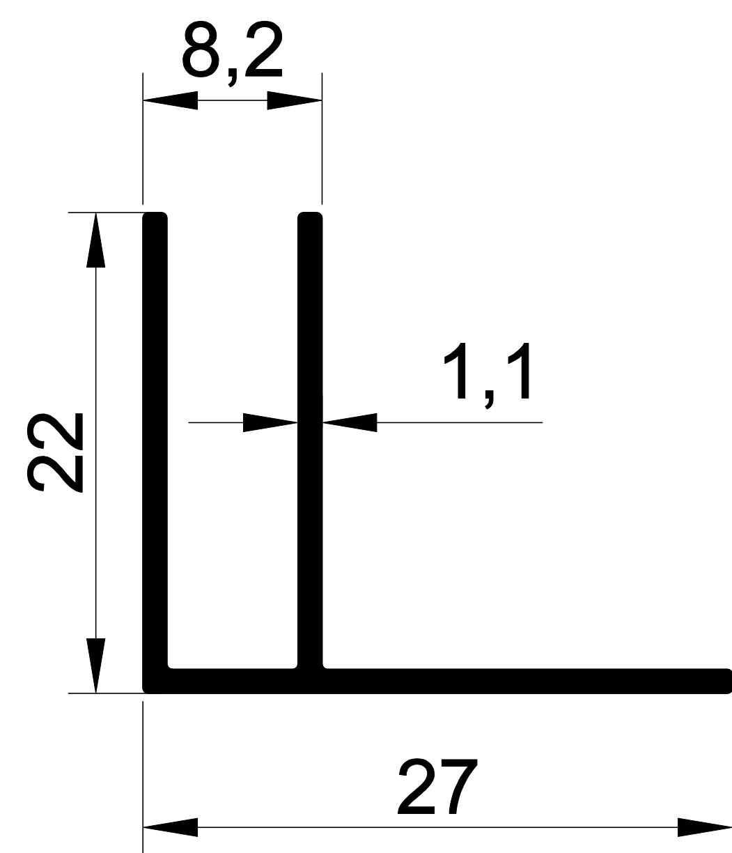
1409 0,205 Kg/m. MOBİLYA F PROFİLİ
