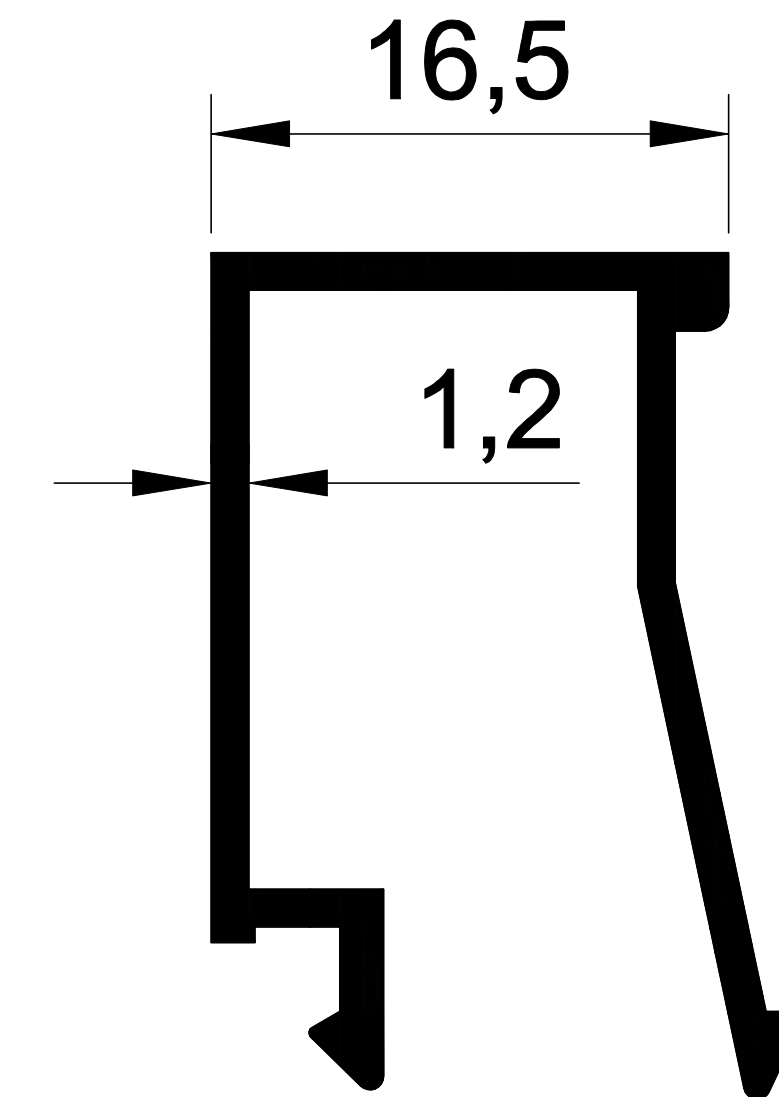
1085 0,249 Kg/m. C-60 ISI CAM ÇİTASI
