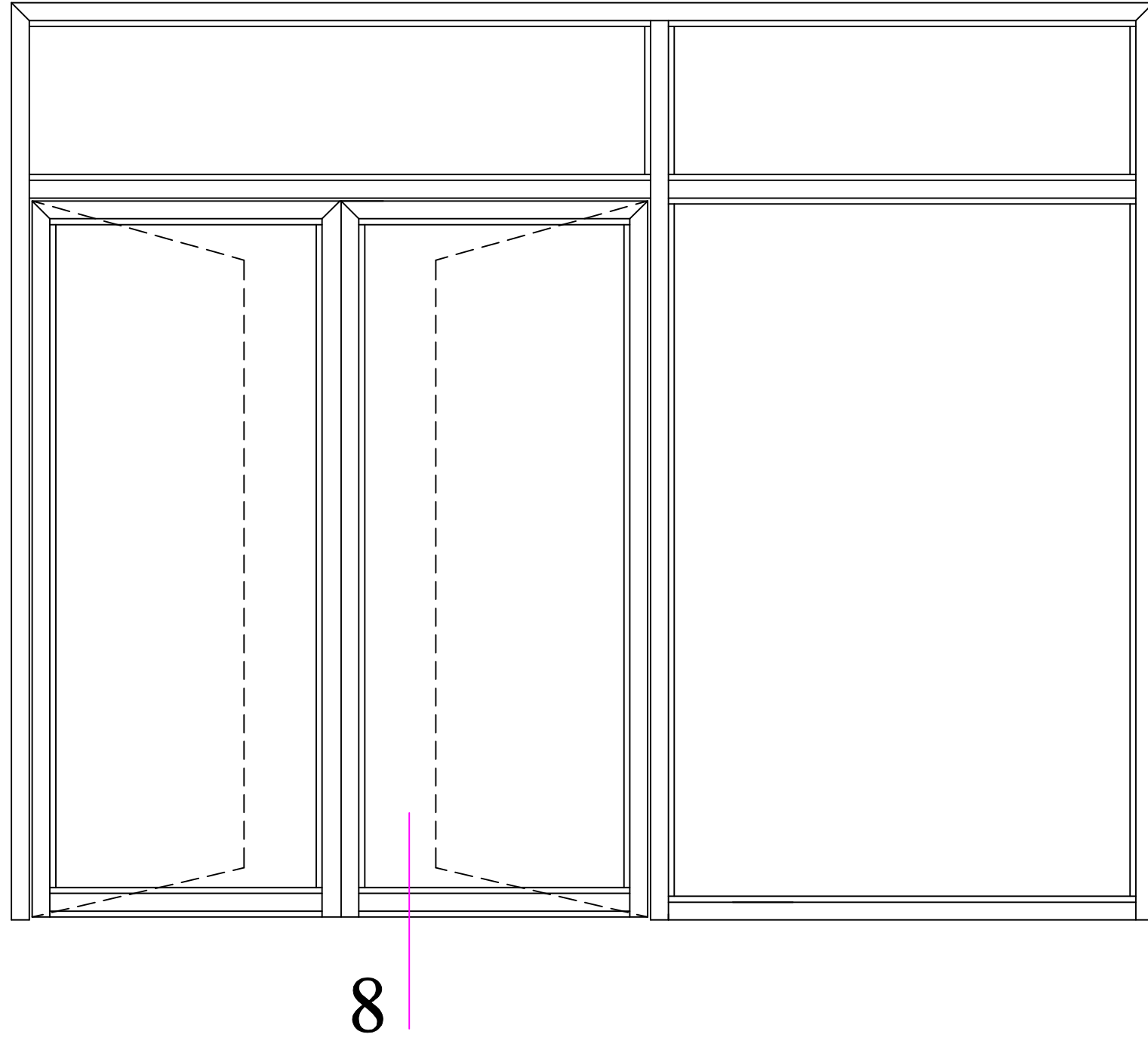
KAPI PENCERE DETAYI
