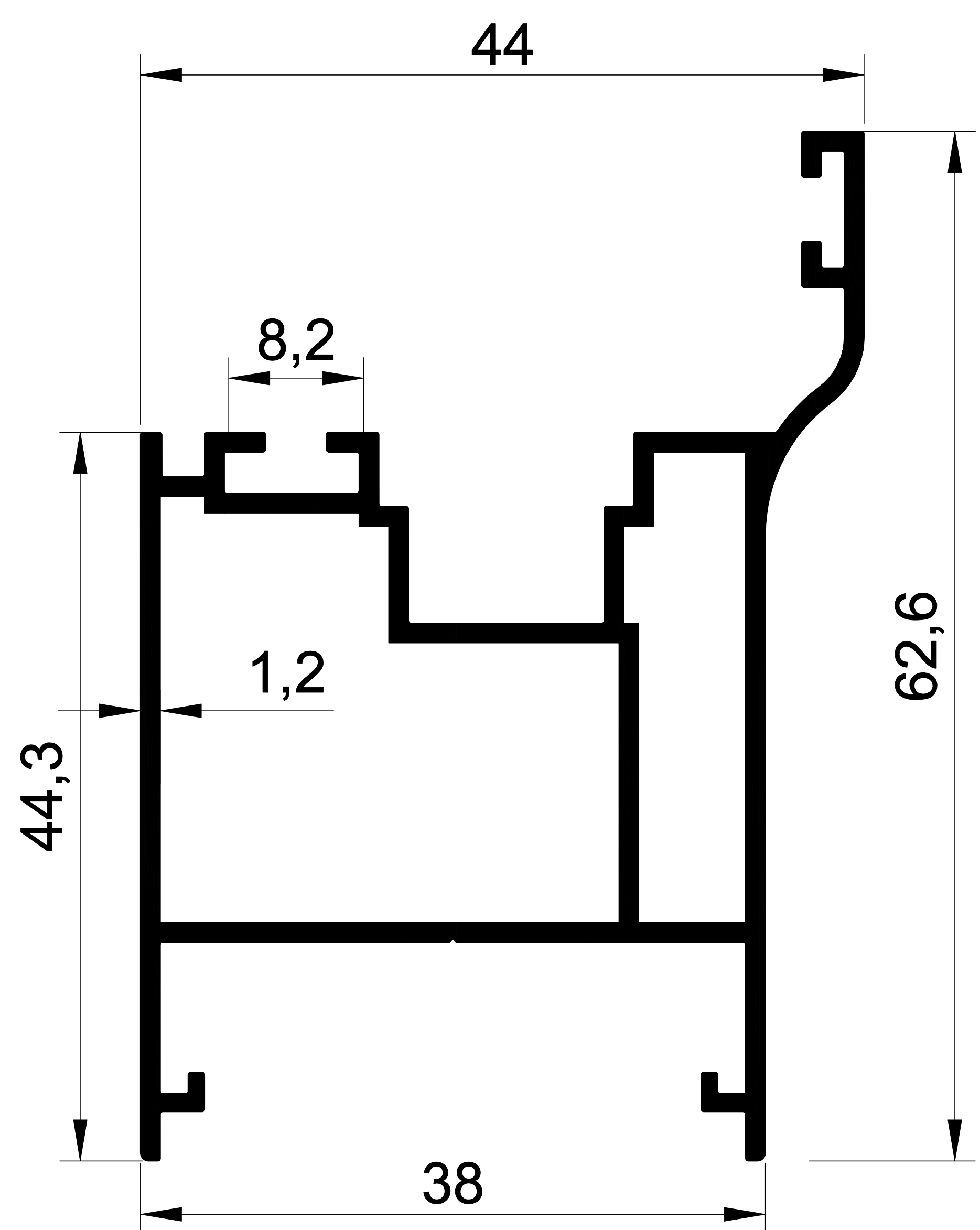
- 2300 0,806 gr/m ISICAMLI CAM BALKON PROFİLLERİ
