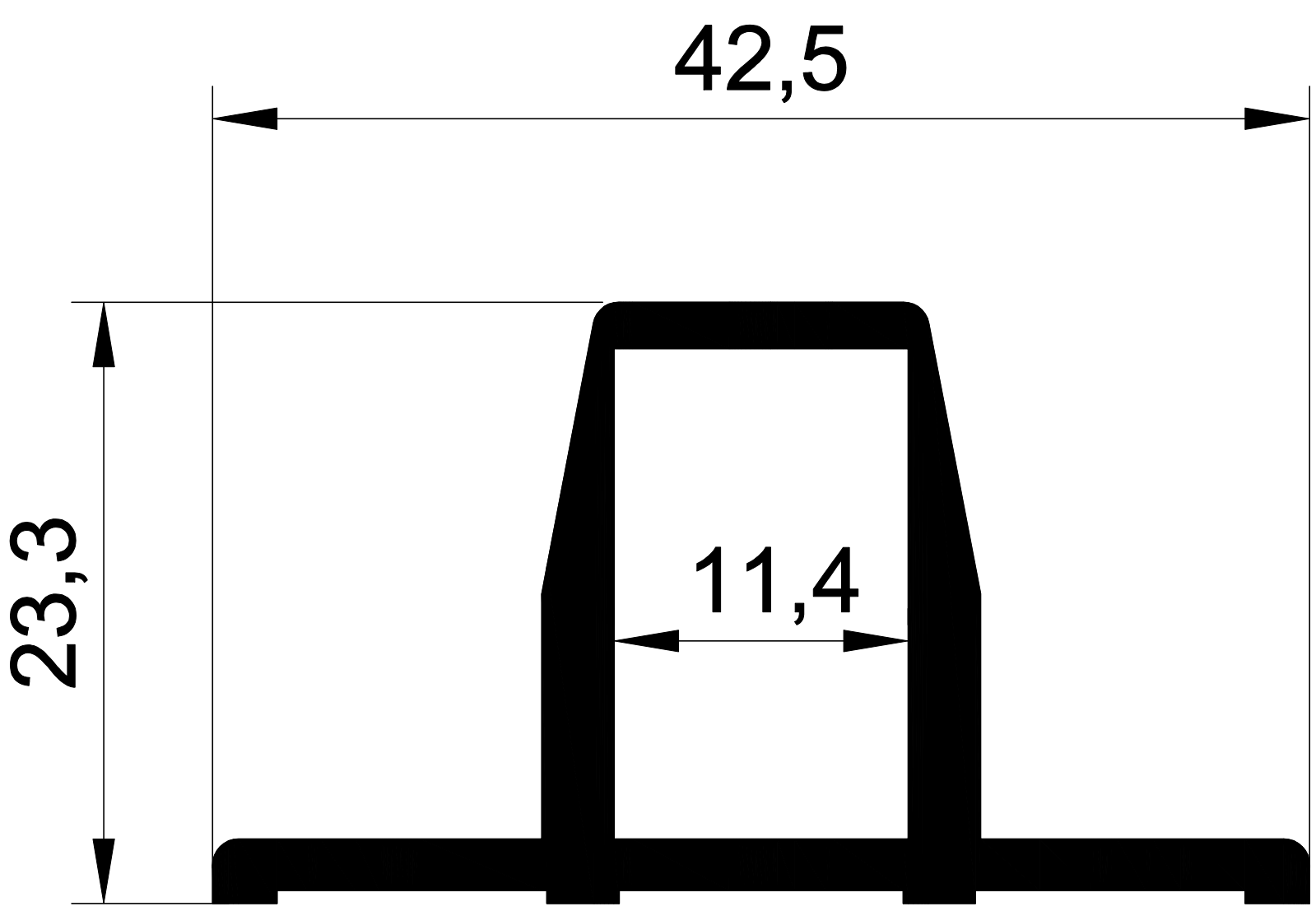
1231 0,548 Kg/m.
