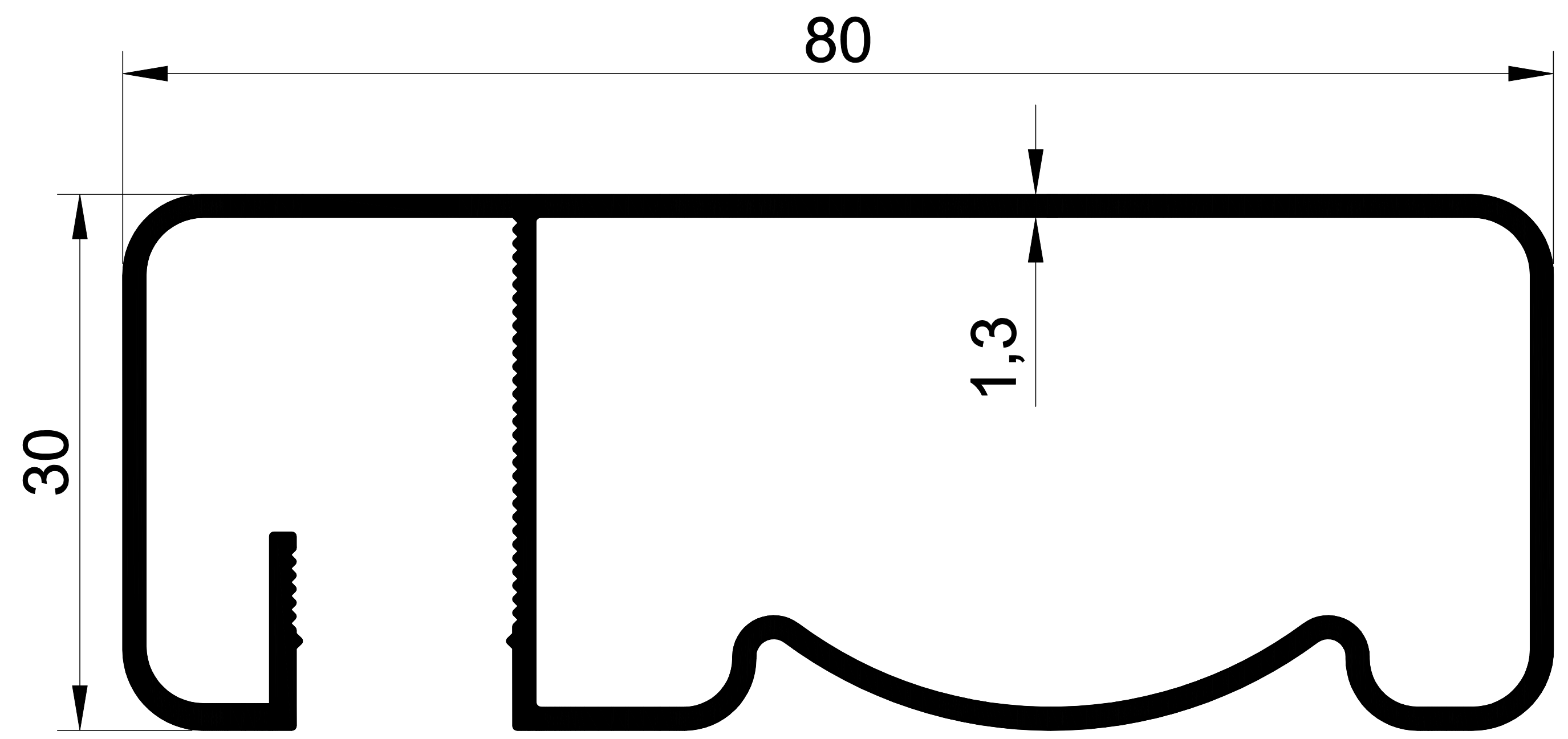
1133 0,852 Kg/m. 30X80 YANDAN CAMLI
