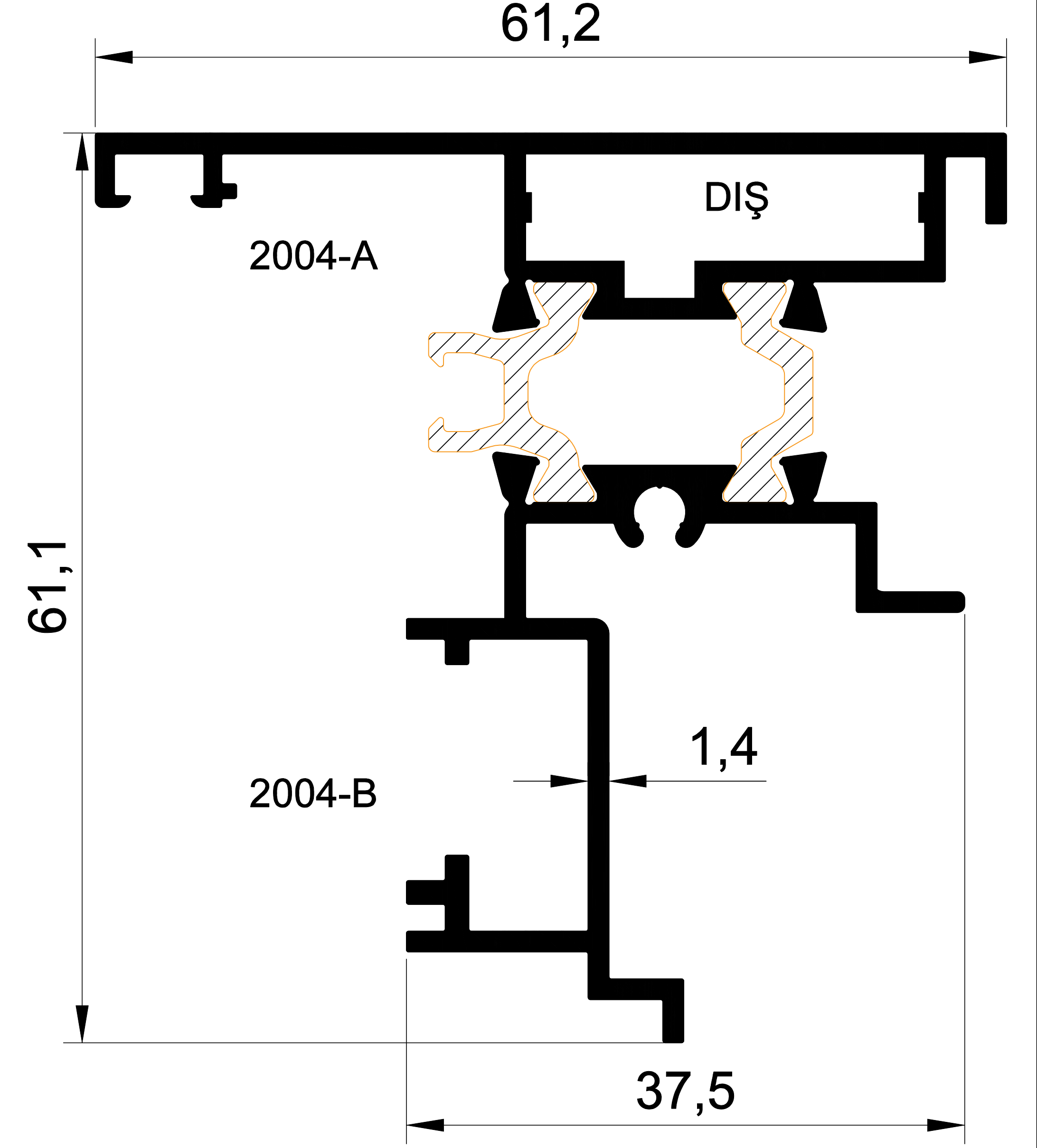
-55- 2004 1,039 Kg/m SİSTEM 55 ISI YALITIM ÇİFT KANAT ADAPTÖR
