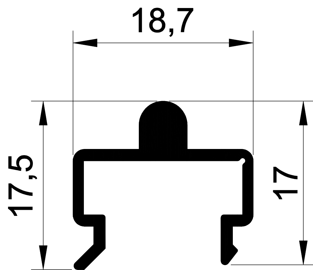
1193 0,203 Kg/m DAR TUBA RAY
