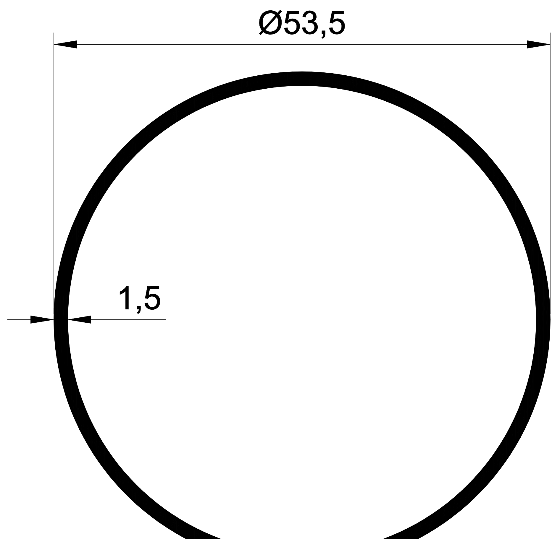
1032 0,664 Kg/m.
