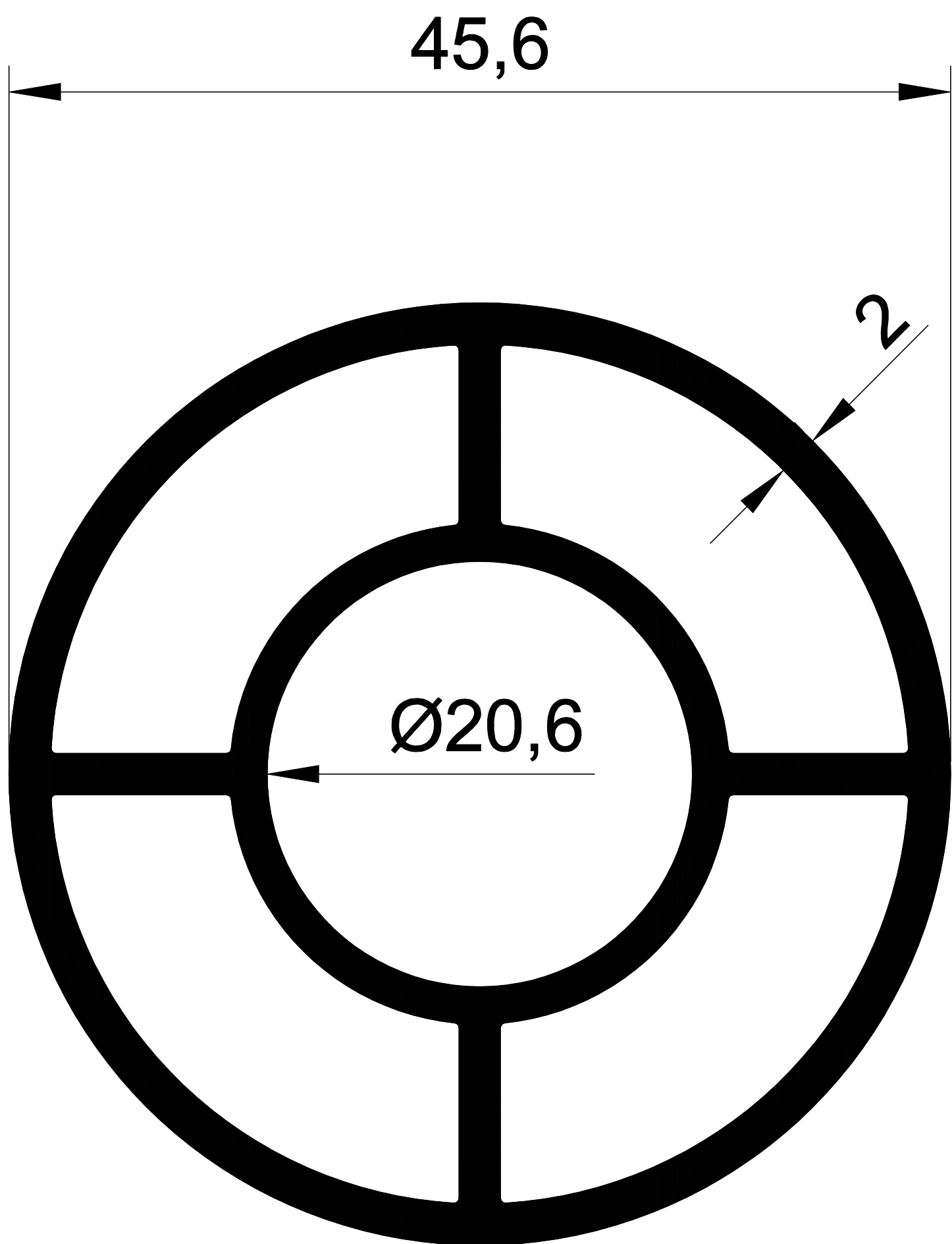
1211 1,274 Kg/m.
