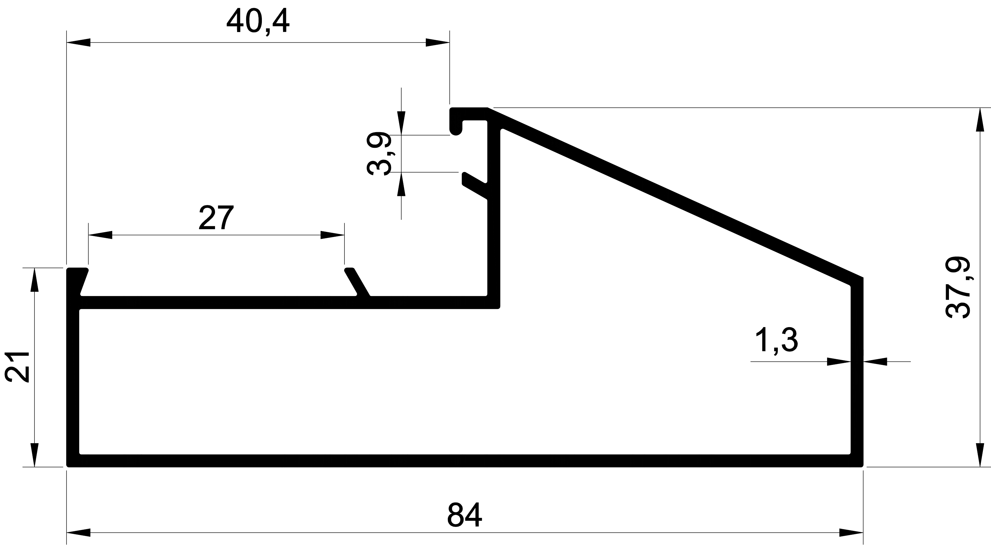
1415 0,846 Kg/m. JALUZİ OFİS BÖLME KAPI KASASI
