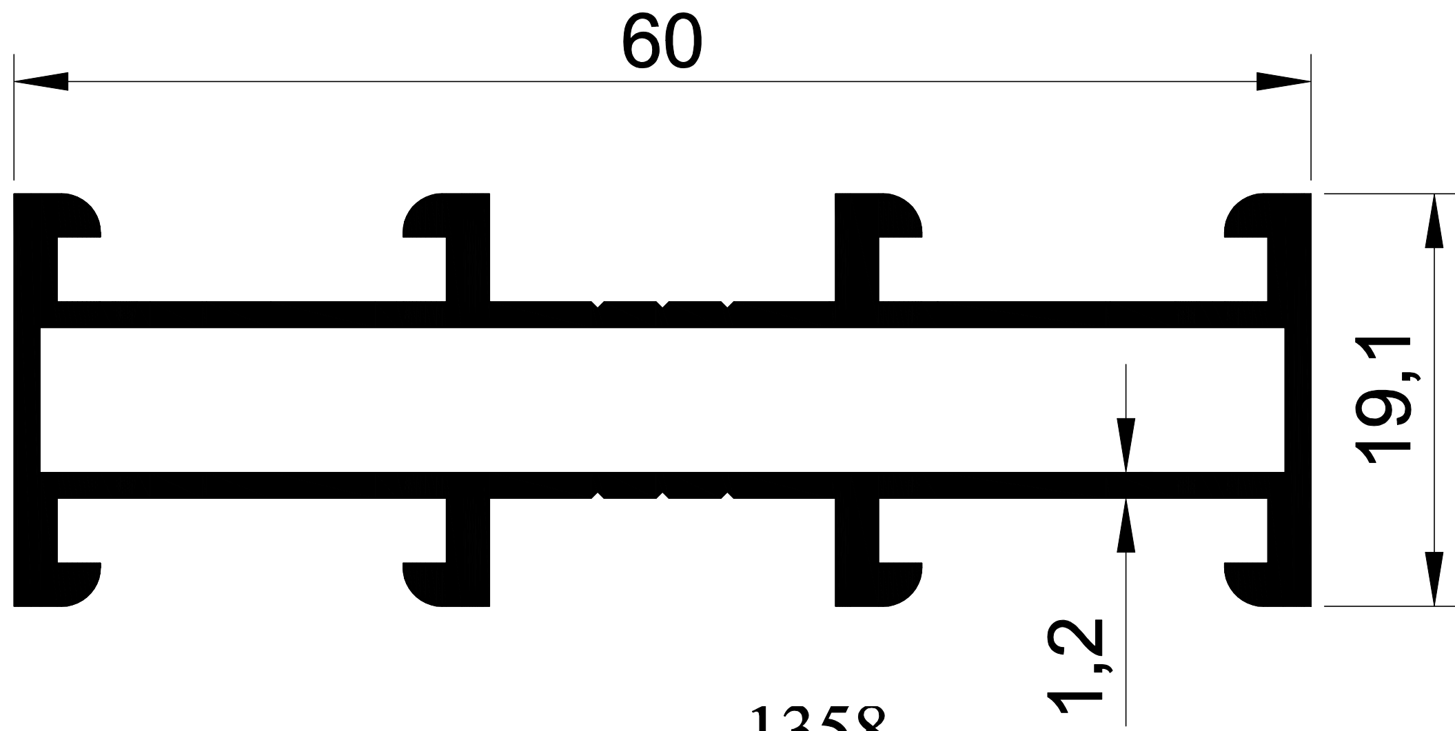
1358 0,721 Kg/m. C-60 DAR KASA
