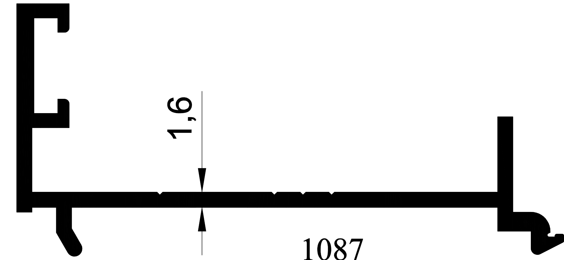
1087 0,462 Kg/m. C-60 ADAPTÖR
