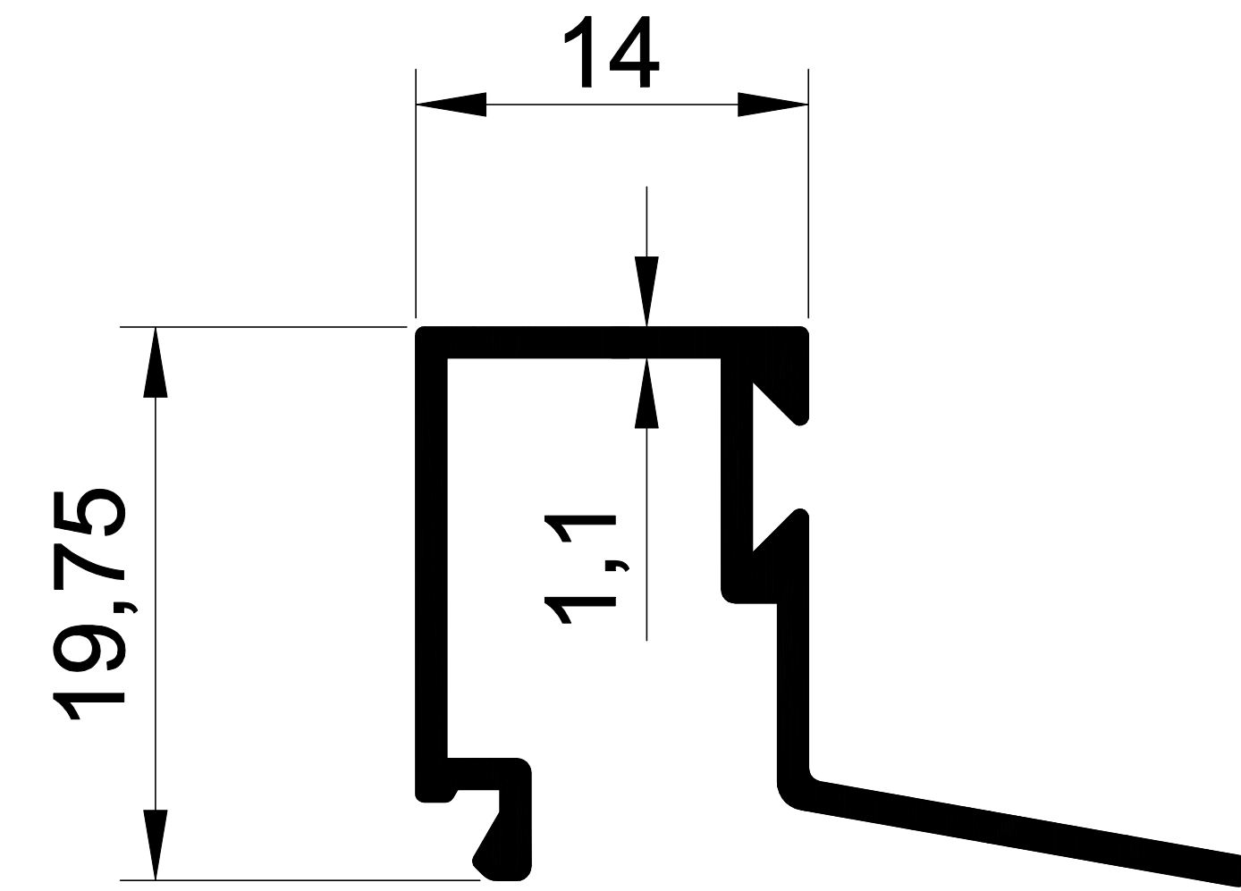
1091 0,232 Kg/m. ALDOKS ISI CAM ÇİTASI
