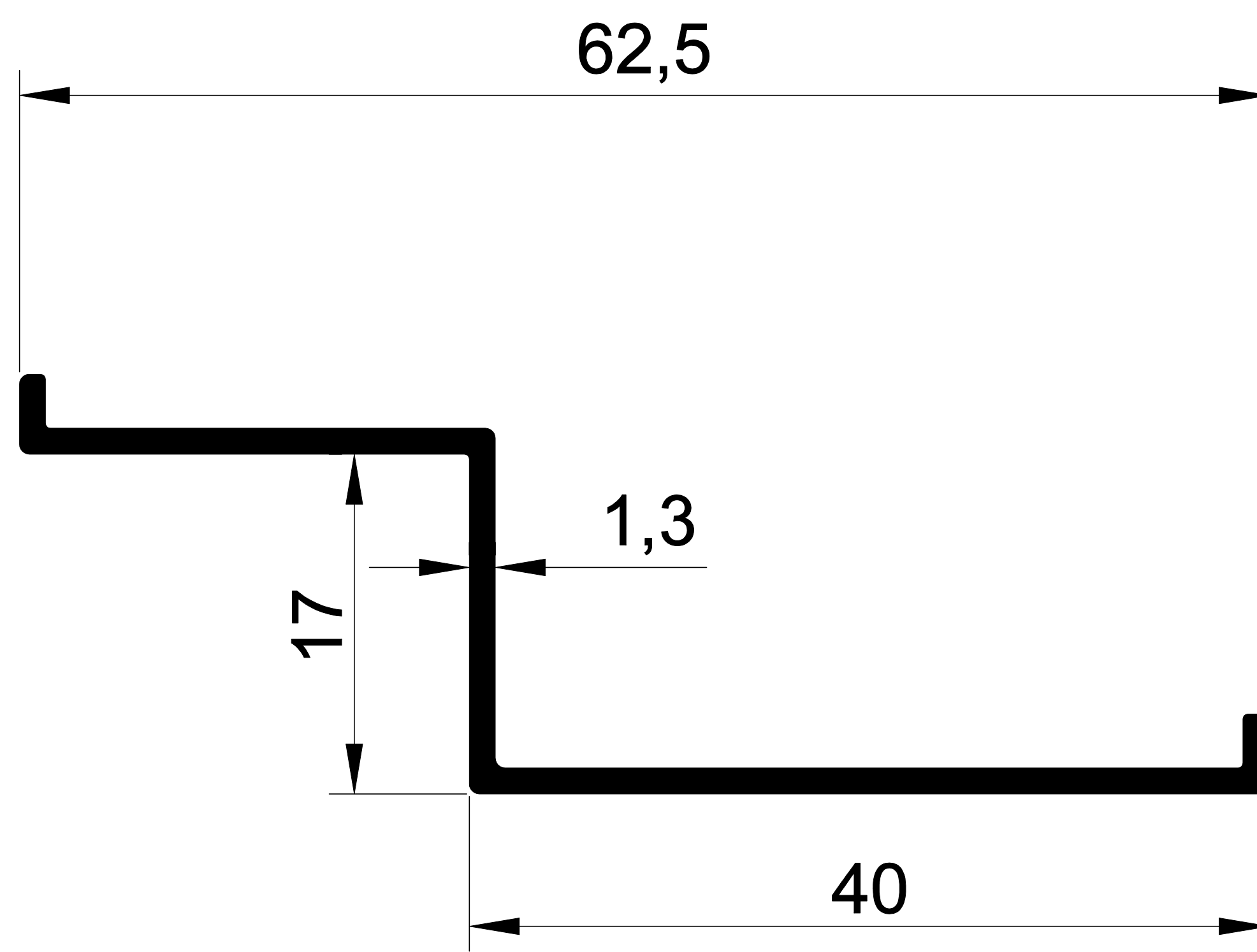
1427 0,298 Kg/m. MS-AHŞAP GİZLİ KAPI KANAT ÇERÇEVESİ
