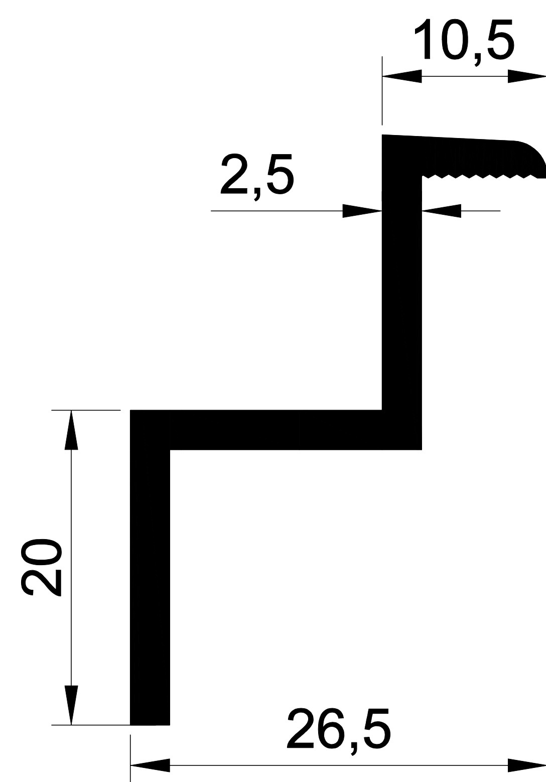
1431 0,410 Kg/m GES PANEL TUTUCU APARATI KÖŞE
