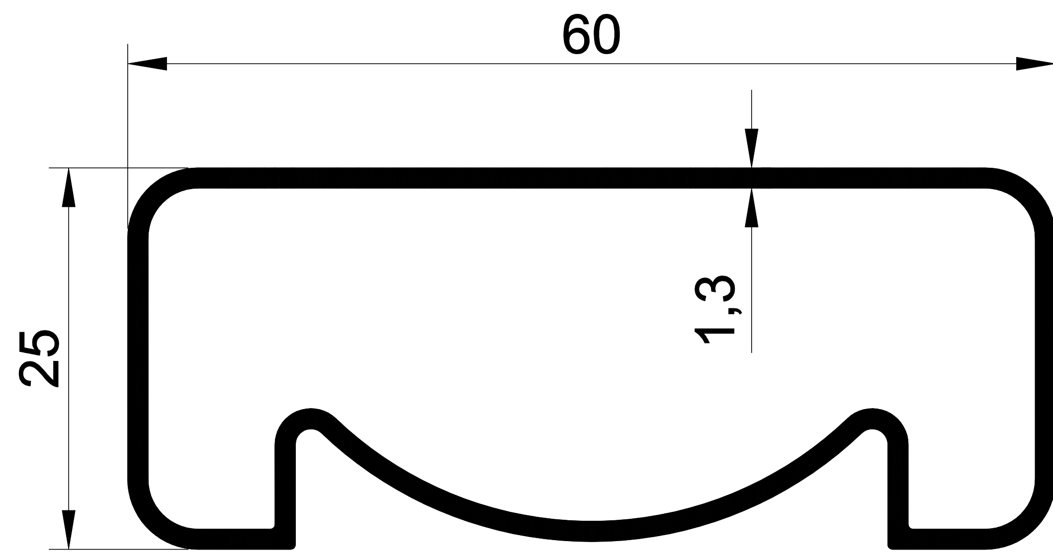
1335 0,613 Kg/m. 25X60 CAMSIZ
