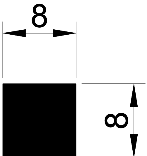
1351 0,173 Kg/m.
