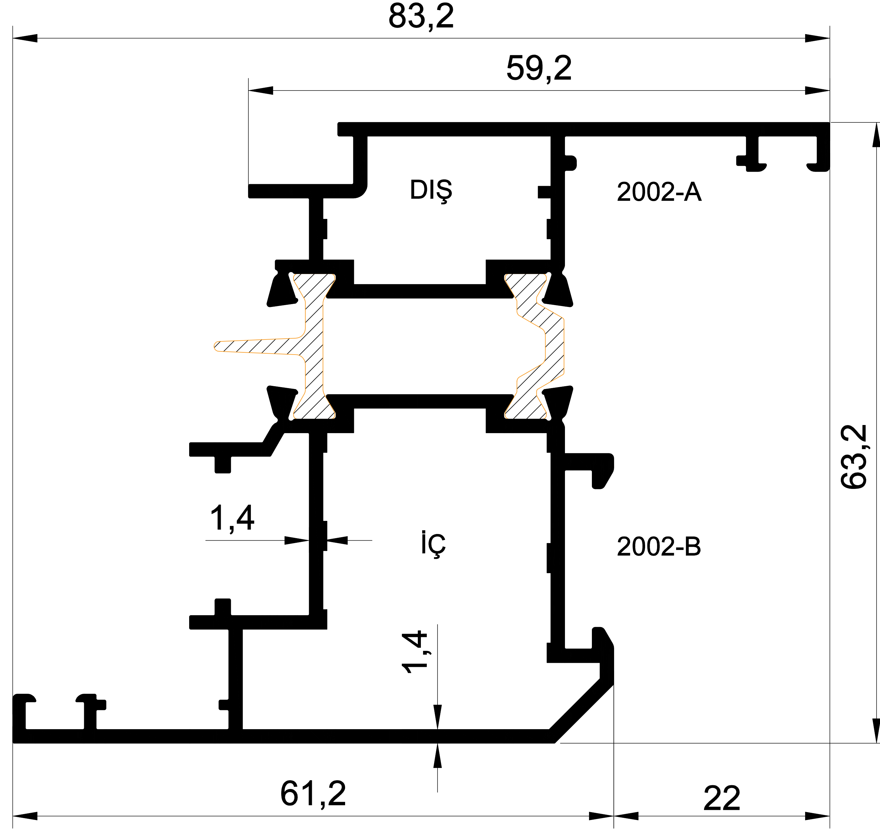
-55- 2002 1,386 gr/m SİSTEM 55 ISI YALITIM KANAT
