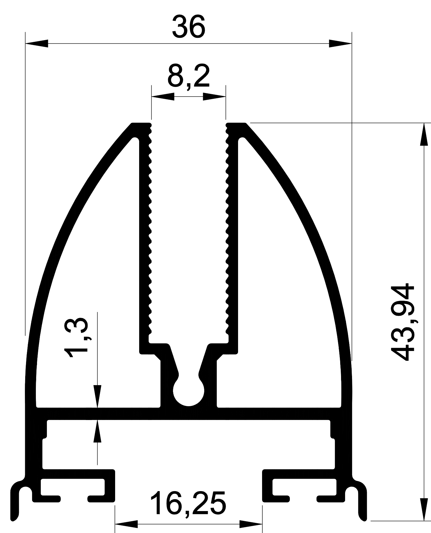
1186 0,756 Kg/m. BKS KANAT
