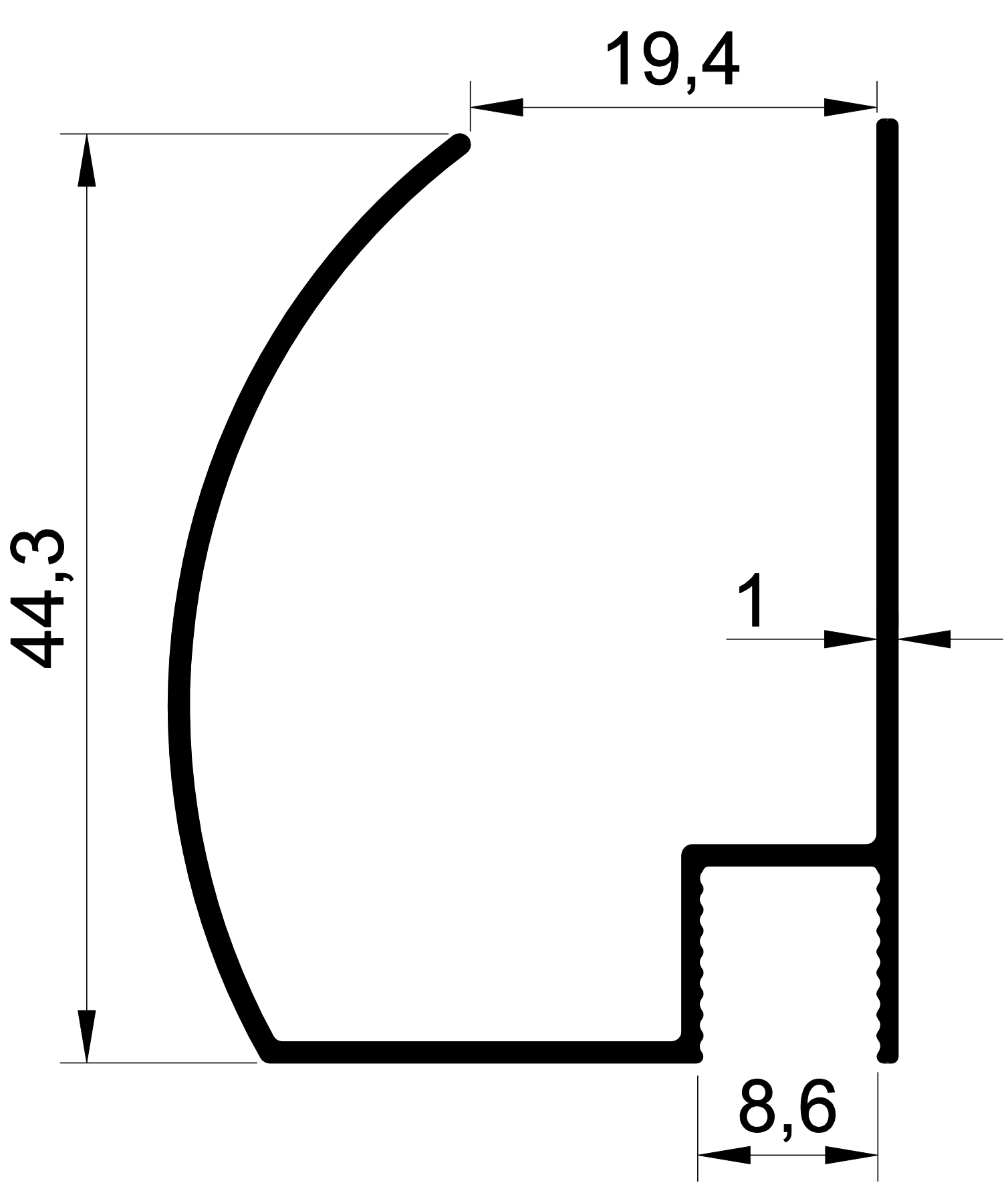
1454 0.353 Kg/m. KENAR PROFİLİ
