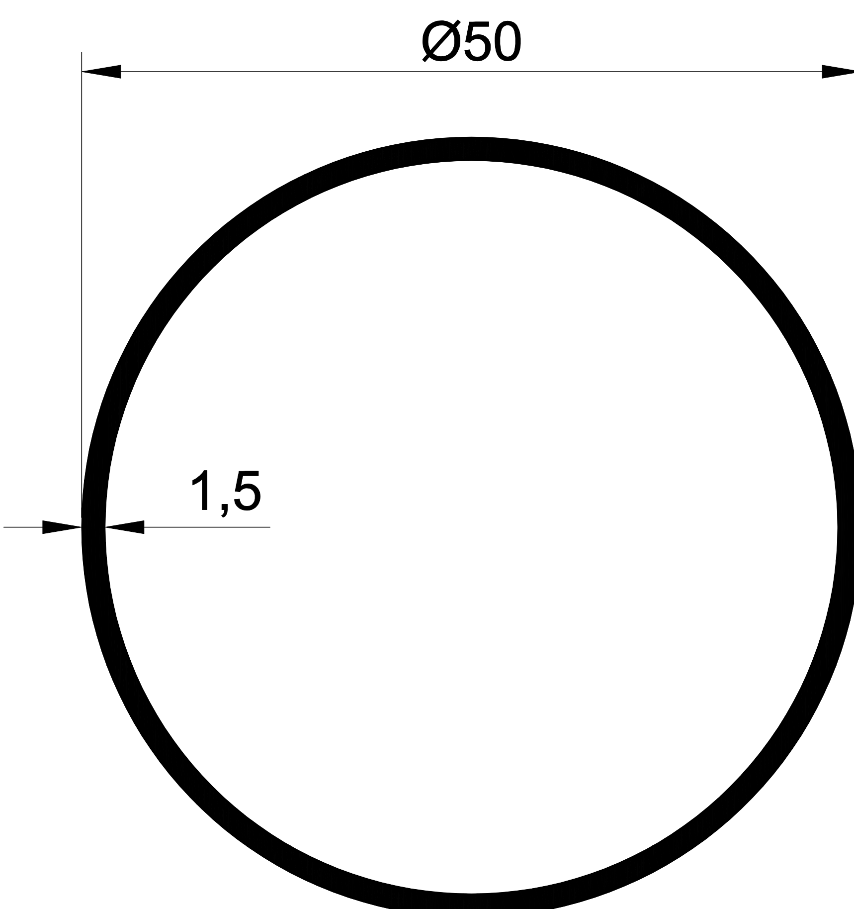
1065 0,620 Kg/m.
