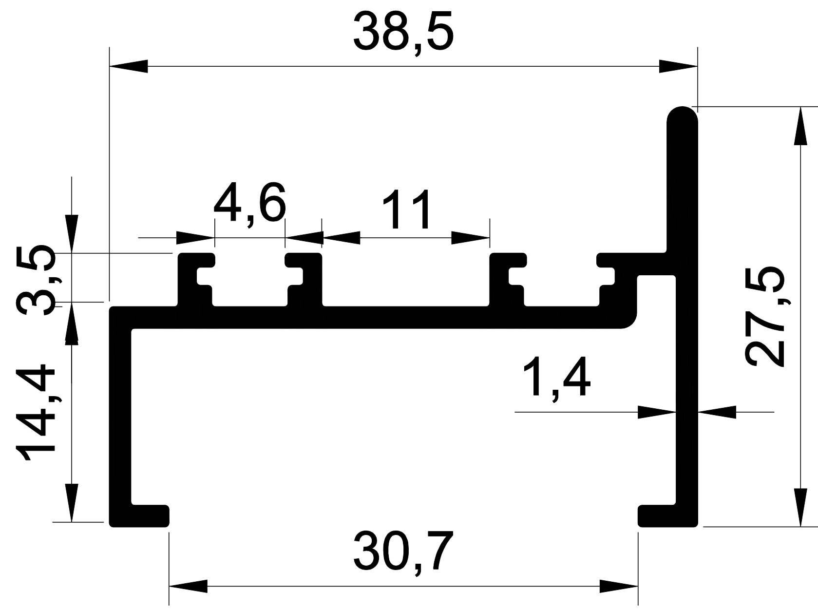
1361 0,402 Kg/m. ISI YALITIM KANAT
