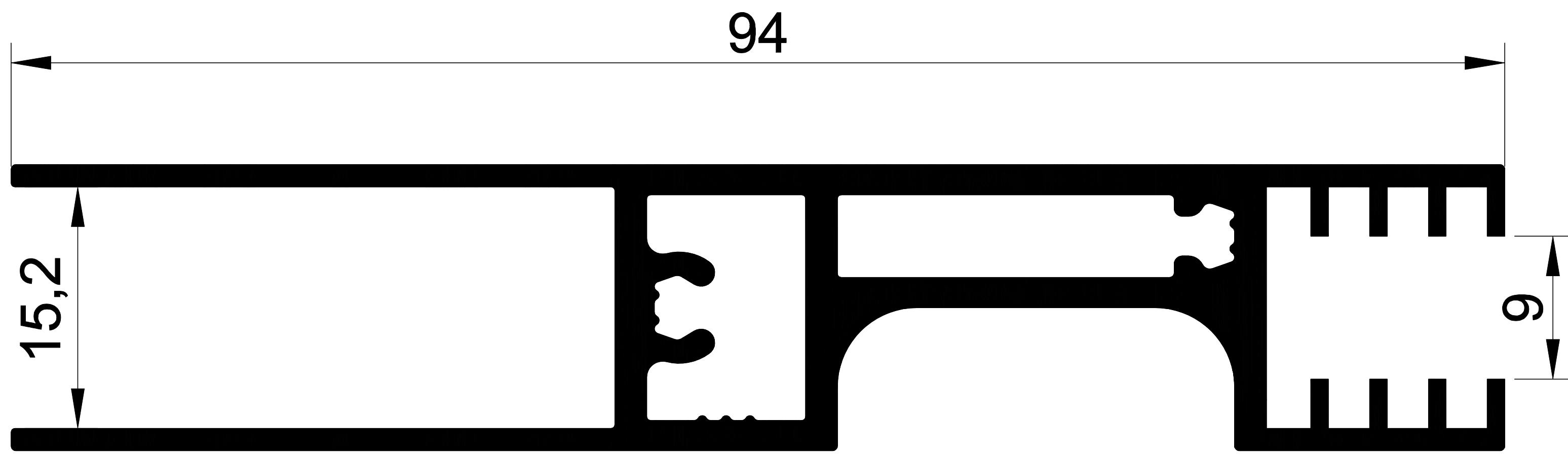
1167 1,225 Kg/m. SÜRME ALT KANAT
