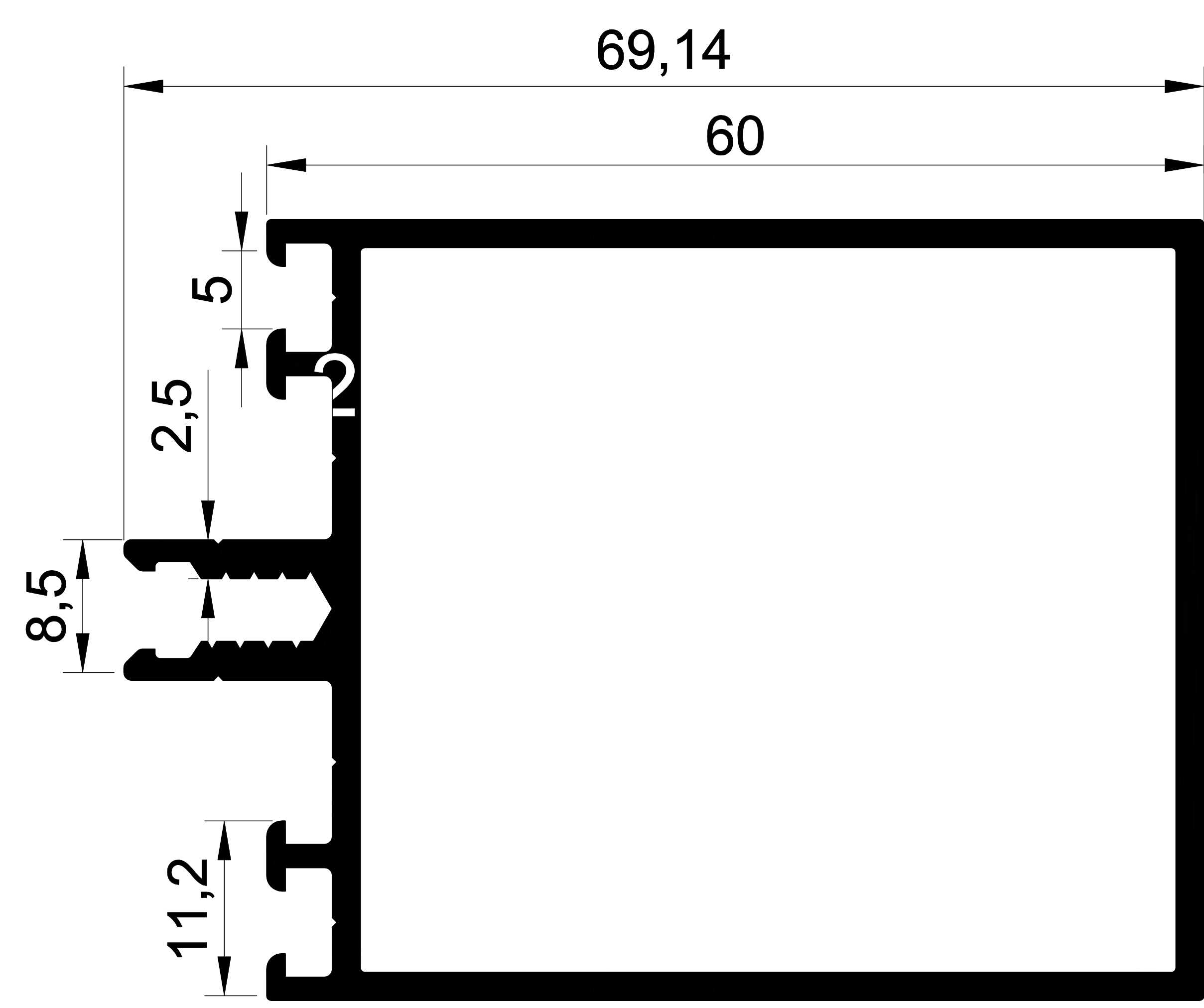
1442 1,251 Kg/m. 60'LIK CEPHE PROFİLİ
