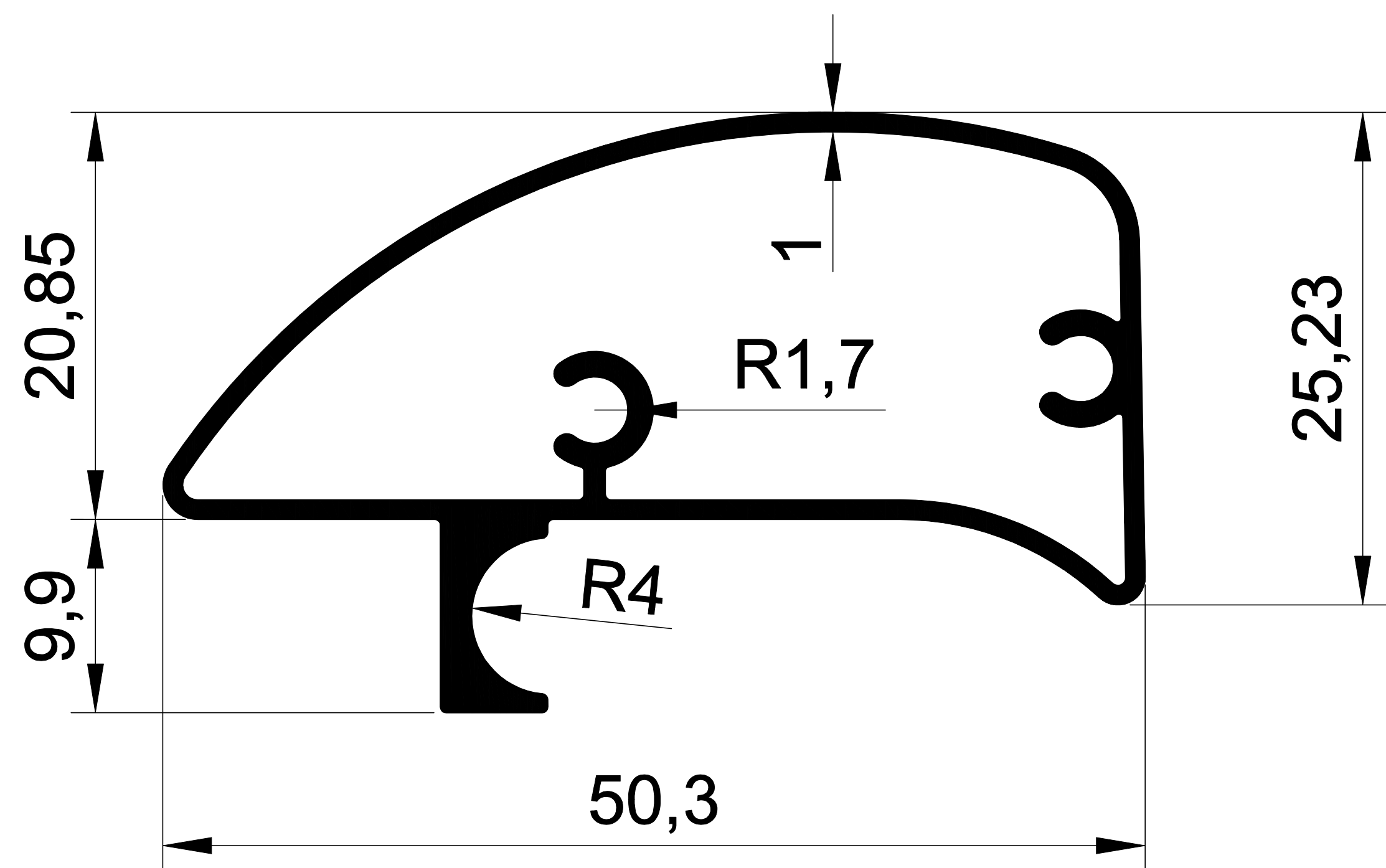
1451 0.505 Kg/m. RAY PROFİLİ
