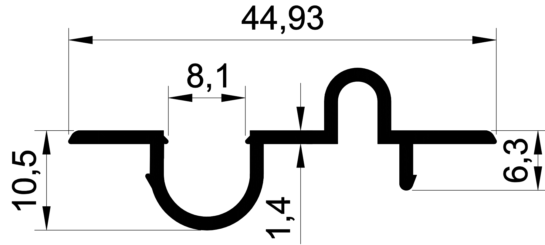
1377 0,283 Kg/m. 100'LÜK TUBA S
