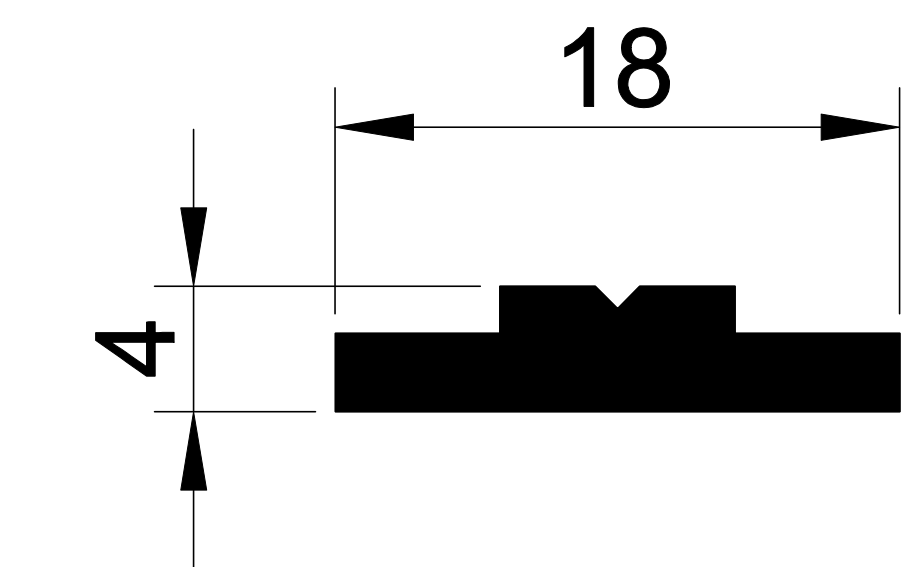
1227 0,152 Kg/m.
