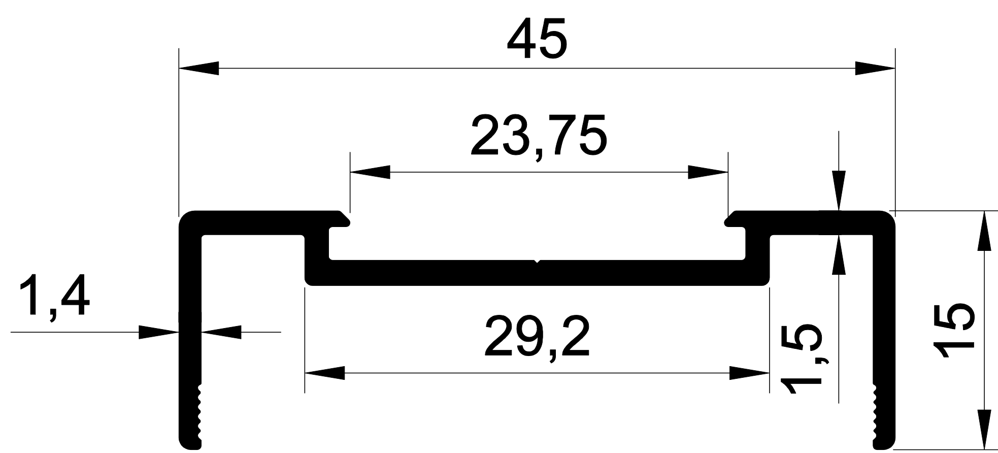
1419 0,320 Kg/m. MS-AHŞAP KANAT ÇERÇEVESİ
