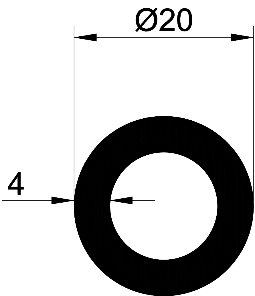
1139 0,545 Kg/m.
