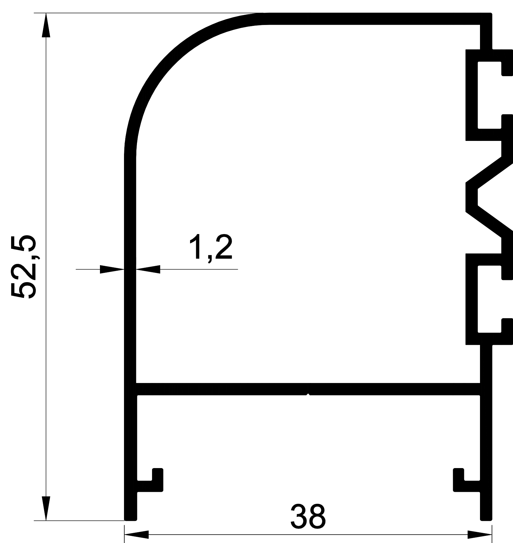
- 2305 0,661 gr/m ISICAMLI CAM BALKON PROFİLLERİ
