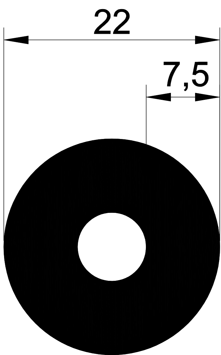
1051 0,927 Kg/m.
