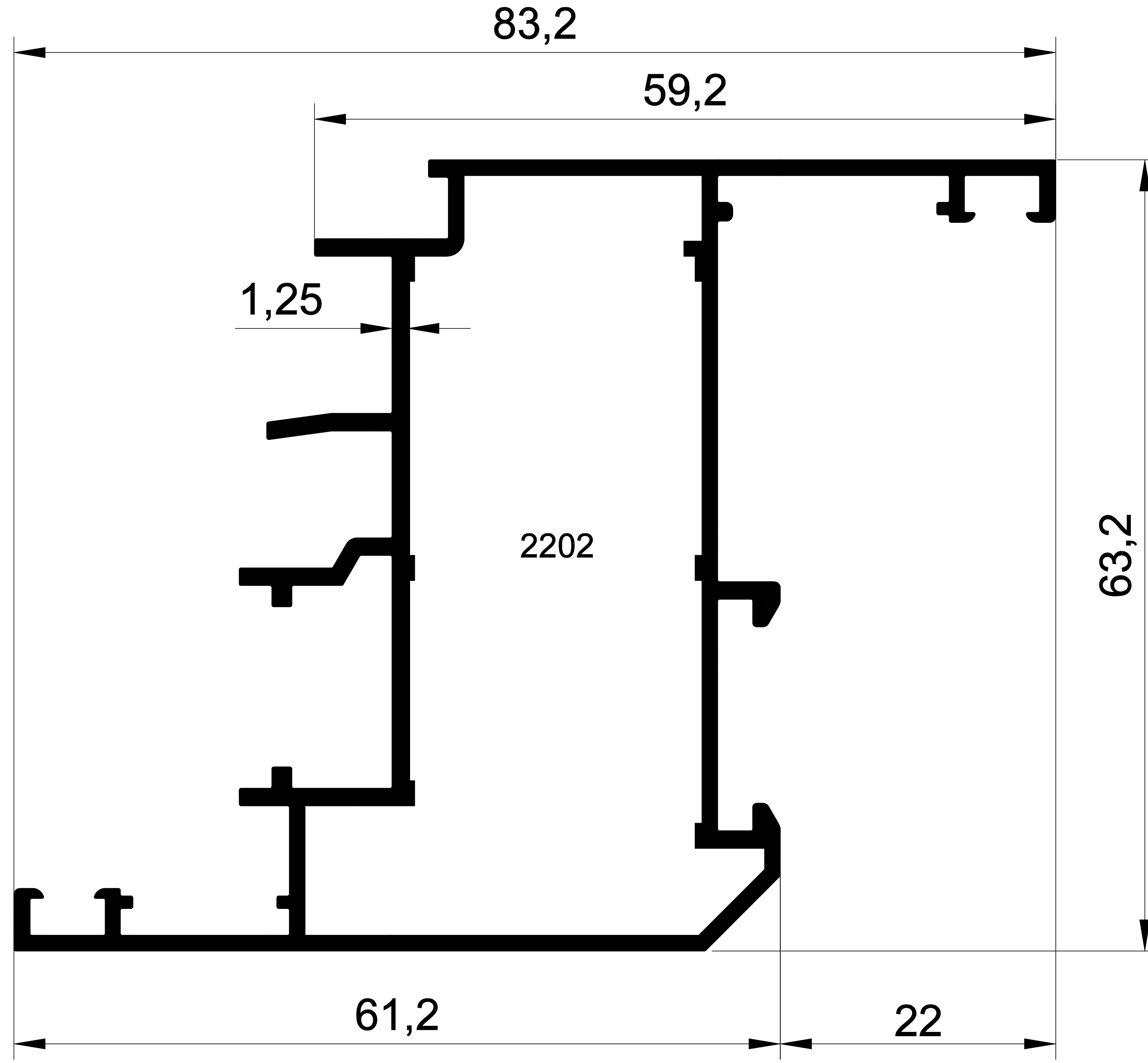
EK-55- 2202 1,135 Kg/m SİSTEM 55 YALITIMSIZ KANAT
