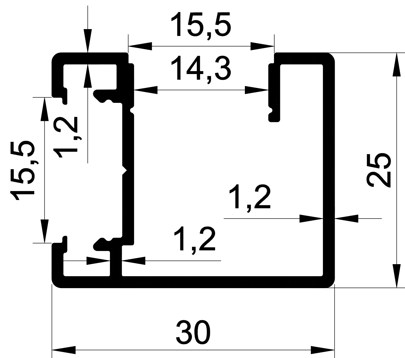
1462 0,357 Kg/m 30*25 GEMİCİ
