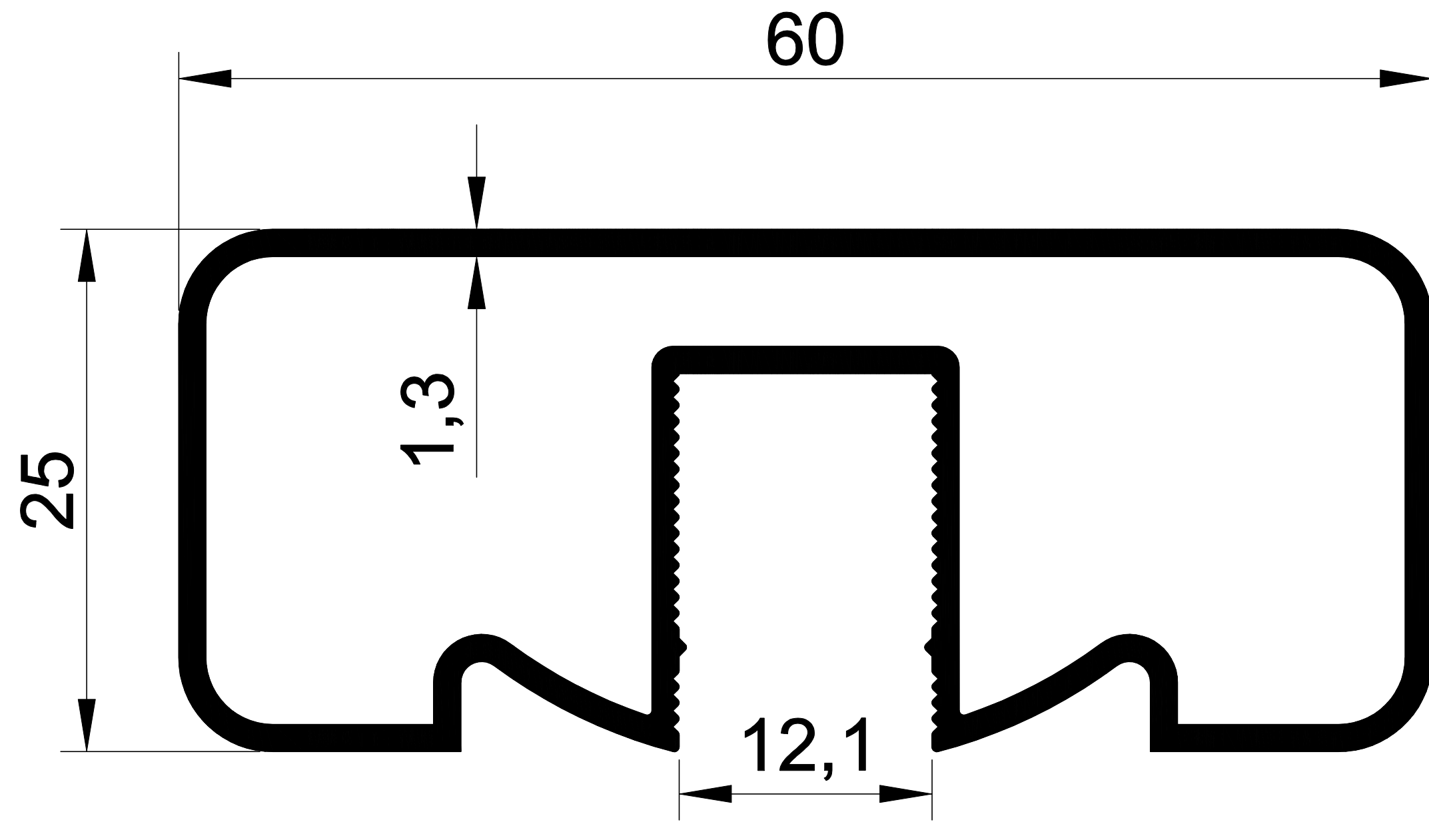
1129 0,706 Kg/m. 25X60 ORTADAN CAMLI
