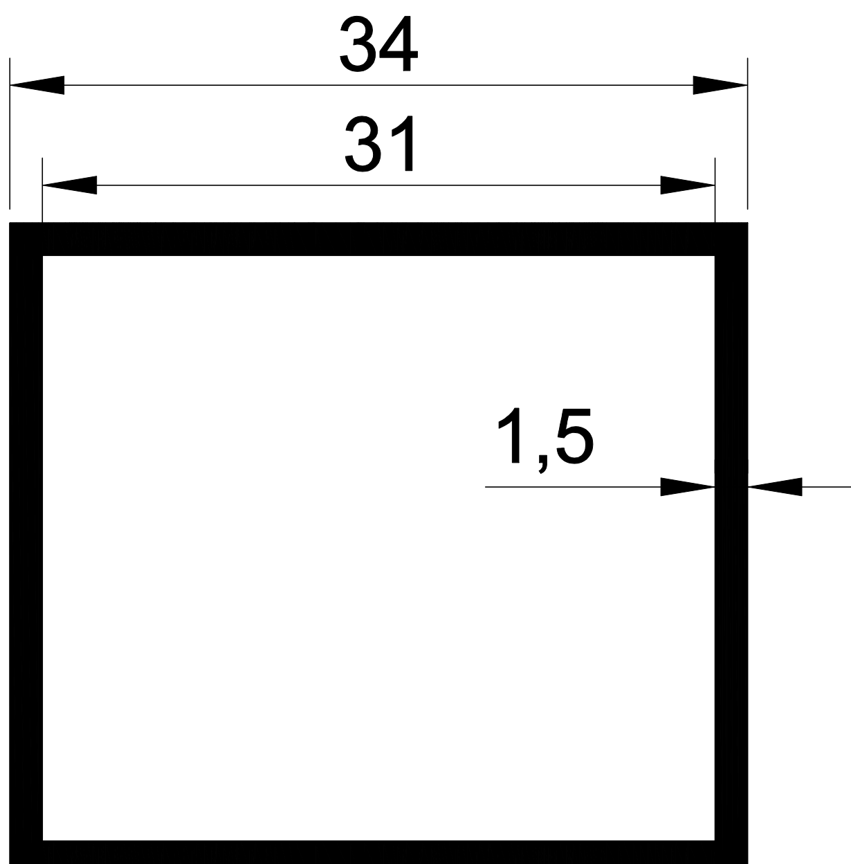
1469 0,496 Kg/M
