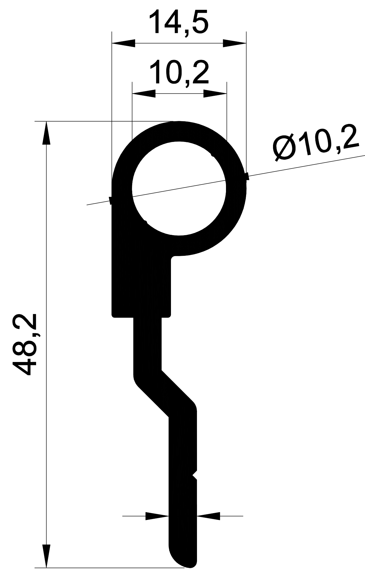
1009 0,599 Kg/m.
