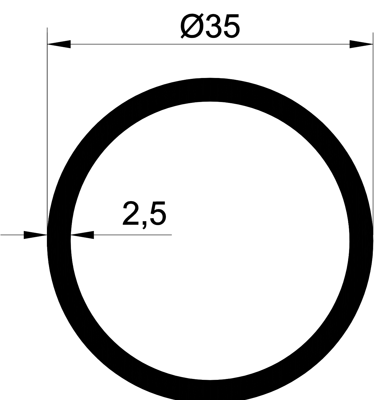
1070 0,692 Kg/m.
