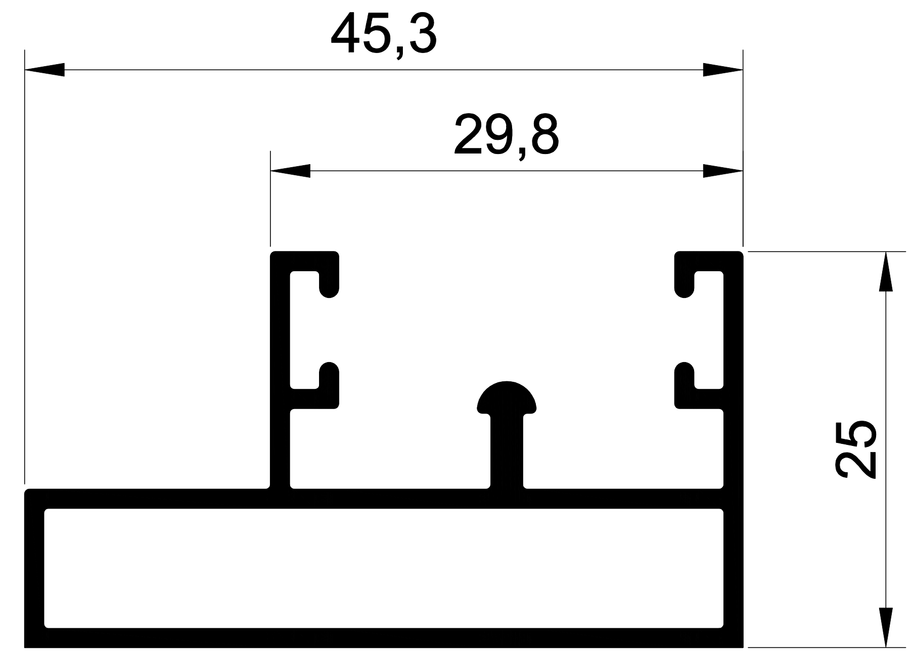
1374 0,545 Kg/m. AYKİM KASA
