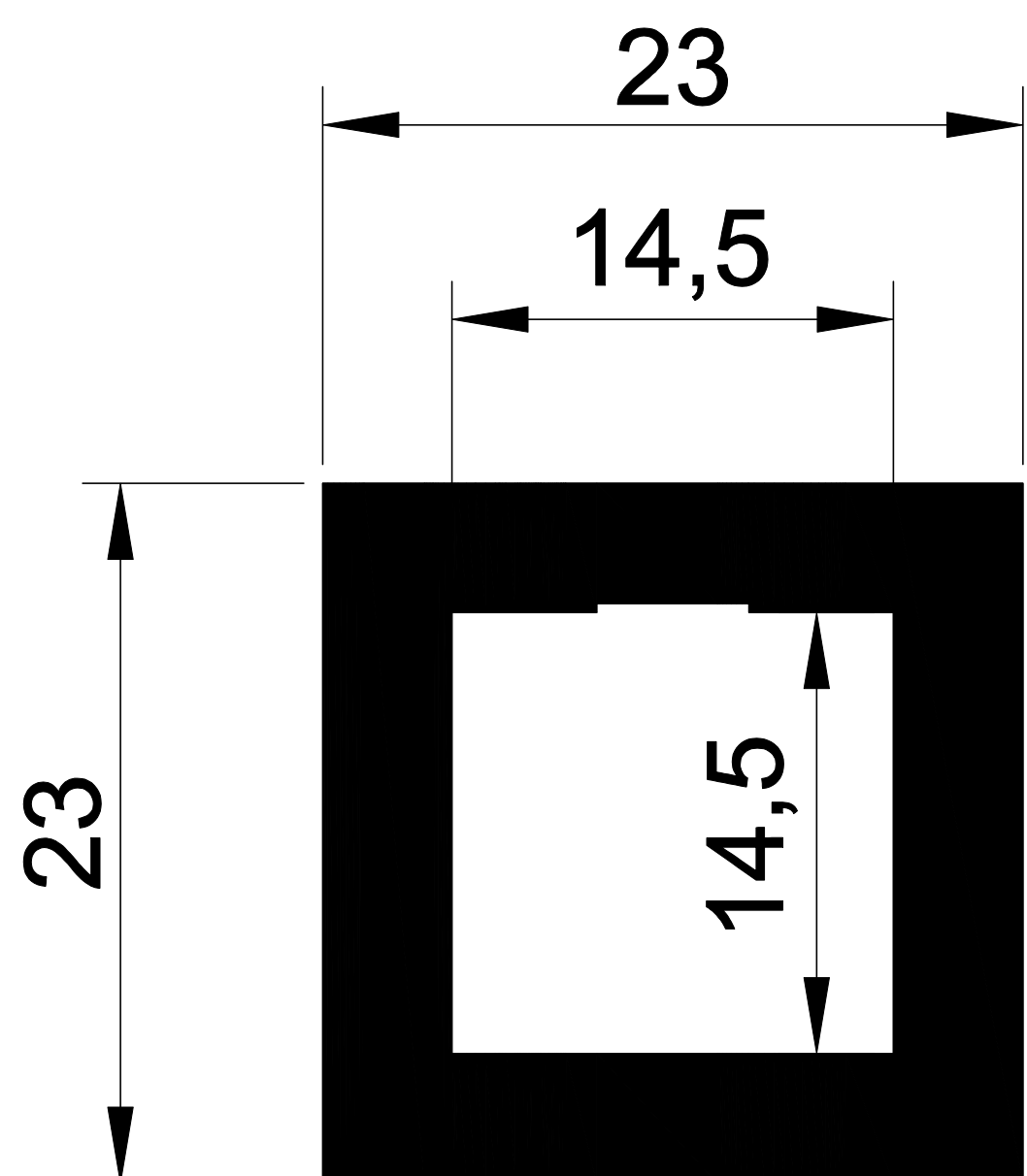
1048 0,859 Kg/m.
