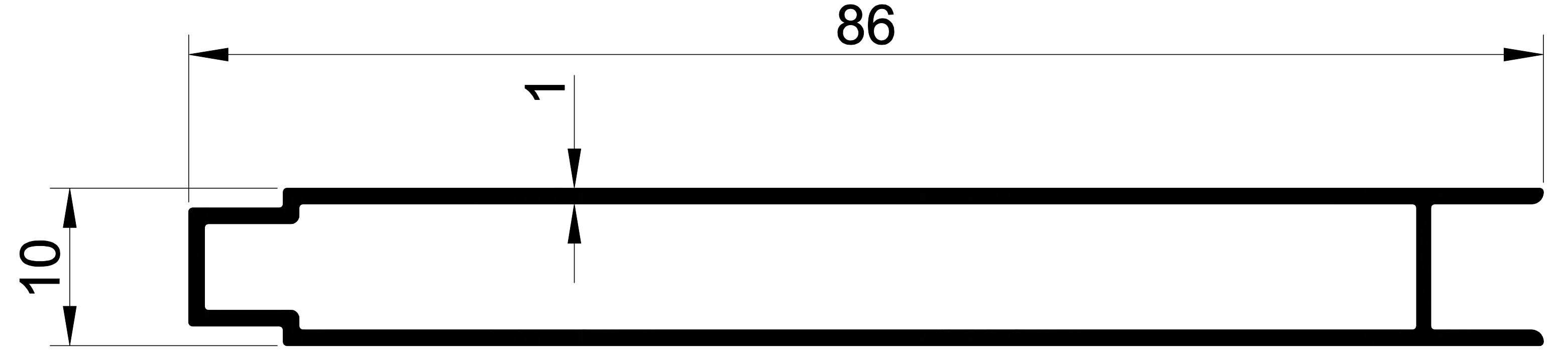
1182 0,507 Kg/m. ALÜMİNYUM TAHTA LAMBİRİ
