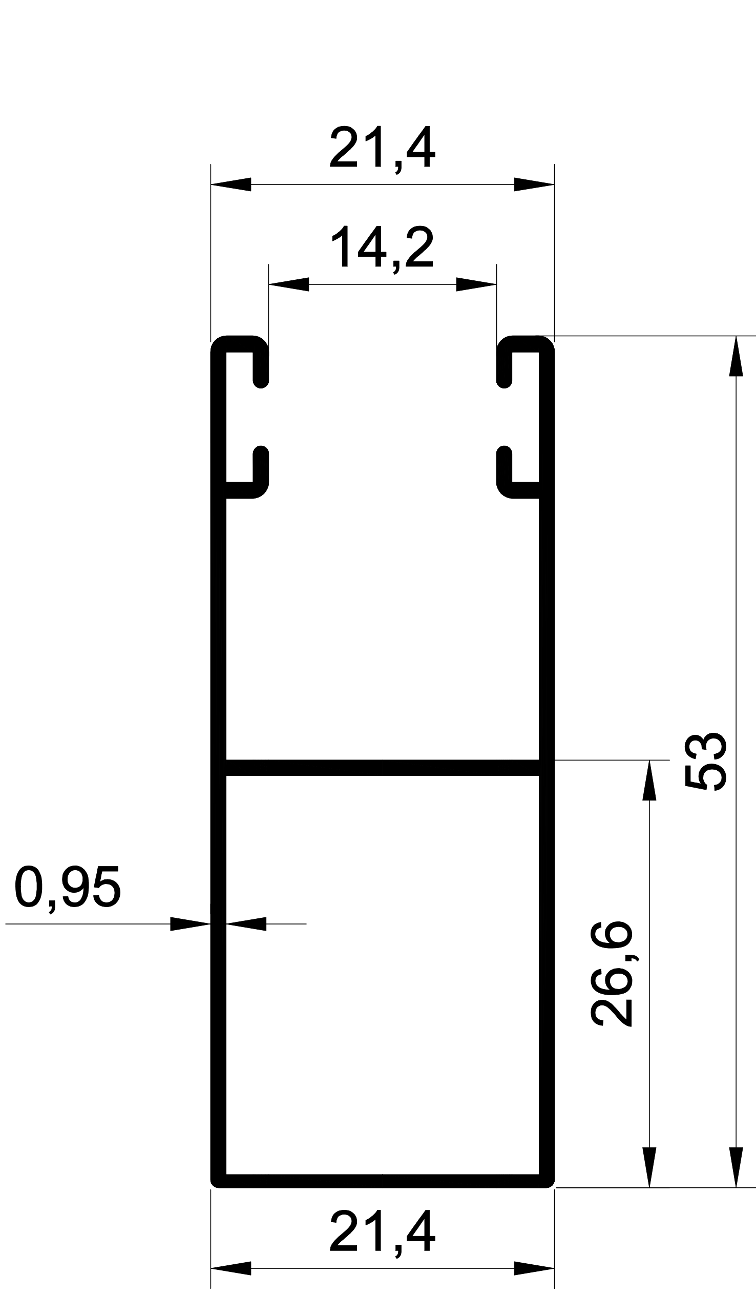
1307 0,412 Kg/m. 53'LÜK DİKME
