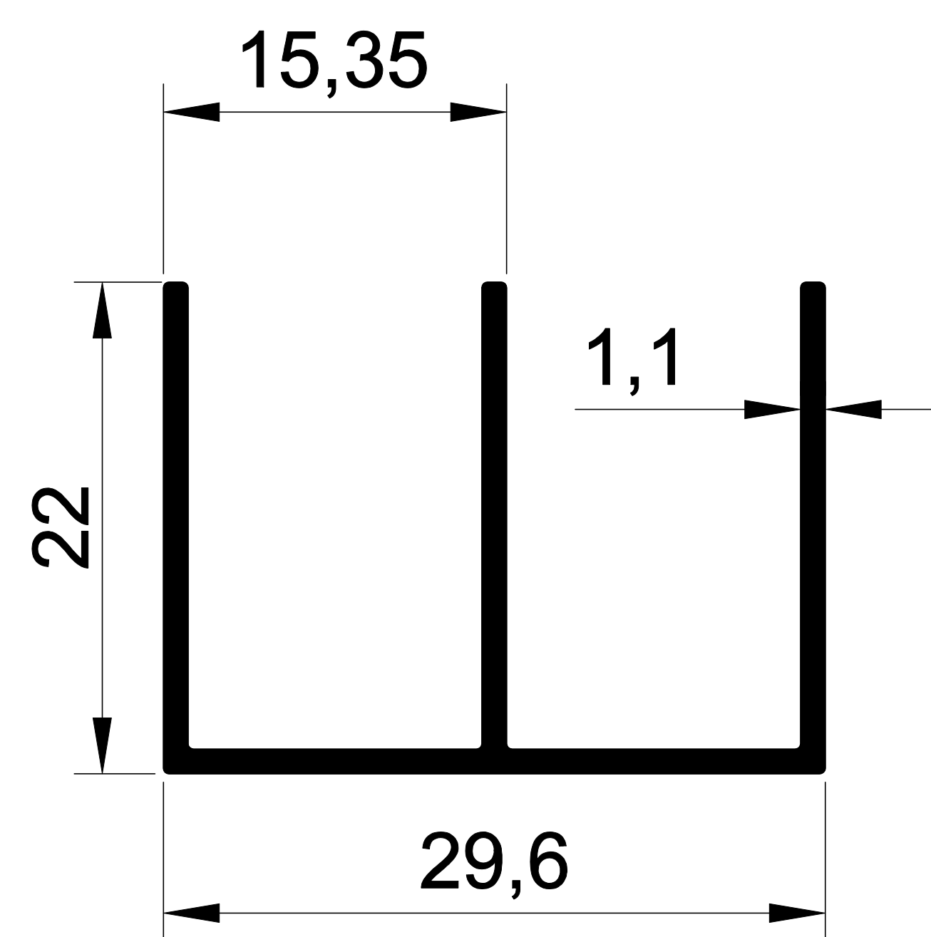
1408 0,275 Kg/m. MOBİLYA E PROFİLİ
