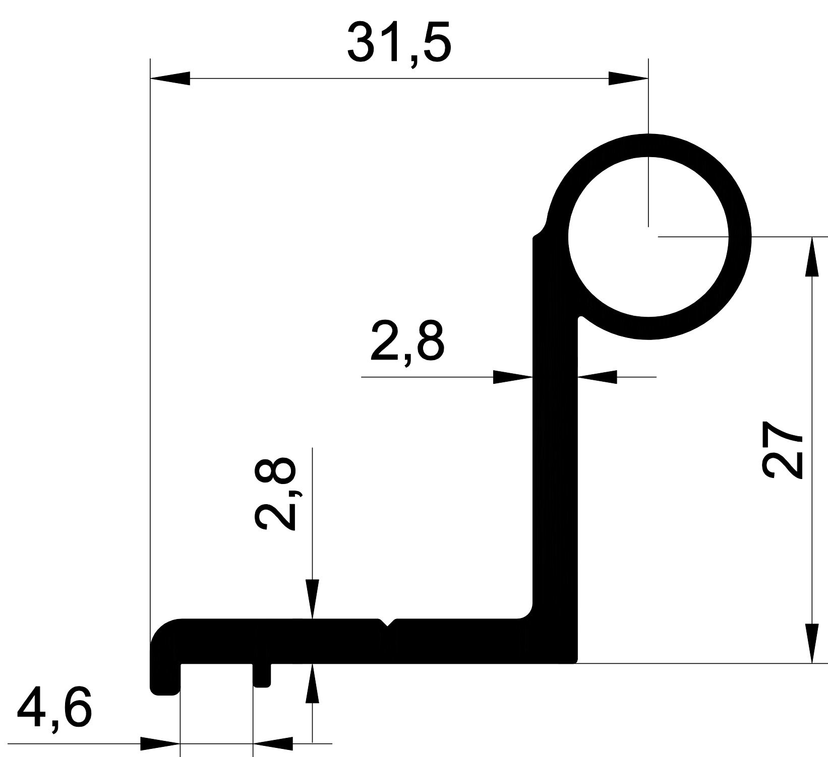
0,522 Kg/m. 1230-B
