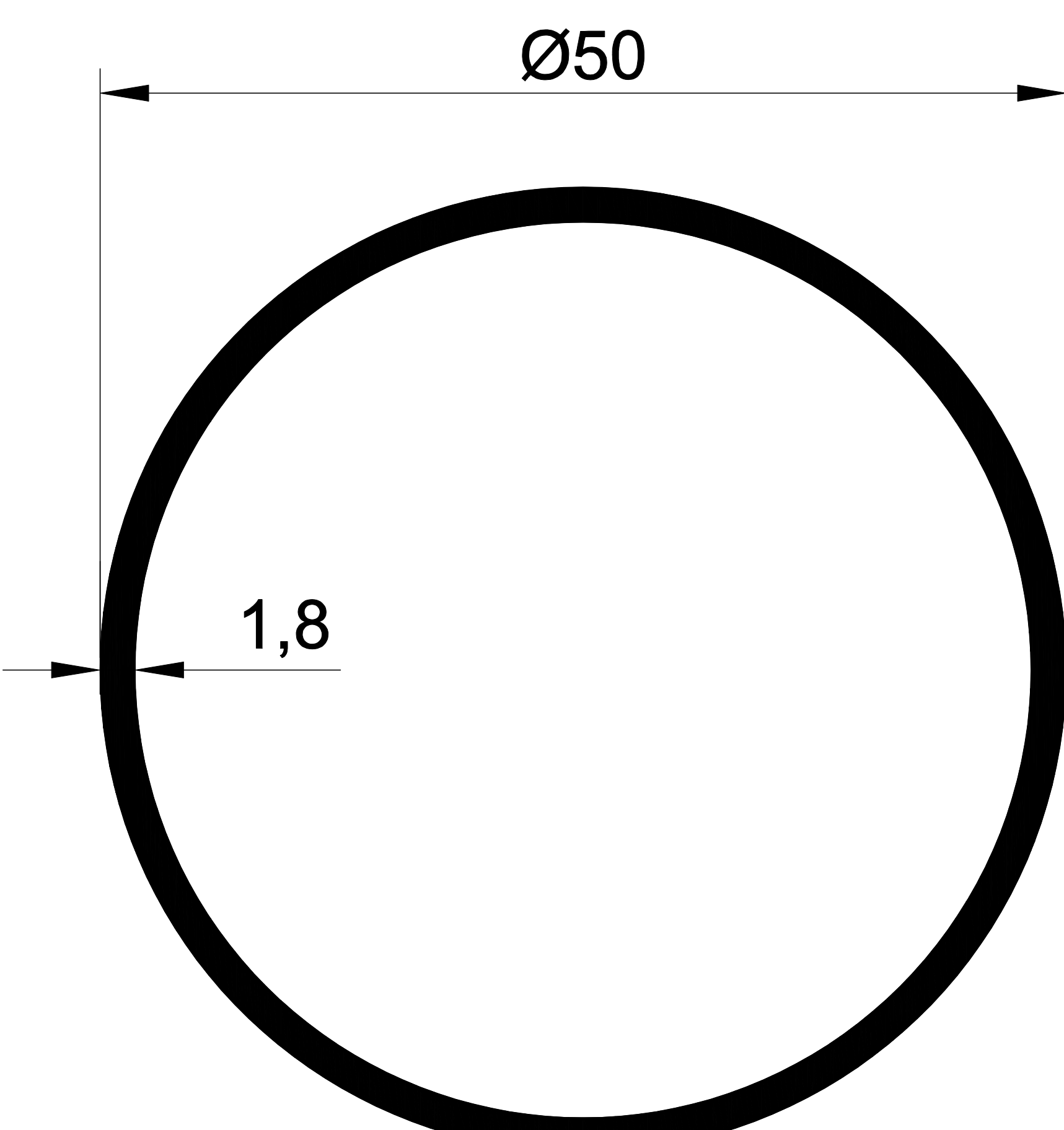
. 1067 0,734 Kg/m.
