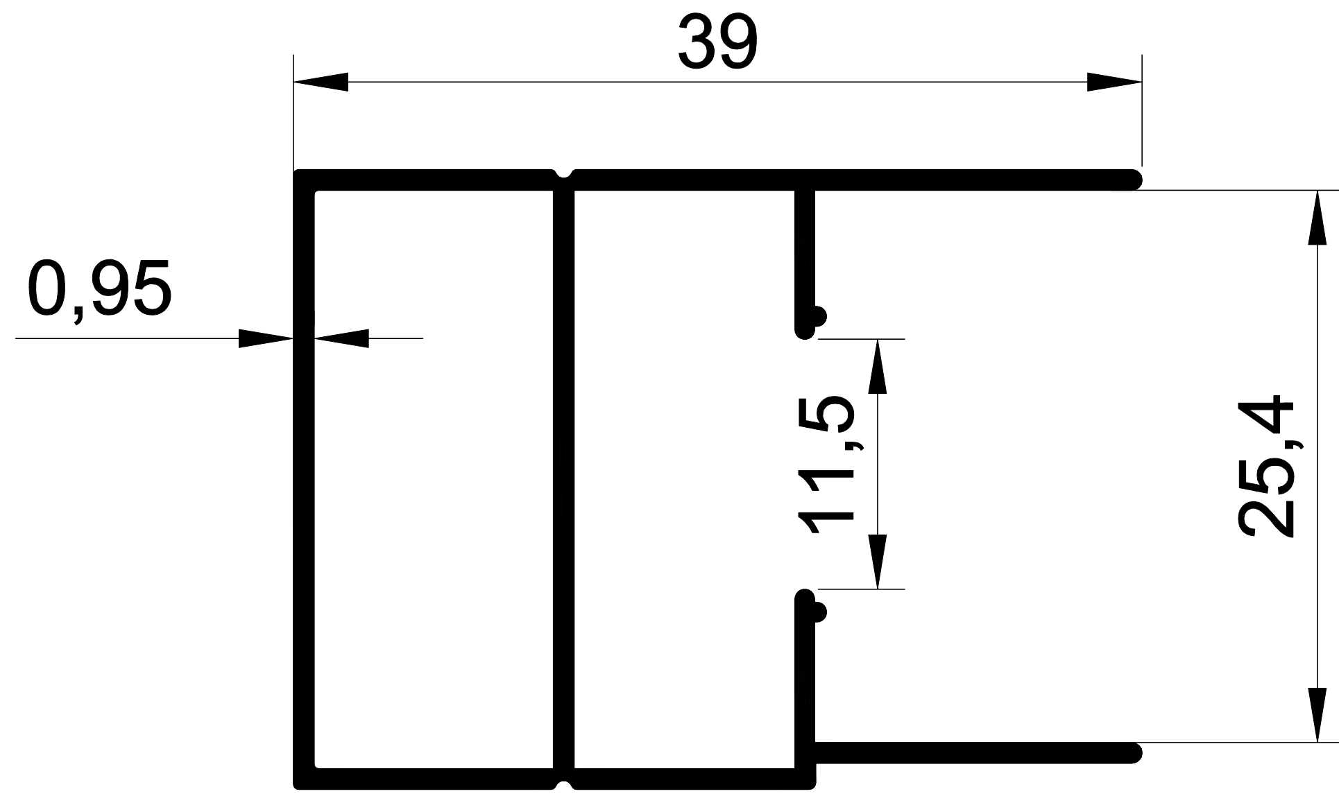
1142 0,374 Kg/m. PİLELİ SİNEKLİK KASA
