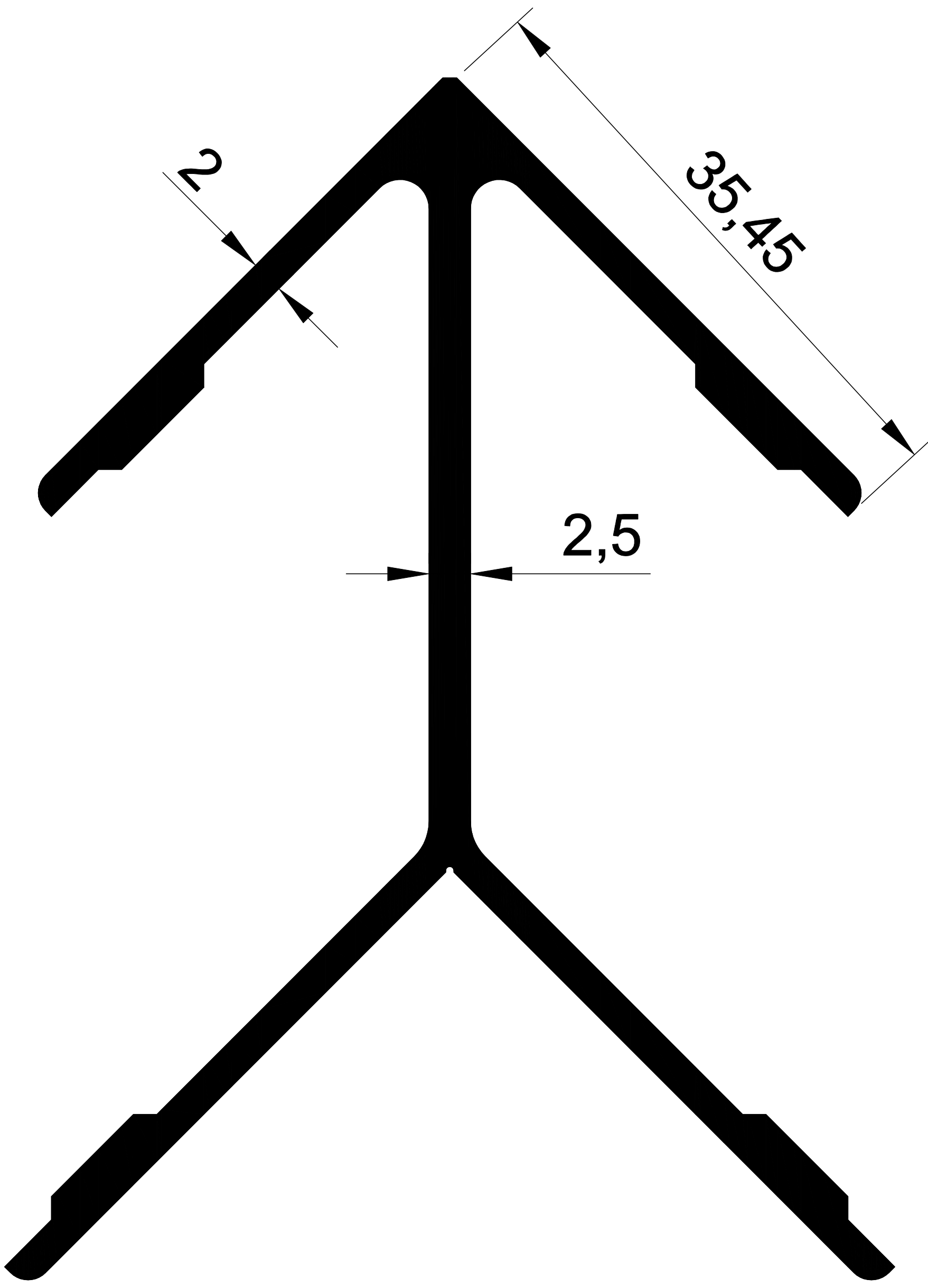
1094 1,170 Kg/m. GENİŞ ÇAVUŞ (KÖŞE BAĞLANTI)
