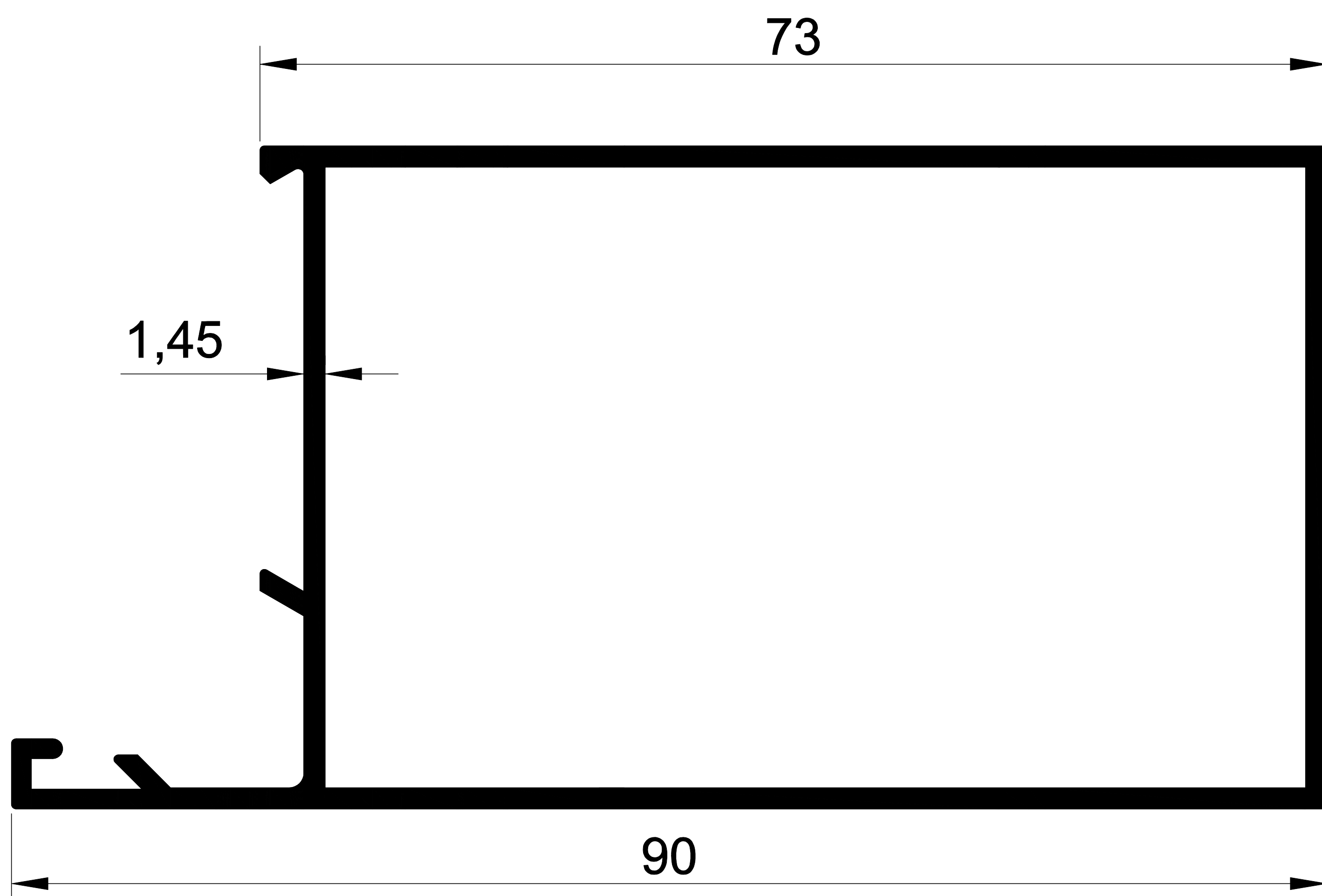
1108 1,022 Kg/m. ALDOKS BAZA KASA
