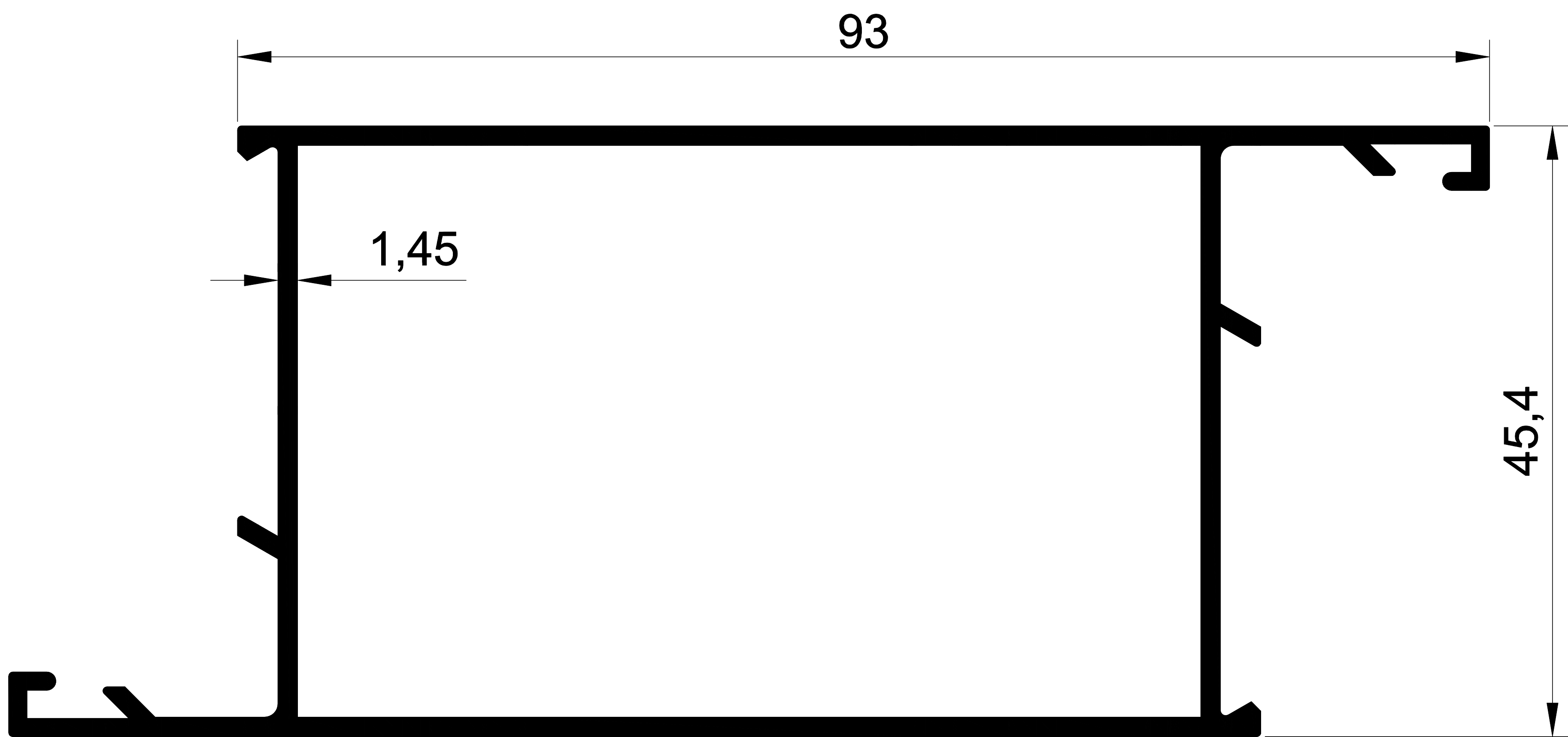
1109 1,162 Kg/m. ALDOKS BAZA KAPI
