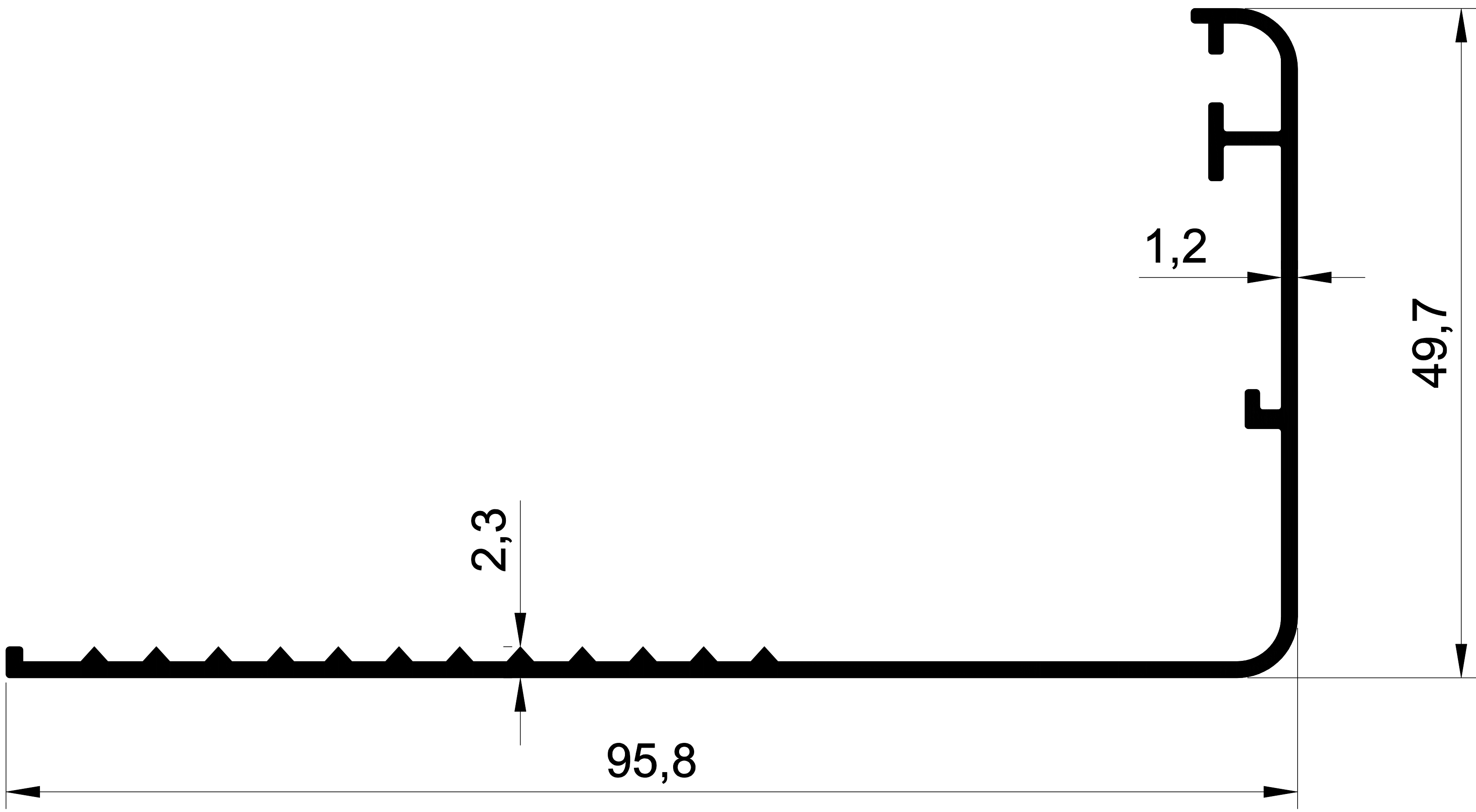
1267 0,566 Kg/m. ALÜMİNYUM PERVAZ
