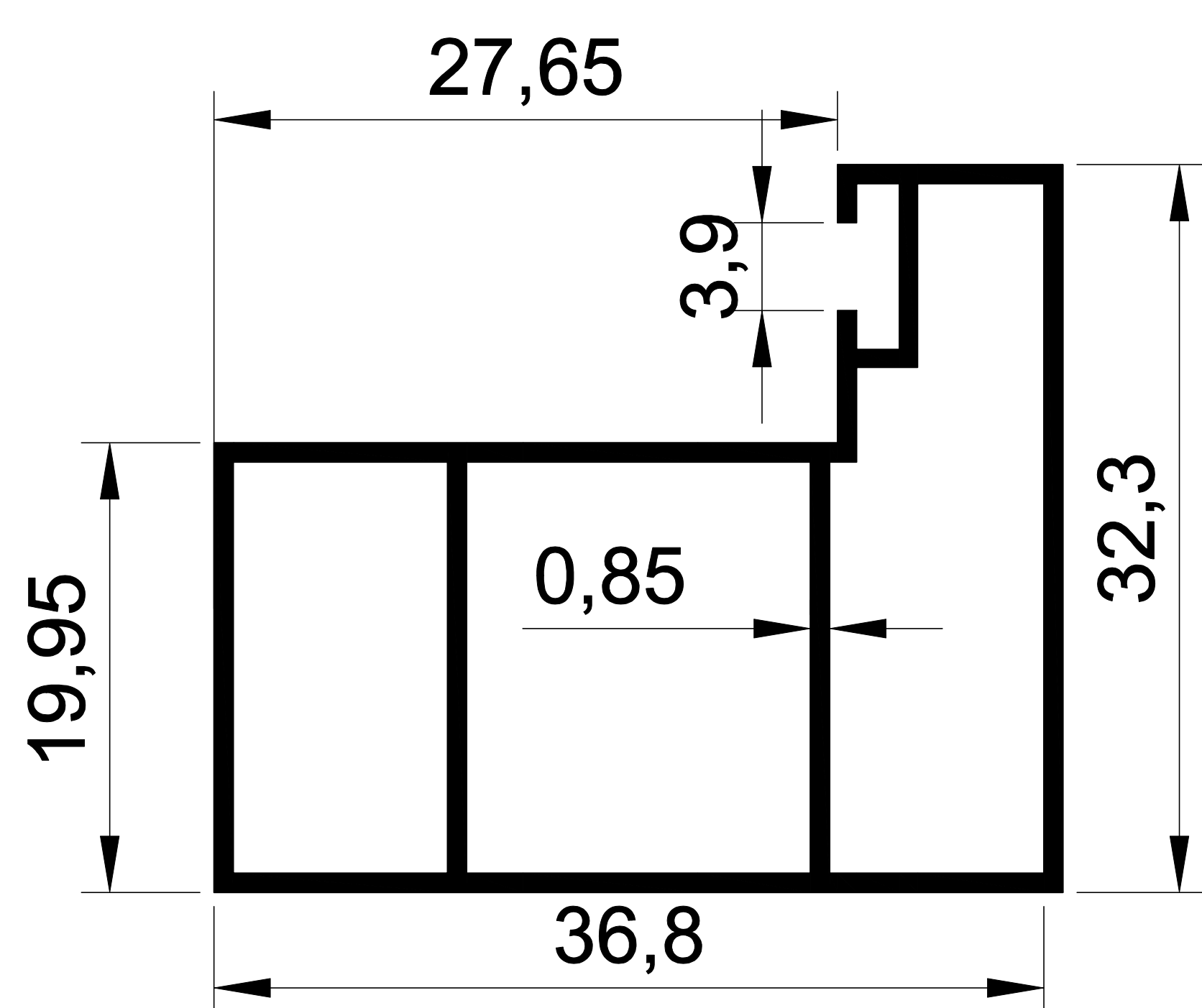
1450 0,411 Kg/m. BKS DİKME
