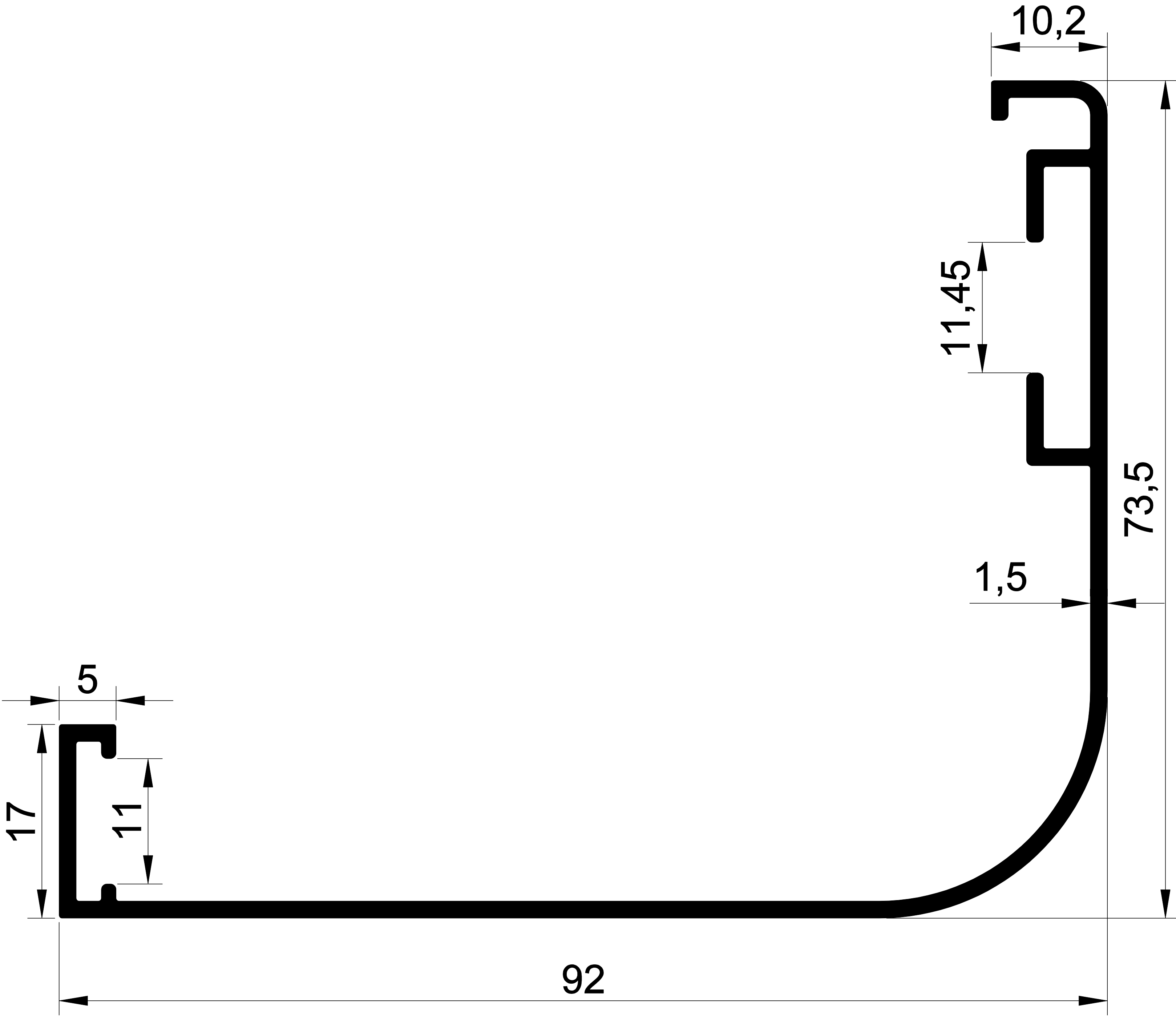
1423 0,859 Kg/m. MS-92'LİK PEERVAZ
