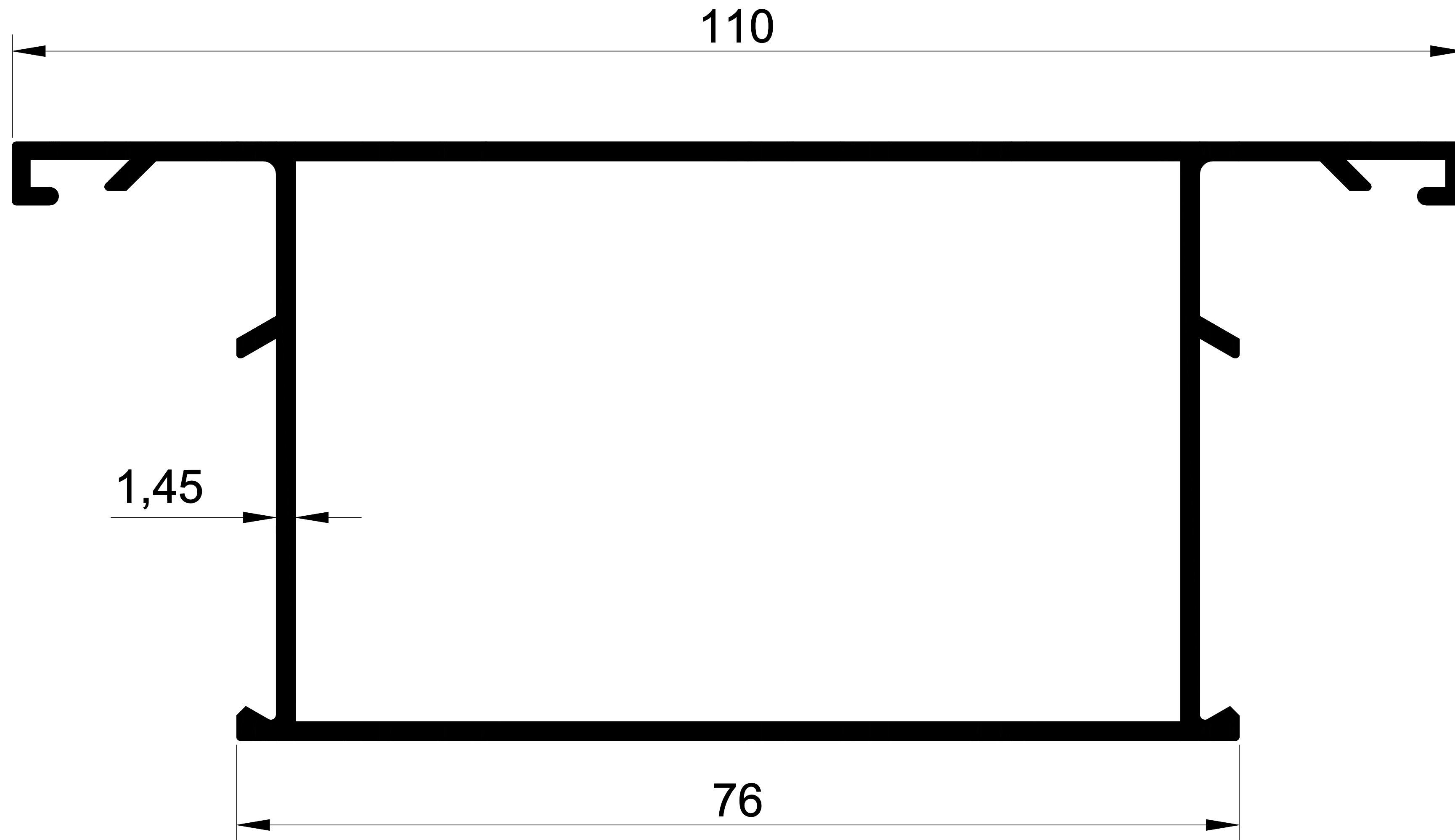
1111 1,162 Kg/m. ALDOKS BAZA ORTA
