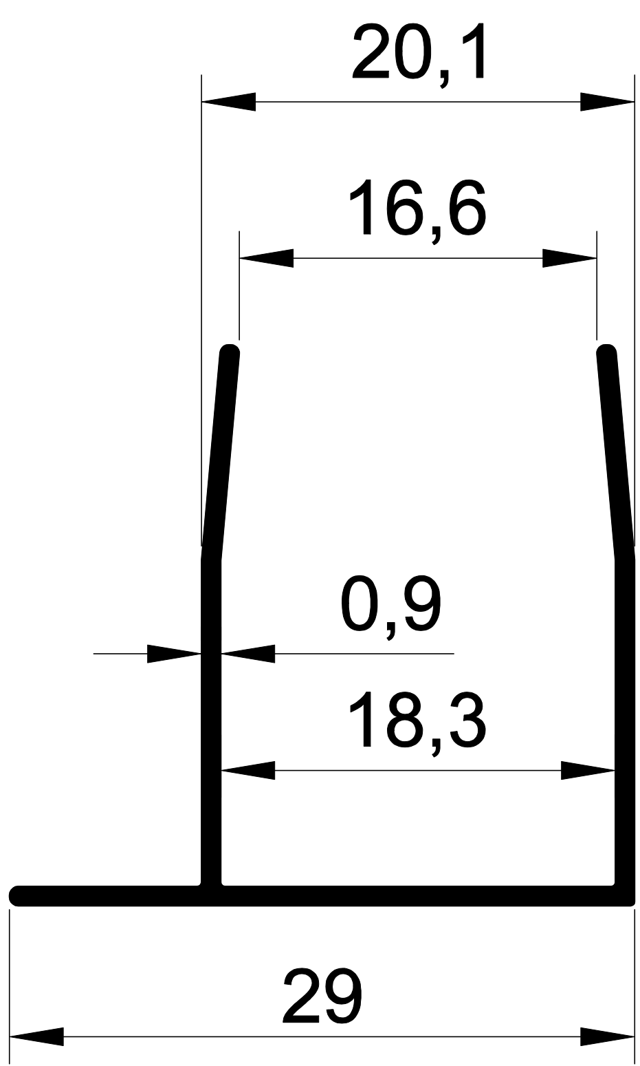
1452 0.193 Kg/m. DUVAR DİKMESİ
