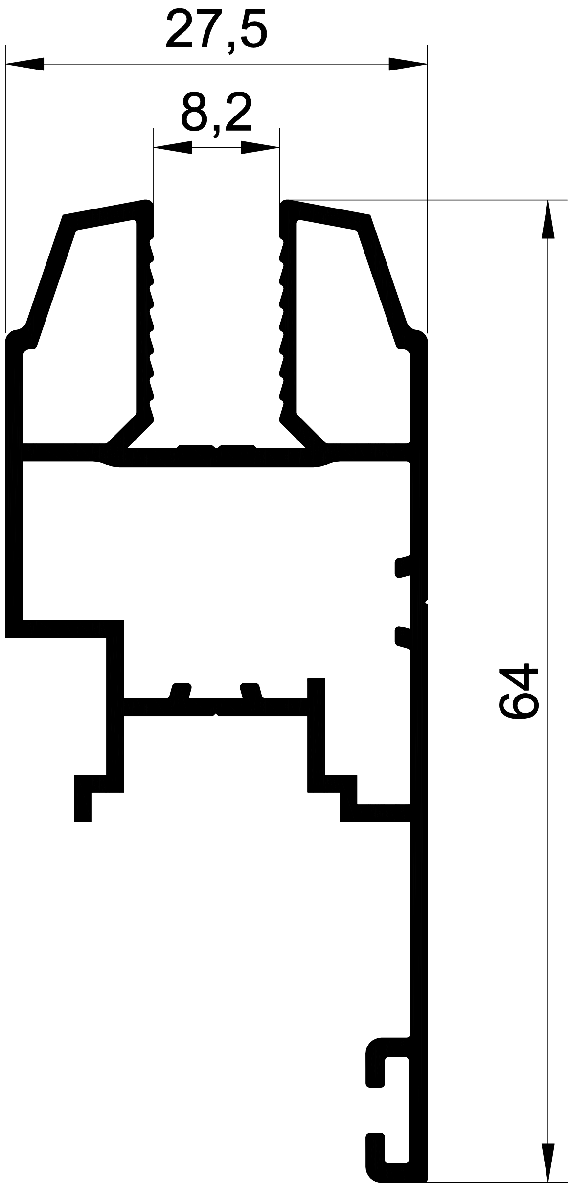
1380 0,663 Kg/m. 64'LÜK CAM BALKON KİLİT
