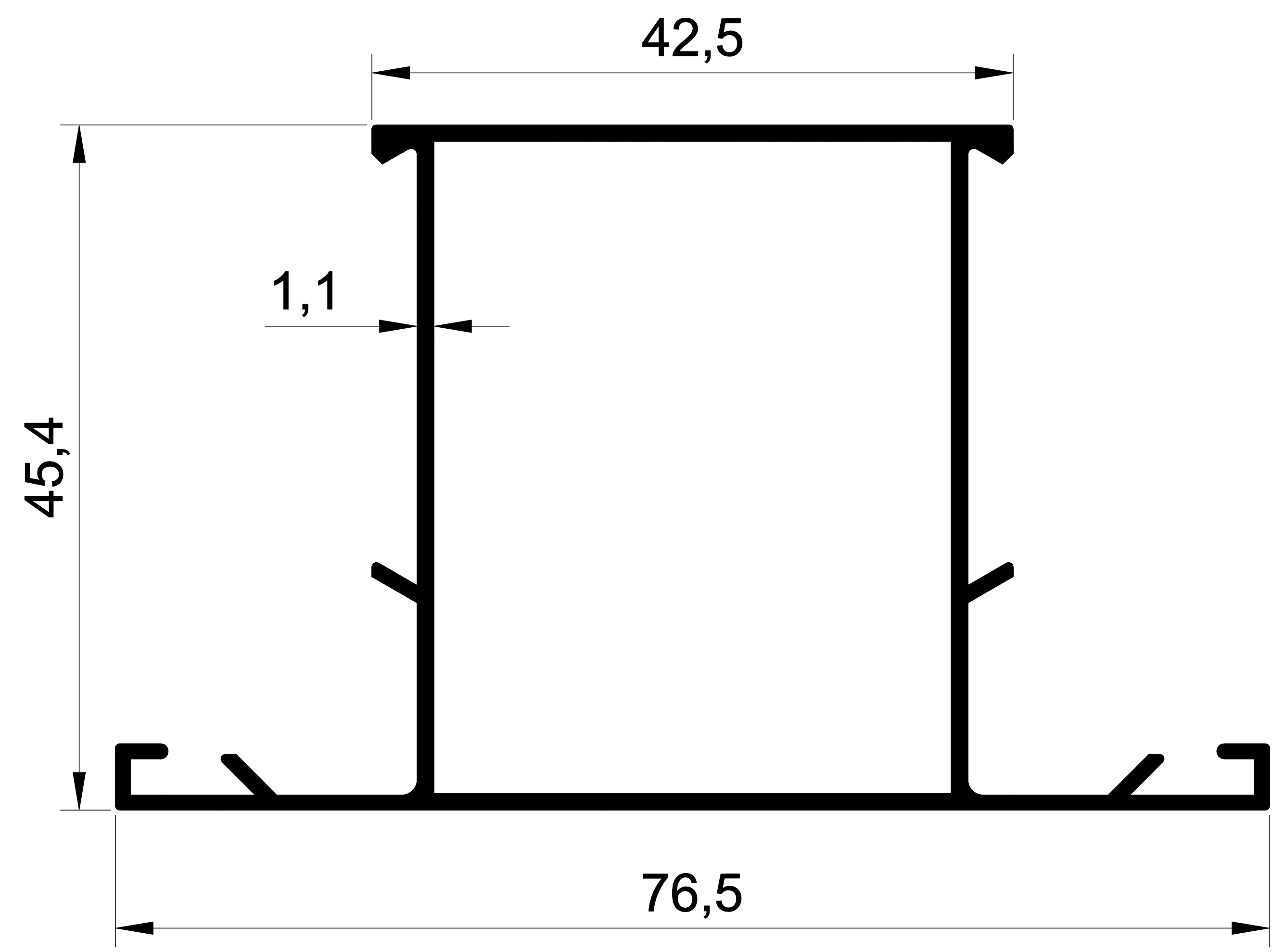
1105 0,645 Kg/m. ALDOKS GENİŞ ORTA
