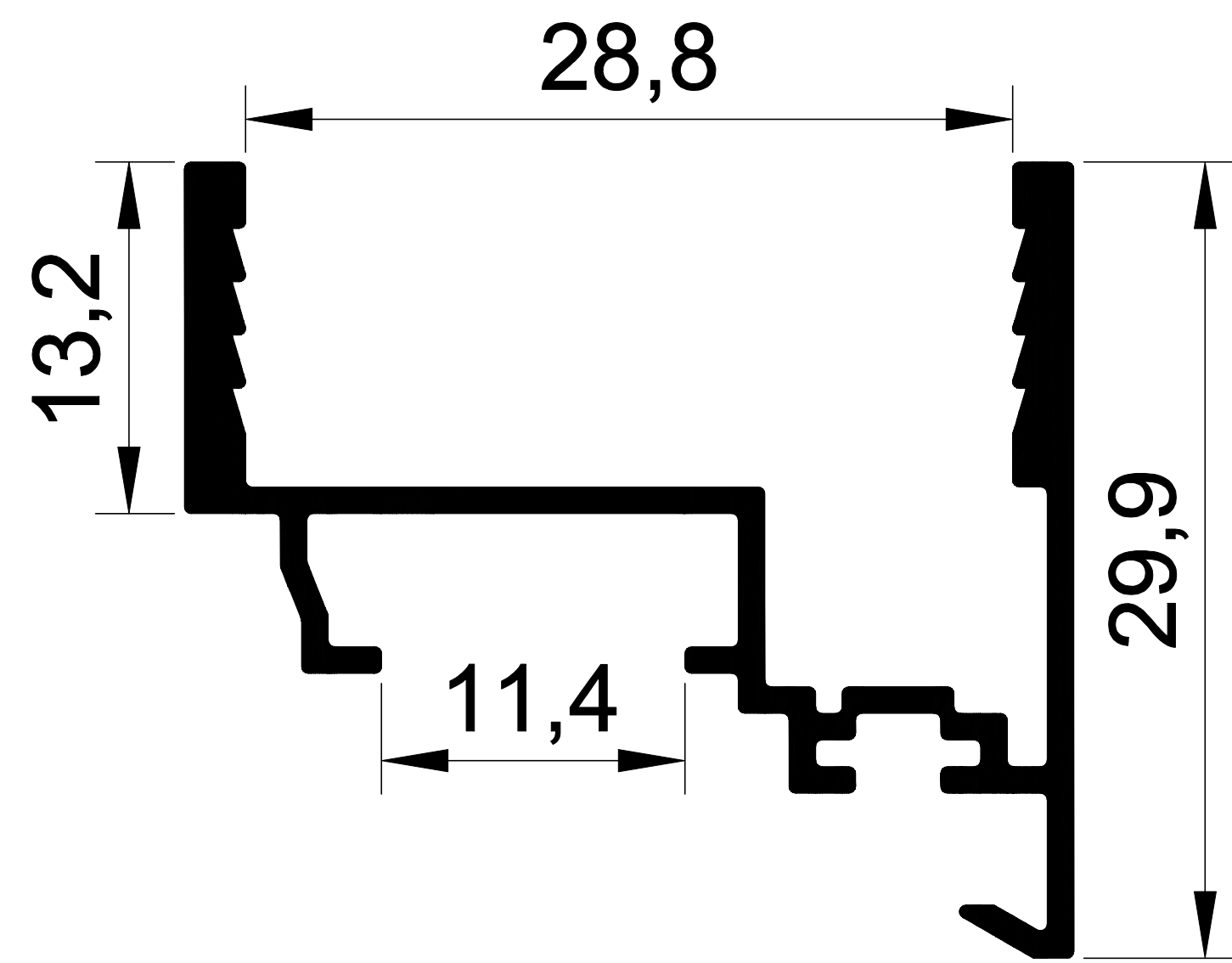
1436 0.358 Kg/m. ISI YALITIM KATLANIR CAM BALKON DÖNÜŞ
