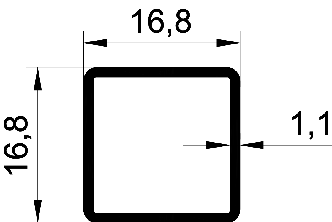
1047 0,181 Kg/m.
