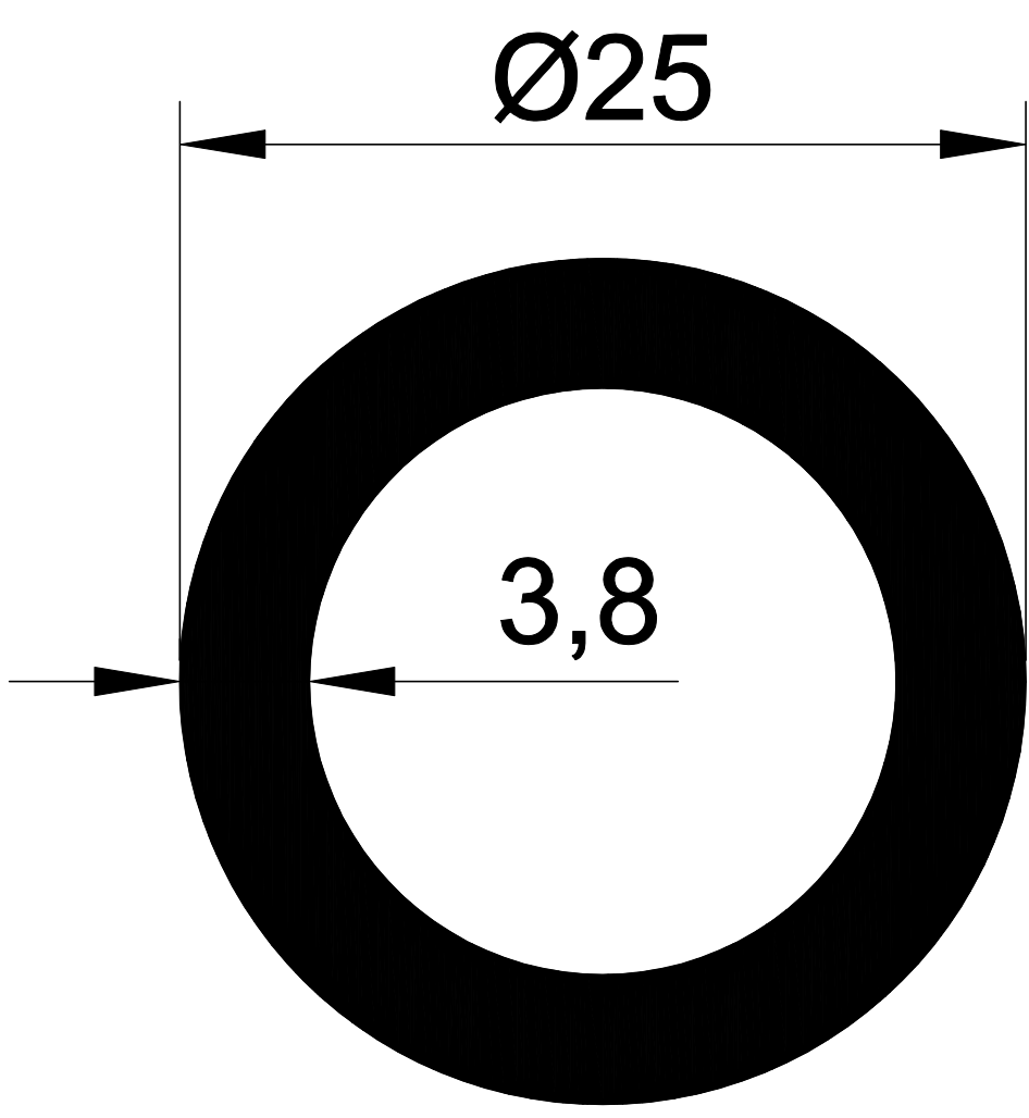
1003 0,680 Kg/m.
