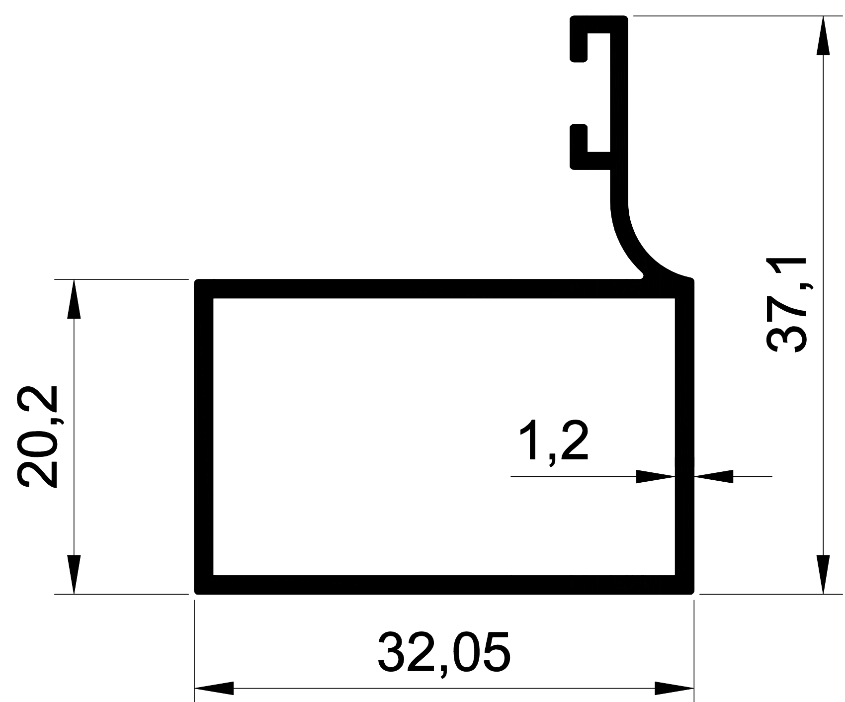
1153 0,404 Kg/m. FIRTINA DIKME
