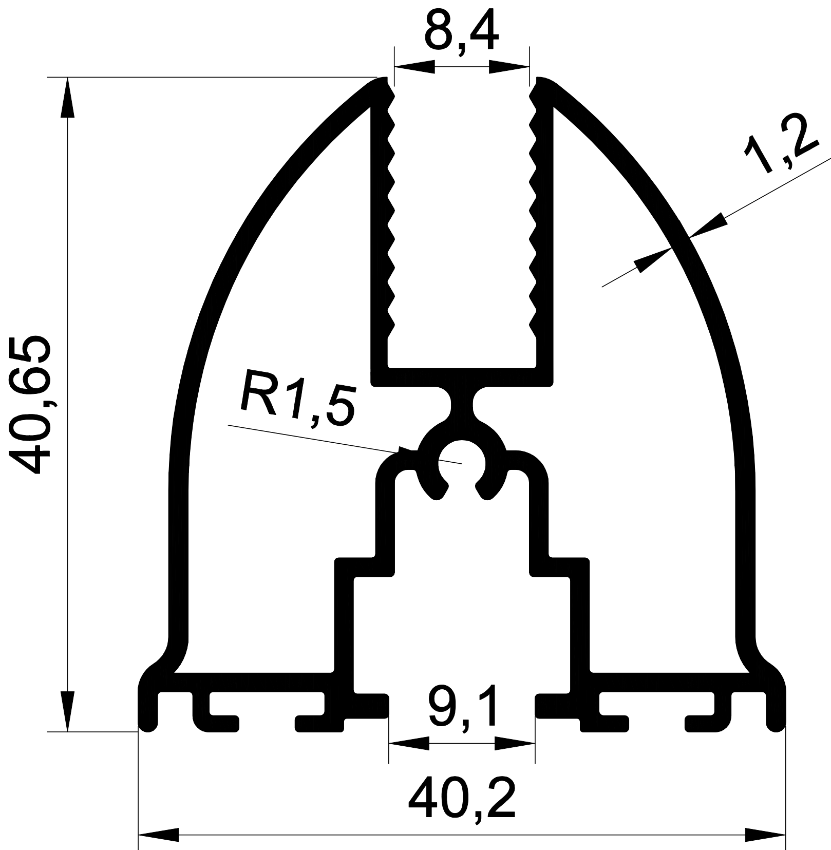
1149 0,738 Kg/m. GOLD KANAT
