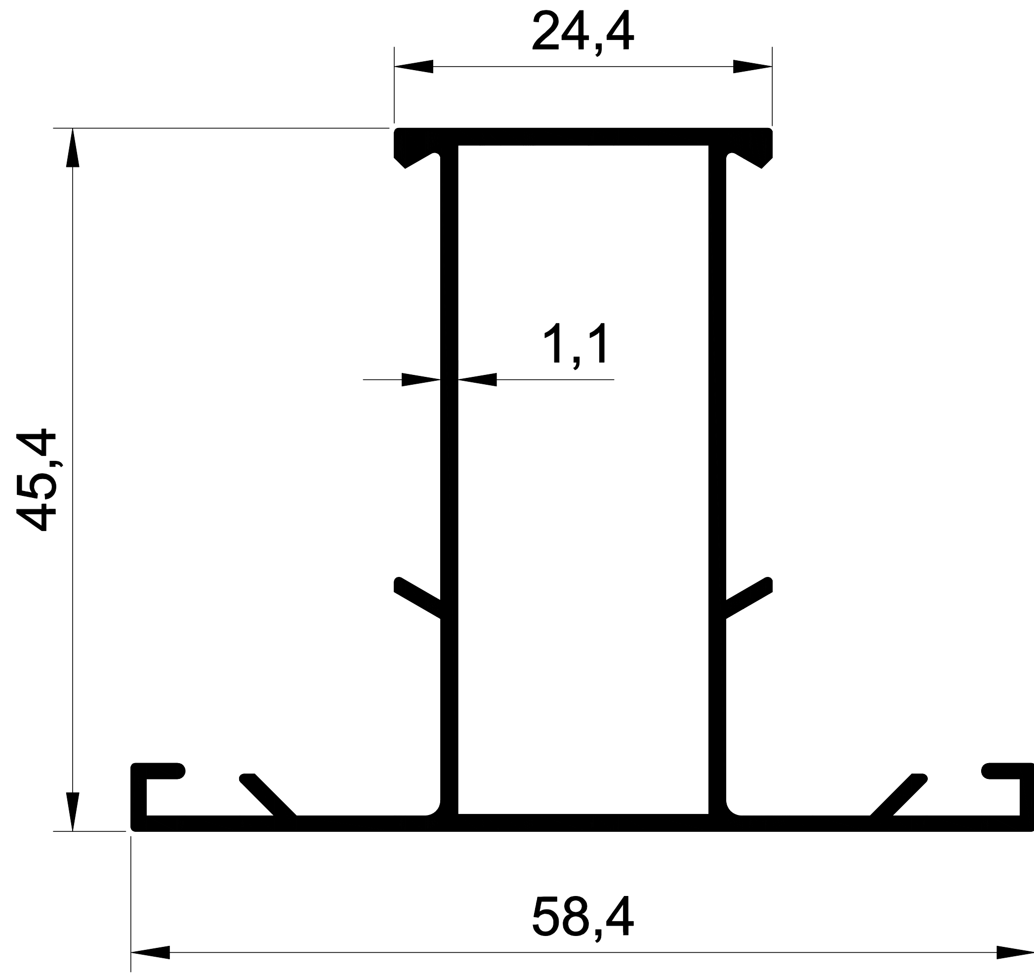
1102 0,547 Kg/m. ALDOKS DAR ORTA
