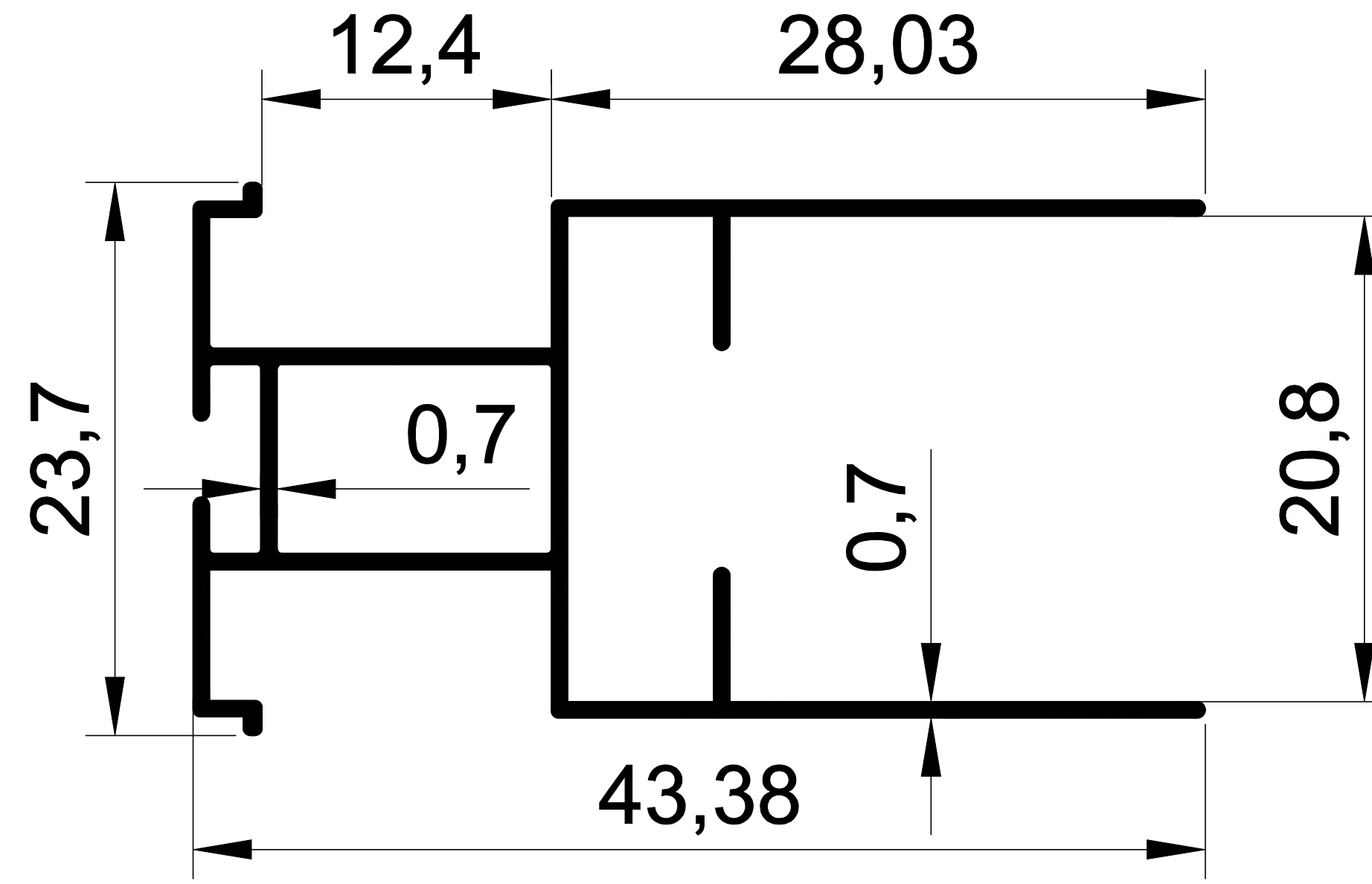
1336 0,285 Kg/m. MAVİ AY SİNEKLİK KANAT
