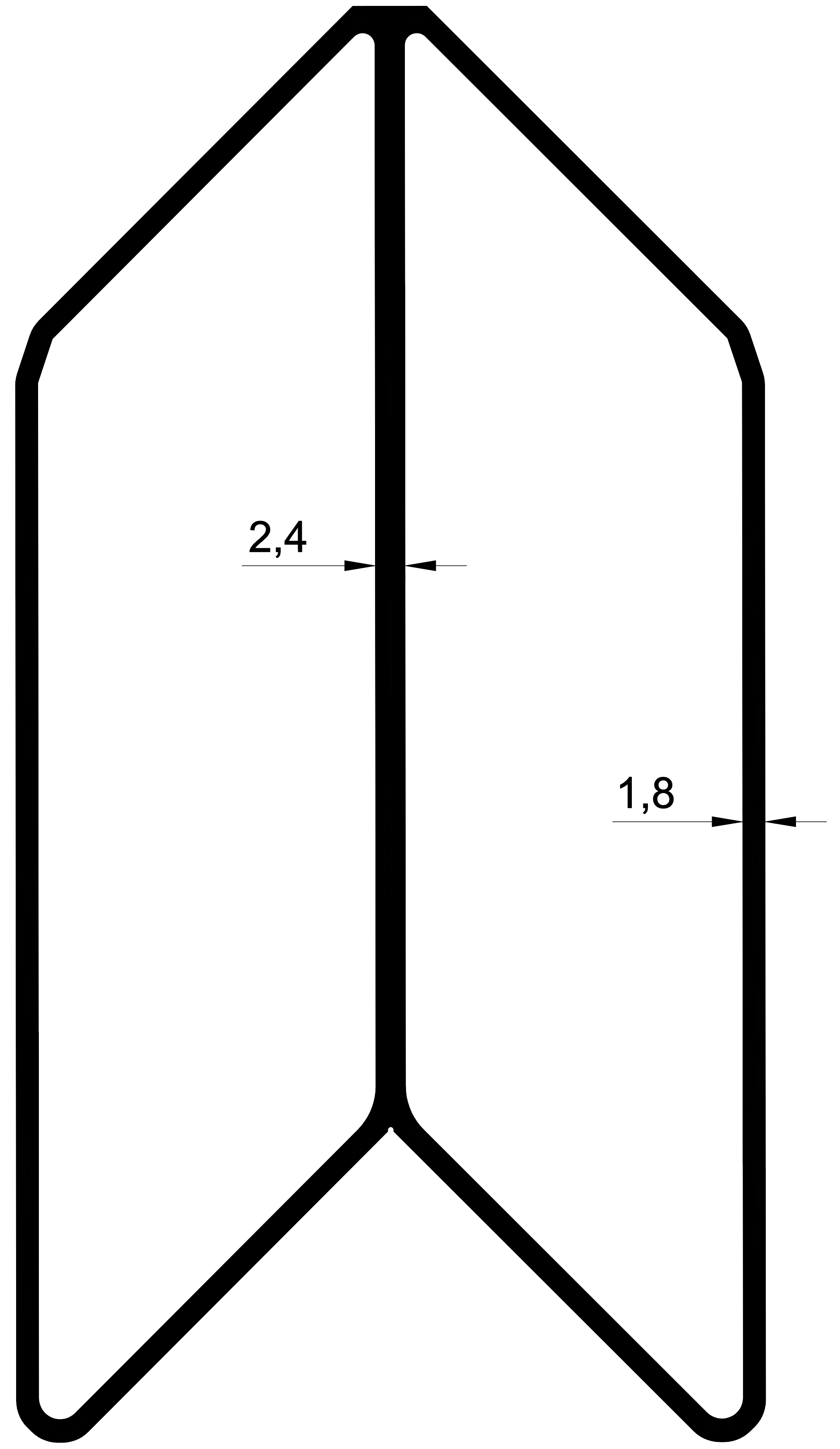
1092 2,205 Kg/m. BAZA ÇAVUŞ (GENİŞ BAĞLANTI)
