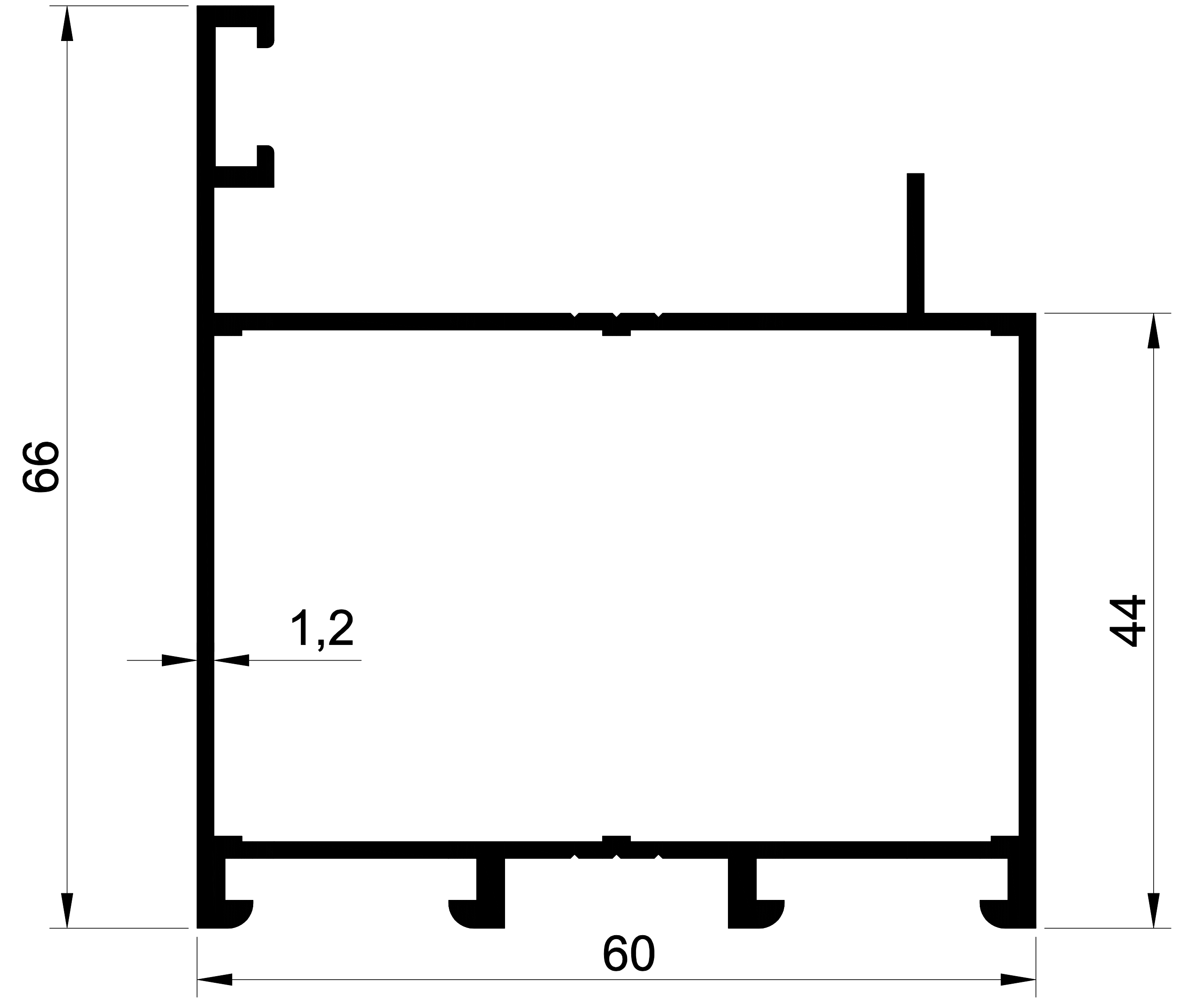
1088 0,935 Kg/m. 1.2 MM C-60 KANAT
