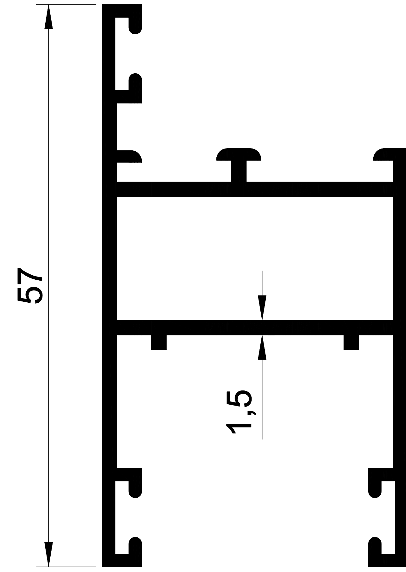
1196 0,753 Kg/m DAR TUBA KANAT
