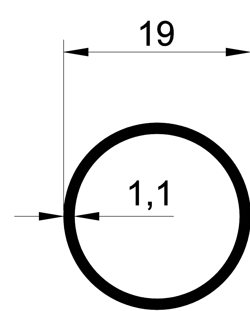
1035 0,152 Kg/m.
