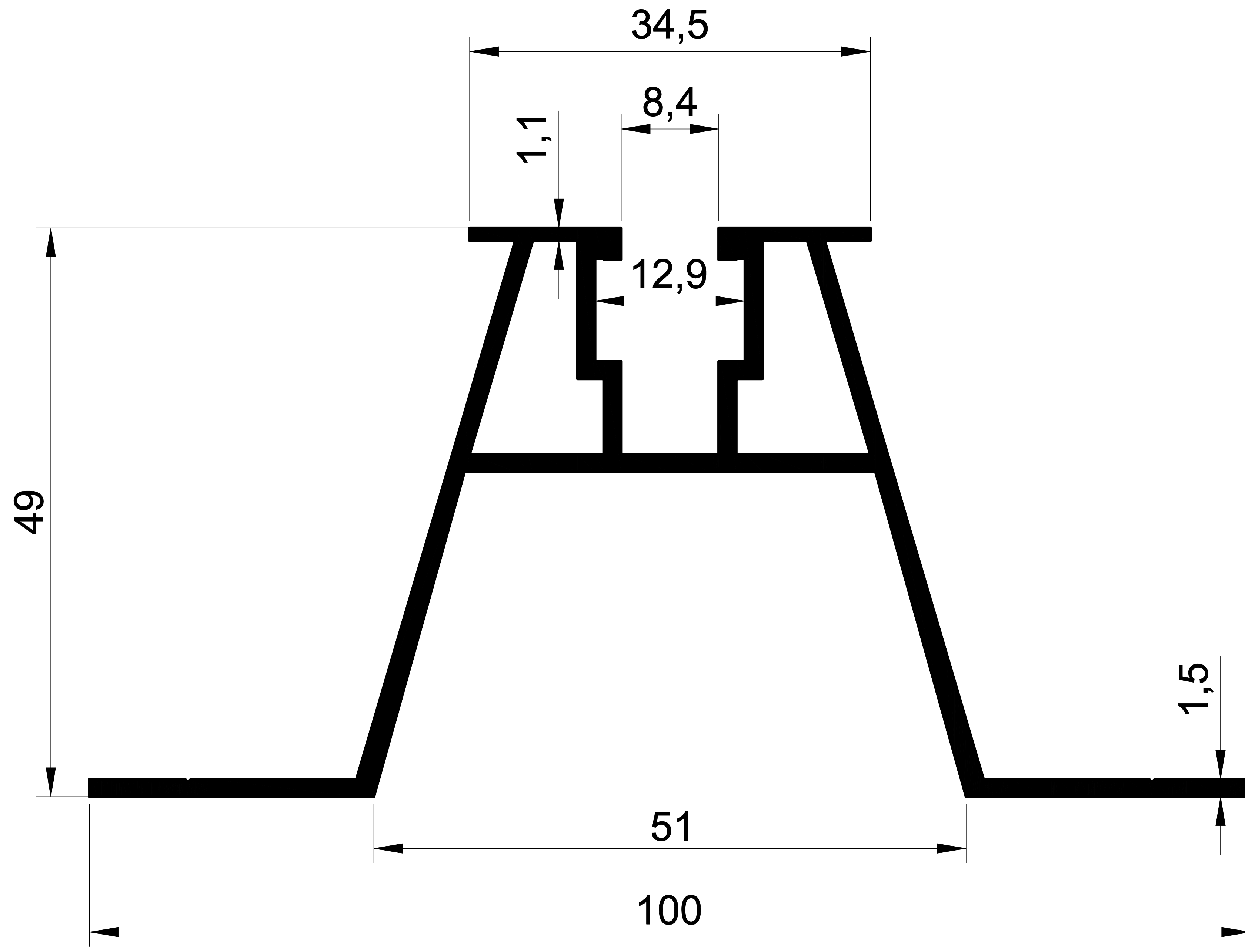
1429 1,009 Kg/m GES ALT KONTRÜKSİYON
