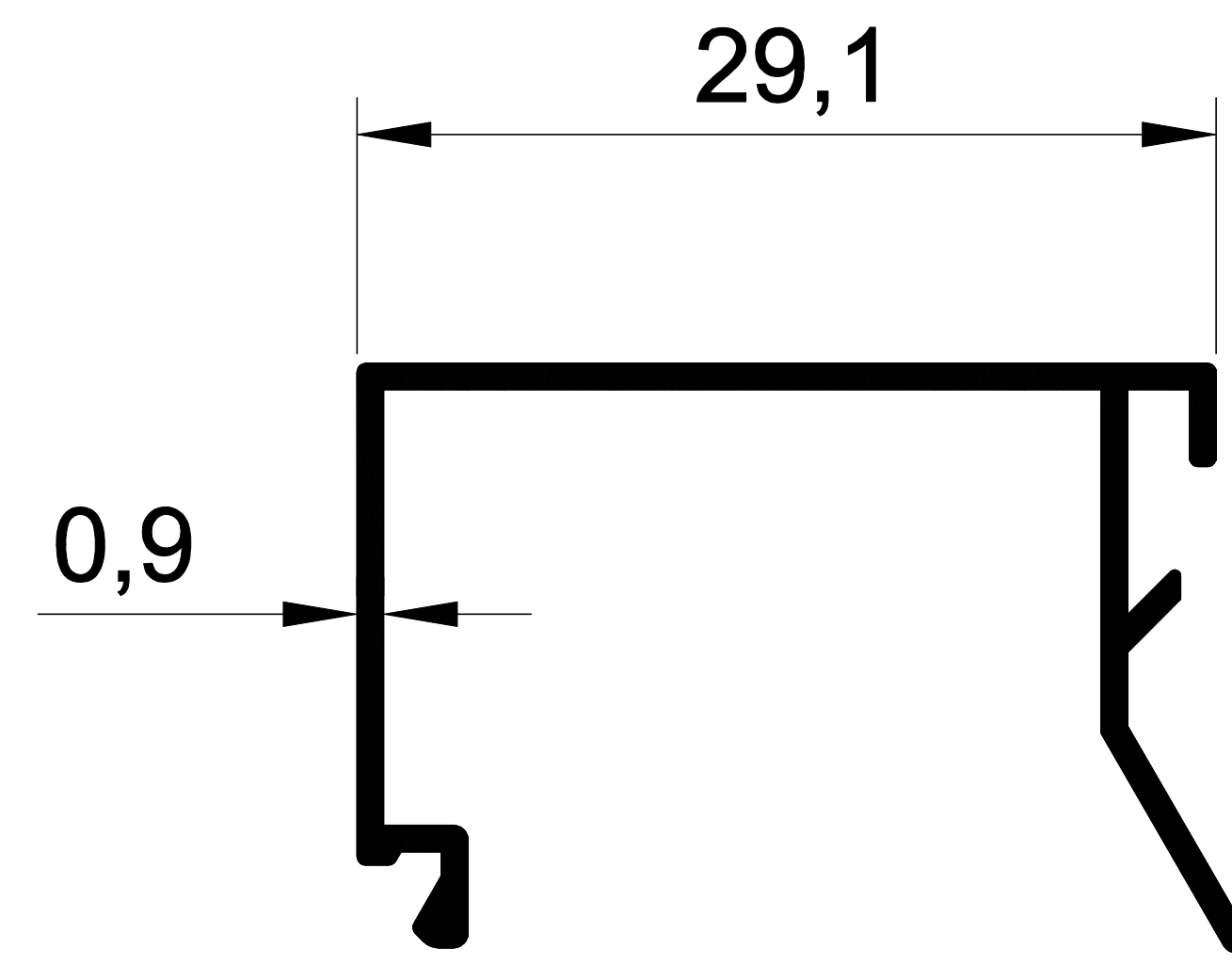
1090 0,191 Kg/m ALDOKS TEK CAM ÇİTASI
