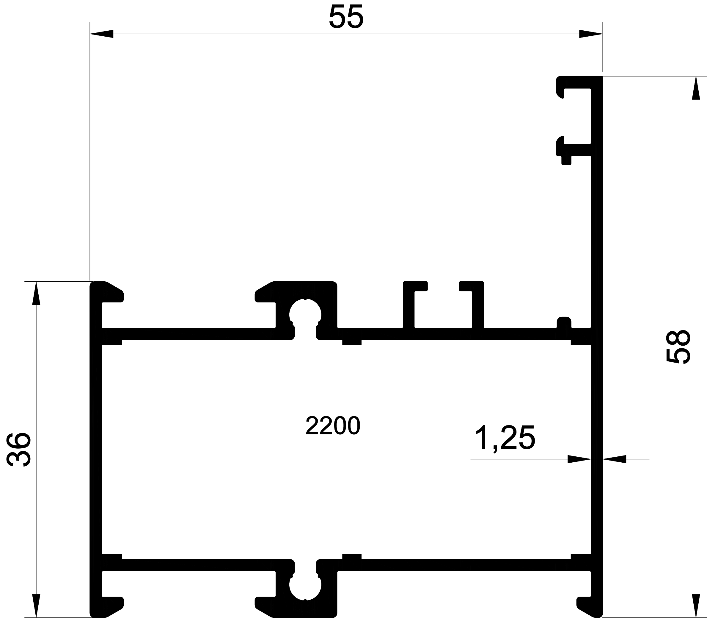
EK-55- 2200 0,929 Kg/m SİSTEM 55 YALITIMSIZ KASA
