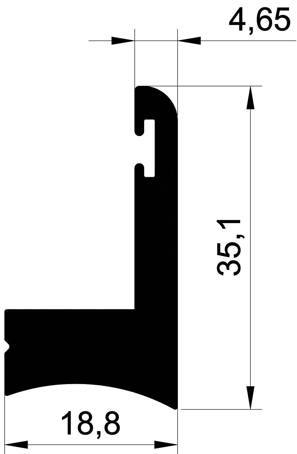
1127 0,715 Kg/m.
