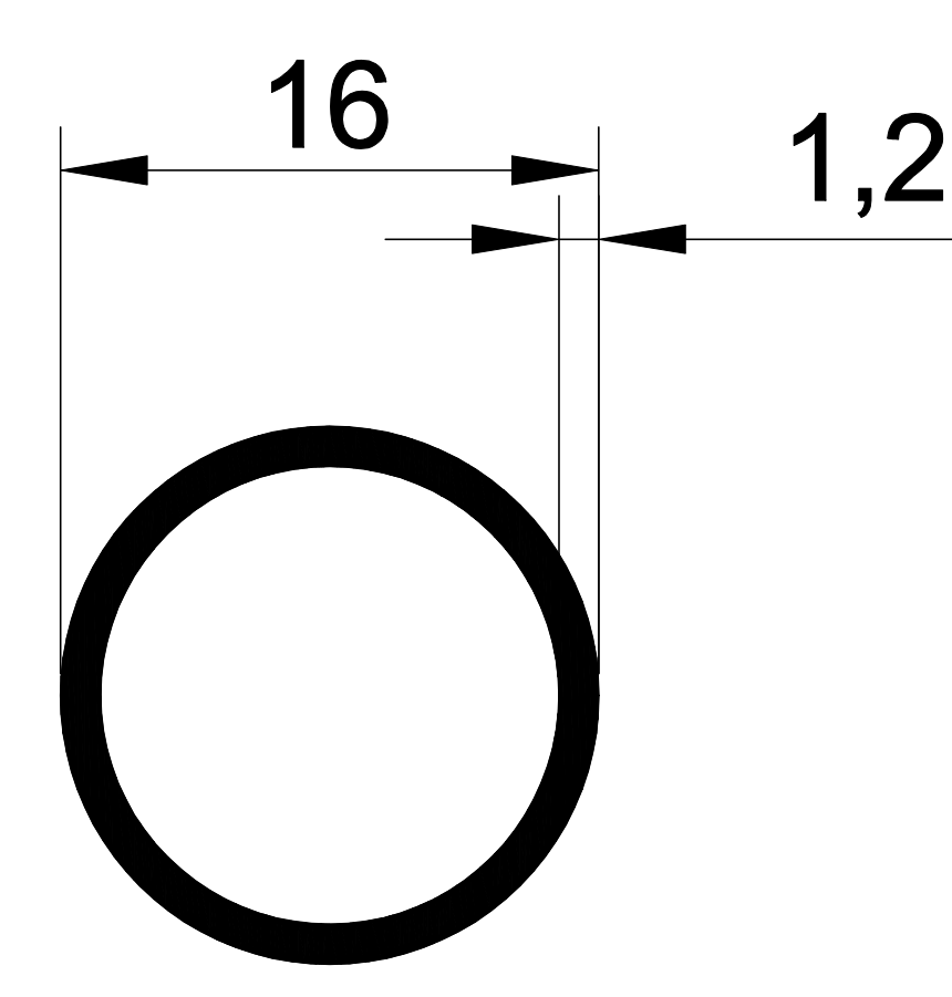
1343 0,140 Kg/m.
