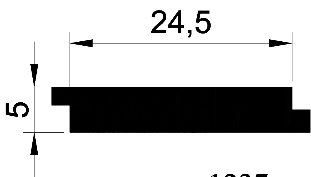
1237 0,358 Kg/m.
