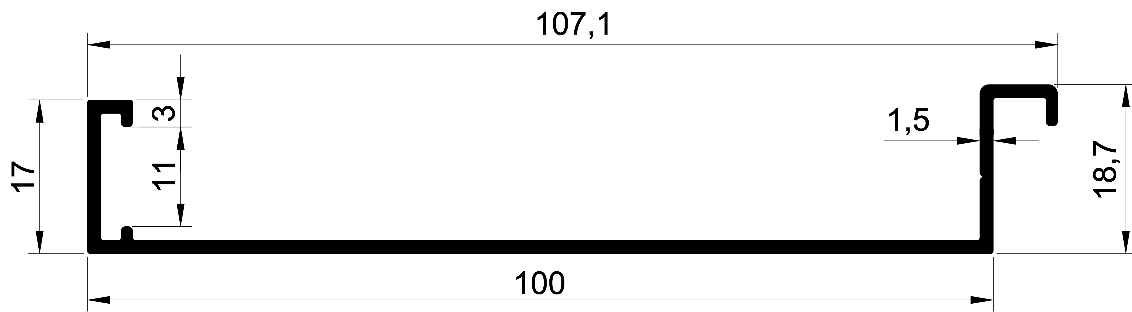
1426 0,602 Kg/m. MS-PEERVAZ UZATMA PROFİLİ
