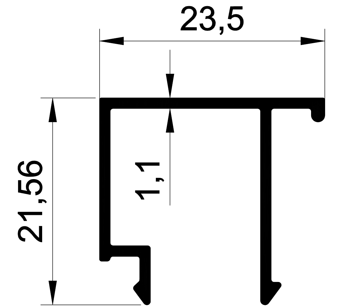
1086 0,215 Kg/m C-60 TEK CAM ÇİTASI
