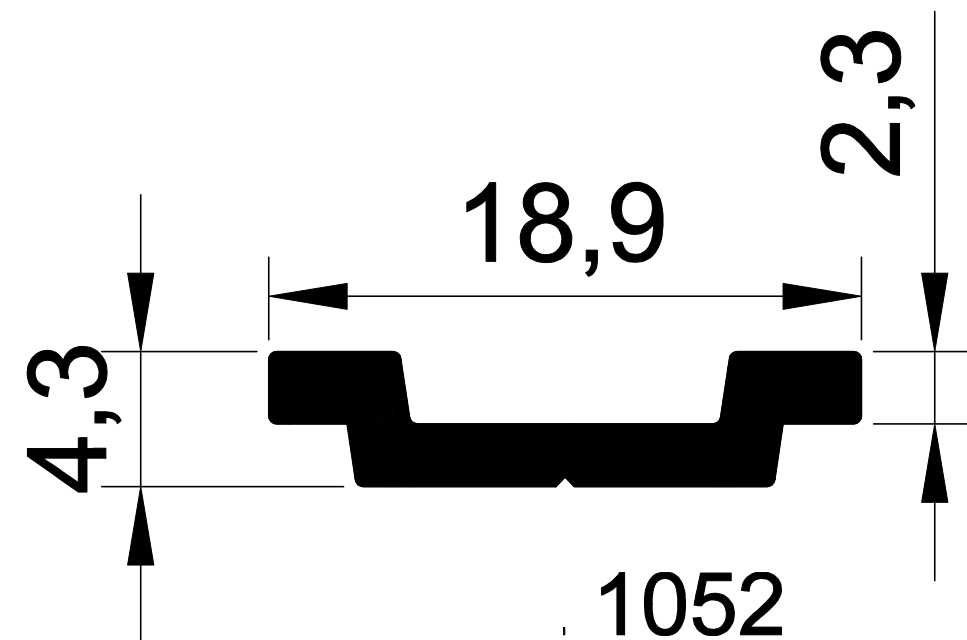
1052 0,127 Kg/m. TİJ ÇUBUĞU İÇİ
