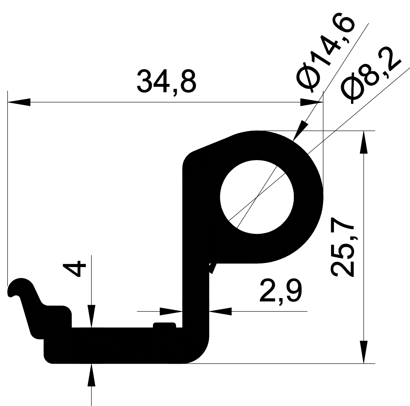
1058 0,686 Kg/m.
