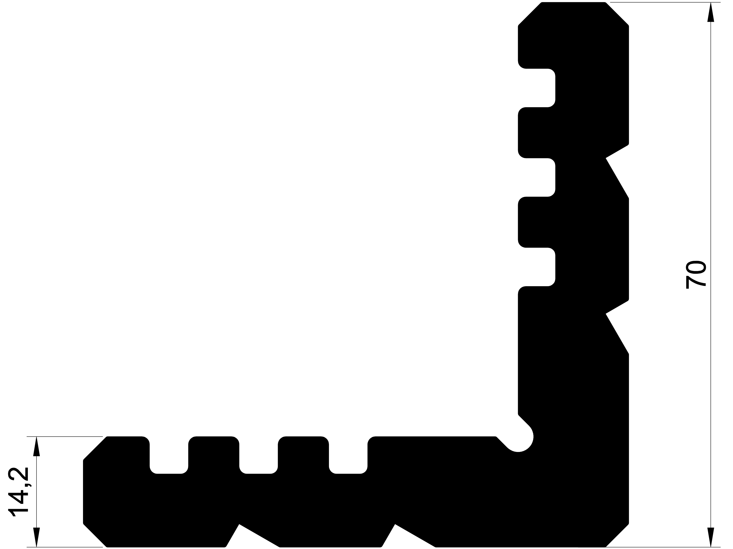
1402 1,402 Kg/m. 14'LÜK CEPHE KÖŞE
