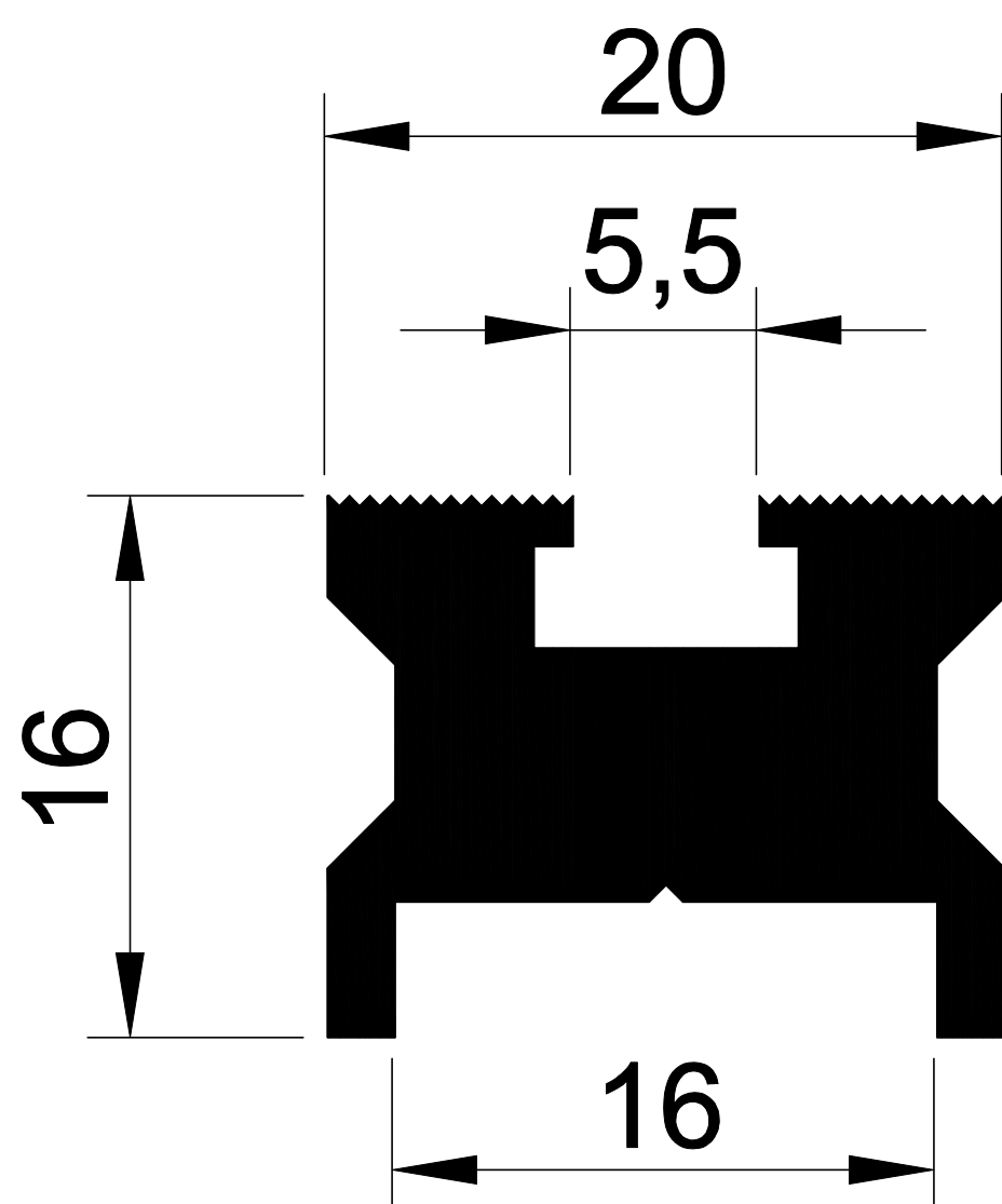
1243 0,537 Kg/m.
