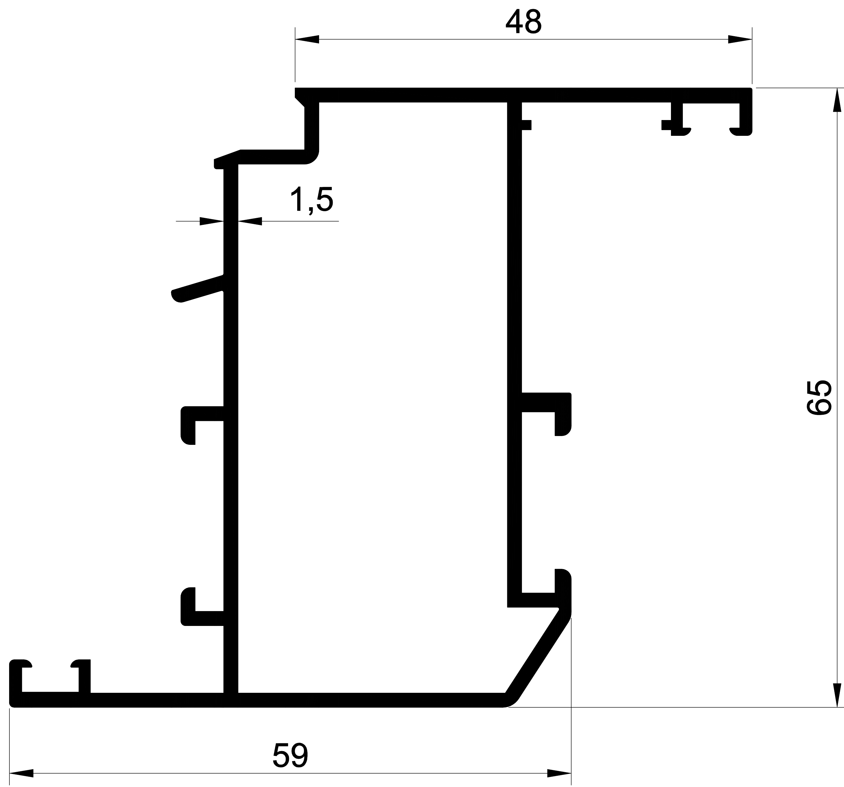
1201 1,168 Kg/m. SİSTEM KANAT
