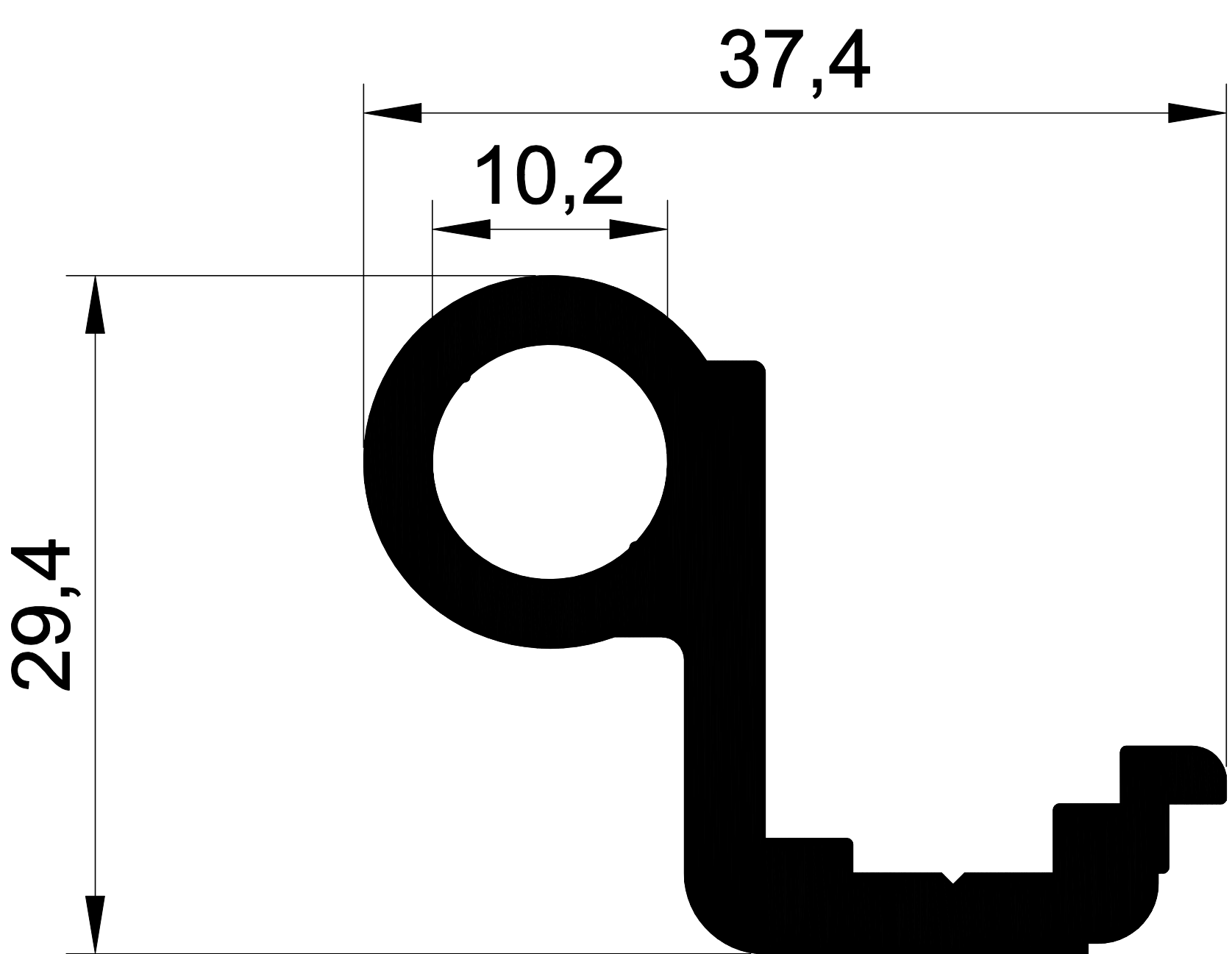
1259 0,772 Kg/m.
