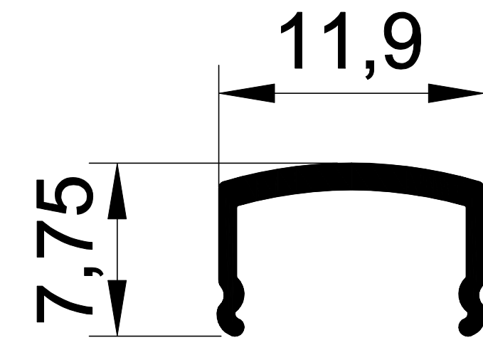
1123 0,065 Kg/m.
