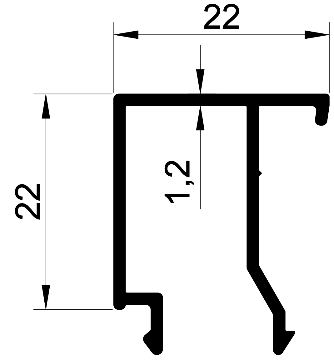
-55- 2008 0,264 Kg/m SİSTEM 55 ÇİFT CAM ÇİTASI
