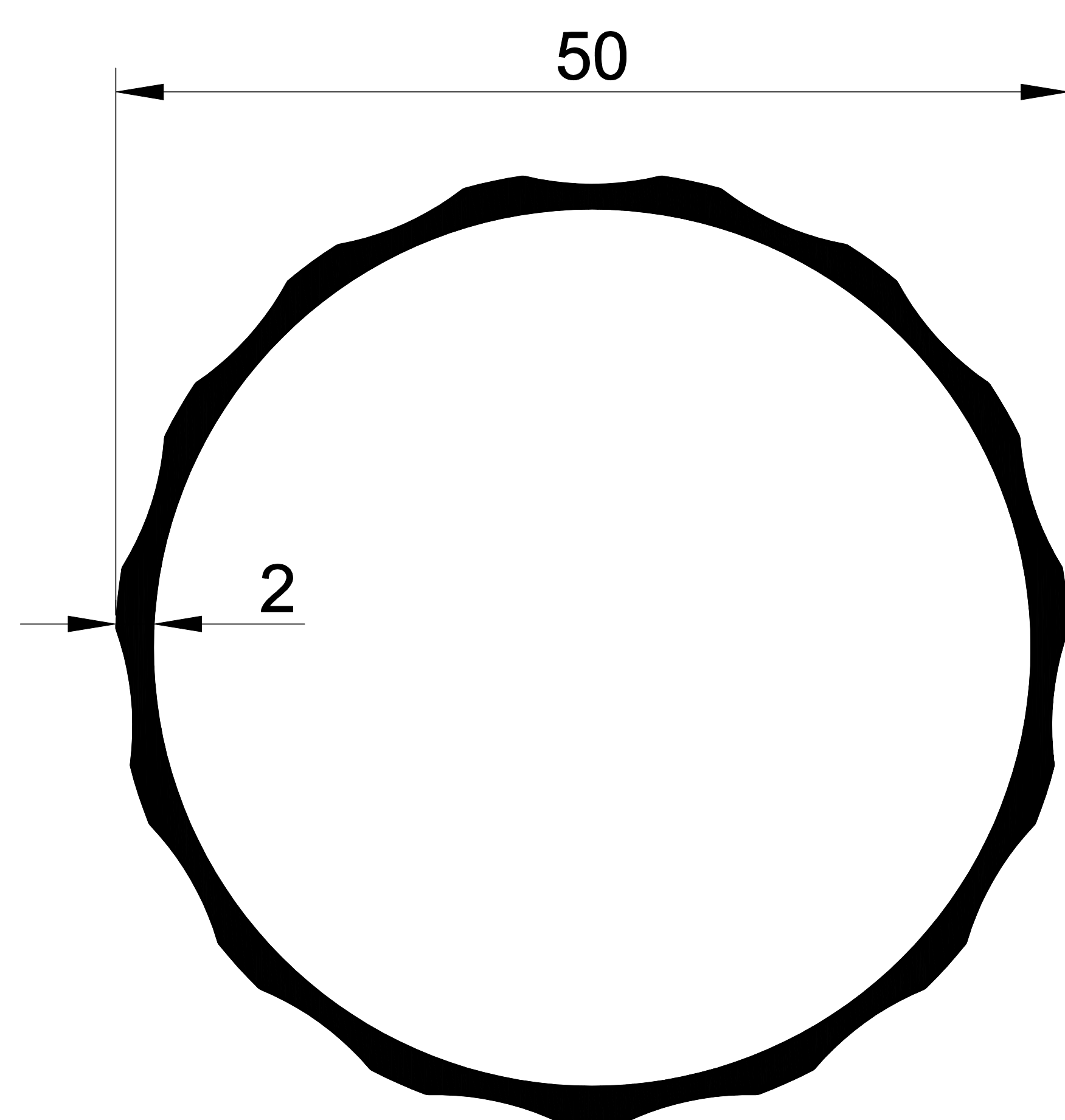
1163 0,680 Kg/m.
