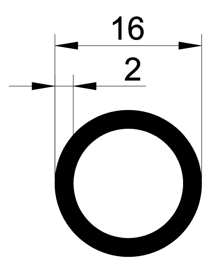
1068 0,240 Kg/m.
