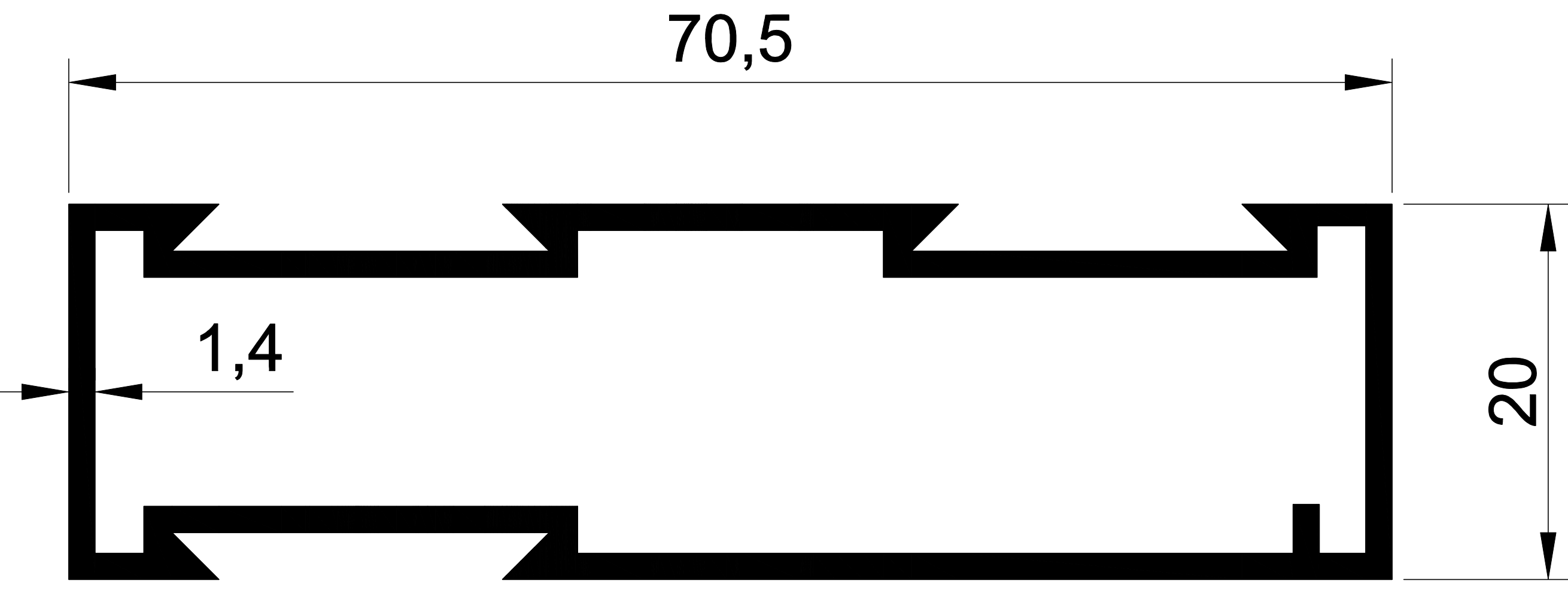
1197 0,786 Kg/m. DAR TUBA KASA
