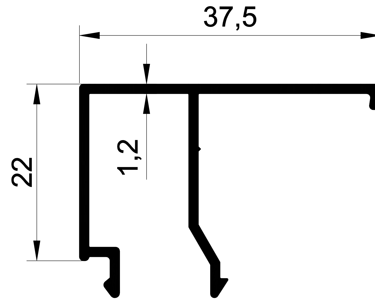
-55- 2009 0,314 Kg/m SİSTEM 55 TEK CAM ÇITASİ
