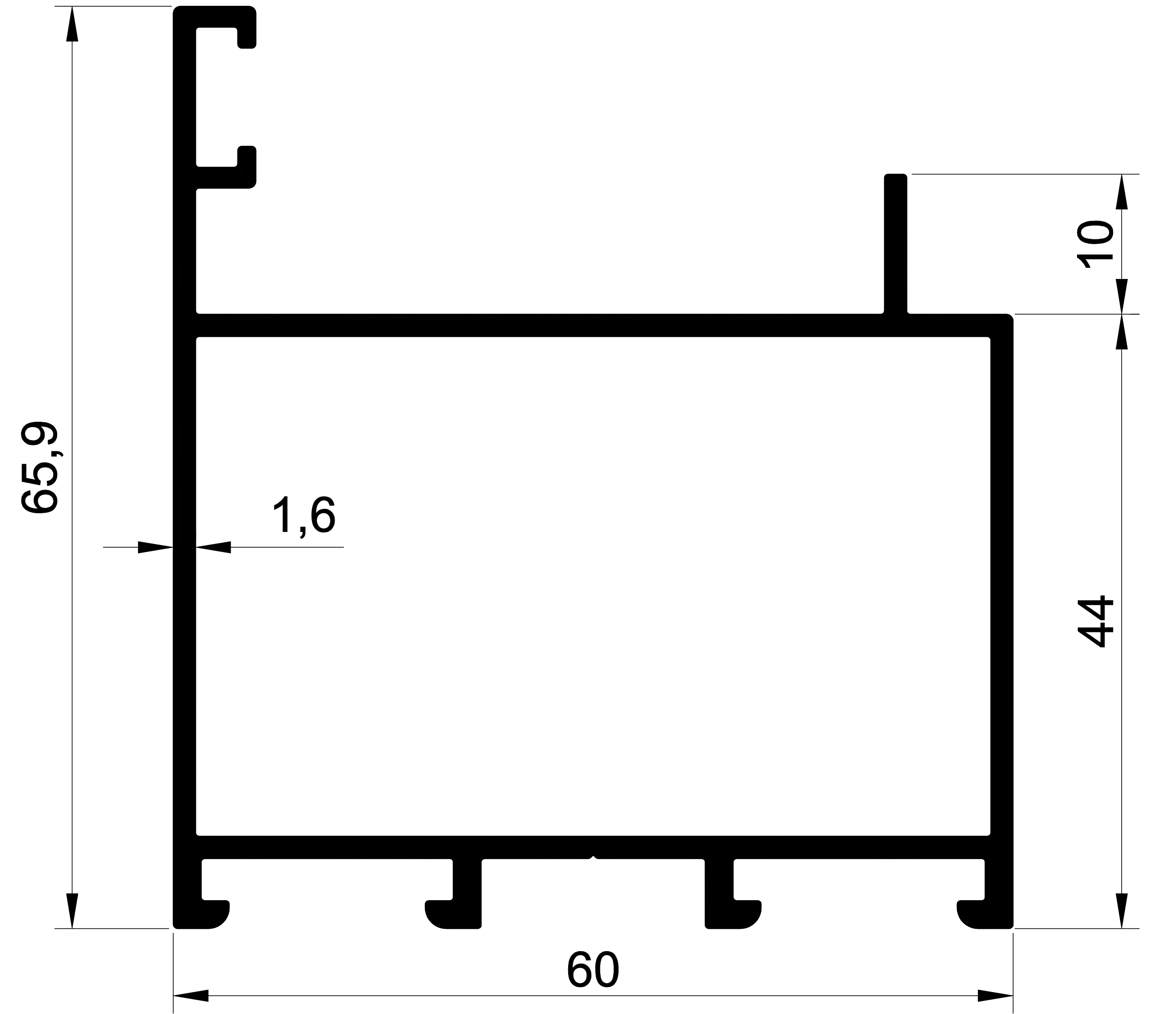
1406 1,160 Kg/m. 1.6 MM C-60 KANAT
