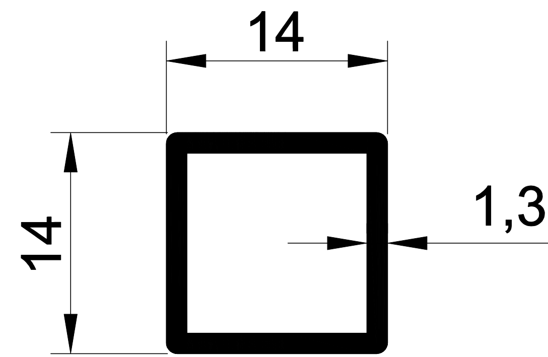
1131 0,179 Kg/m. 14X14 BARIYER
