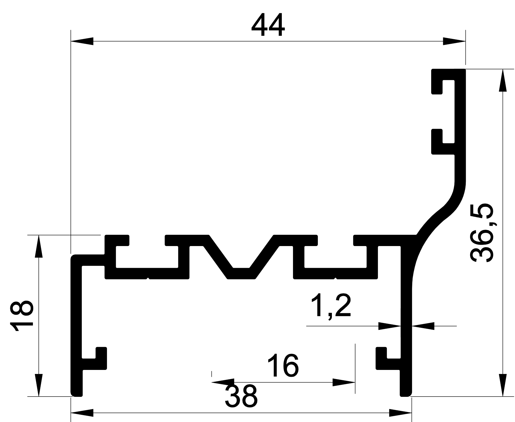
- 2302 0,438 gr/m ISICAMLI CAM BALKON PROFİLLERİ
