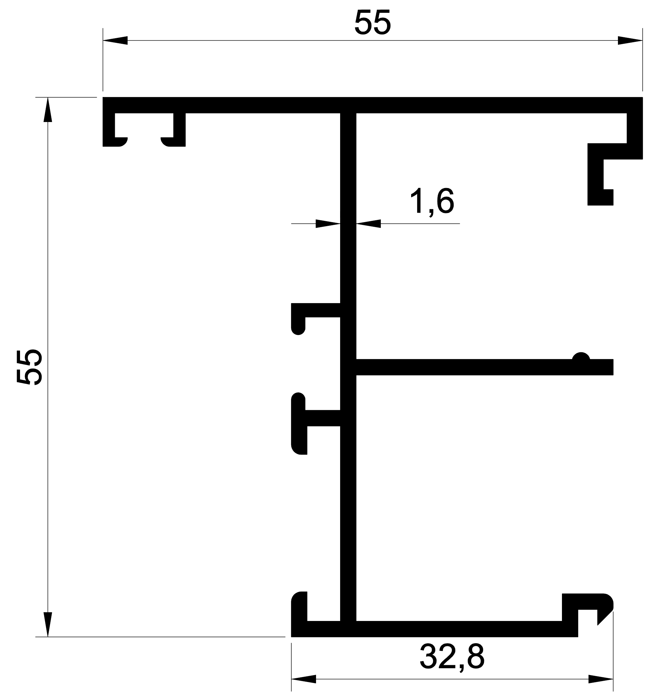
1354 0,915 Kg/m. SİSTEM ÇİFT KAPI ADAPTÖRÜ
