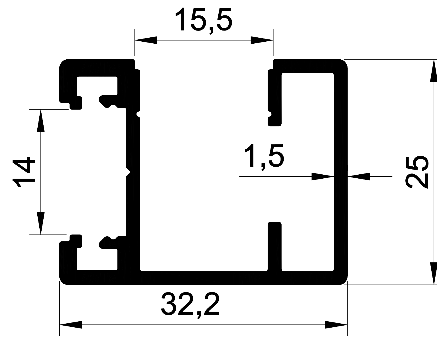
1269 0,504 Kg/m 32*25 GEMİCİ
