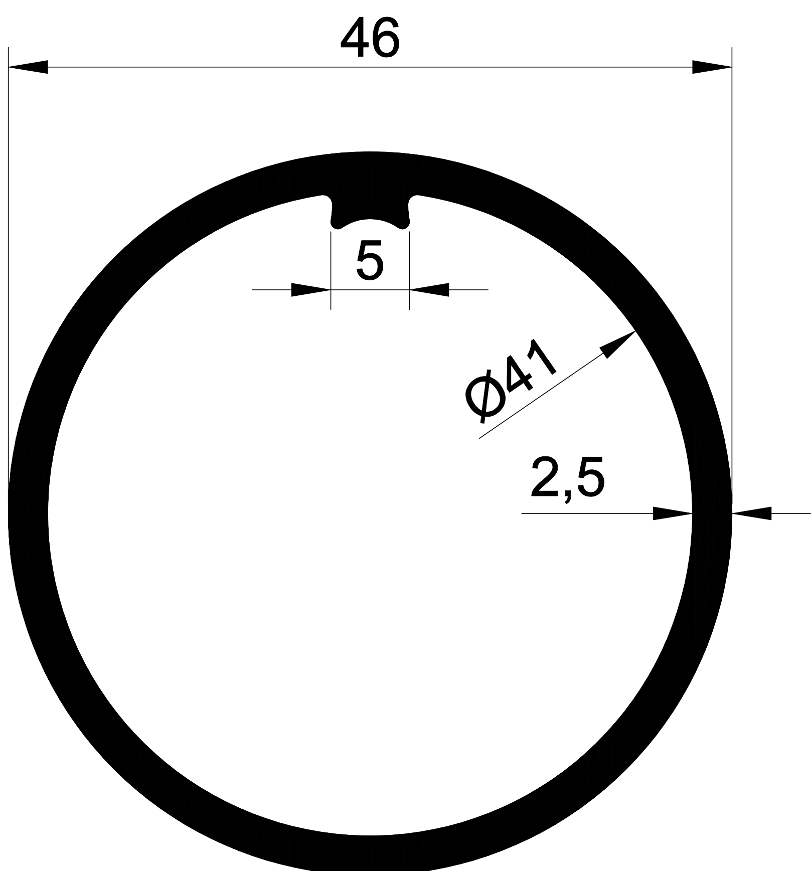
1018-B 0,954 Kg/m.
