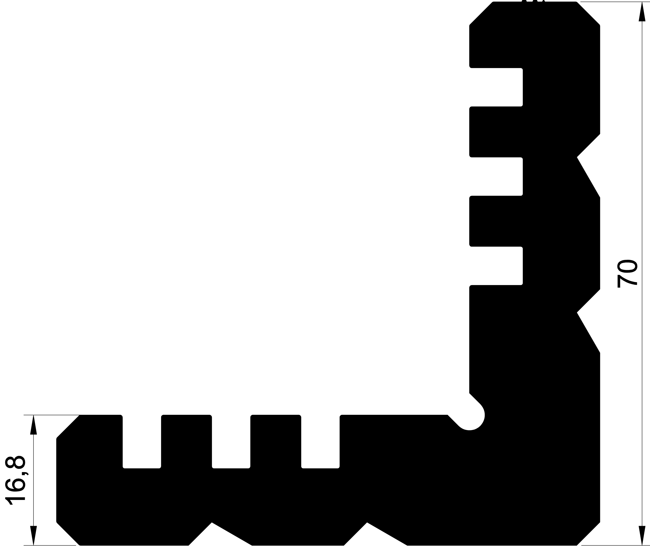
1399 4,827 Kg/m. 17 MM CEPHE KÖŞE
