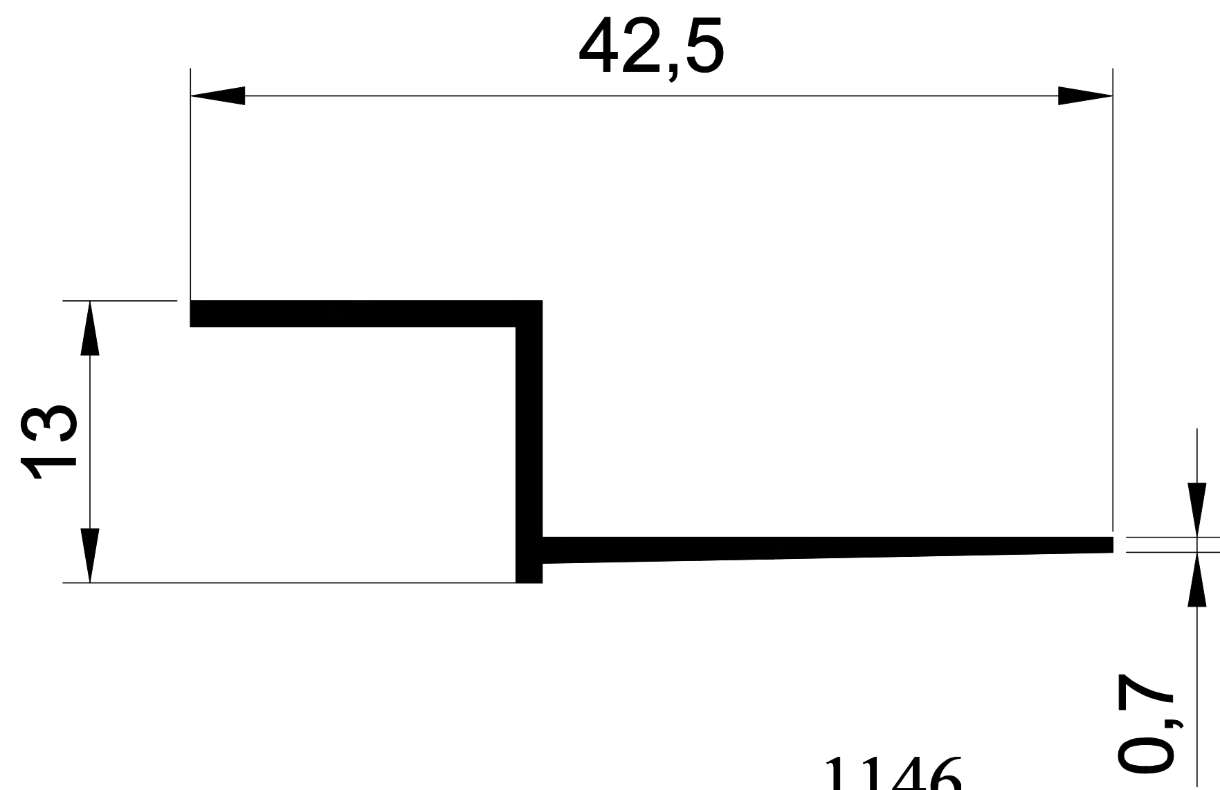
1146 0,160 Kg/m.
