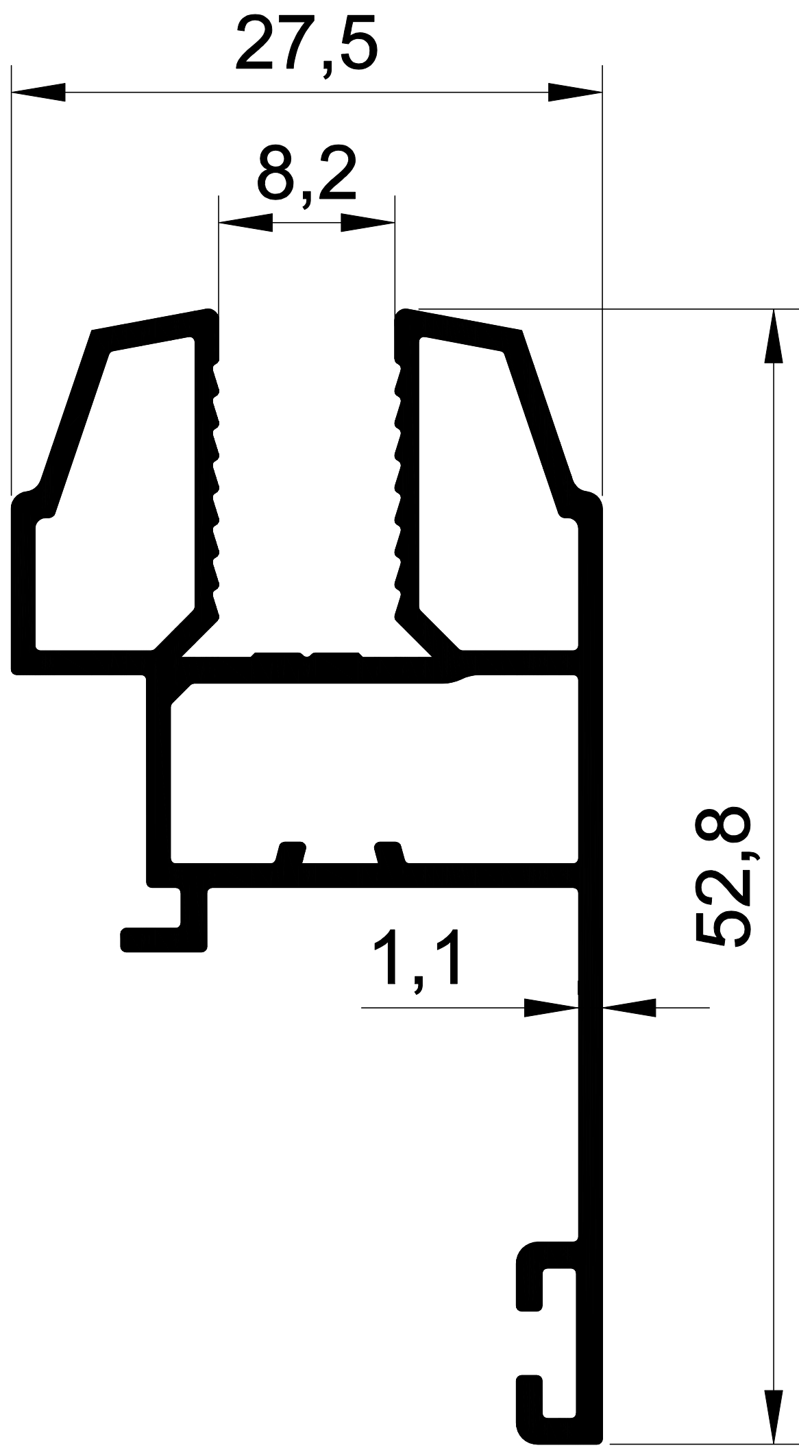
1379 0,549 Kg/m. 53'LÜK CAM BALKON KİLİT
