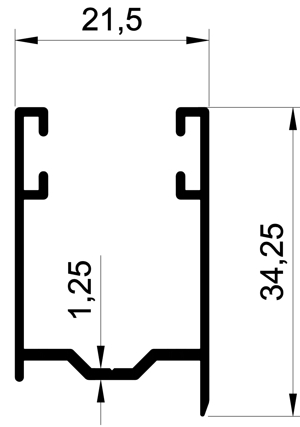
1310 0,287 Kg/m. MAKAS FİTİLLİ U
