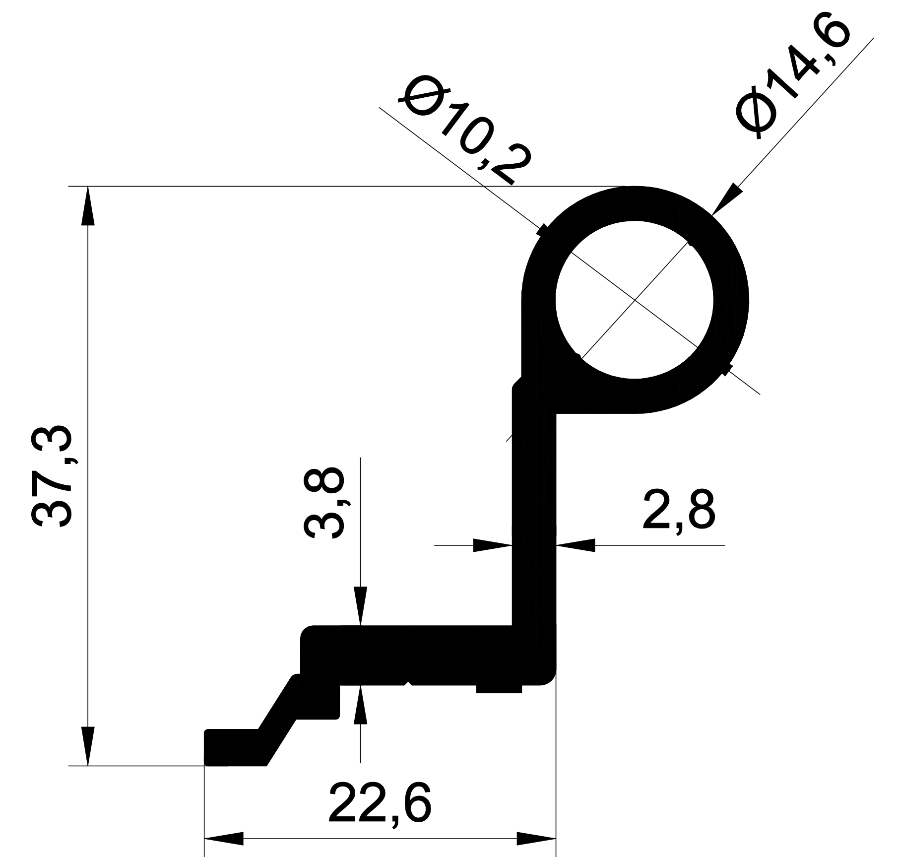
1008 0,775 Kg/m.
