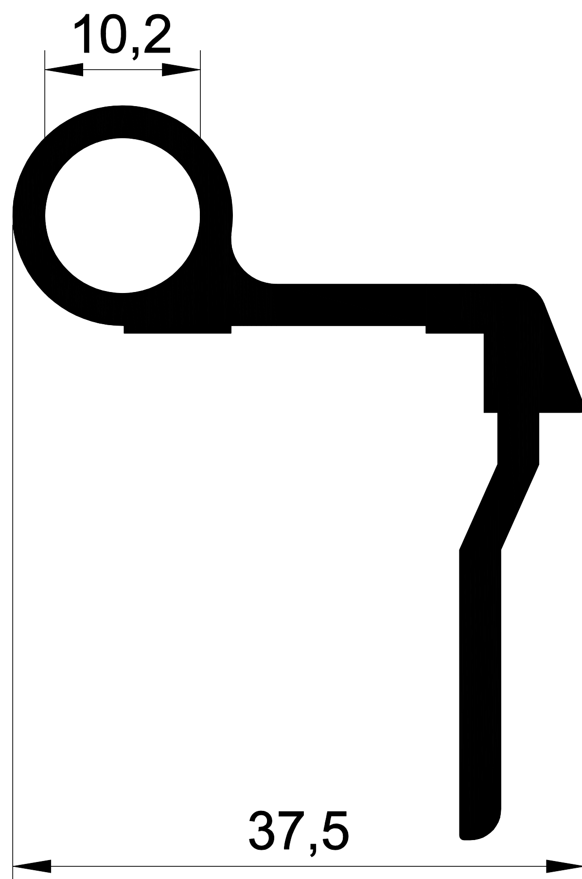
1318 0,707 Kg/m.
