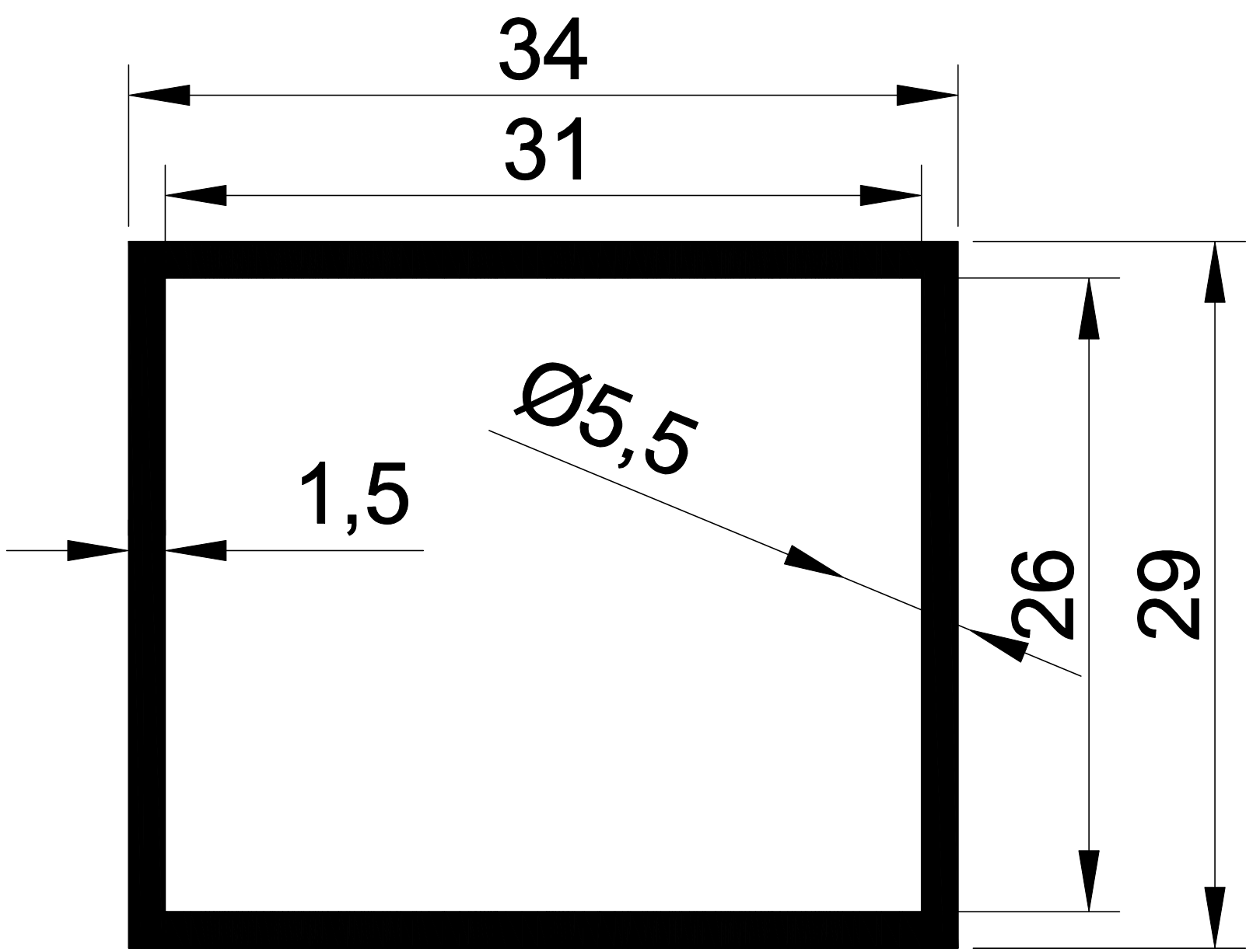
1460 0,487 Kg/m
