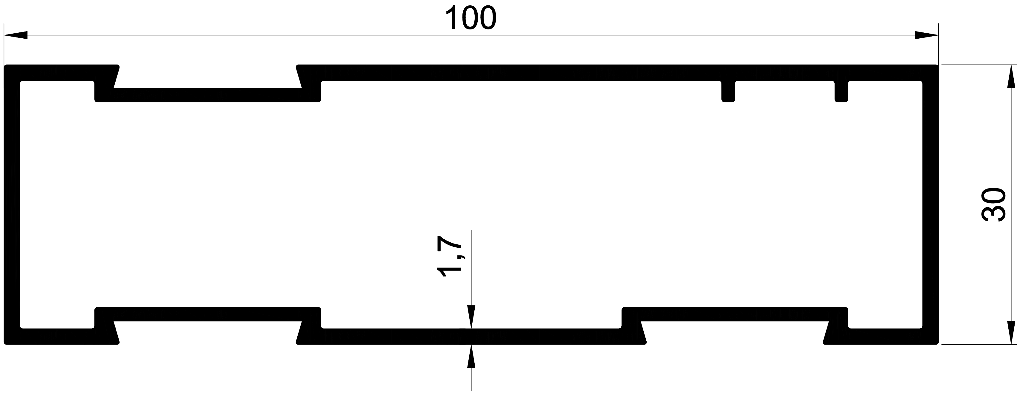
1385 1,240 Kg/m. 100'LÜK TUBA KASA
