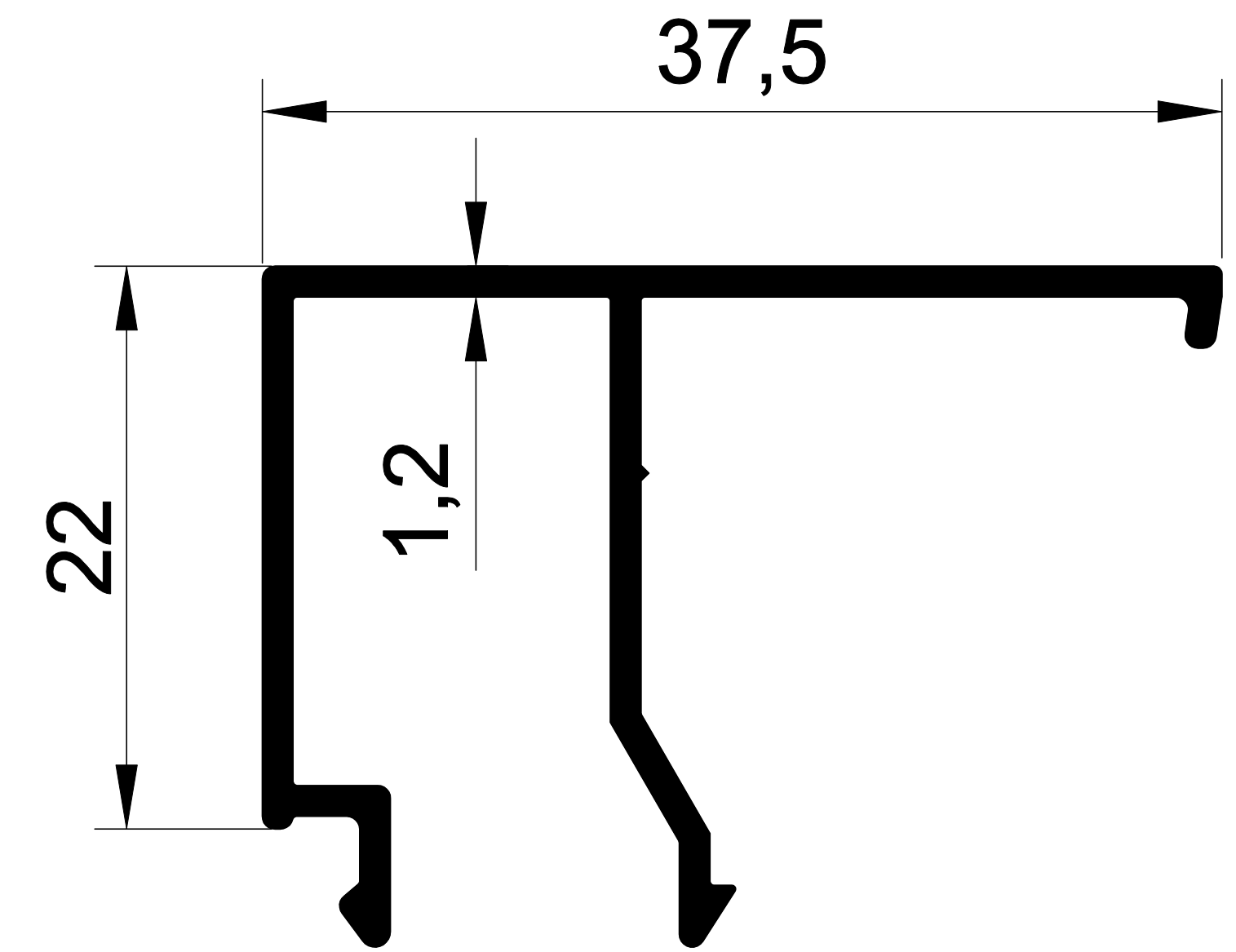
-55- 2009 0,314 Kg/m SİSTEM 55 TEK CAM ÇİTASI
