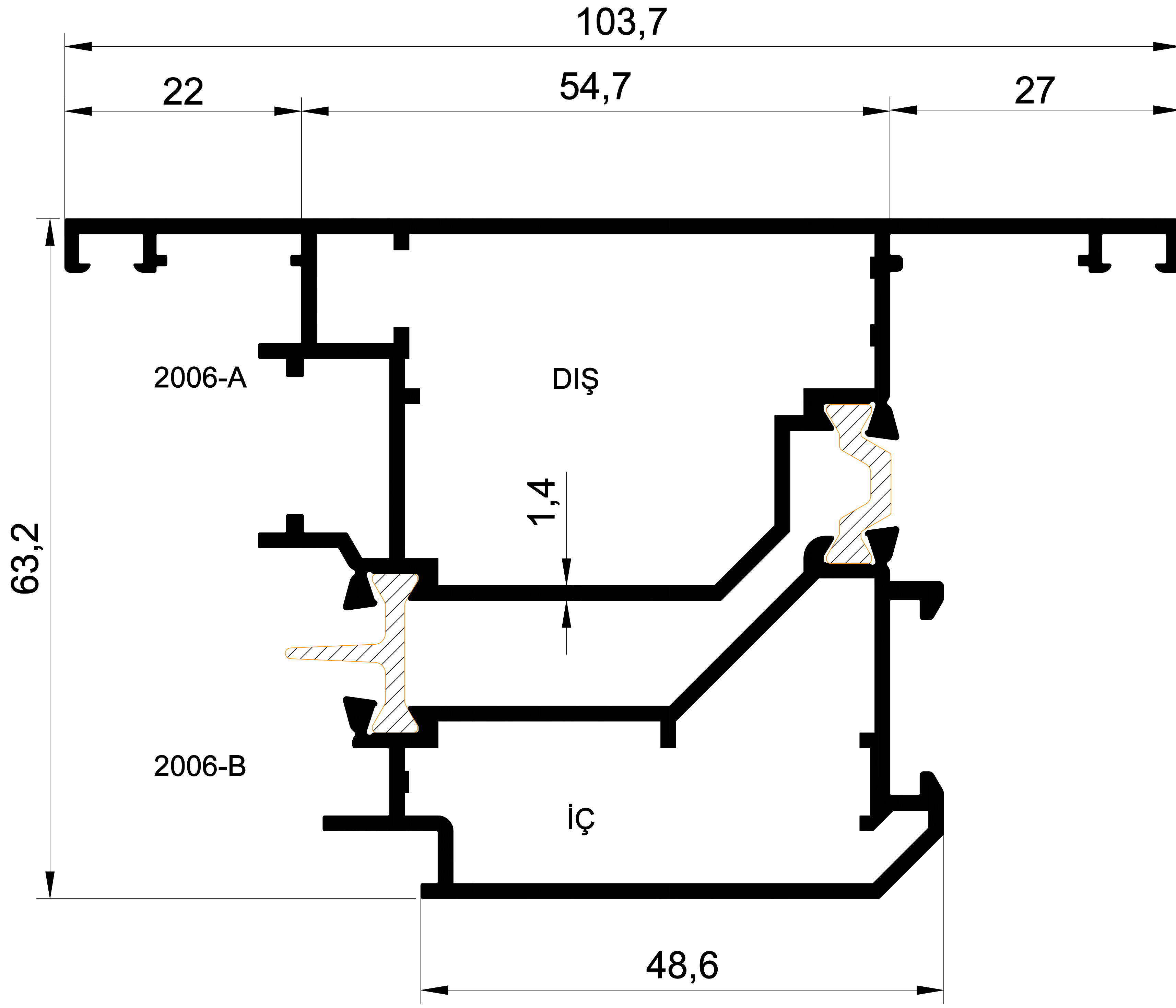
-55- 2006 1,794 Kg/m SİSTEM 55 ISI YALITIM DIŞA AÇILIR KAPI
