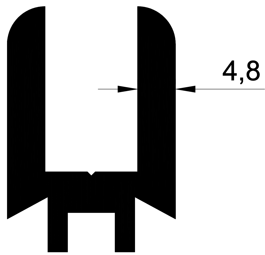
1217 0,870 Kg/m.
