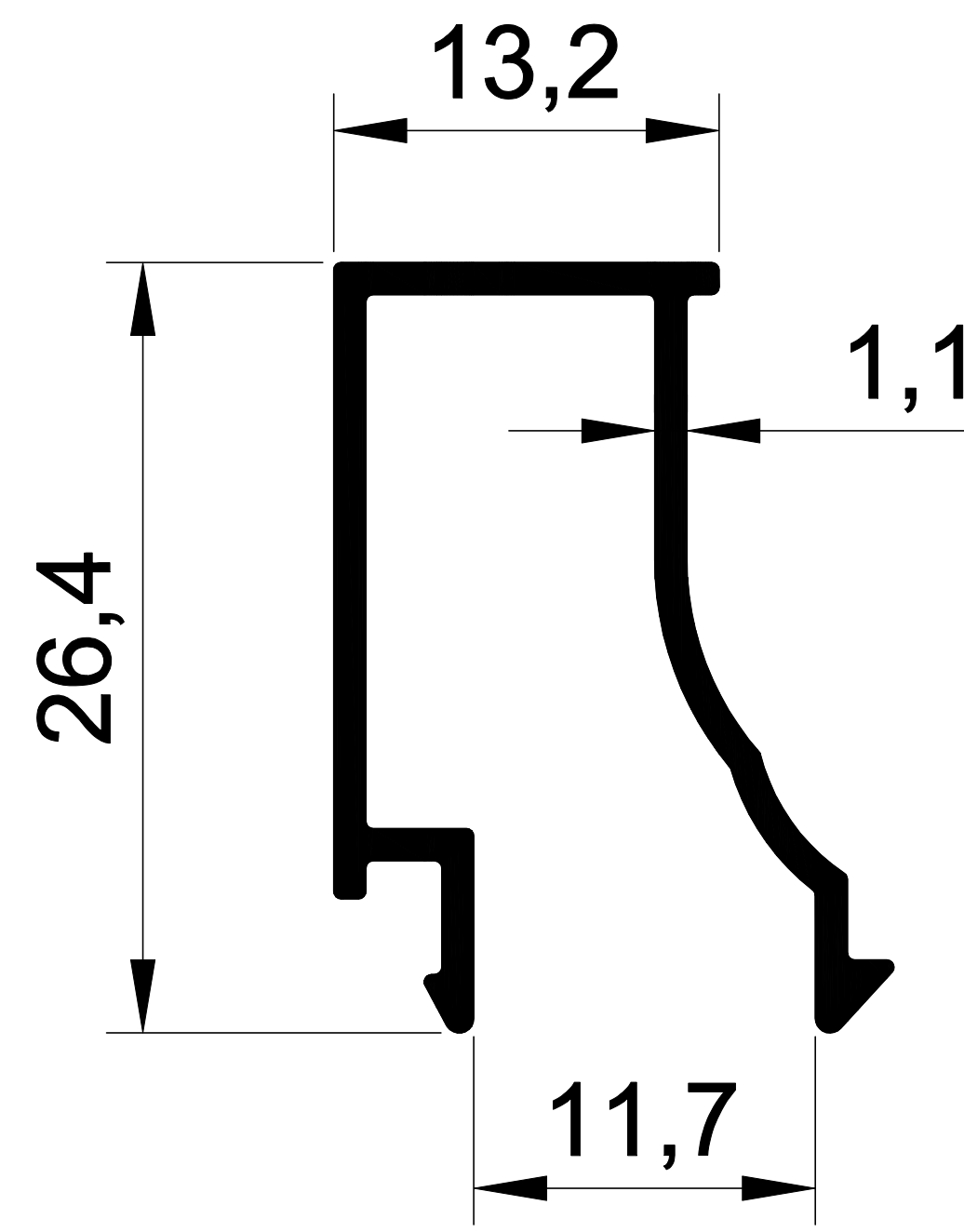
1370 0,216 Kg/m. OVAL ÇİTA
