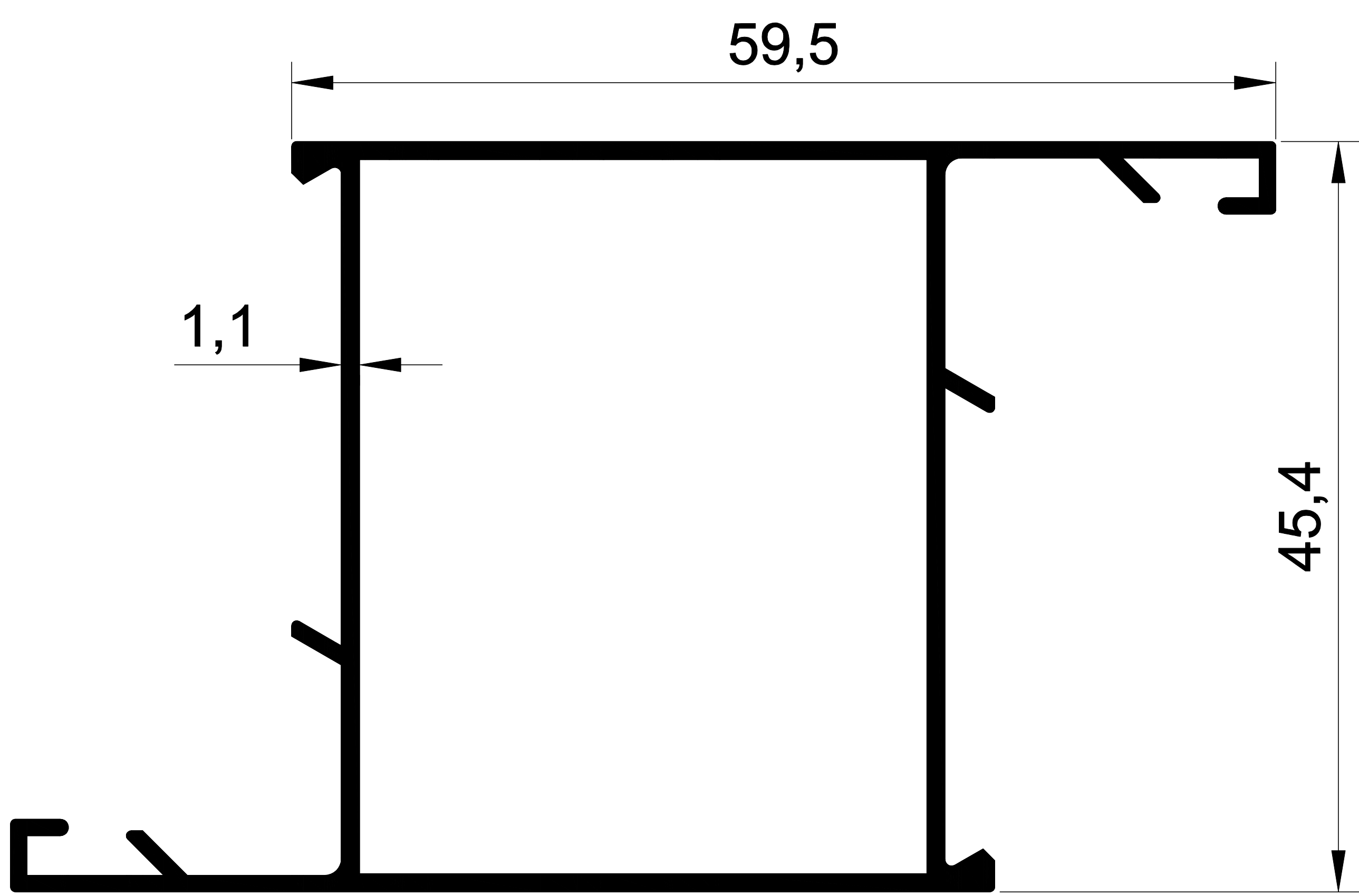
1104 0,645Kg/m. ALDOKS GENİŞ KANAT
