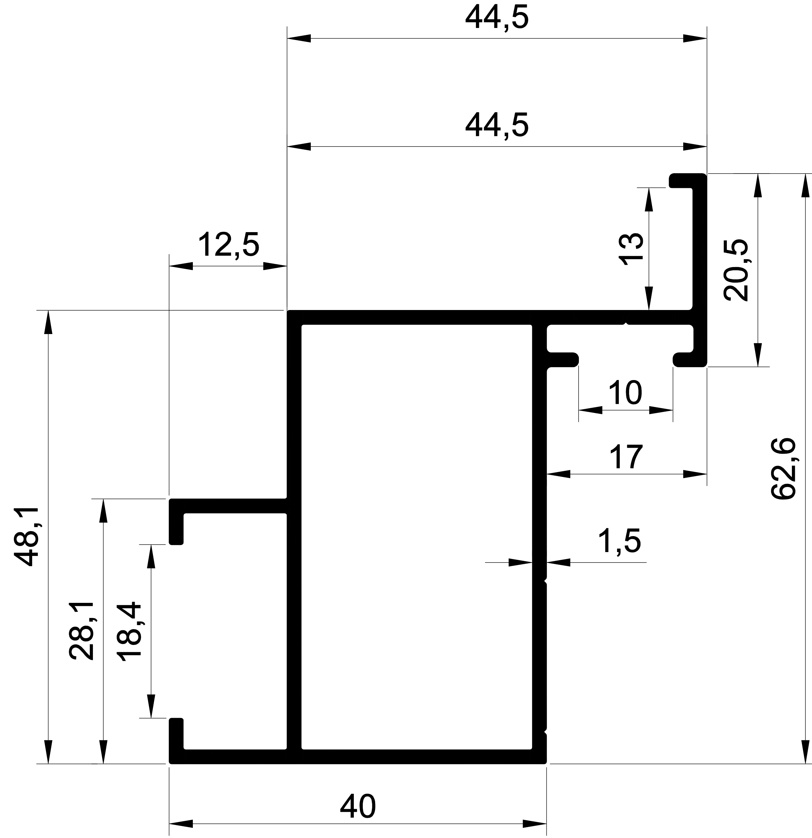
1418 0,897 Kg/m. MS-AHŞAP GİZLİ KAPI KASASI
