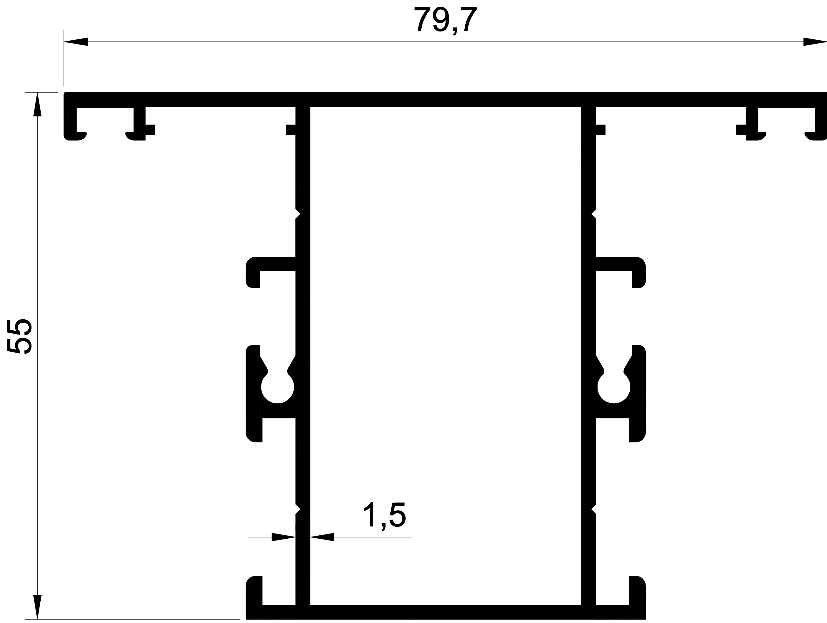
1199 1,195 Kg/m. SİSTEM ORTA
