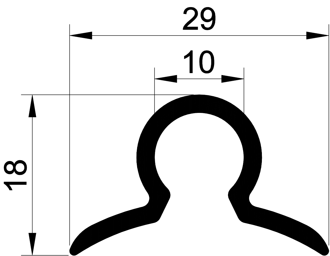
1178 0,282 Kg/m.
