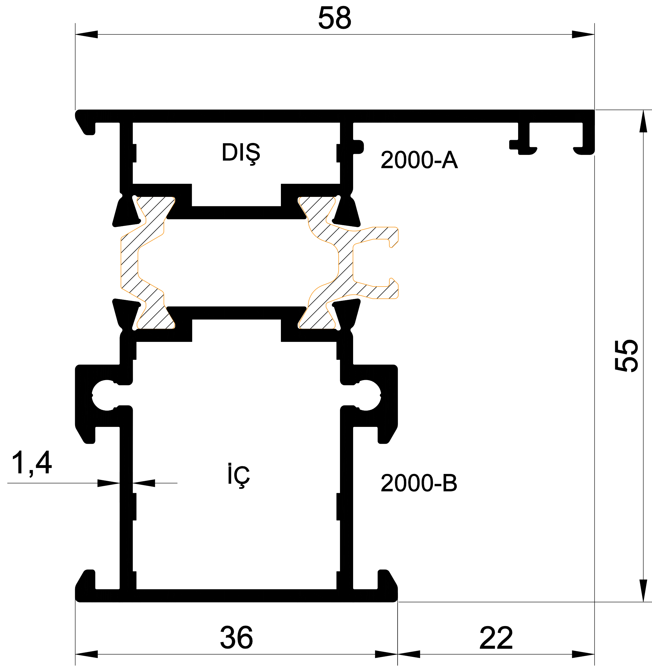
-55- 2000 1,171 Kg/m SİSTEM 55 ISI YALITIM KASA
