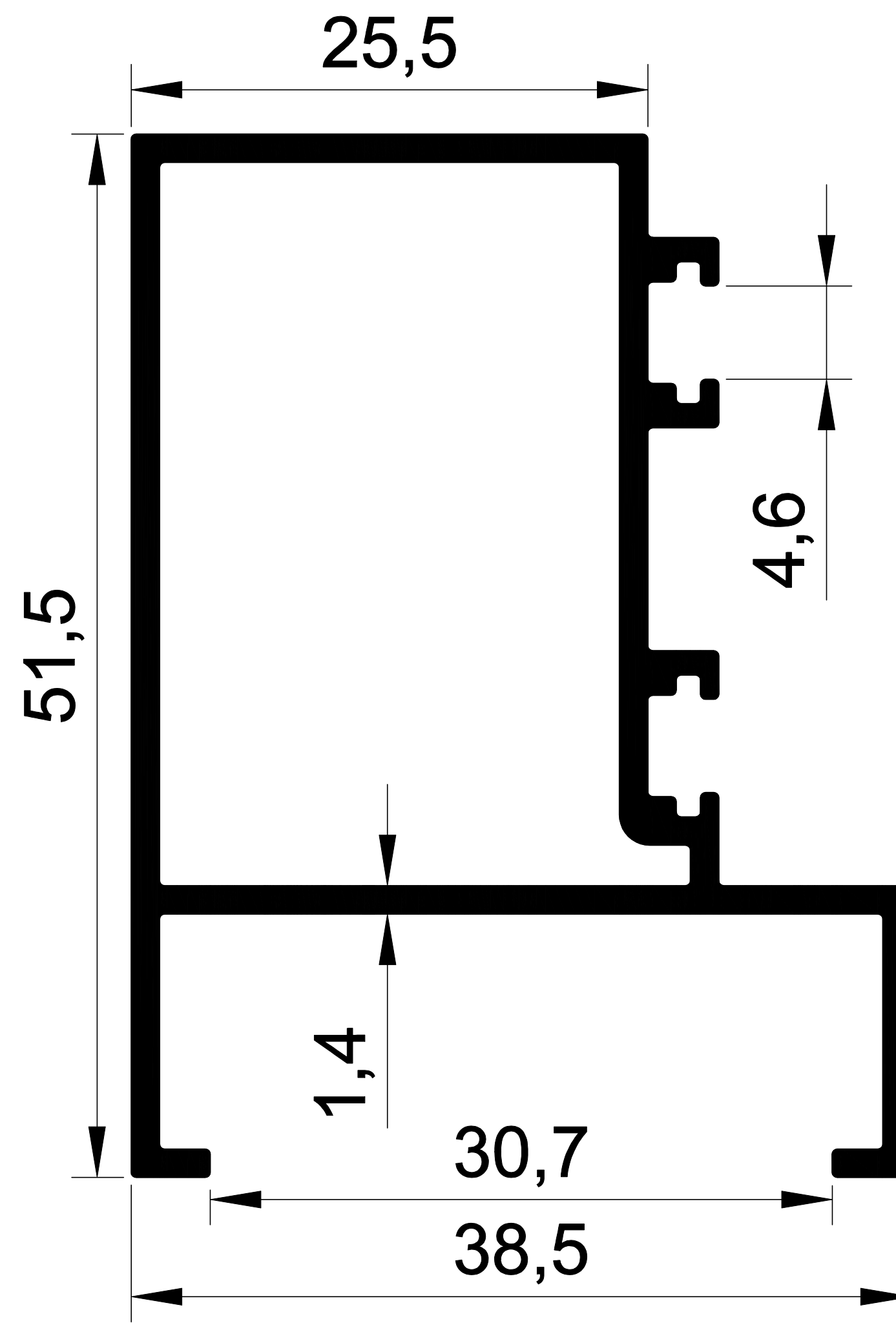
1363 0,704 Kg/m. ISI YALITIM KANAT 90° DÖNÜŞ
