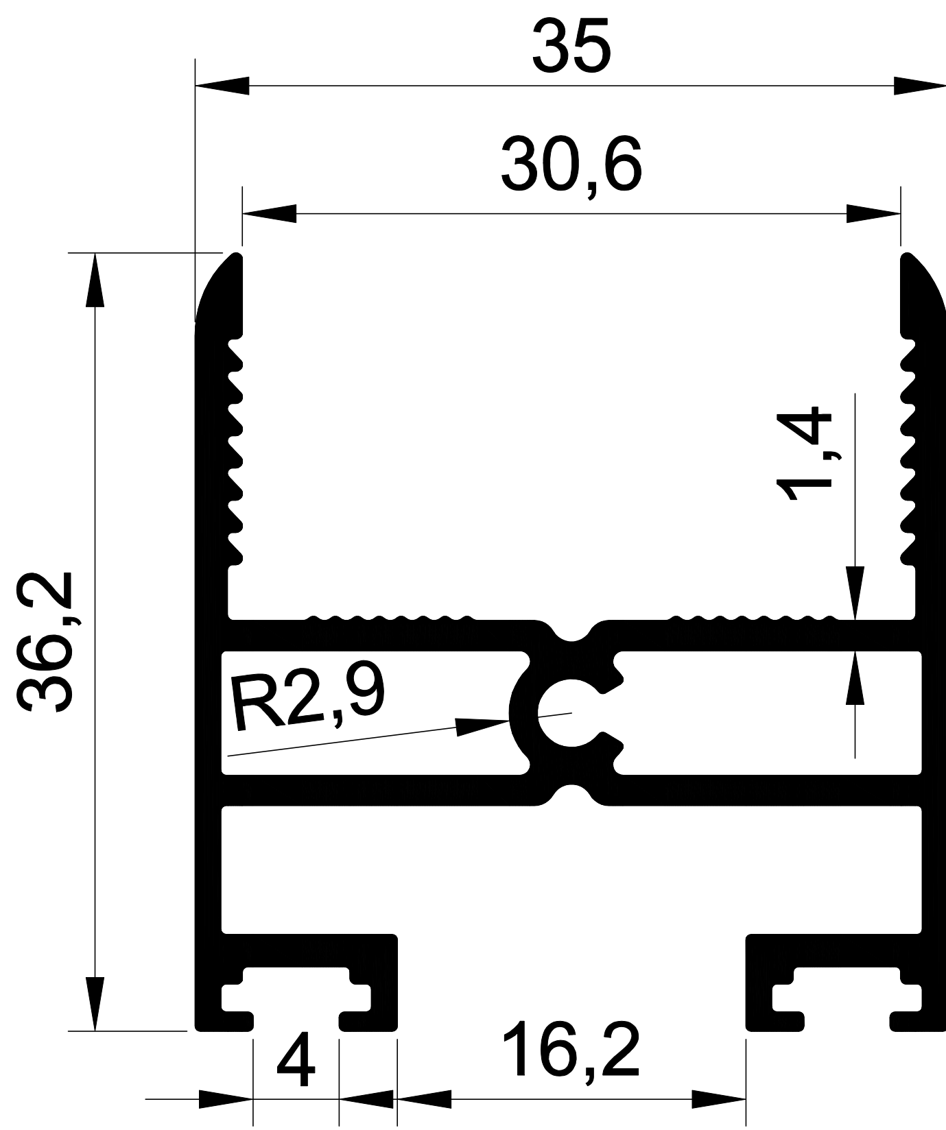
1360 0,686 Kg/m. ISI YALITIM BAZA
