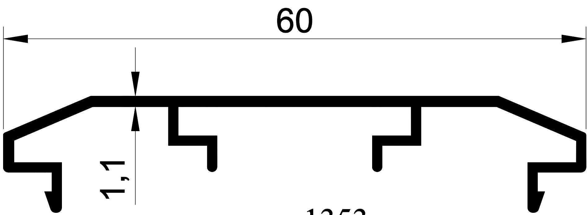
1353 0,310 Kg/m. C-60 ÇARPMA KAPI ADAPTÖRÜ
