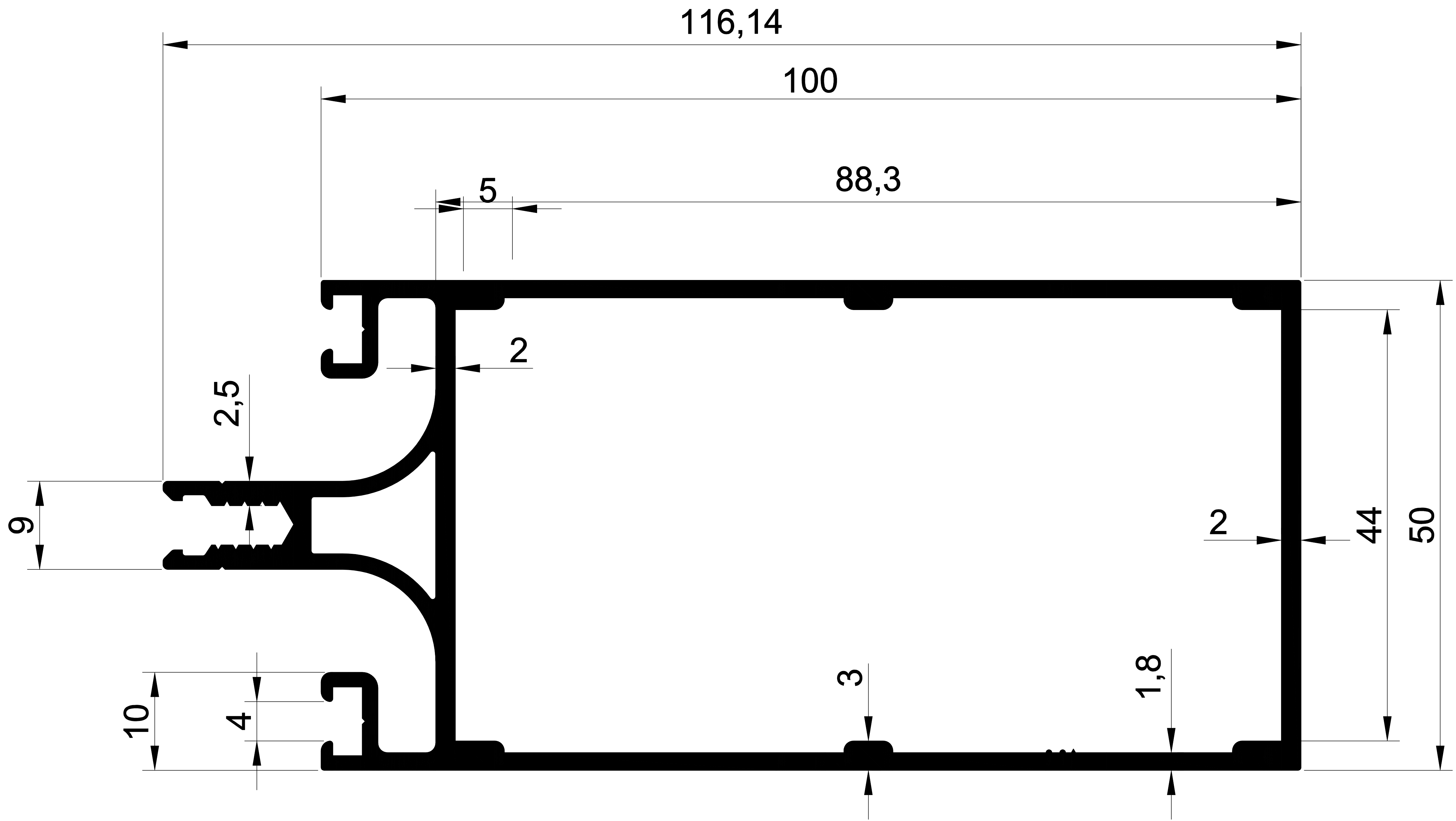
1439 2,024 Kg/m. 110'LİK CEPHE PROFİLİ UZUN GAGA
