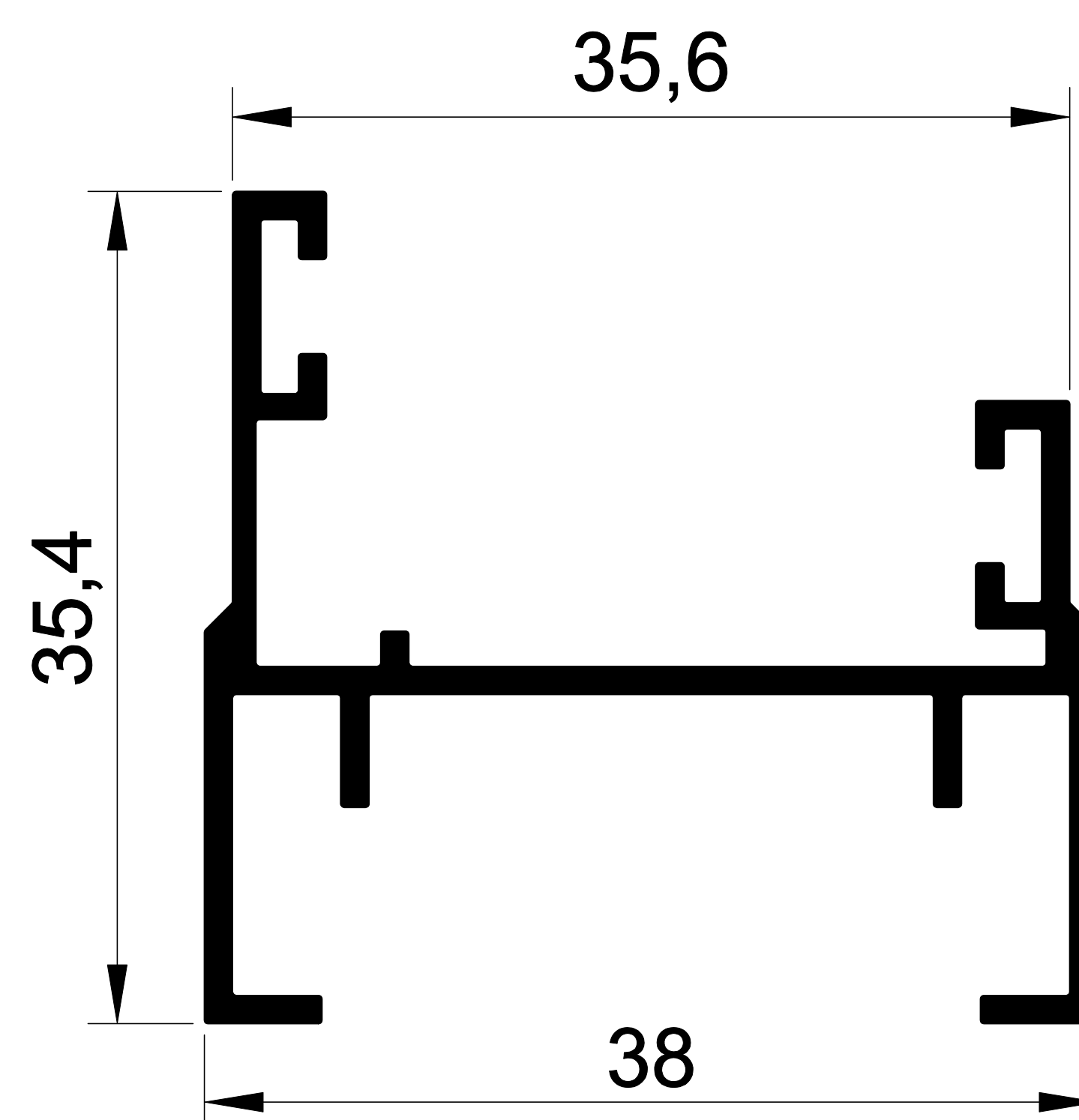
- 2303 0,442 gr/m ISICAMLI CAM BALKON PROFİLLERİ
