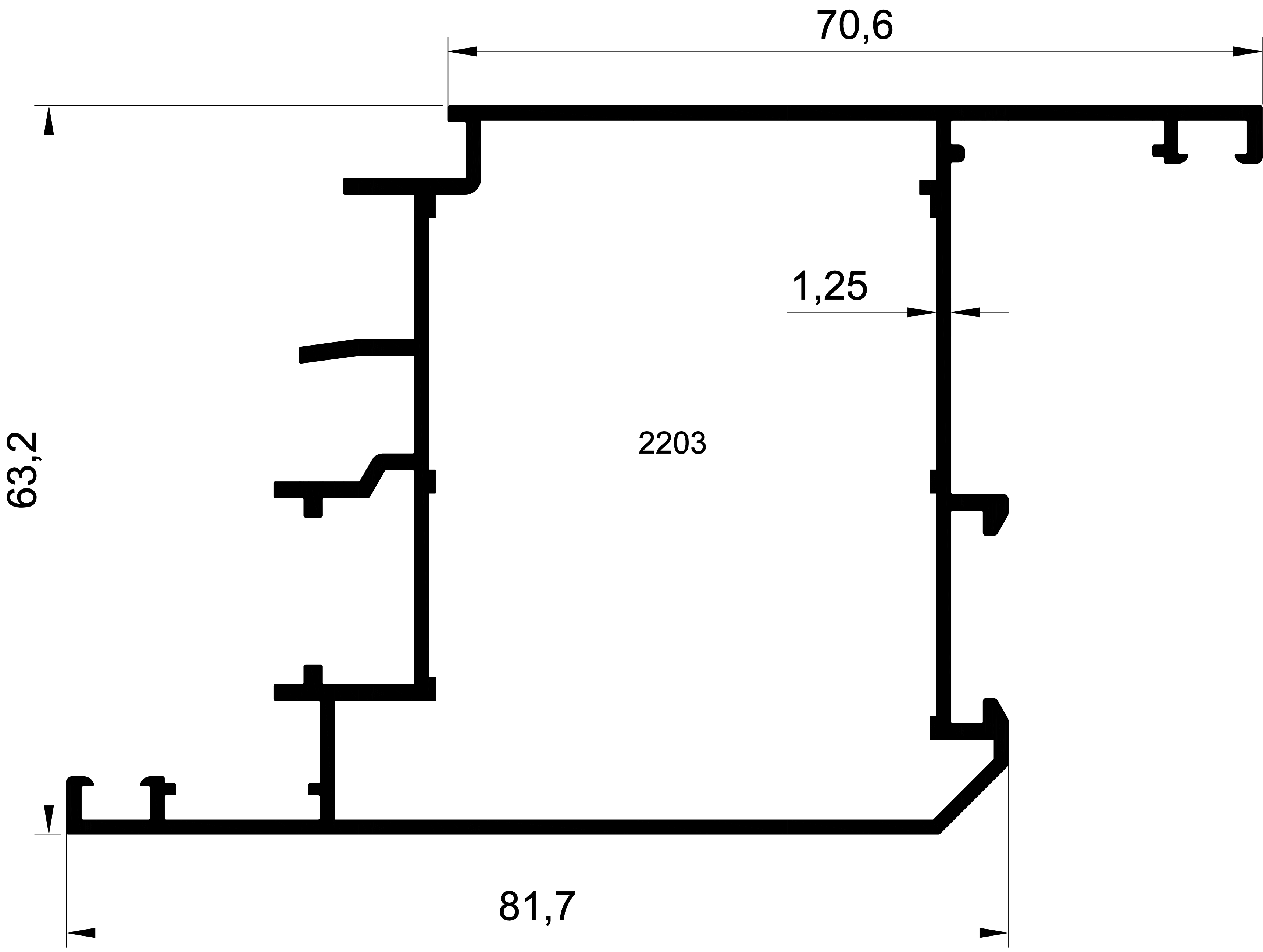
EK-55- 2203 1,257 Kg/m SİSTEM 55 YALITIMSIZ İÇE AÇILIR KAPI
