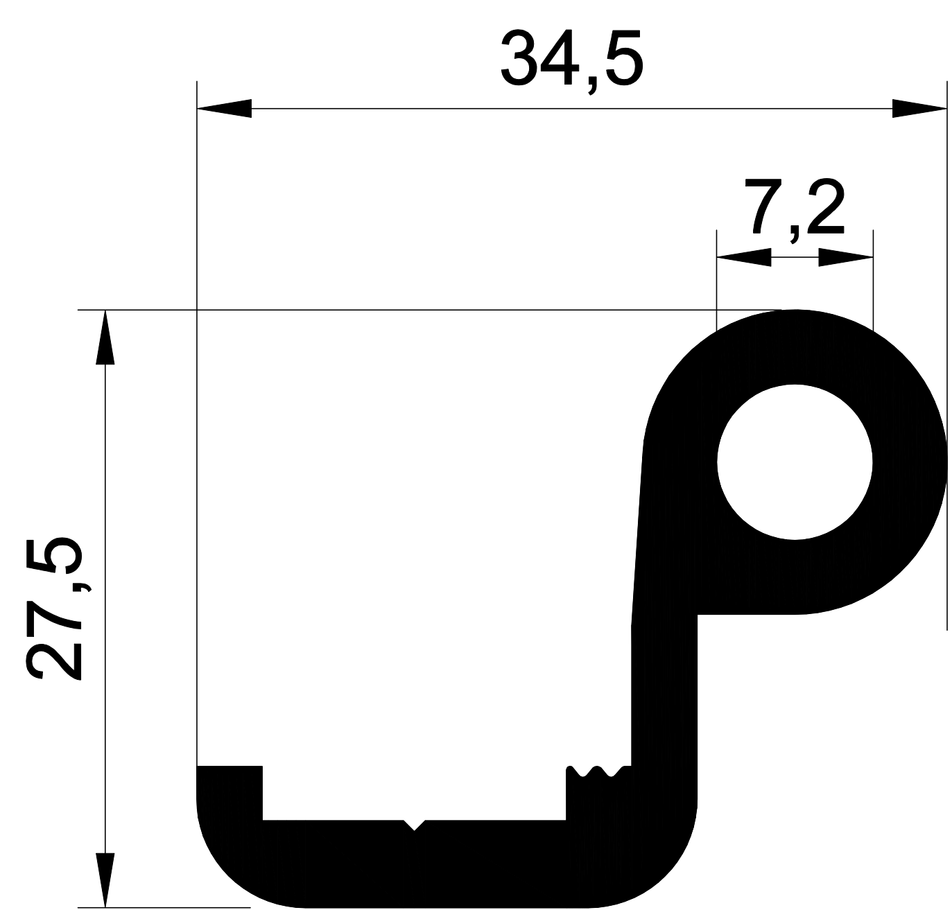
1221 0,544 Kg/m.
