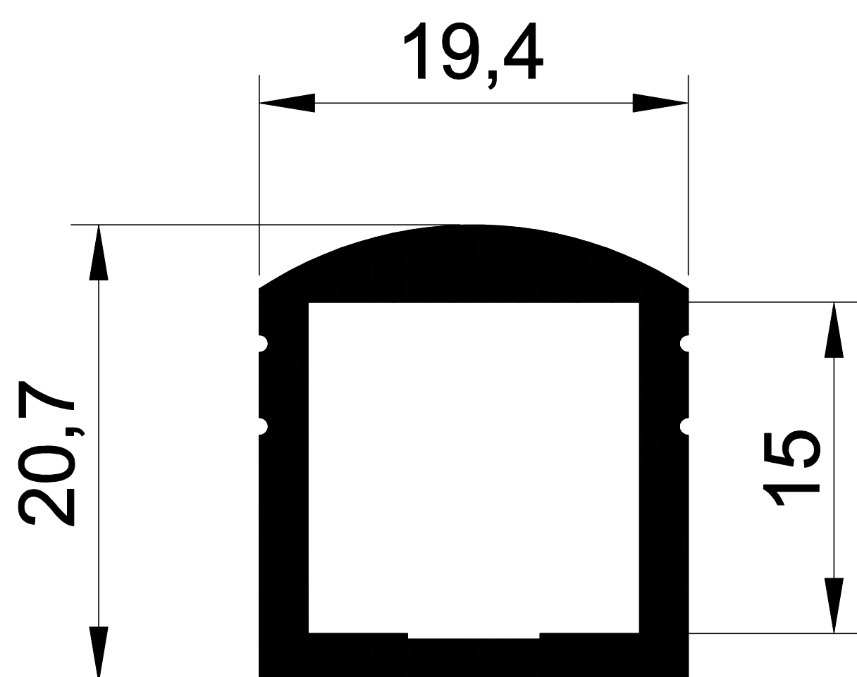
1291 0,423 Kg/m.
