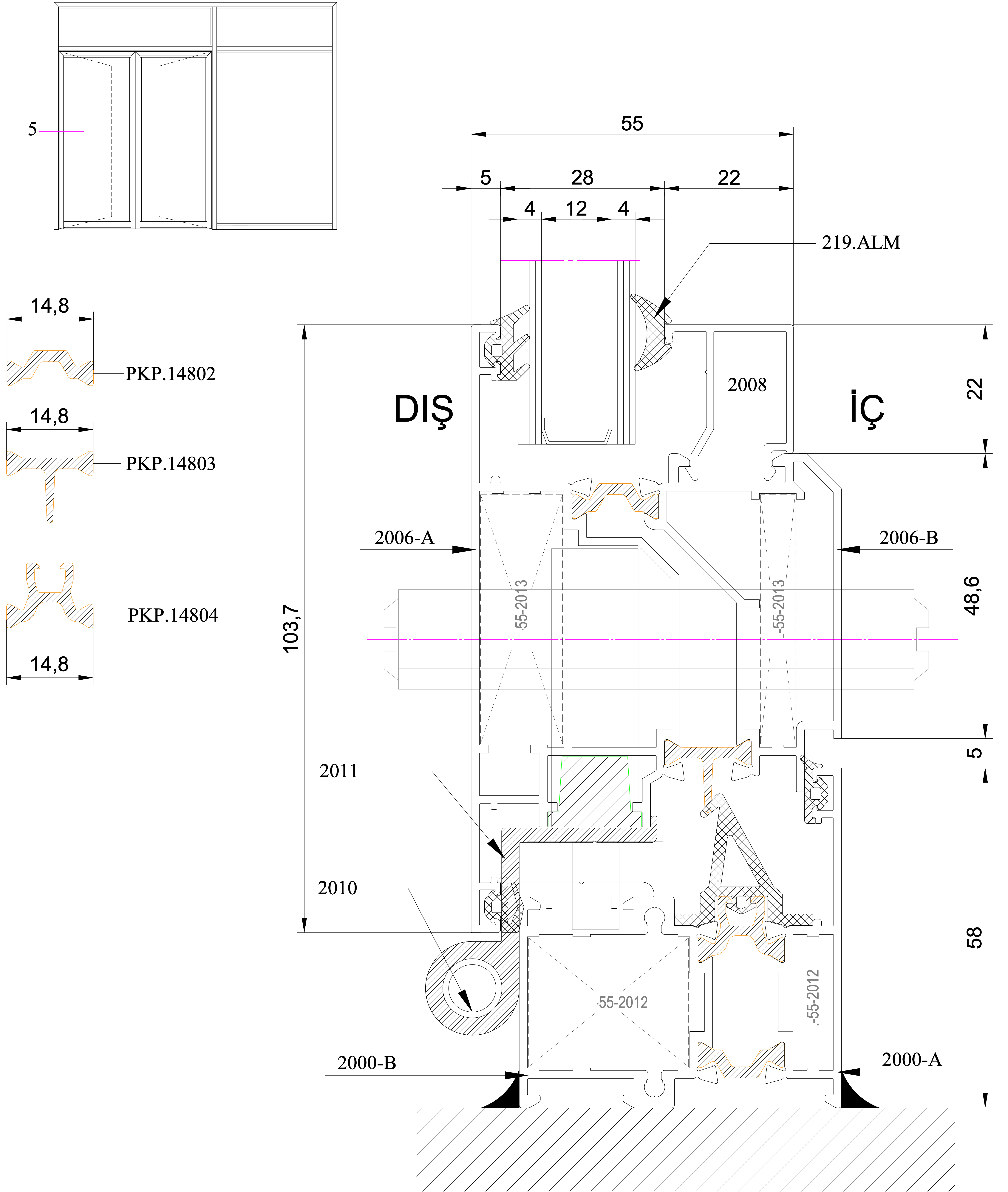
DIŞA AÇILIR ÇİFT KAPI DETAYI
