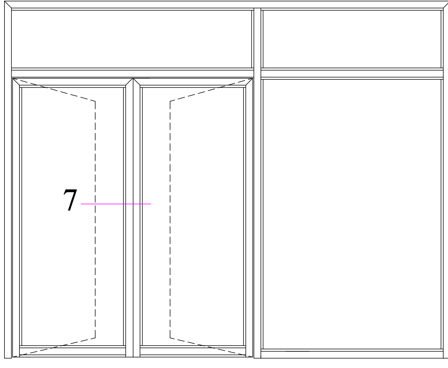
DIŞA AÇILIR ÇİFT KAPI DETAYI
