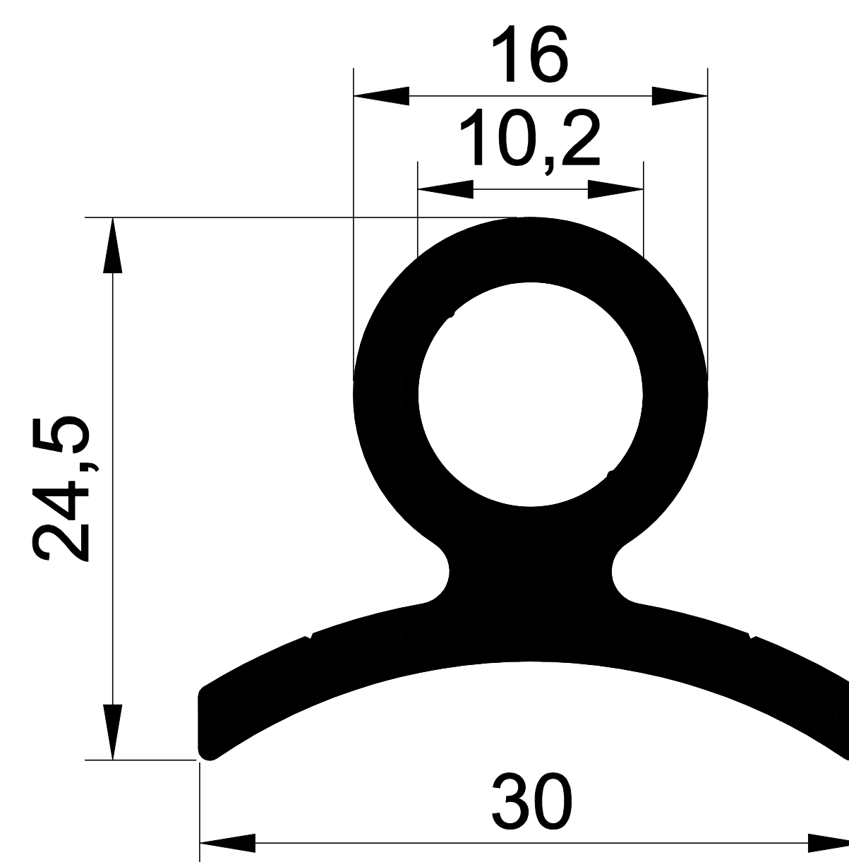
1176 0,612 Kg/m.
