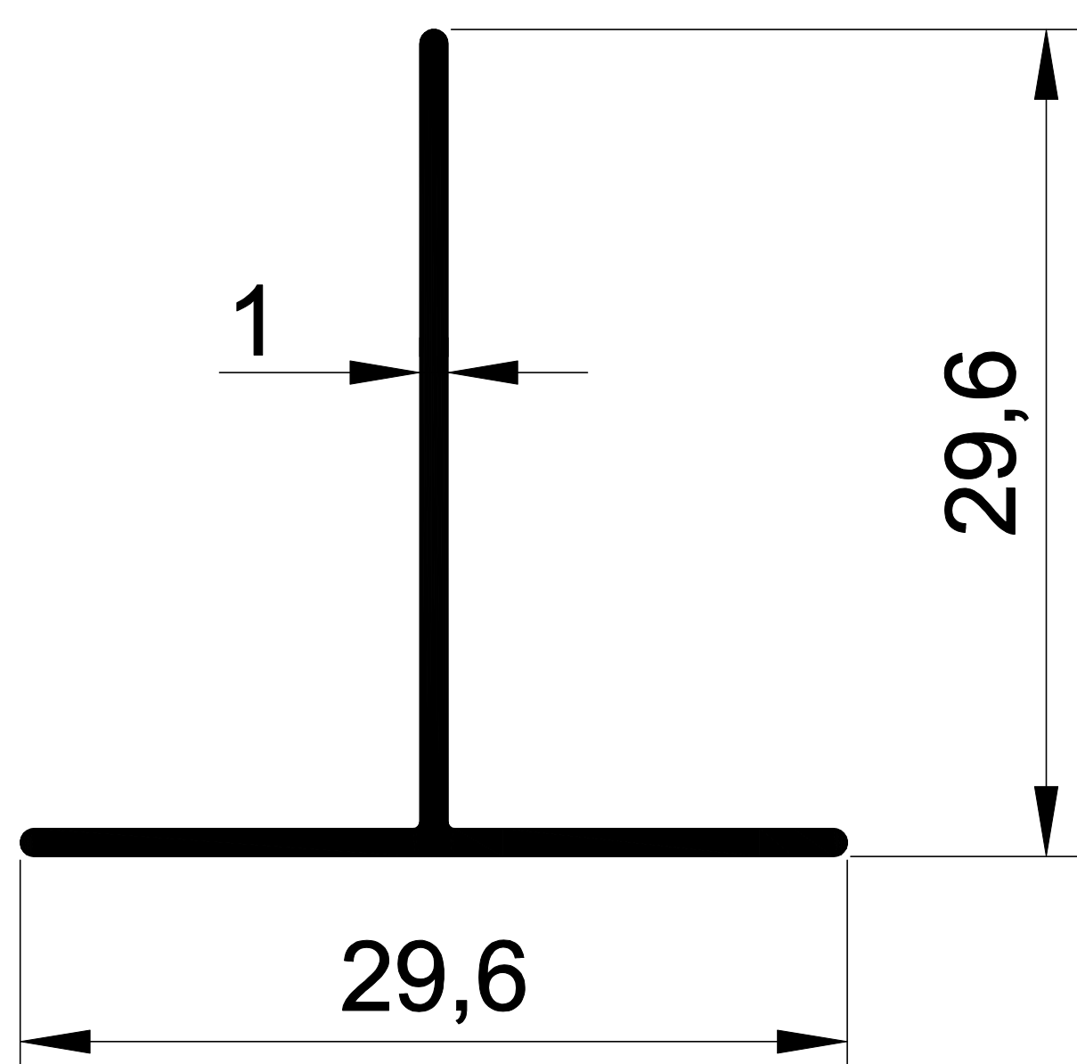
1188 0,157 Kg/m. 30X30 T BİNİ
