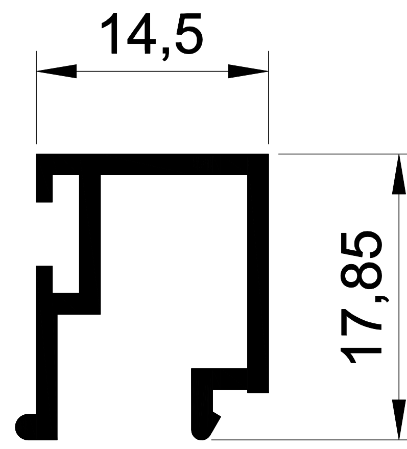
1189 0,206 Kg/m TEK CAM ÇİTASI
