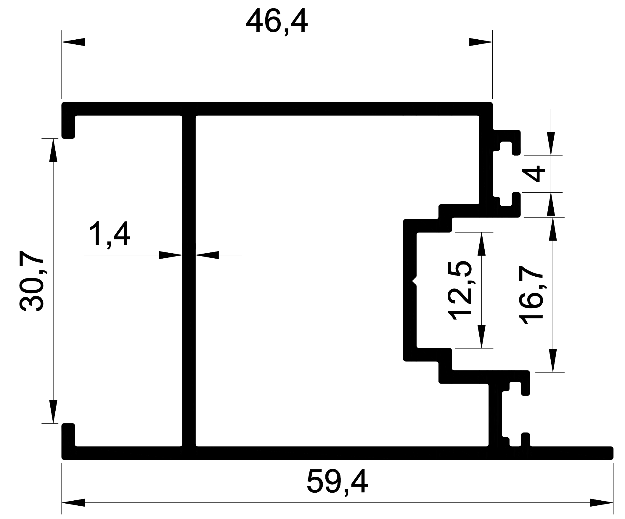
1362 0,809 Kg/m. ISI YALITIM KANAT KİLİTLEME
