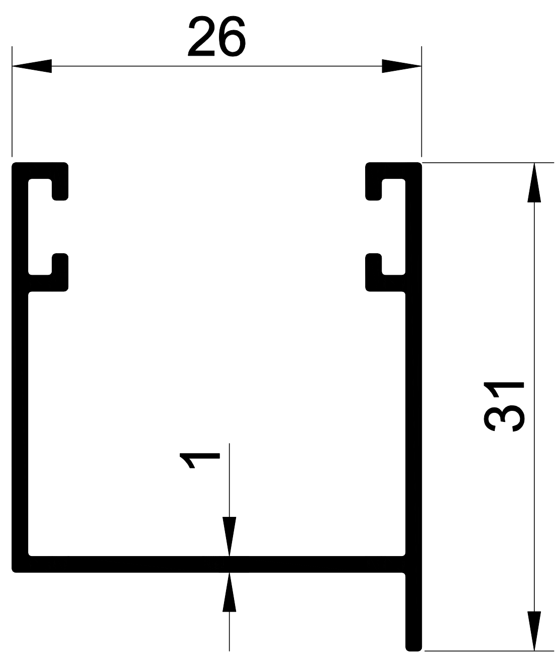
1180 0,263 Kg/m. PANJUR FİTİLLİ U
