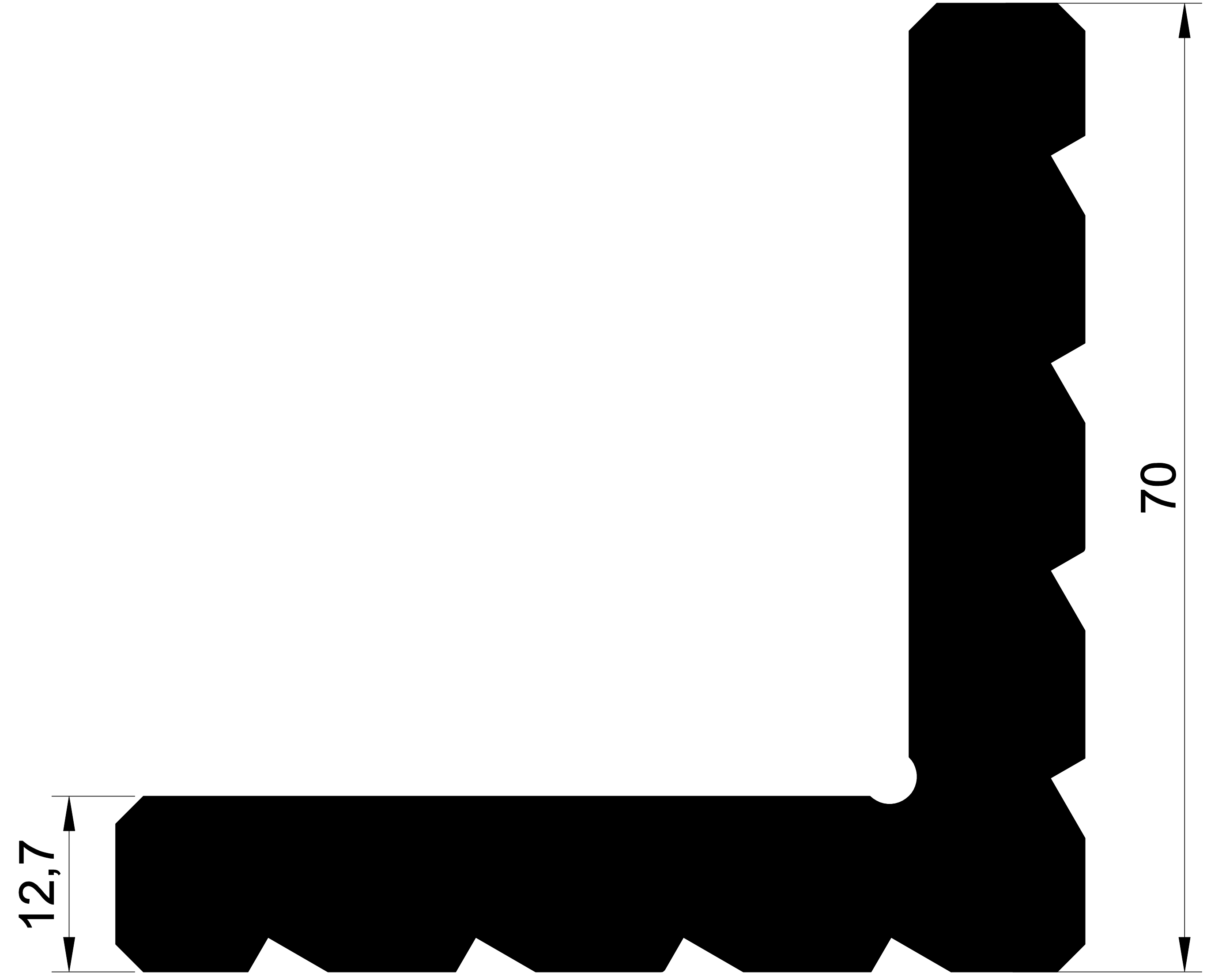
1400 4,192 Kg/m. 13 MM CEPHE KÖŞE
