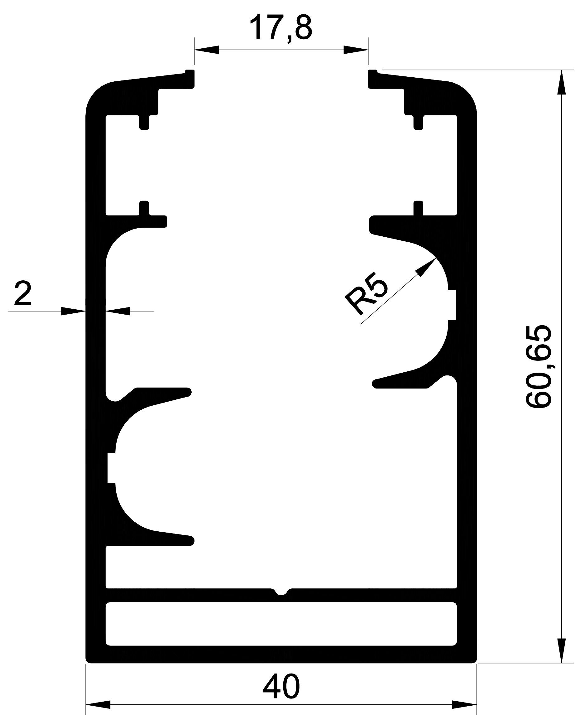
1212 1,371 Kg/m. FIRTINA KASA
