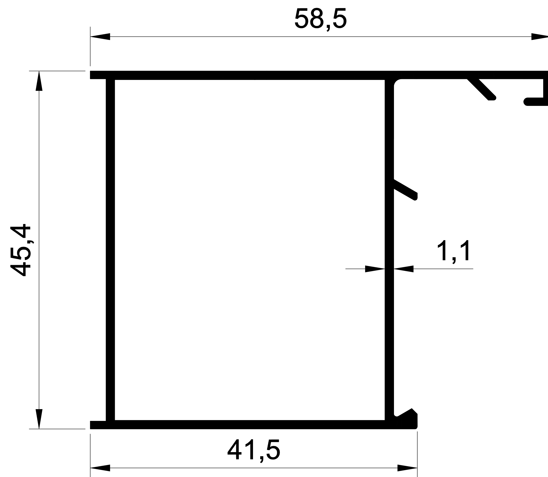
1106 0,550 Kg/m. ALDOKS GENİŞ KASA
