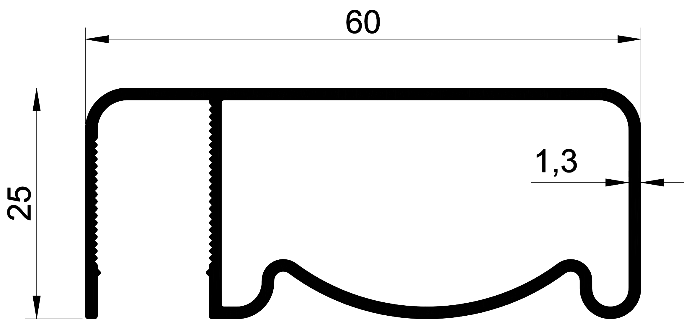
1134 0,622 Kg/m. 25X60 YANDAN CAMLI
