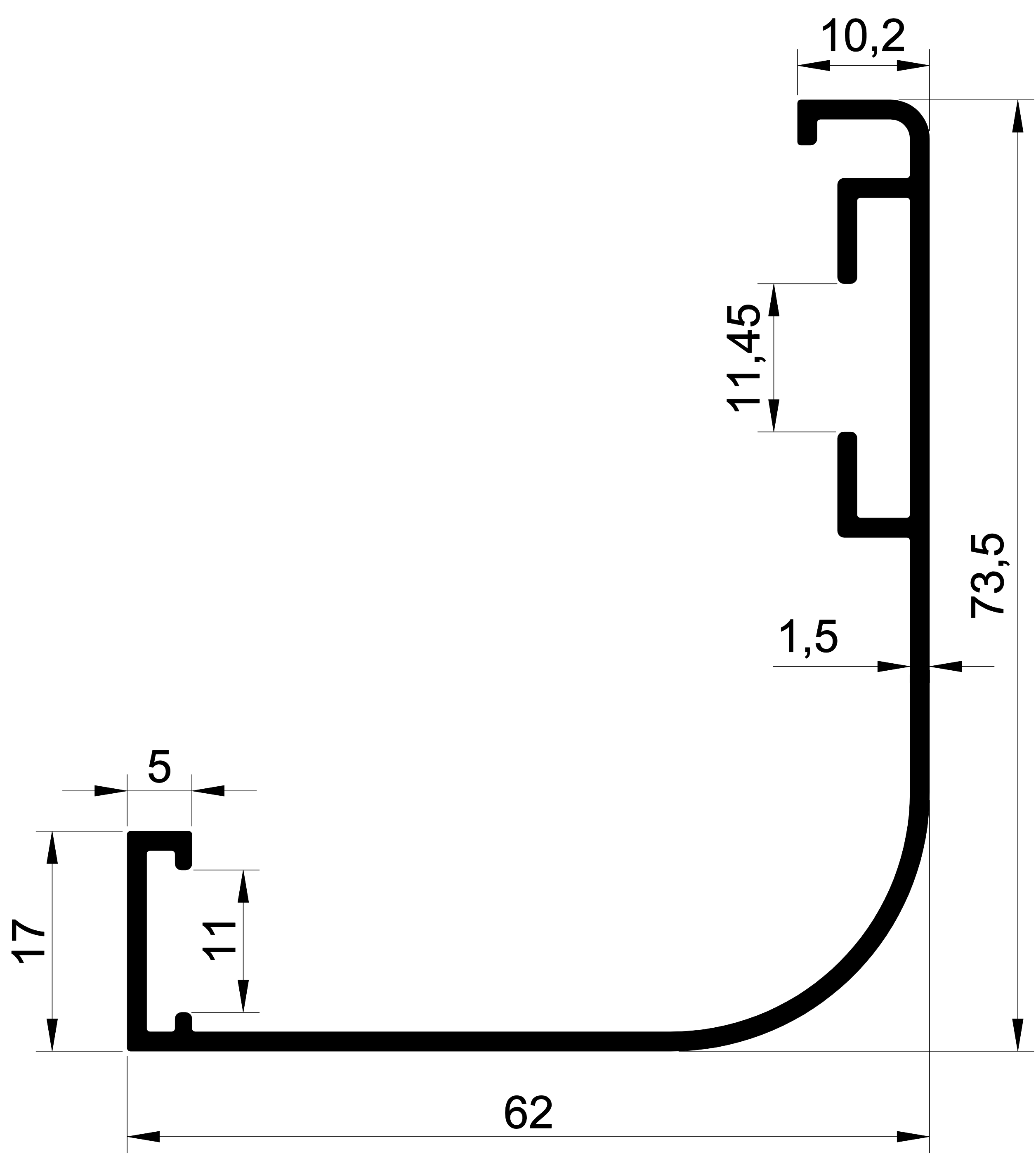
1422 0,737 Kg/m. MS-62'LİK PEERVAZ
