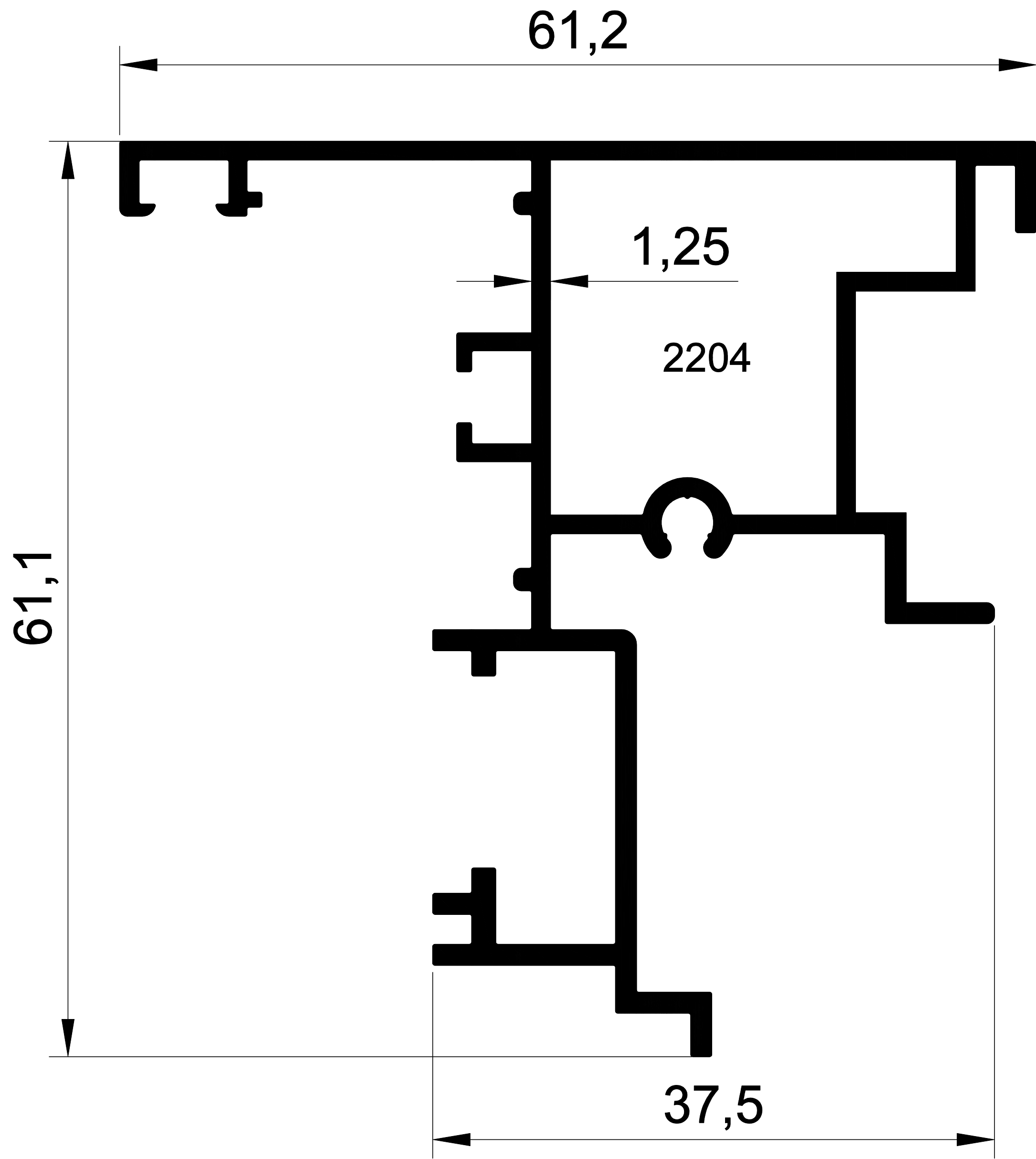
EK-55- 2204 0,932 Kg/m SİSTEM 55 YALITIMSIZ ÇİFT KANAT ADAPTÖR
