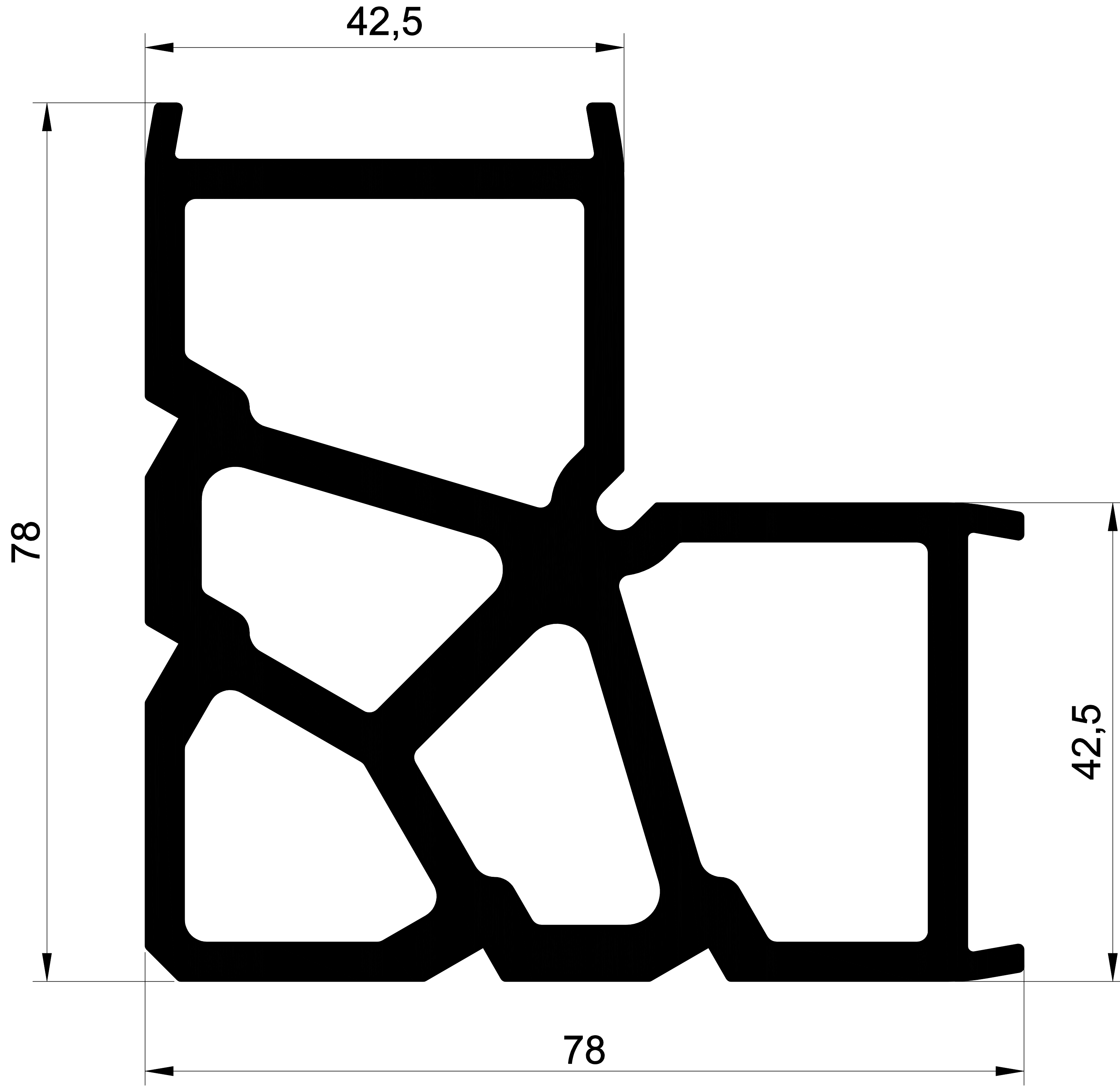
-55- 2013 4,600 Kg/m SİSTEM 55 KÖŞE TAKOZU
