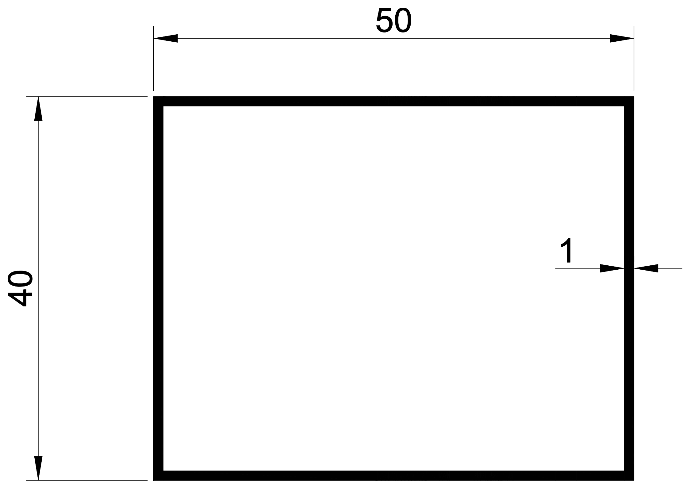
1093 0,454 Kg/m. 40*50 KUTU
