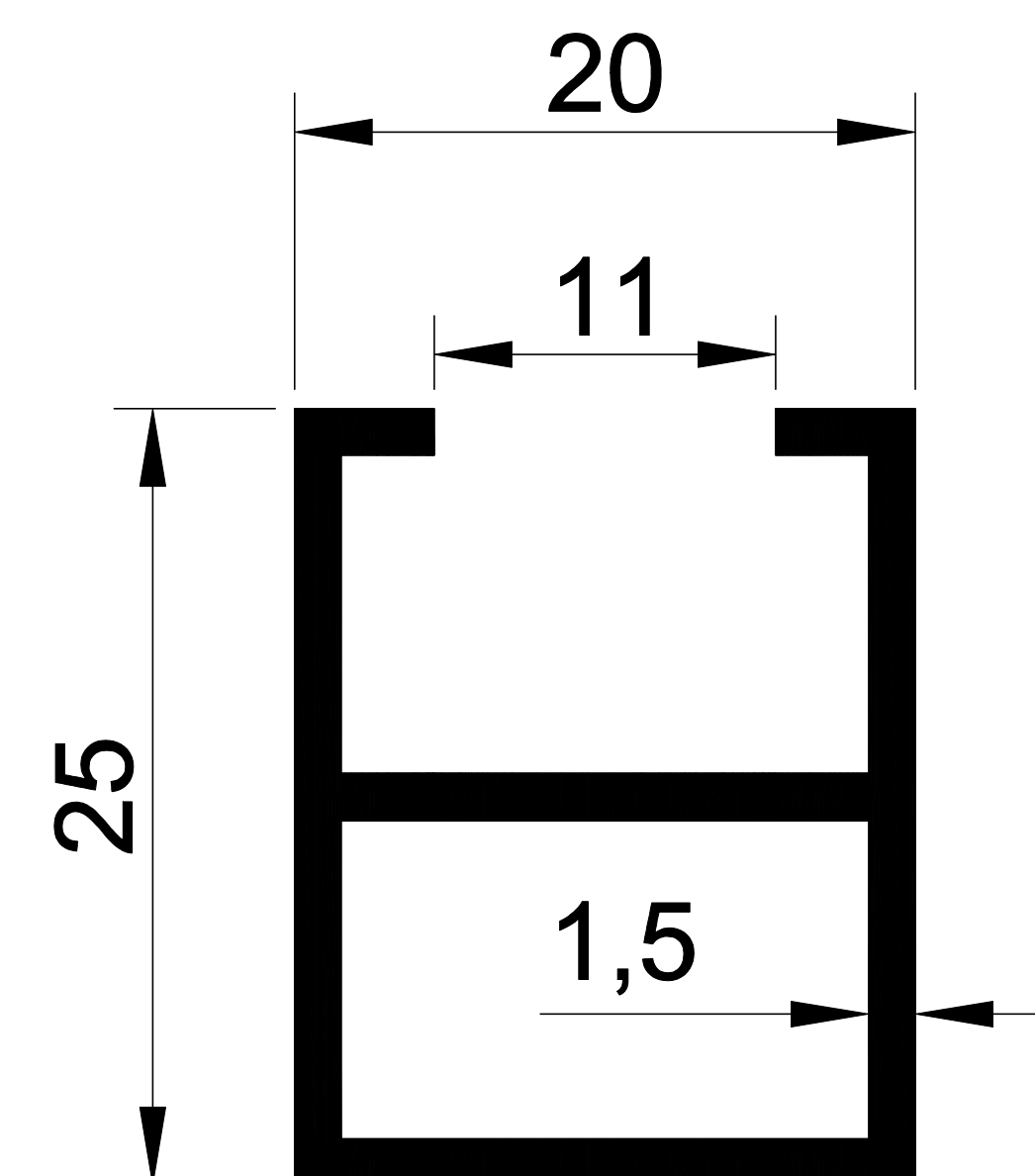
1141 0,366 Kg/m. MİNİ GEMİCİ
