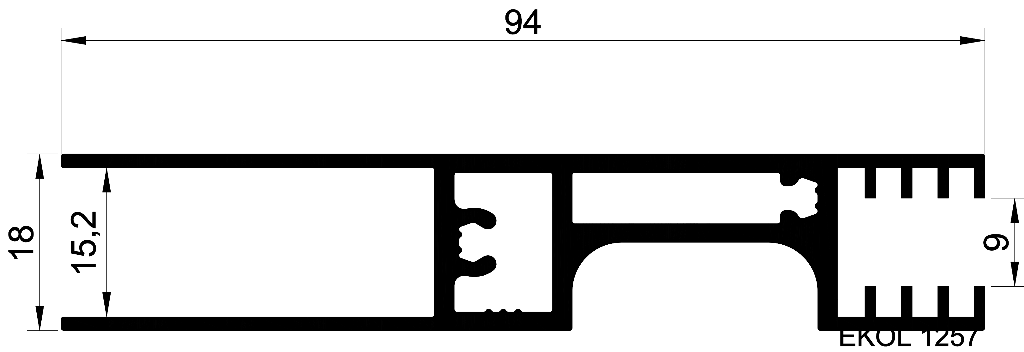
1167 1,225 Kg/m. SÜRME ALT KANAT
