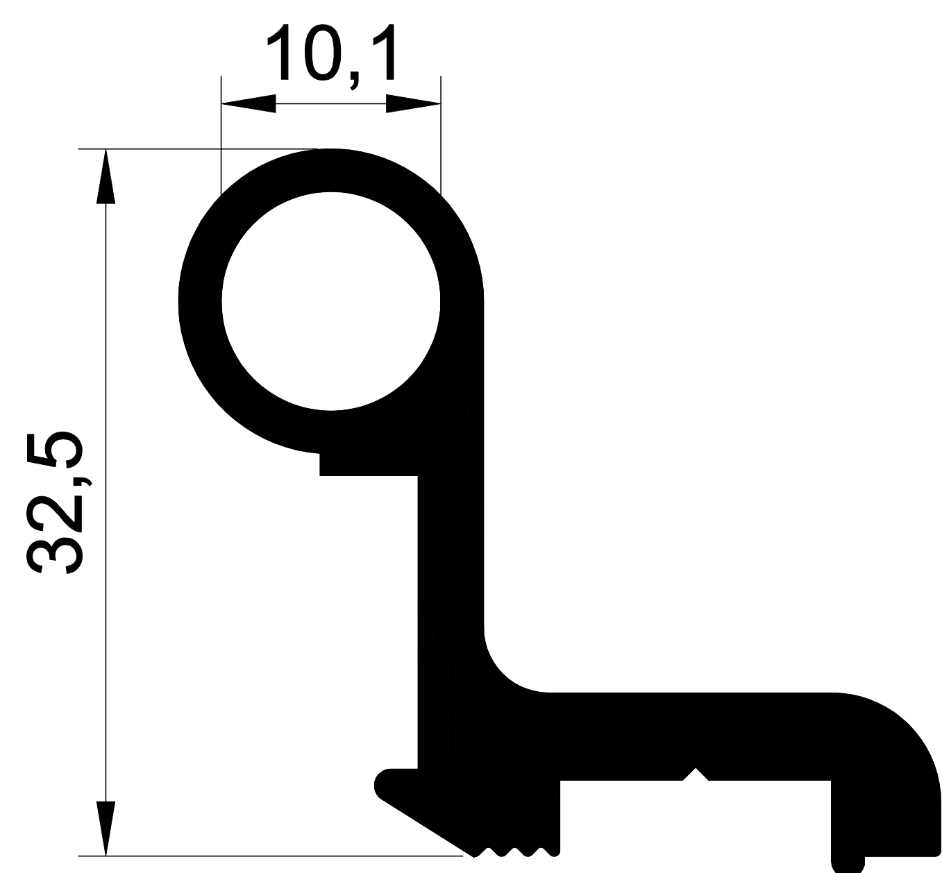
1241 0,694 Kg/m.
