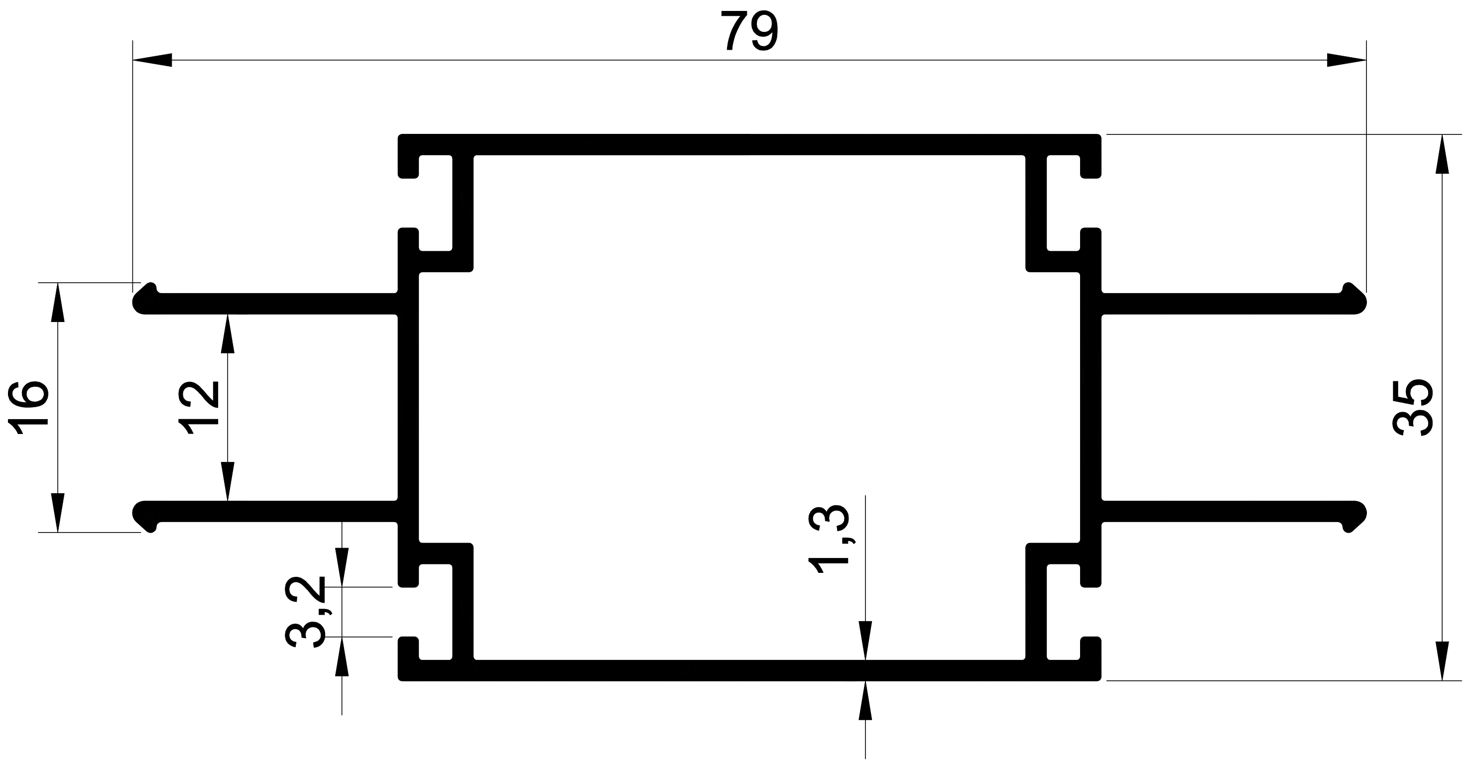
1414 0,882 Kg/m. JALUZİ OFİS BÖLME KASA
