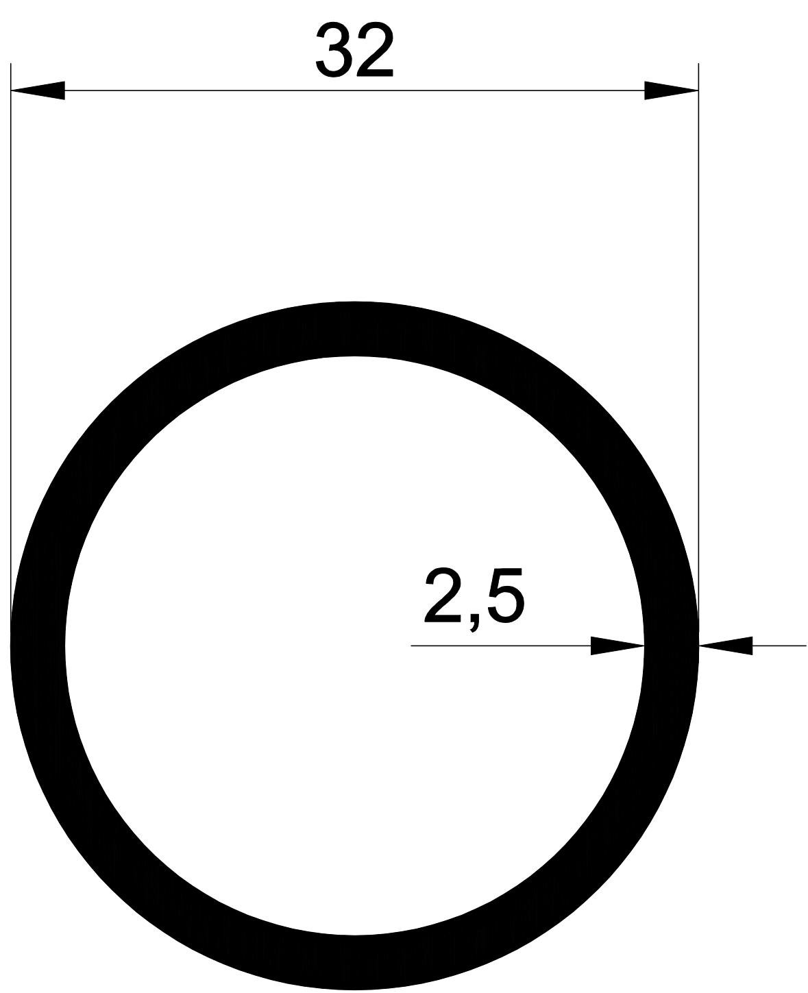
1459 0,627 Kg/m
