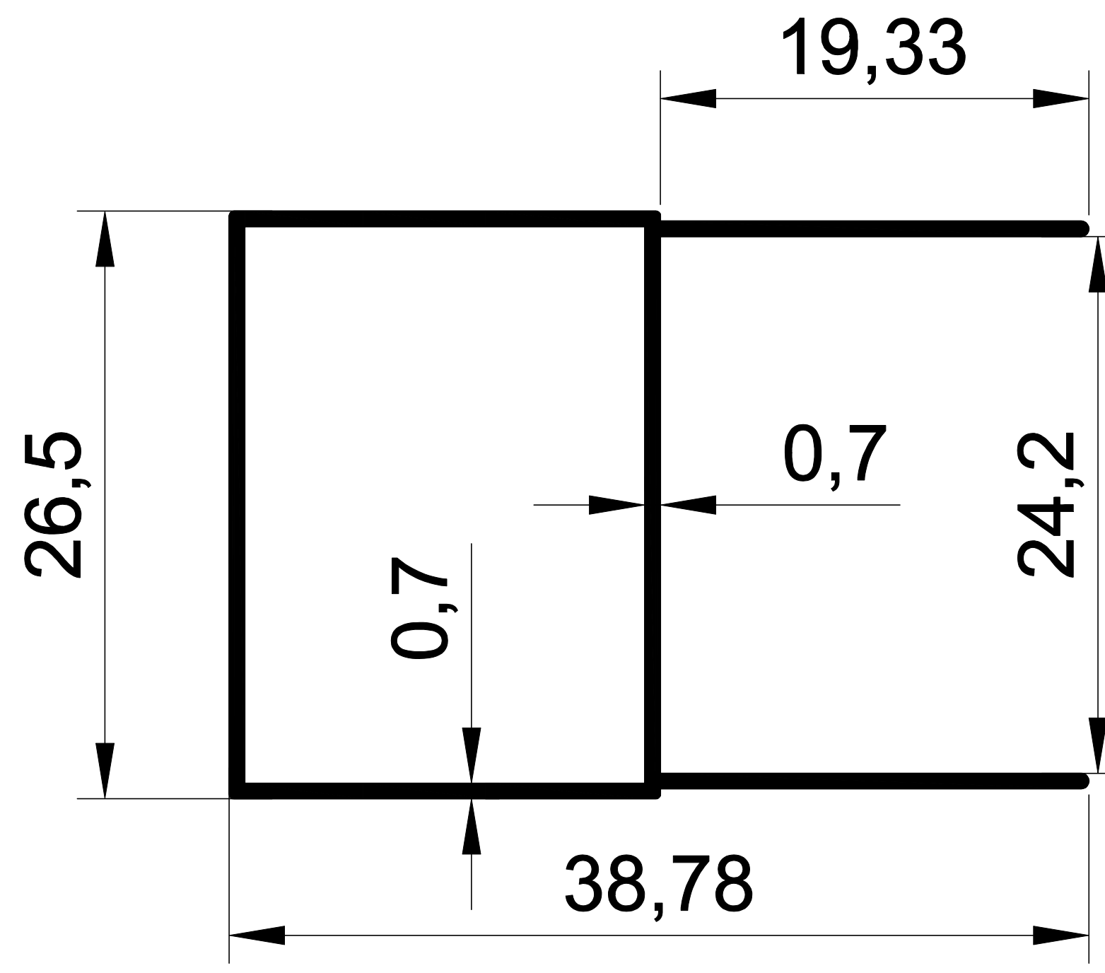
1325 0,243 Kg/m. MAVİ AY SİNEKLİK KASA
