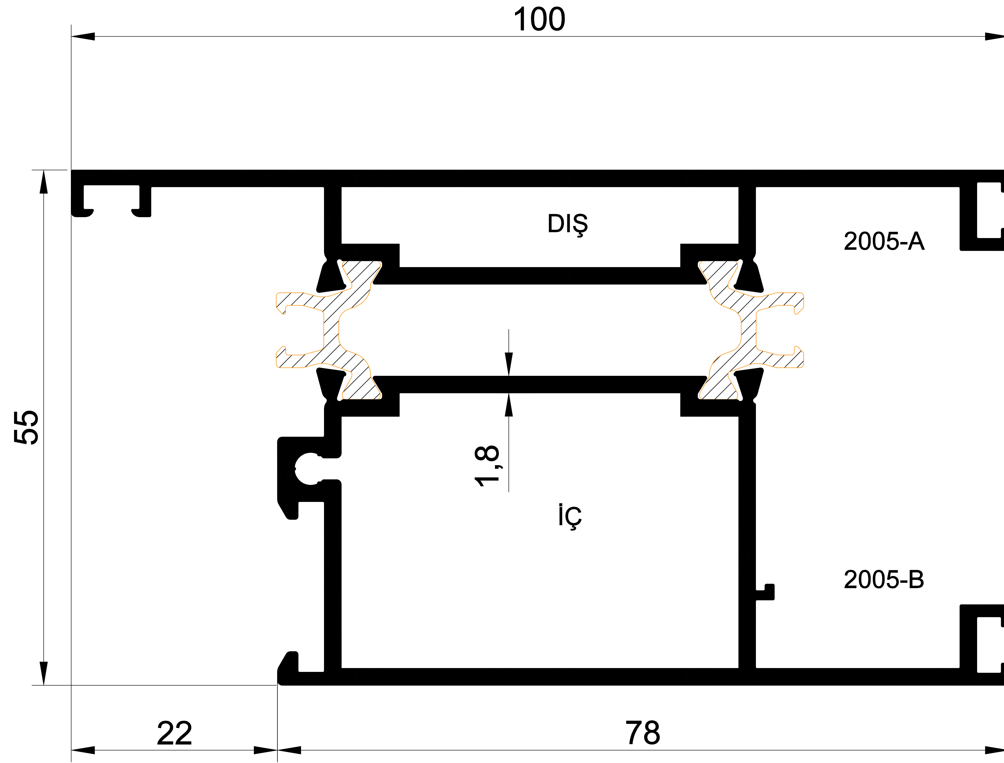
-55- 2005 1,964 Kg/m SİSTEM 55 ISI YALITIM ETEK
