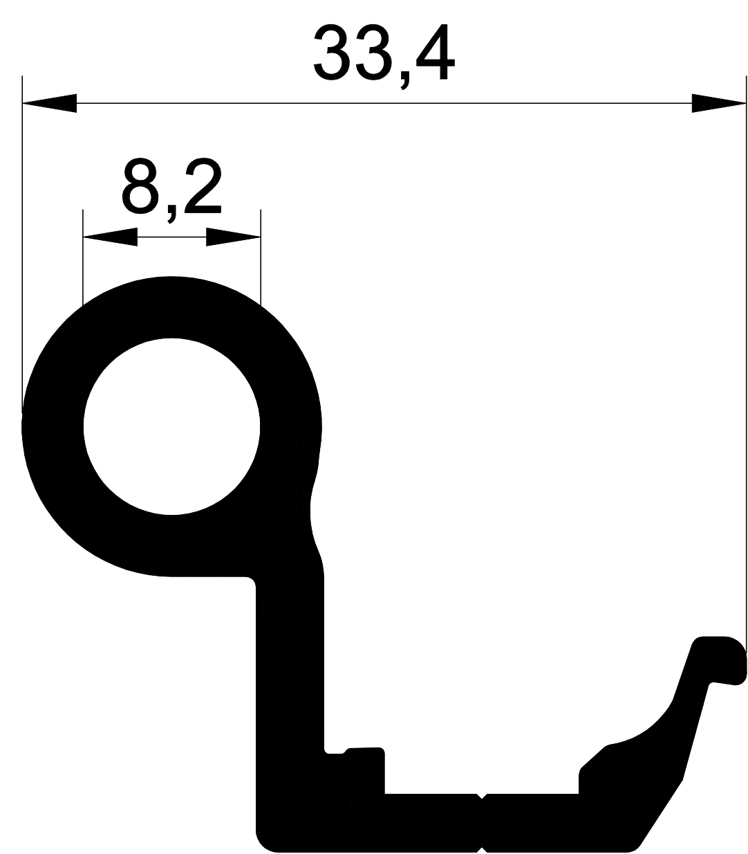
1255 0,575 Kg/m.
