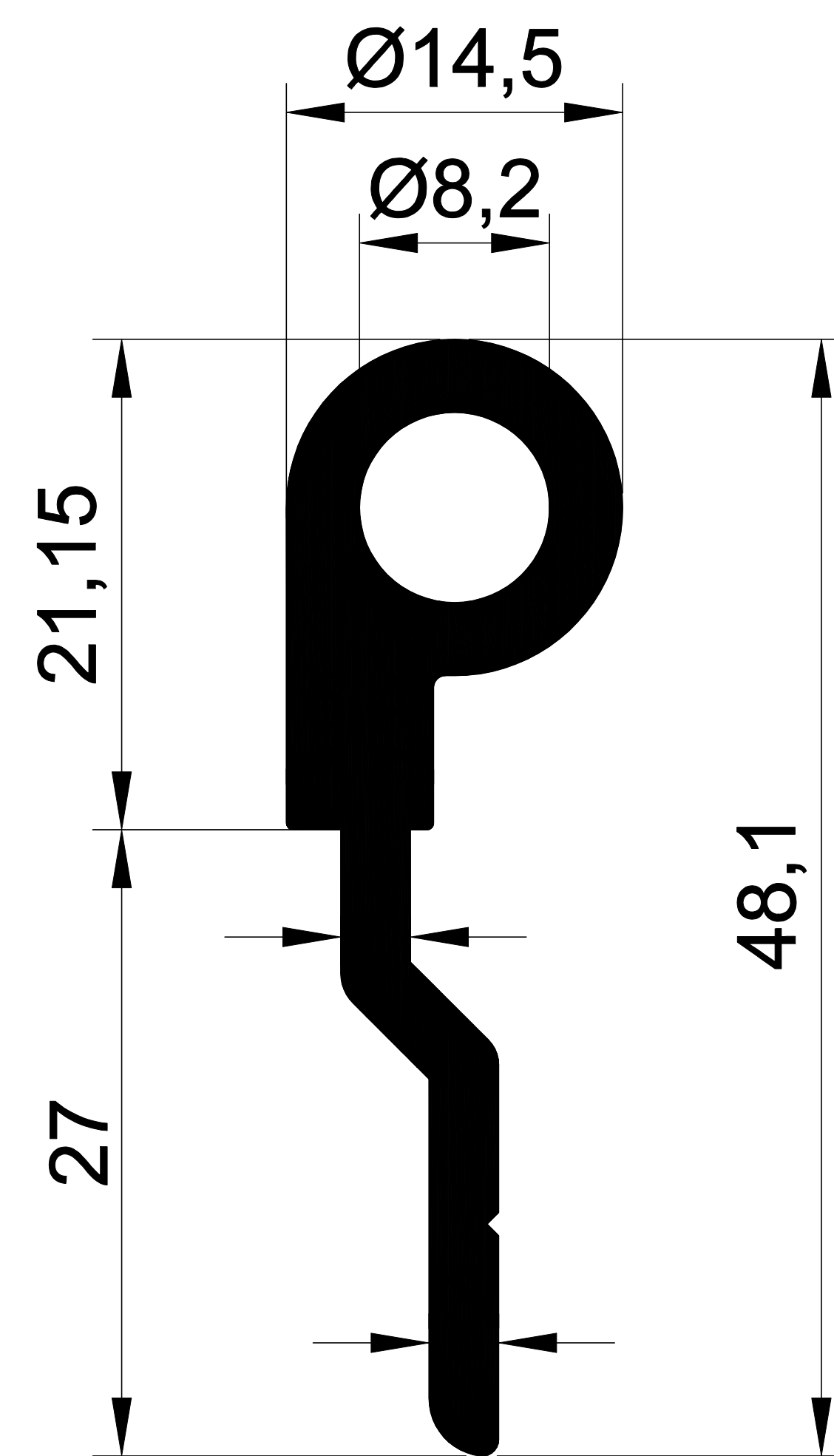
1007 0,713 Kg/m.
