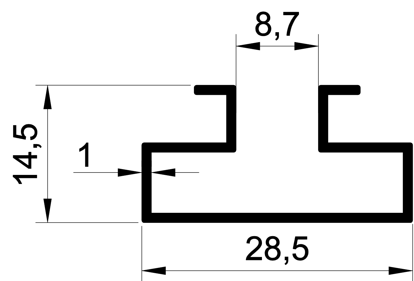
1154 0,217 Kg/m. RAF ASKILIK PROFİLİ
