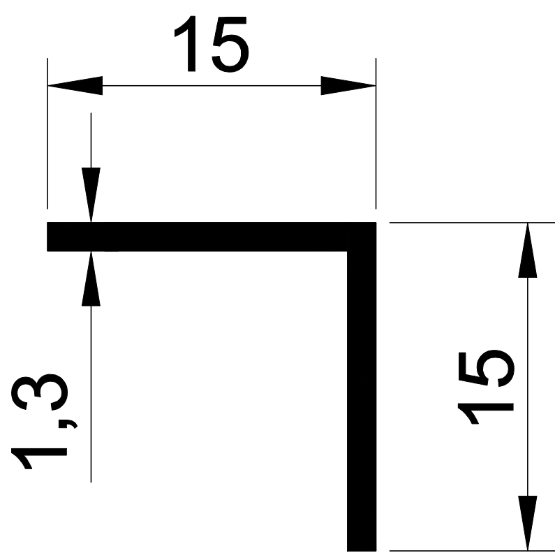
1257 0,100 Kg/m.
