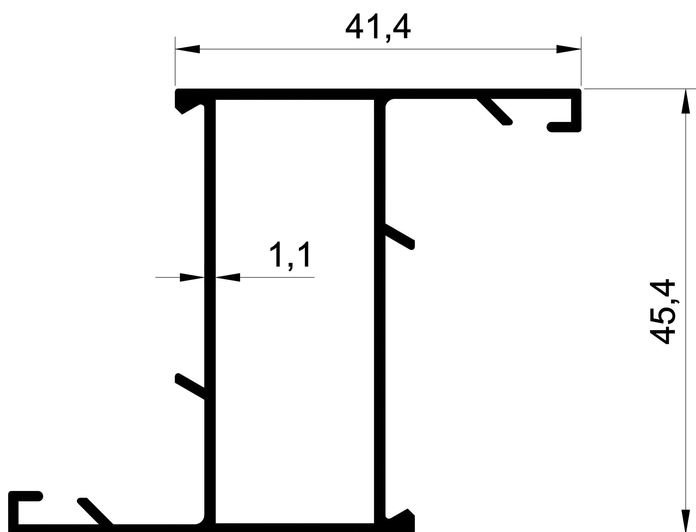
1101 0,547 Kg/m. ALDOKS DAR KANAT
