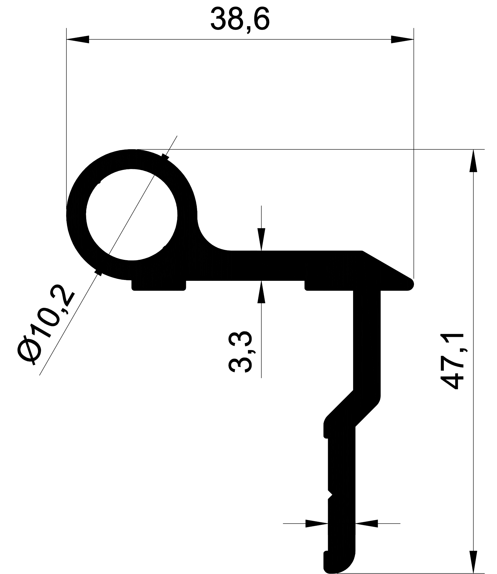
1008 0,775 Kg/m.
