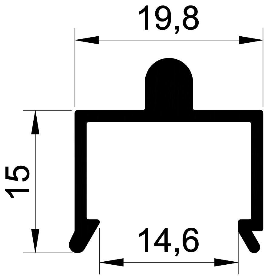
1376 0,234 Kg/m. 100'LÜK TUBA RAY
