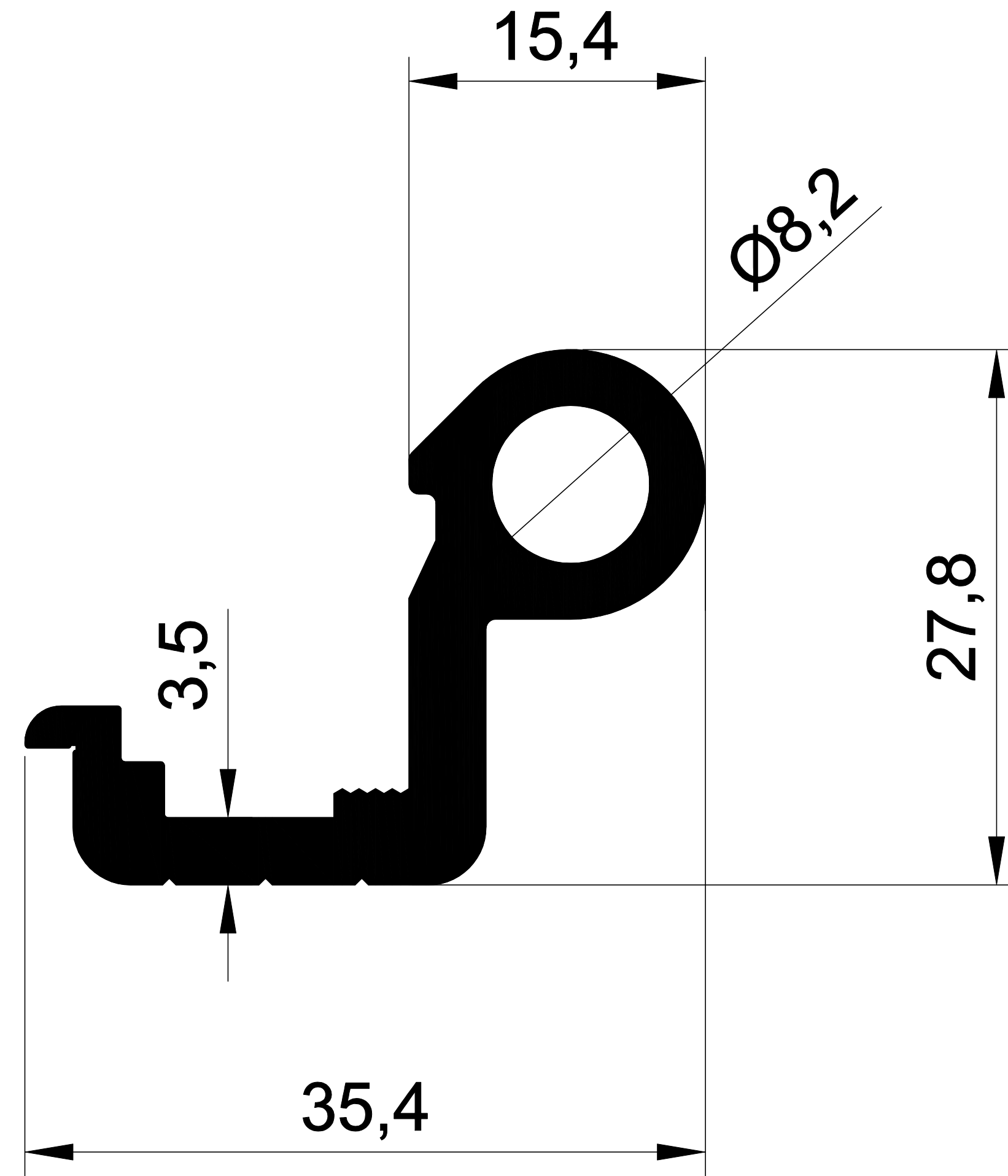
1007 0,713 Kg/m.
