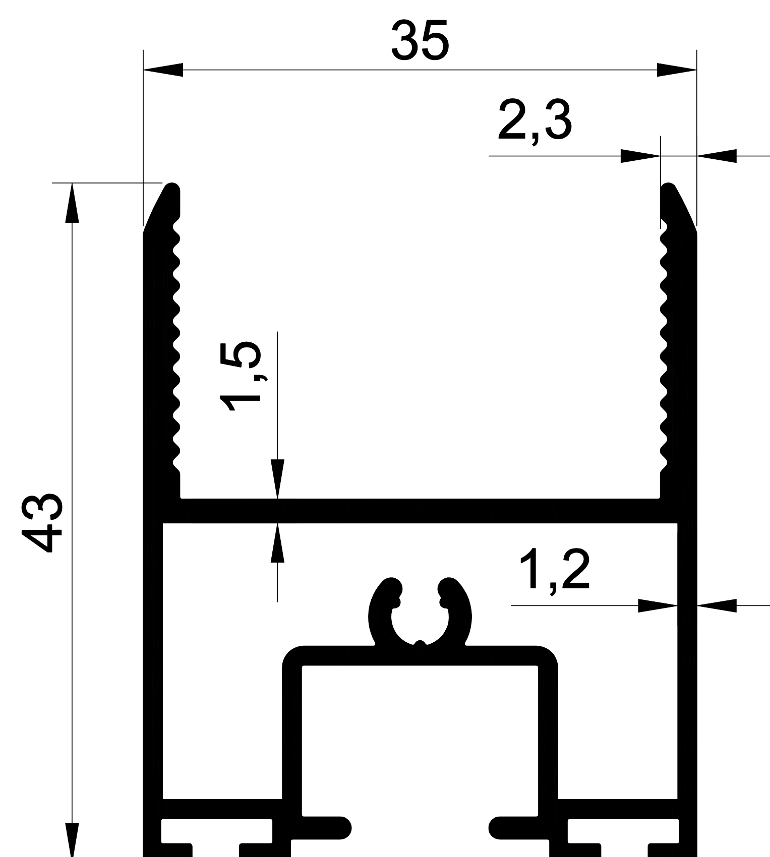
- 2303 0,442 gr/m ISICAMLI CAM BALKON PROFİLLERİ
