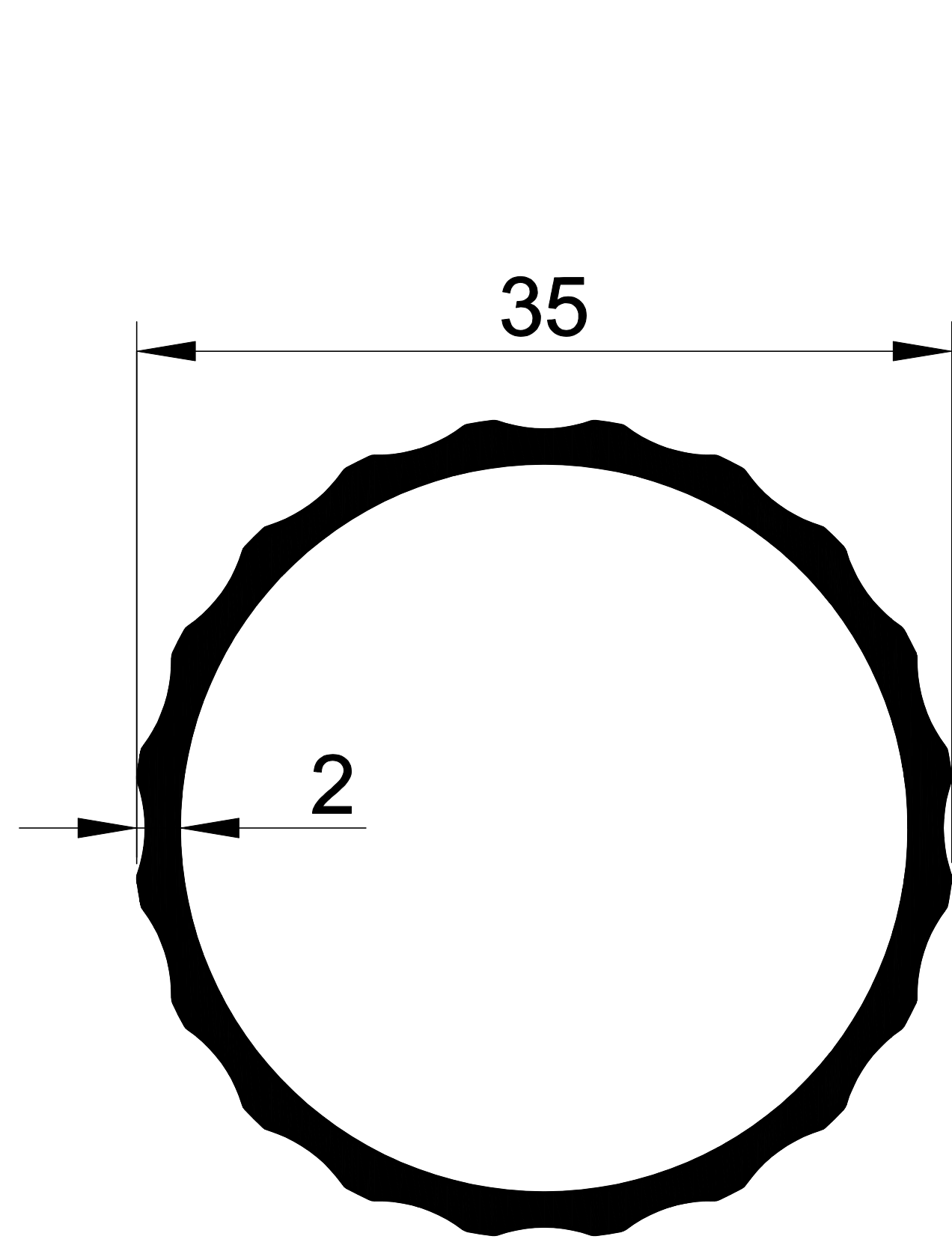
1162 0,486 Kg/m.
