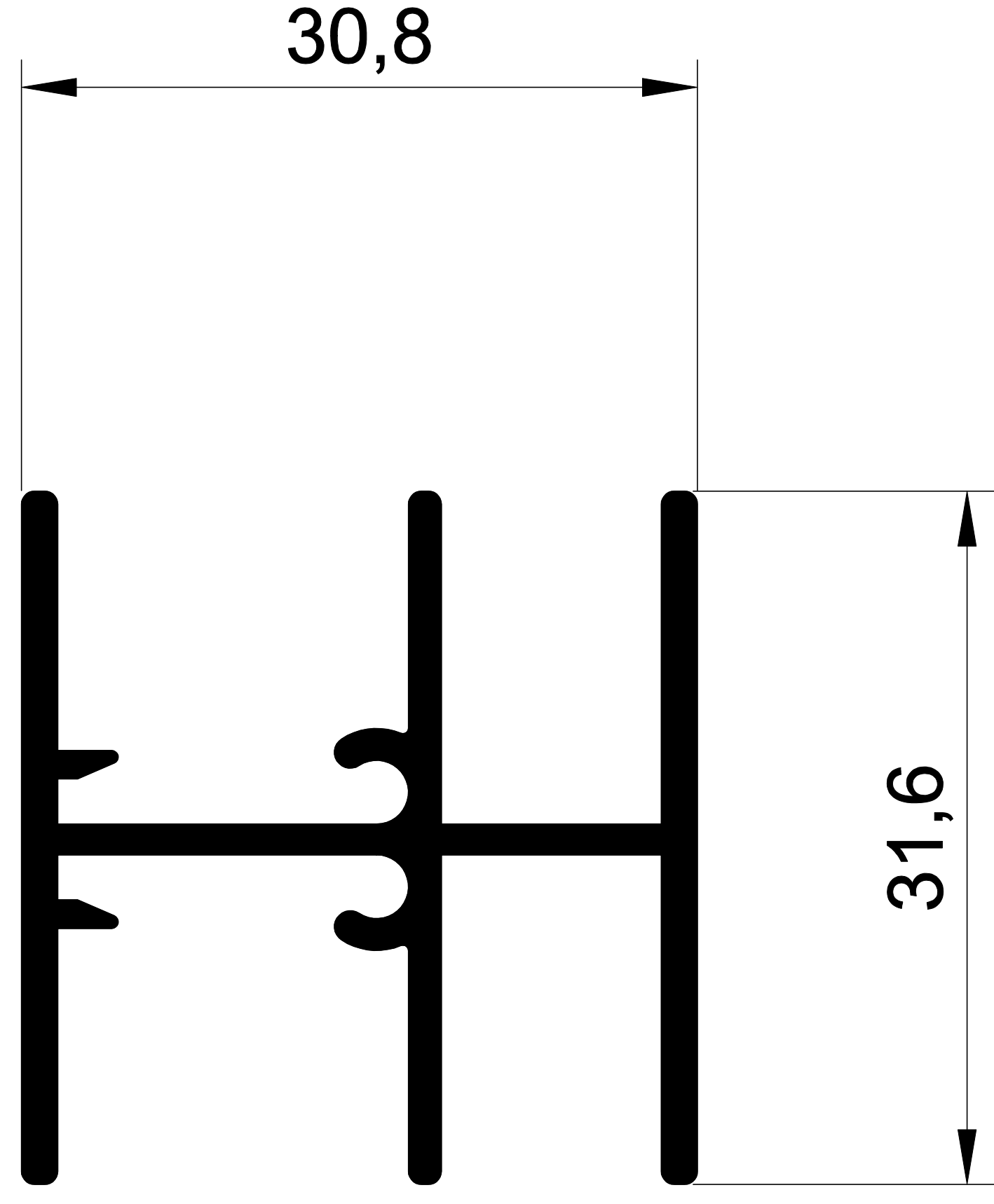
1156 0,550 Kg/m. MEBO ORTA
