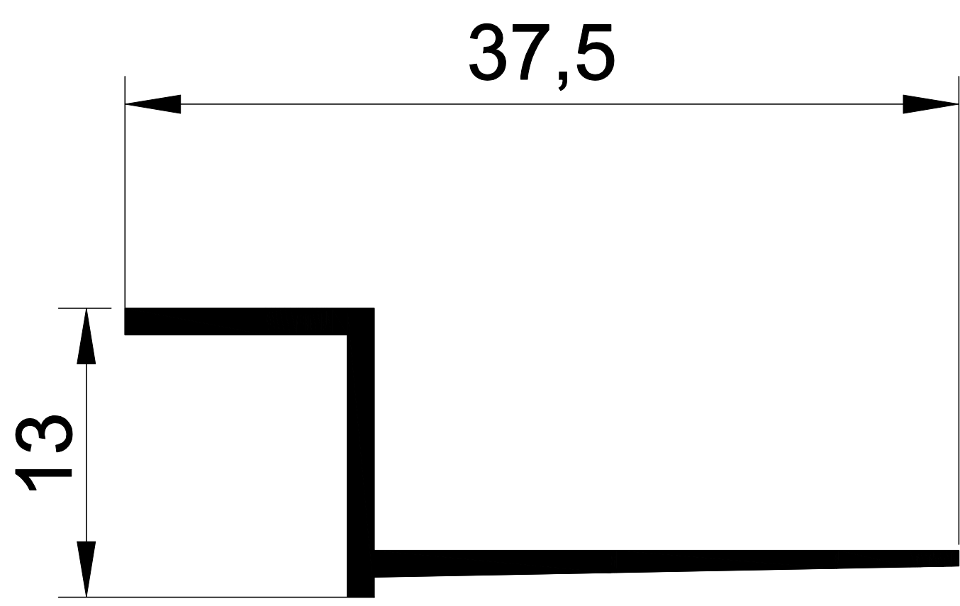
1147 0,144 Kg/m.
