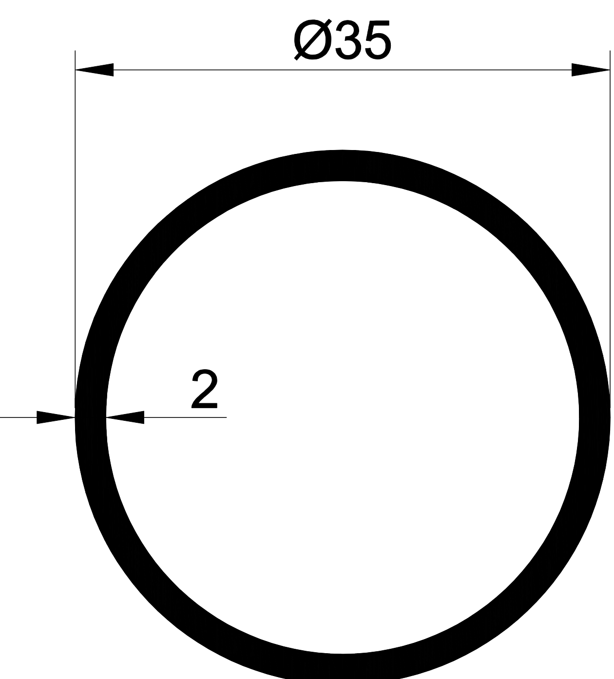
1070-B 0,561 Kg/m.
