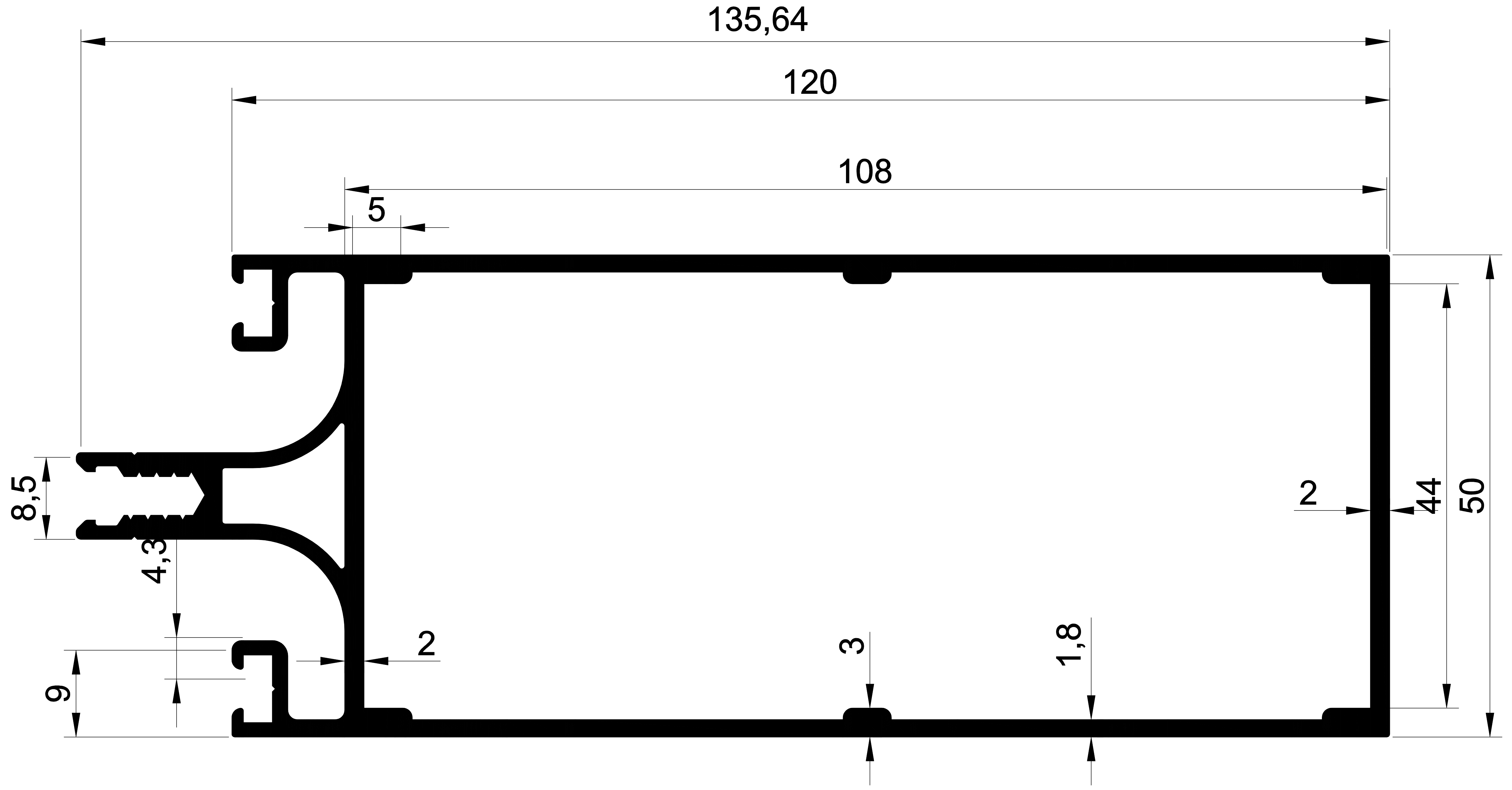
1438 2,219 Kg/m. 120'LİK CEPHE PROFİLİ UZUN GAGA
