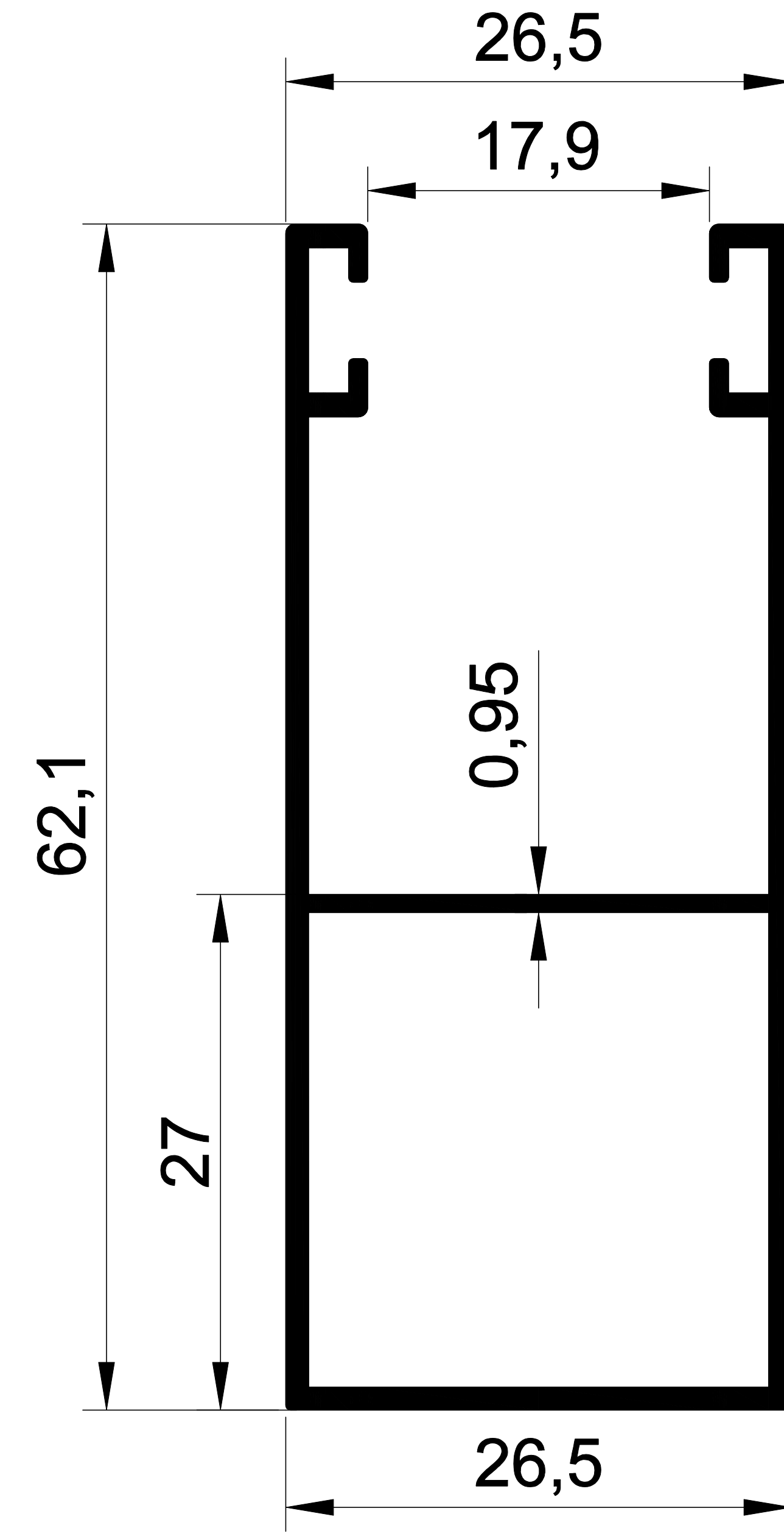
1308 0,604 Kg/m. 63'LÜK DİKME
