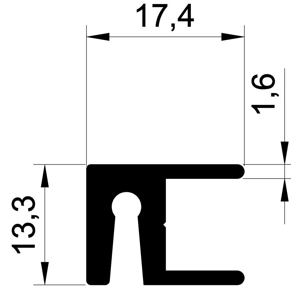
1155 0,298 Kg/m. MEBO ÇITA
