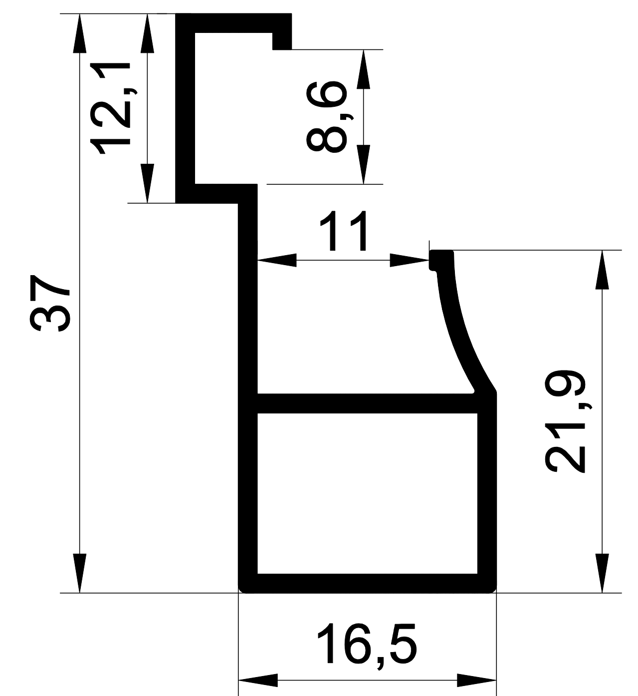
GİZLİ VİDALI MİNİ GEMİCİ 1458 0,320 Kg/m
