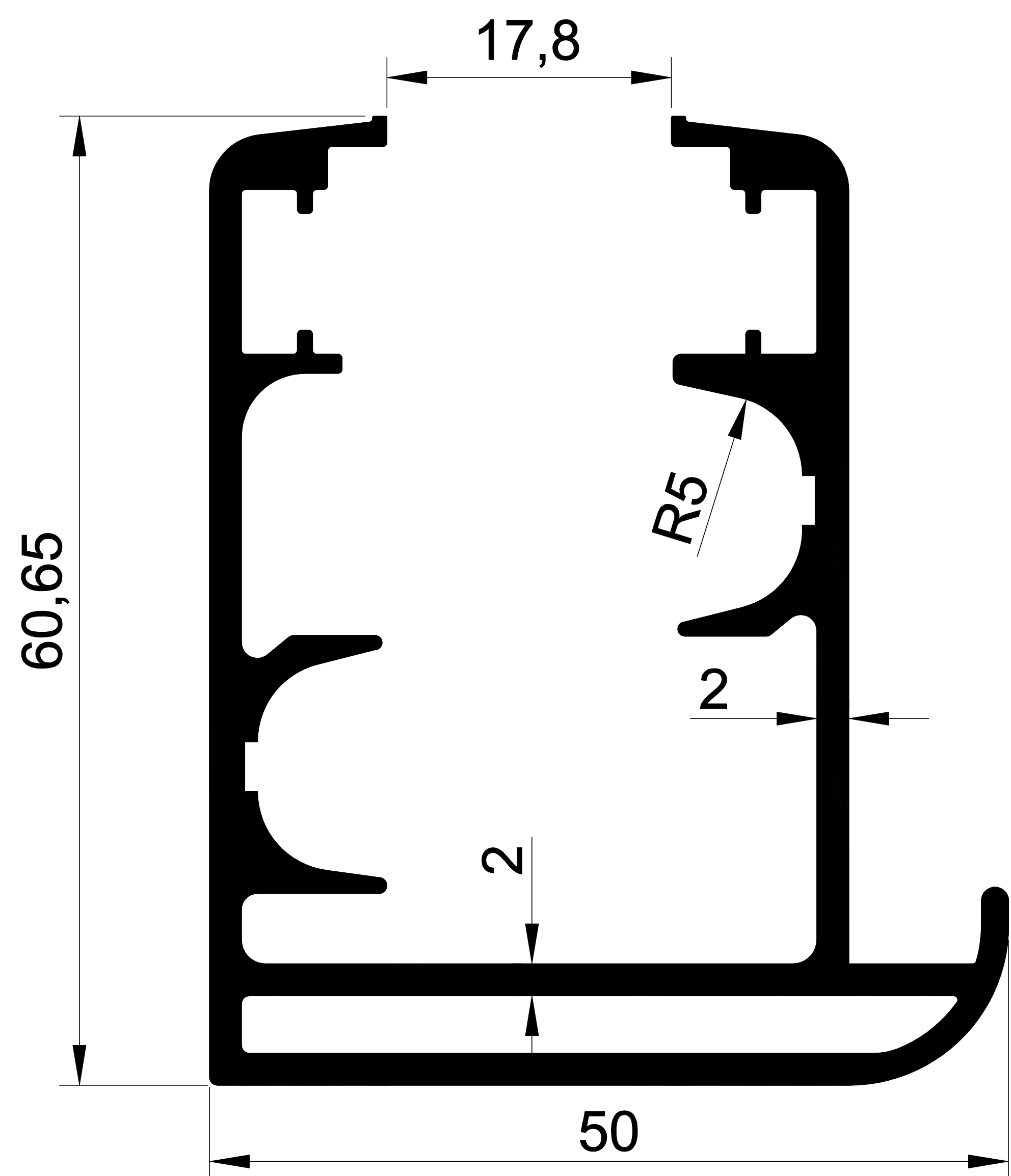
1271 1,561 Kg/m. FIRTINA DAMLALIKLI KASA
