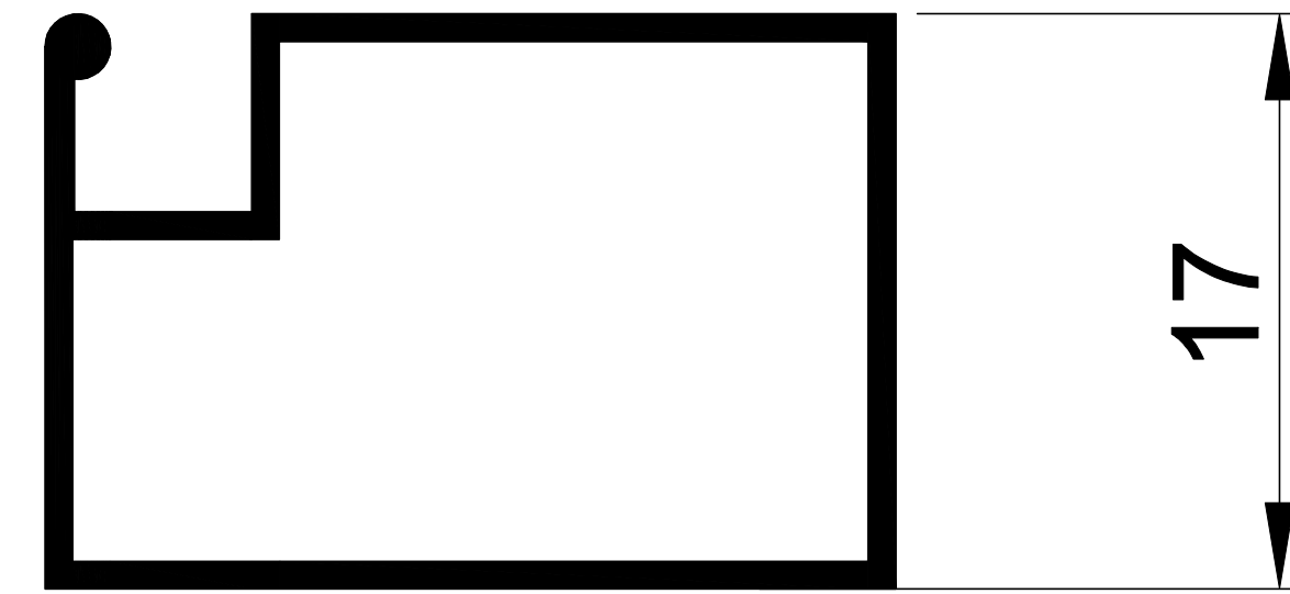
1072 0,169 Kg/m. 17*25 SİNEKLİK
