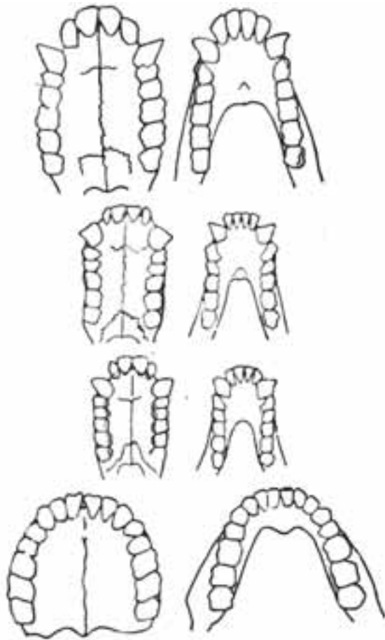
Fig. 11.5. Comparación de los arcos dentarios maxilar y mandibular. De arriba hacia abajo: chimpancé, gorila, orangután y hombre.
