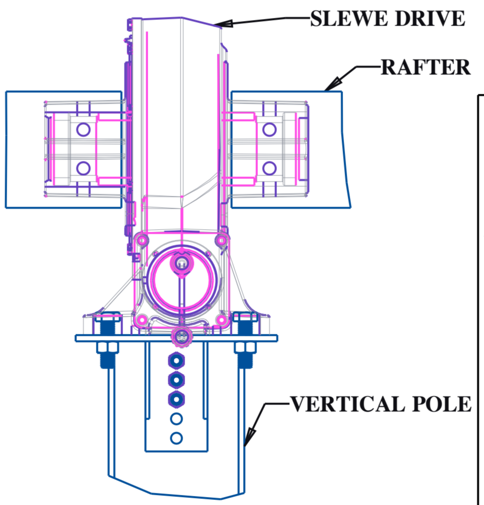
DETAIL : C
