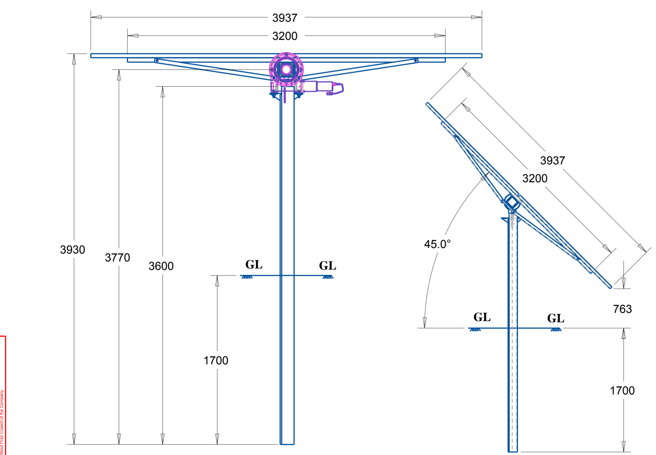
DETAIL : A
