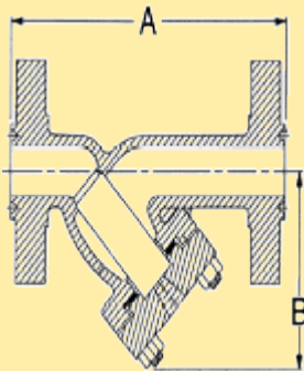
S8-1500/S8-2500
