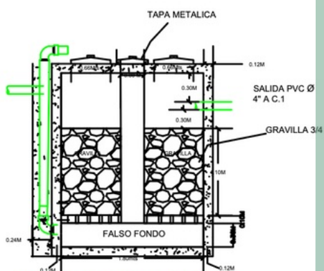
PERFIL FILTRO ANAEROBIO DE FLUJO ASCENDENTE ESC 1_15
