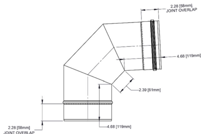
87° ELBOW
