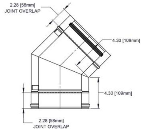
45° ELBOW
