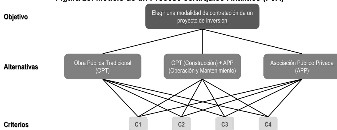
Figura 15: Modelo de un Proceso Jerárquico Analítico (PJA)
