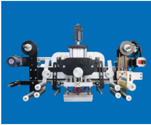
HOT STAMPING MODULE
