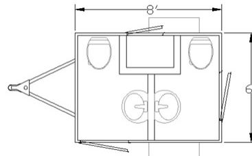
Petite Suite Layout
