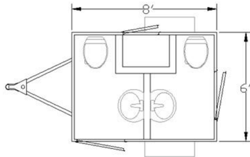
Petite Suite 2-Stall Layout
