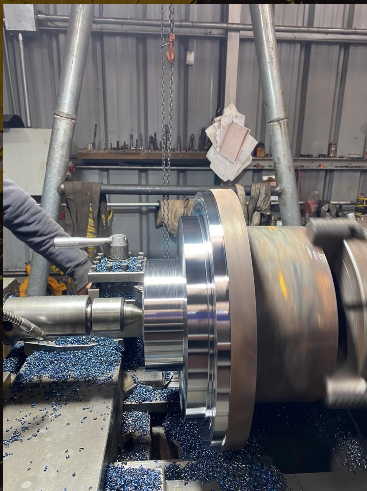
Fabricación Eje Cabezal Peletera
