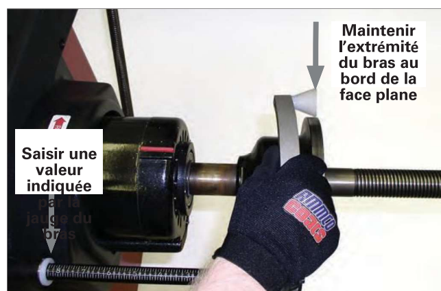
Figure 3 – En maintenant le bras sur le bord de la face plane, saisir A
