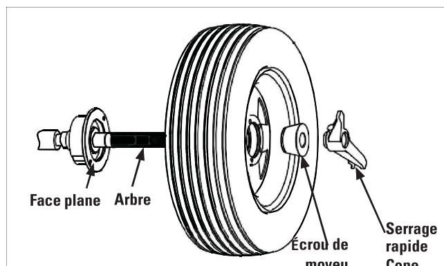
Figure 17 - Montage du cône avant standard
