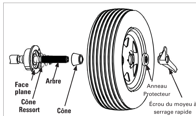
Figure 18 - Montage alternatif
