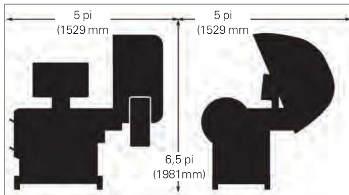
Figure 1 – Espace nécessaire
