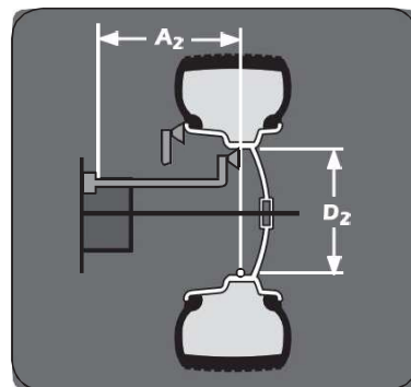
Figure 21 - Dimensions A2 et D2 de pneu
