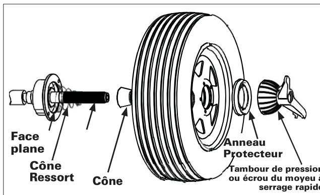
Figure 16 - Montage du cône arrière standard
