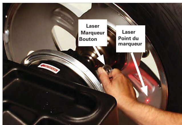
Figure 10 – Positionnement du point du laser à l'emplacement du poids Adhésif T2 caché (A2)
