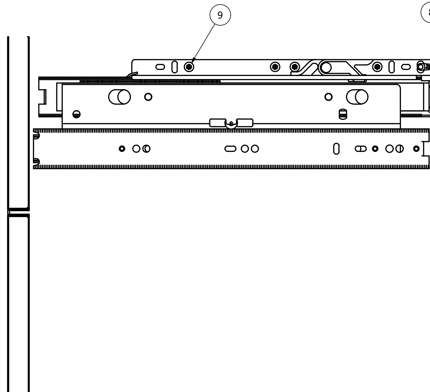
SECTION D-D SCALE 1 : 2
