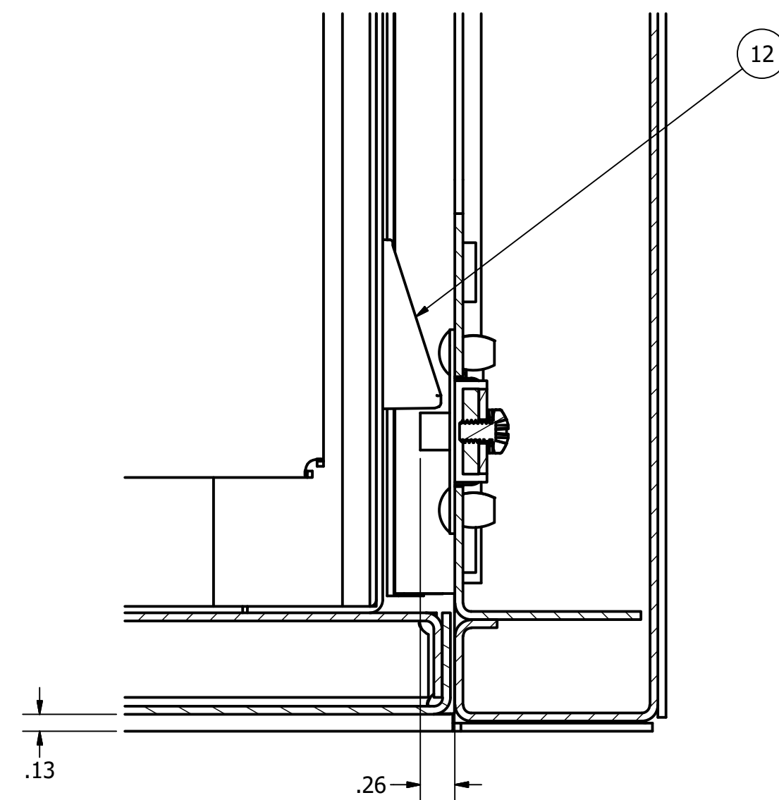
SECTION D-D SCALE 1 : 1
