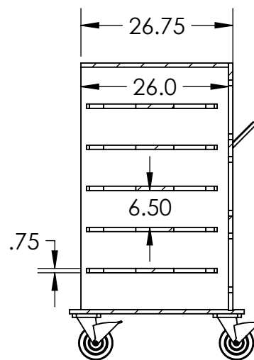
SECTION A-A SCALE 1 : 24
