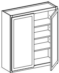
Double Door 42" Height 24", 27", 30", 33", 36", *39" or *42" Width
