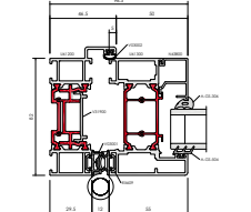
F82 Jamb
