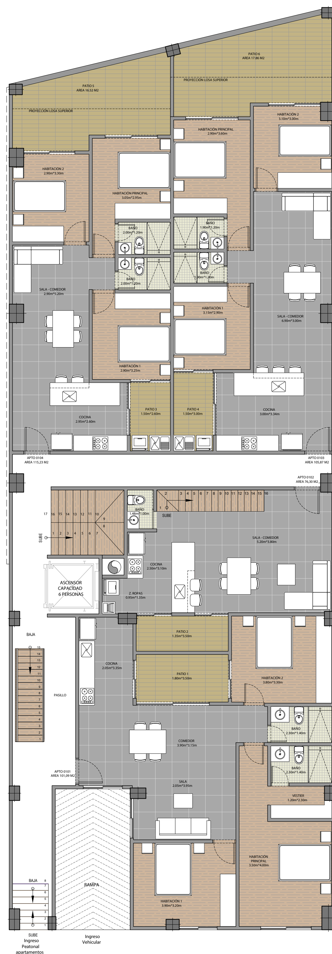
PLANTA PRIMER PISO
