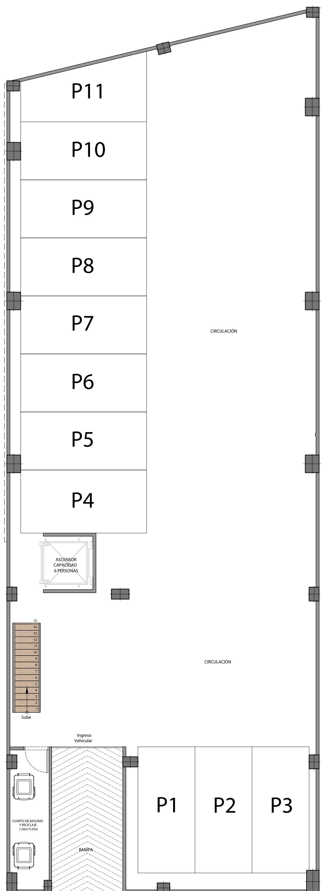
PLANTA SEMISÓTANO
