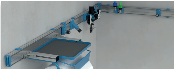
MULTIFUNCTION SYSTEM WITH DOUBLE DISTRIBUTION DUCT SISTEMA MULTIFUNZIONE CON DOPPIO CANALE DI DISTRIBUZIONE
