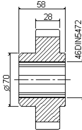
S5/060 Z51 gear SD50d690a
