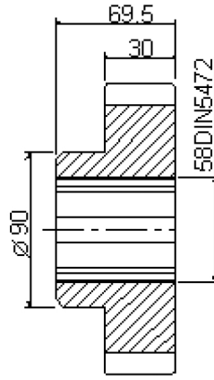
S7/054 Z52 gear 685
