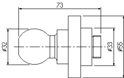
S5/039 pivot
