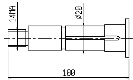
S5/034P pin
