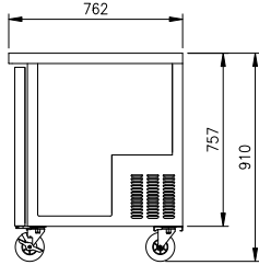
DOOR MODEL
