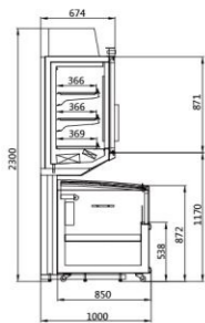
悉尼子母柜
