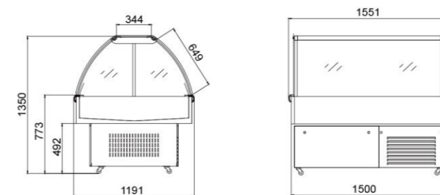
双面熟食柜
