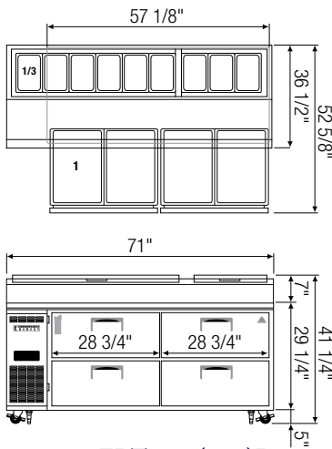
▲ EPT180-(800)D4
