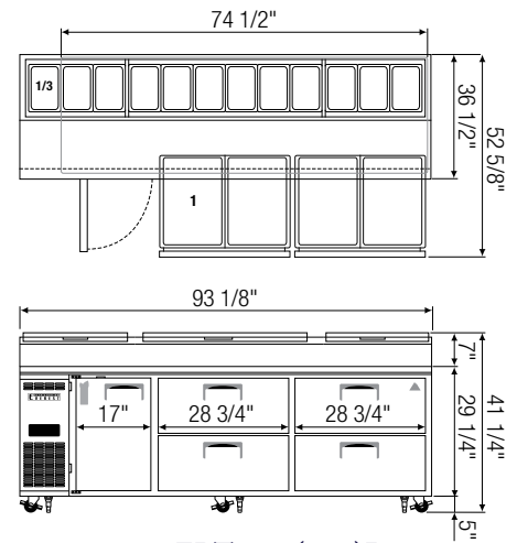
▲ EPT240-(800)D4
