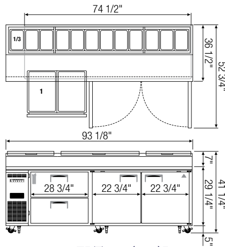
▲ EPT240-(800)D2
