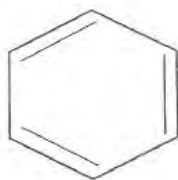
BENZENE
