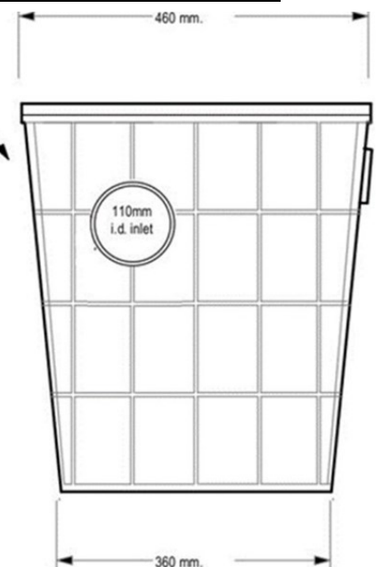
End Elevation
