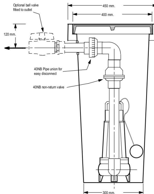
End Elevation
