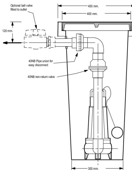
End Elevation
