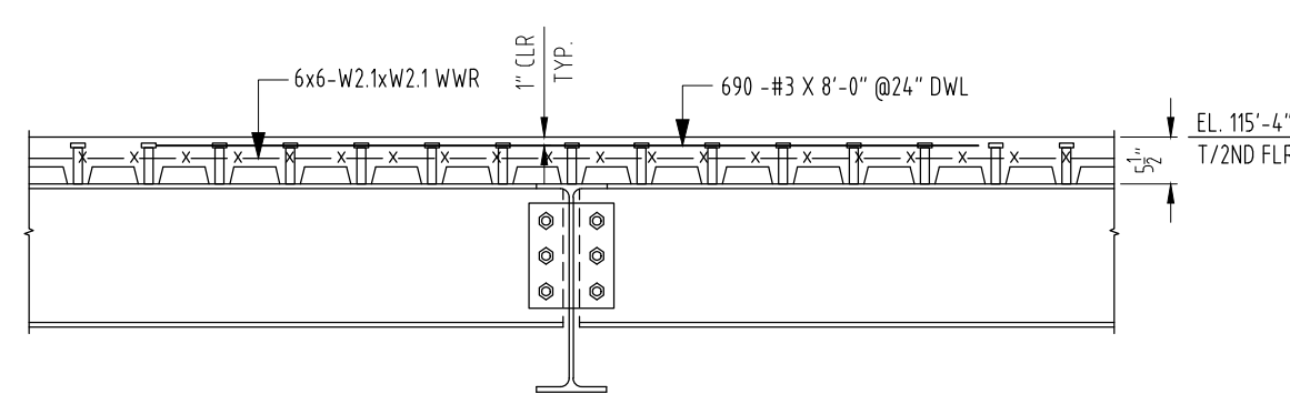
SECTION 10 SCALE: 1/2"=1'-0" SDR: 5/55.62
