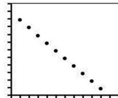
Correlação perfeita
