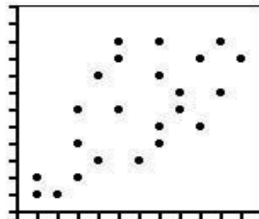
Correlação fraca
