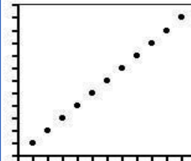
Correlação perfeita
