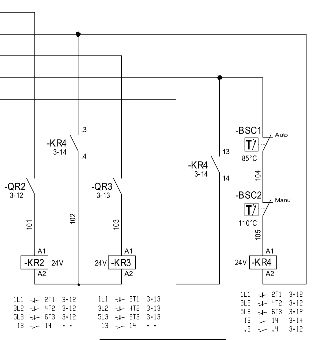
Batterie 2 étages Step 2 electric heater
