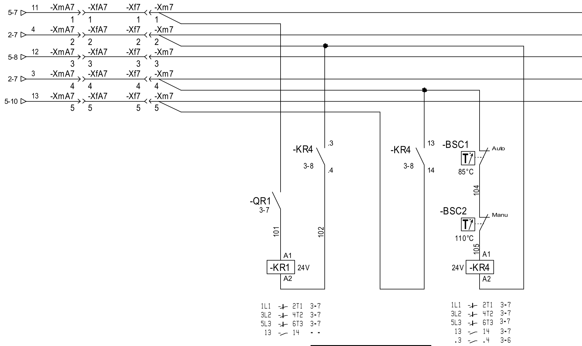
Batterie 1 étage Step 1 electric heater
