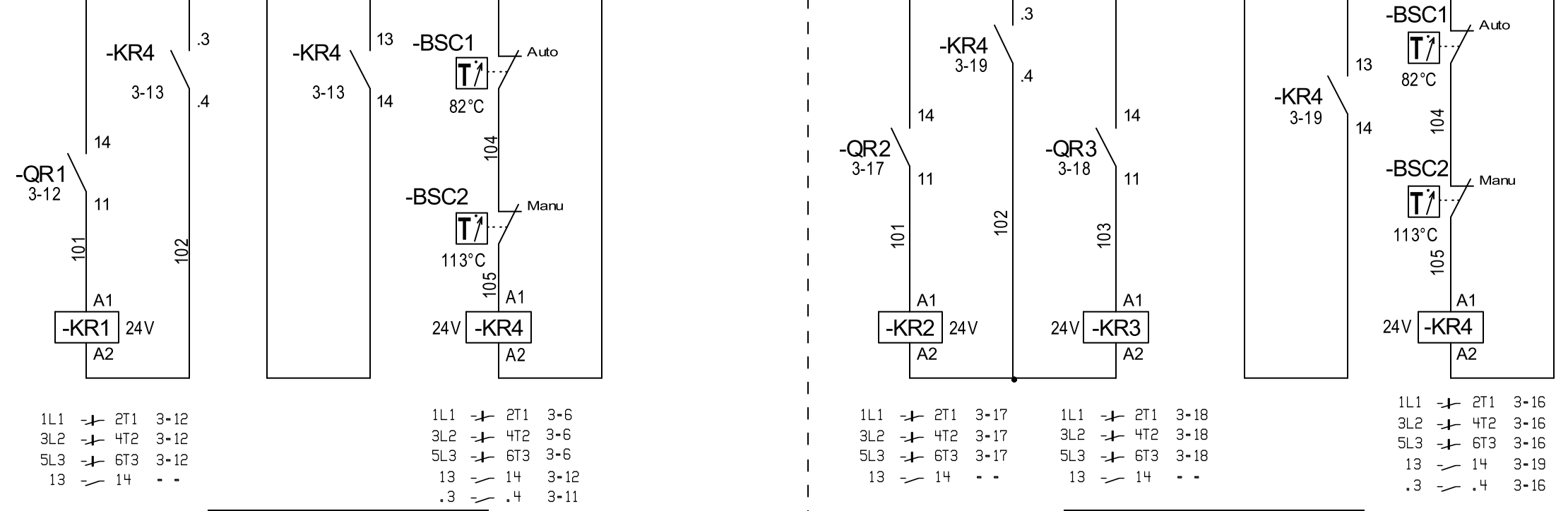
Batterie 1 étage Step 1 electric heater
