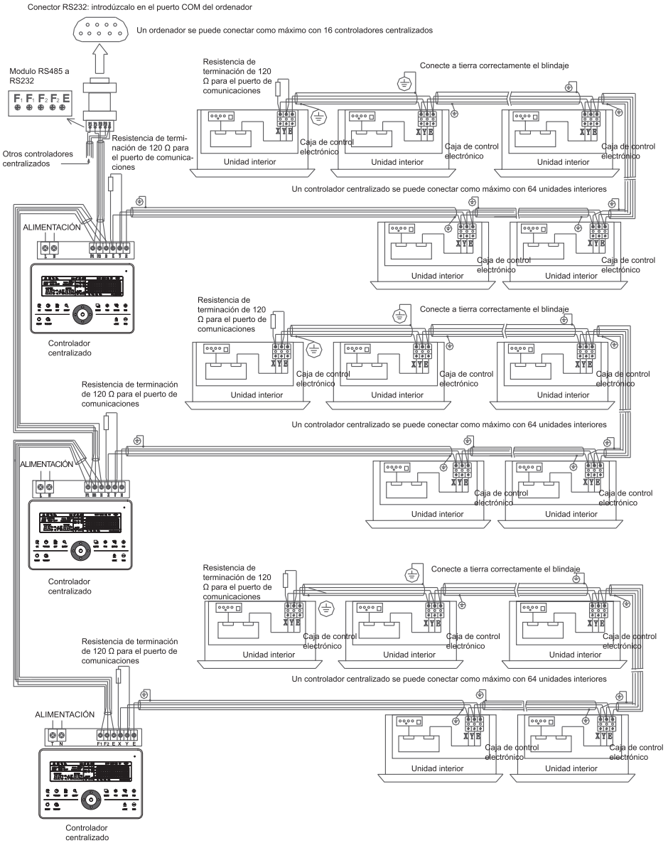
Fig. 1.4 Diagrama de instalación eléctrica
