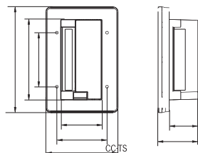
Fig. 1.1 Dimensiones del controlador centralizado (unidades: mm)
