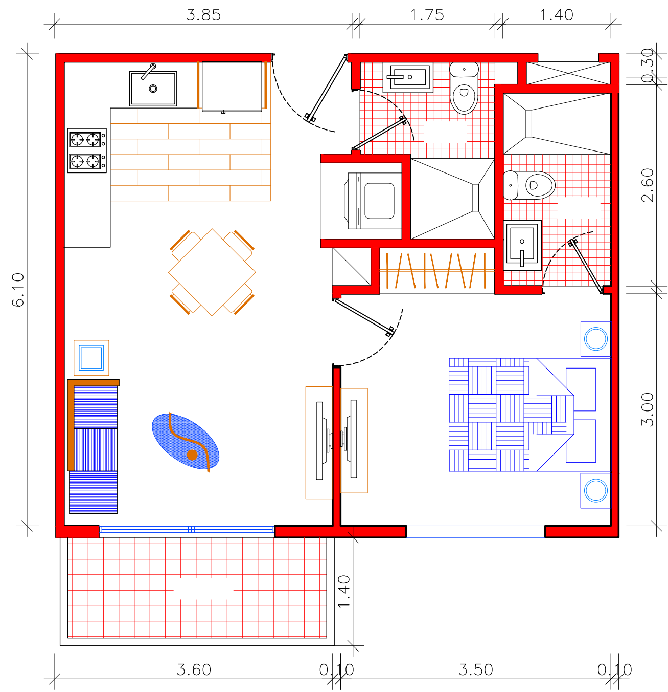
1 A1H PLANTA ARQ. AMUEBLADA 1er NIVEL APTO. TIPO 1-HABITACION ESCALA 1:50 50.00 MTS2 DE APTO.
