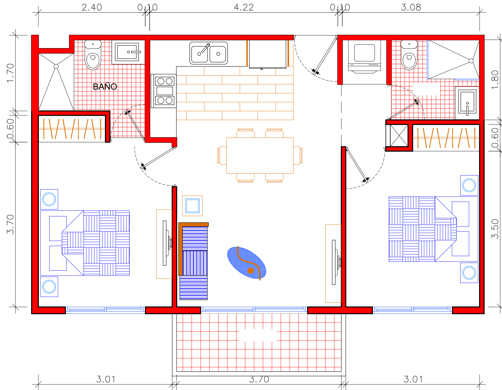
1 PLANTA ARQ. AMUEBLADA 1er NIVEL APTO. TIPO 2-HABITACIONES A2H ESCALA 1:50 68.28 MTS2 DE APTO.
