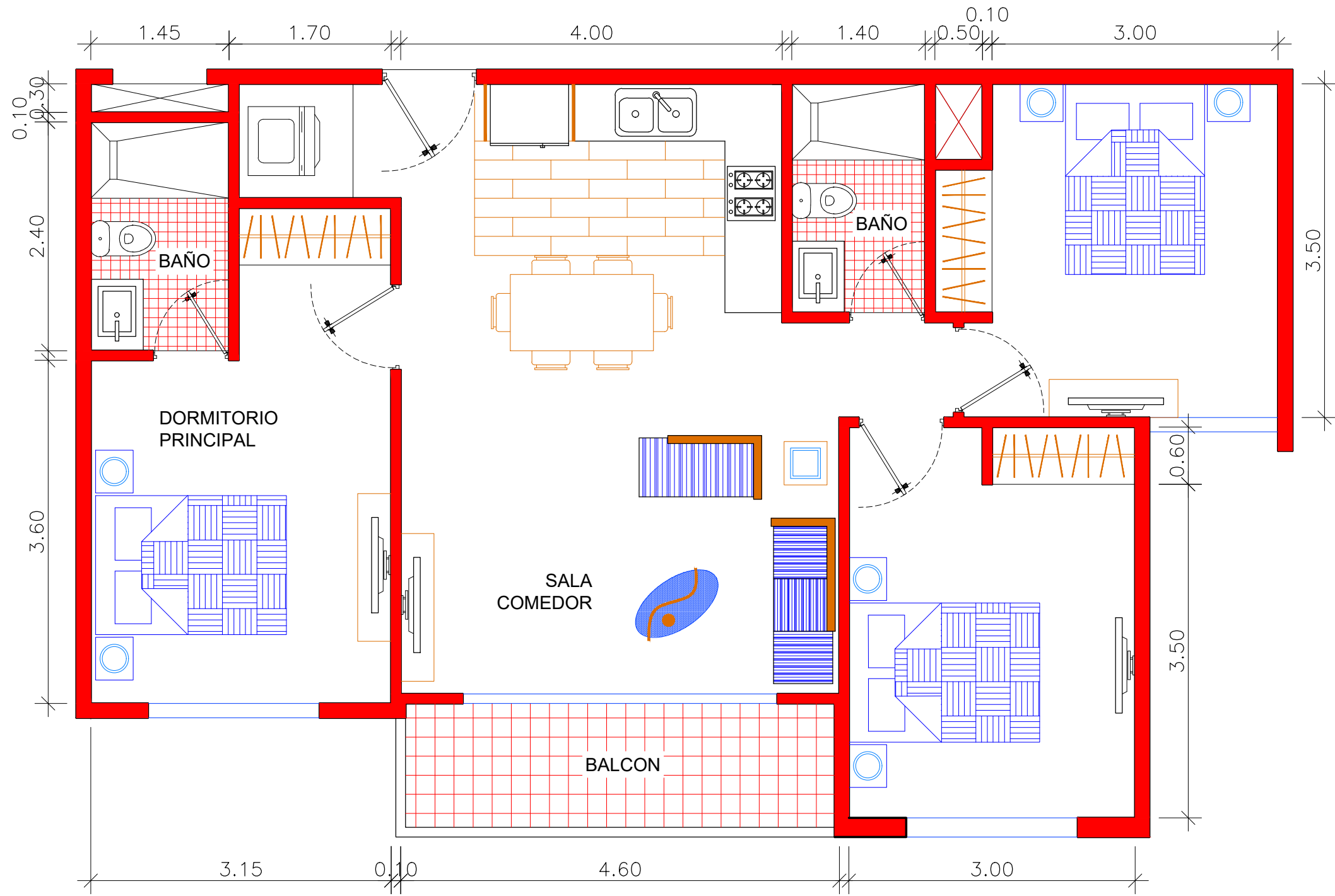
1 A3H PLANTA ARQ. AMUEBLADA 1er NIVEL APTO. TIPO 3-HABITACIONES ESCALA 1:50 91.80 MTS2 DE APTO.
